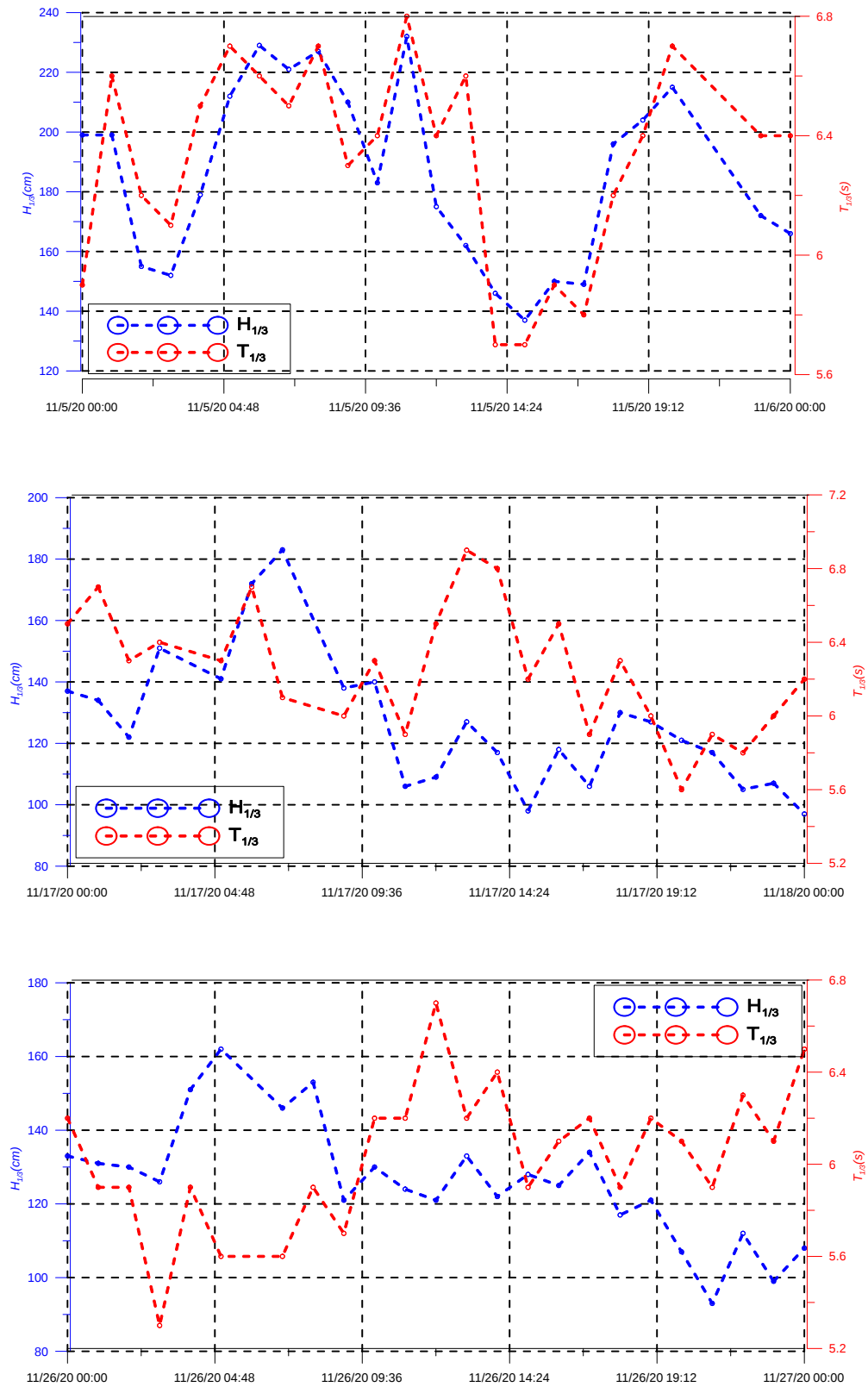
圖 2-3 波浪時序列變化圖
