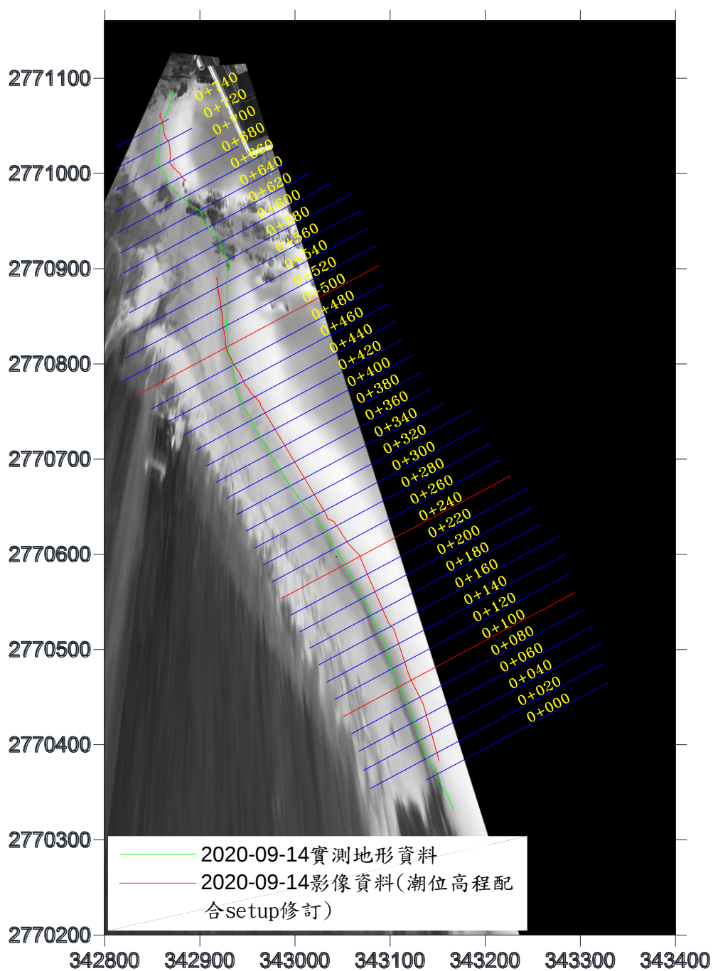
圖 3-22 水位線分析結果圖(2020/9/14)
