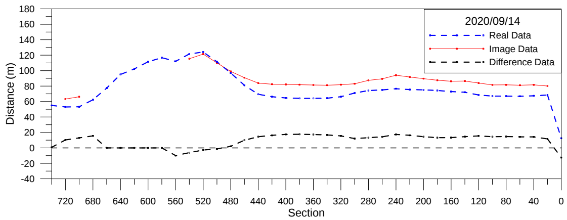
圖 3-23 海岸線分析比較圖(2020/9/14)
