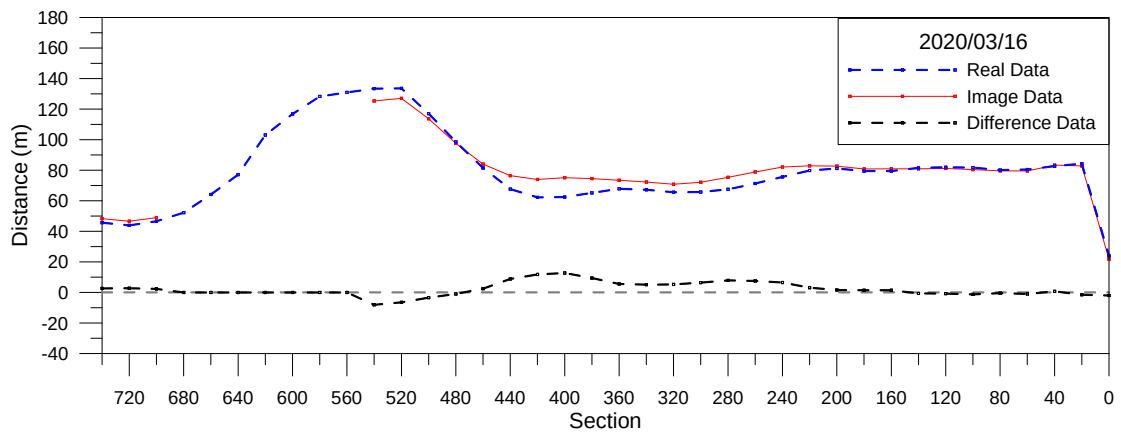
圖 3-23 海岸線分析比較圖(2020/3/16)
