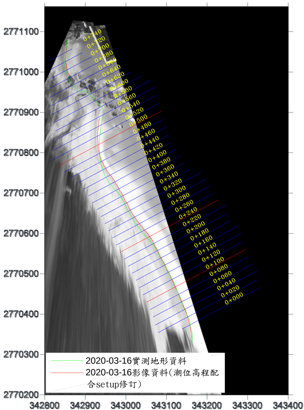
圖 3-22 水位線分析結果圖(2020/3/16)
