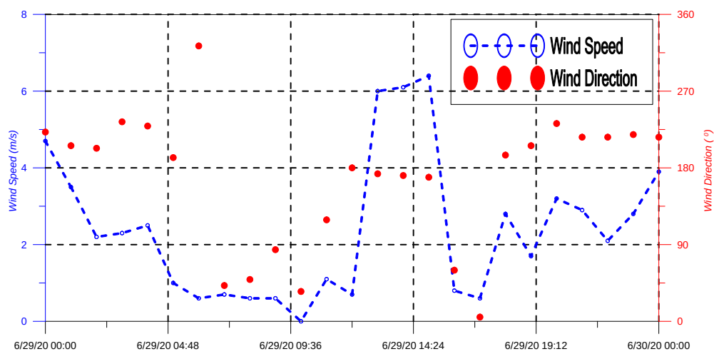
圖 2-2 風速風向時序列變化圖
