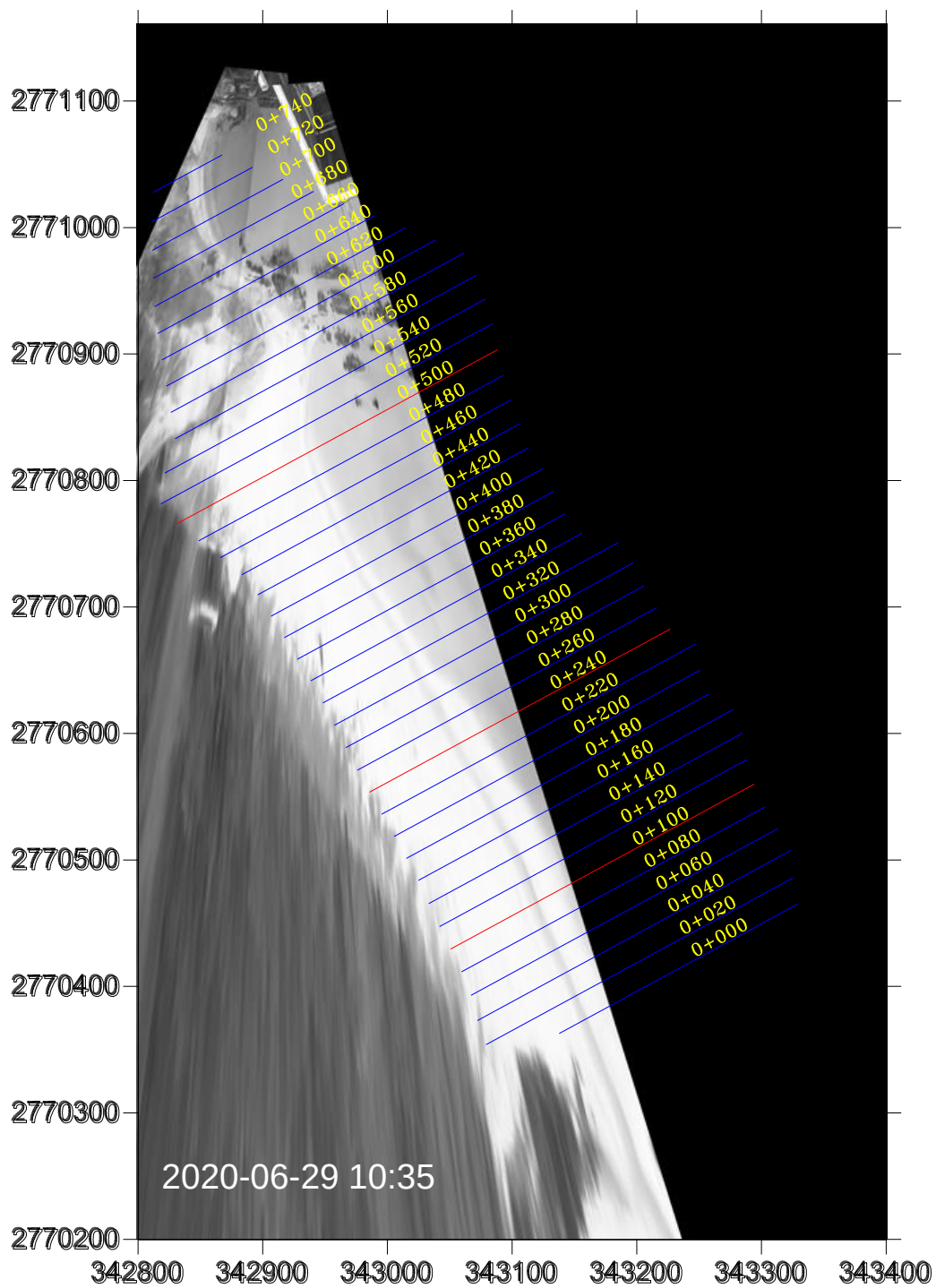
圖 4-14 鹽寮海岸地形影像全景圖(2020/06/29 10 : 35)
