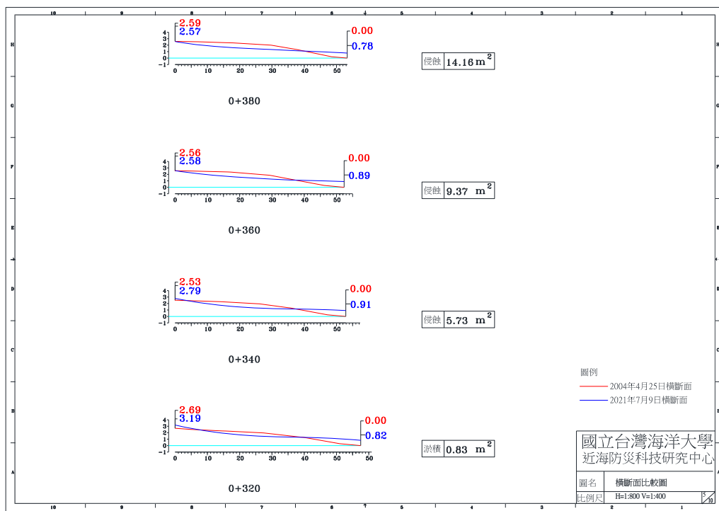
圖 4-4(f) 2021 年 7 月 9 日 A 監測區橫斷面比較圖
