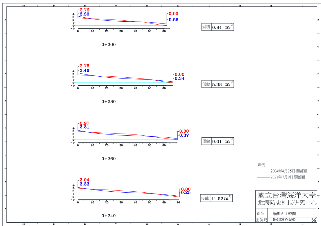
圖 4-4(g) 2021 年 7 月 9 日 A 監測區橫斷面比較圖
