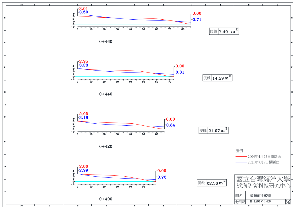
圖 4-4(e) 2021 年 7 月 9 日 A 監測區橫斷面比較圖
