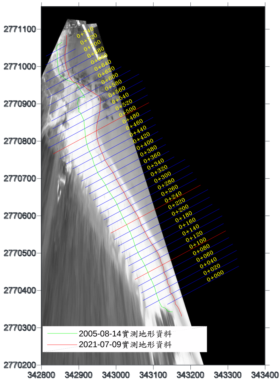
圖 4-22 實測地形水位線分析結果圖(2021/07/09)
