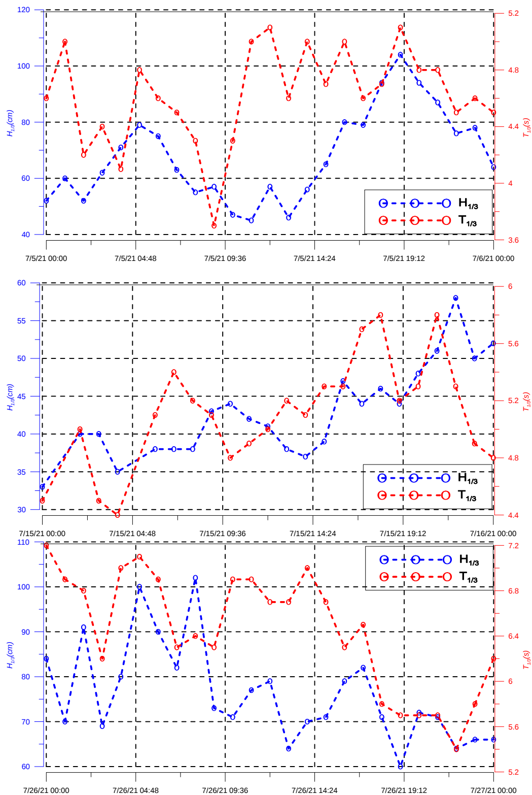
圖 2-3 波浪時序序列變化圖
