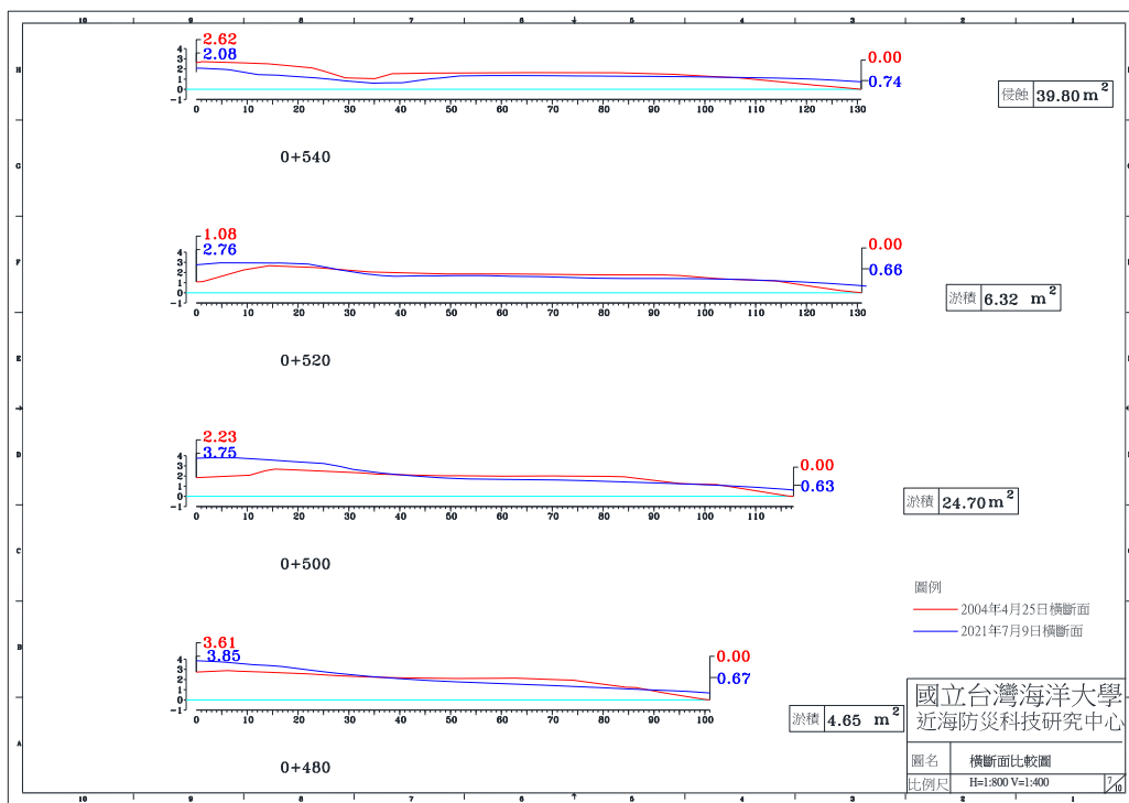
圖 4-4(d) 2021 年 7 月 9 日 A 監測區橫斷面比較圖
