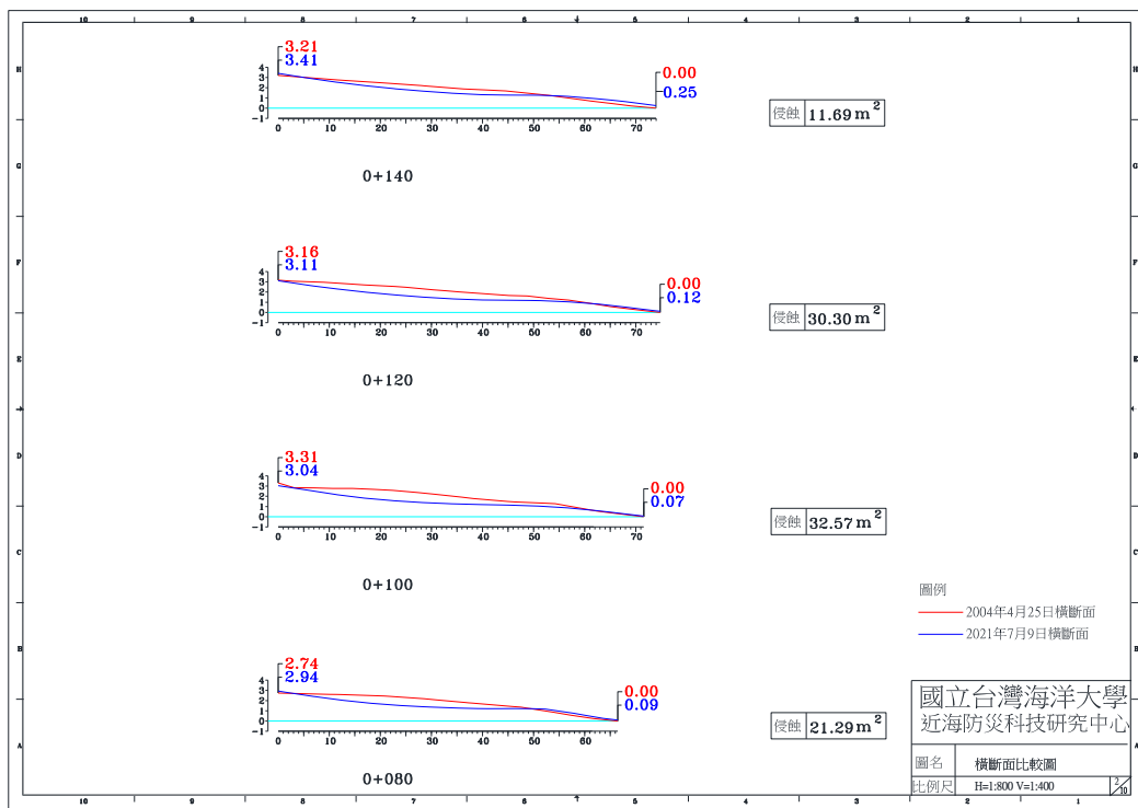
圖 4-4(i) 2021 年 7 月 9 日 A 監測區橫斷面比較圖
