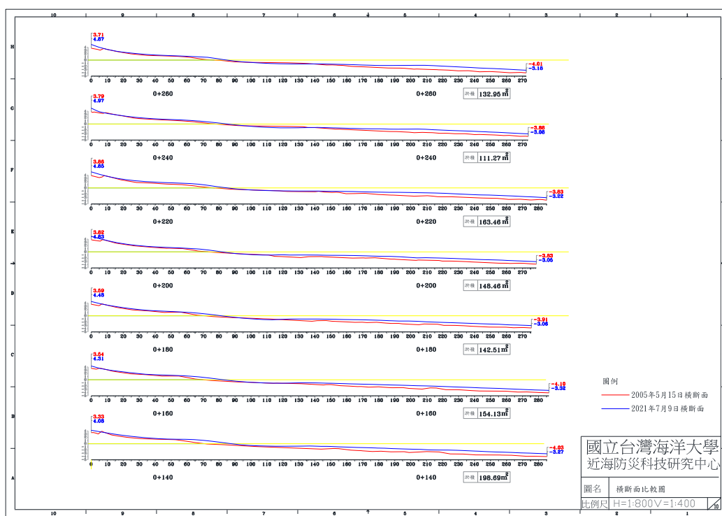
圖 4-5(e) 2021 年 7 月 9 日 B 監測區橫断面比較圖
