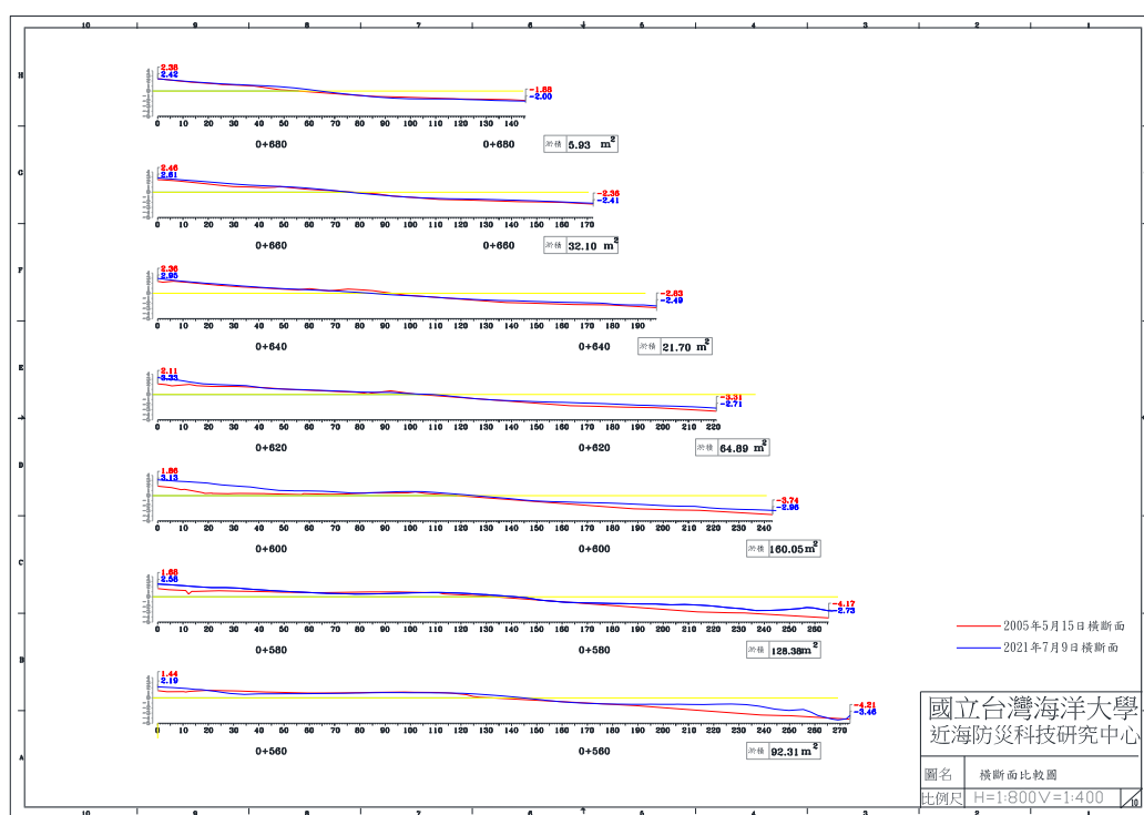
圖 4-5(b) 2021 年 7 月 9 日 B 監測區橫斷面比較圖
