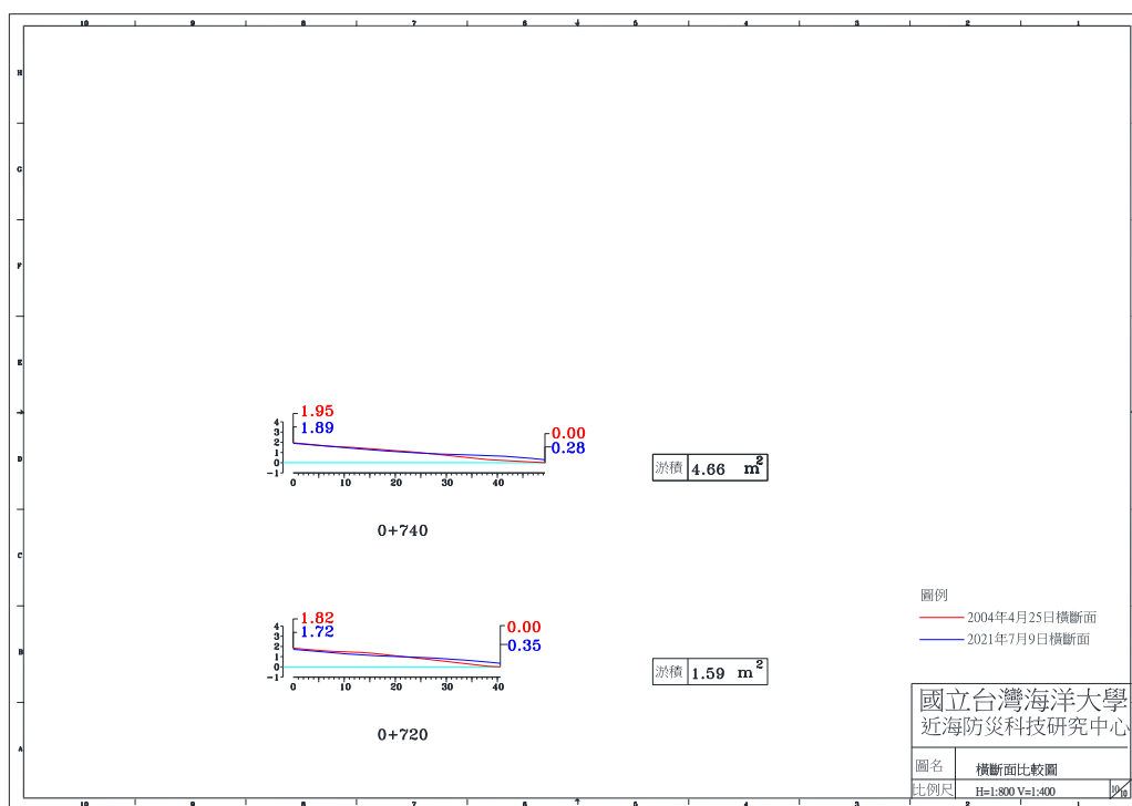
圖 4-4(a) 2021 年 7 月 9 日 A 監測區橫斷面比較圖
