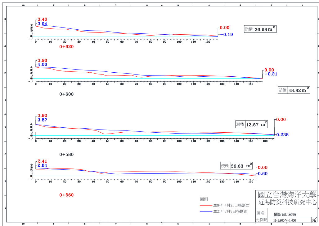
圖 4-4(c) 2021 年 7 月 9 日 A 監測區橫斷面比較圖
