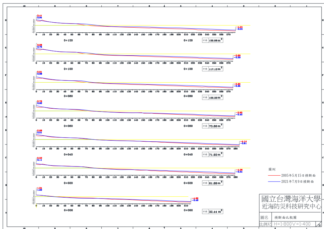
圖 4-5(f) 2021 年 7 月 9 日 B 監測區橫断面比較圖
