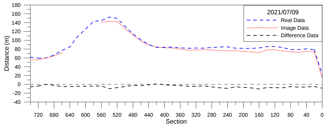
圖 3-23 海岸線分析比較圖(2021/07/09)
