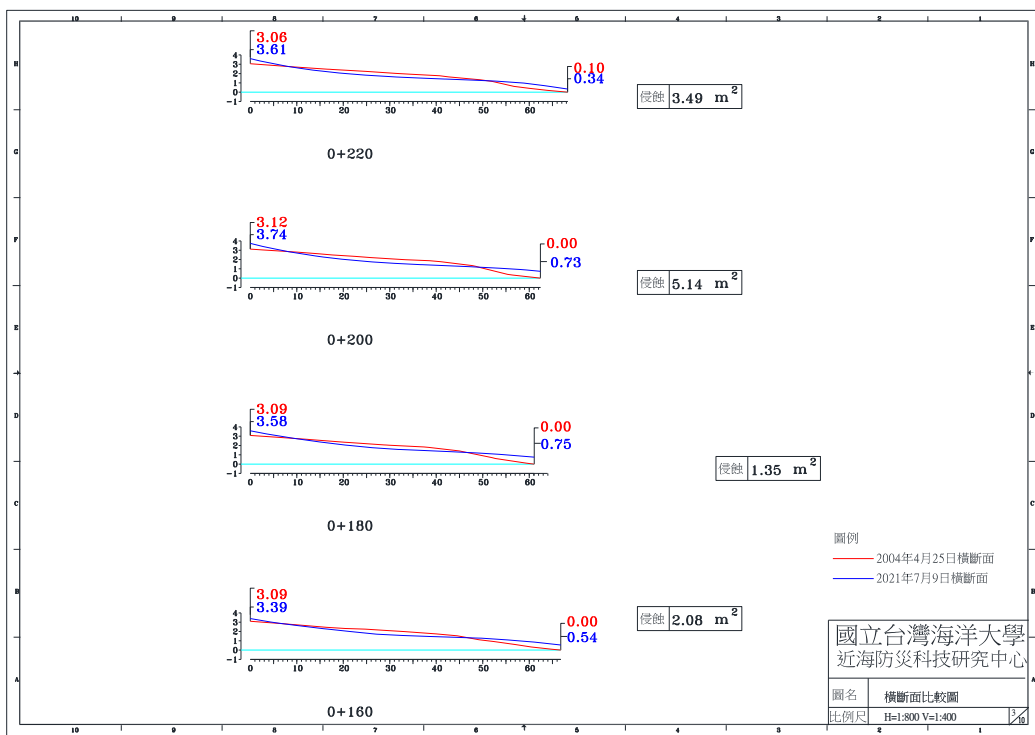
圖 4-4(h) 2021 年 7 月 9 日 A 監測區橫斷面比較圖
