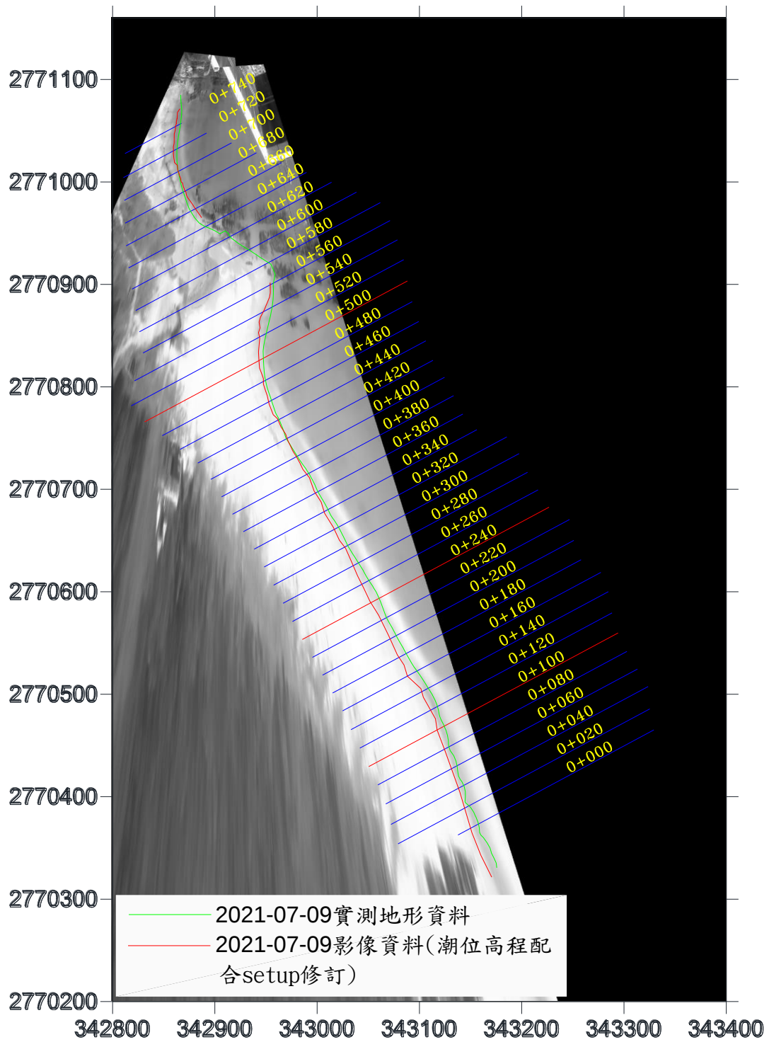
圖 3-22 水位線分析結果圖(2021/07/09)
