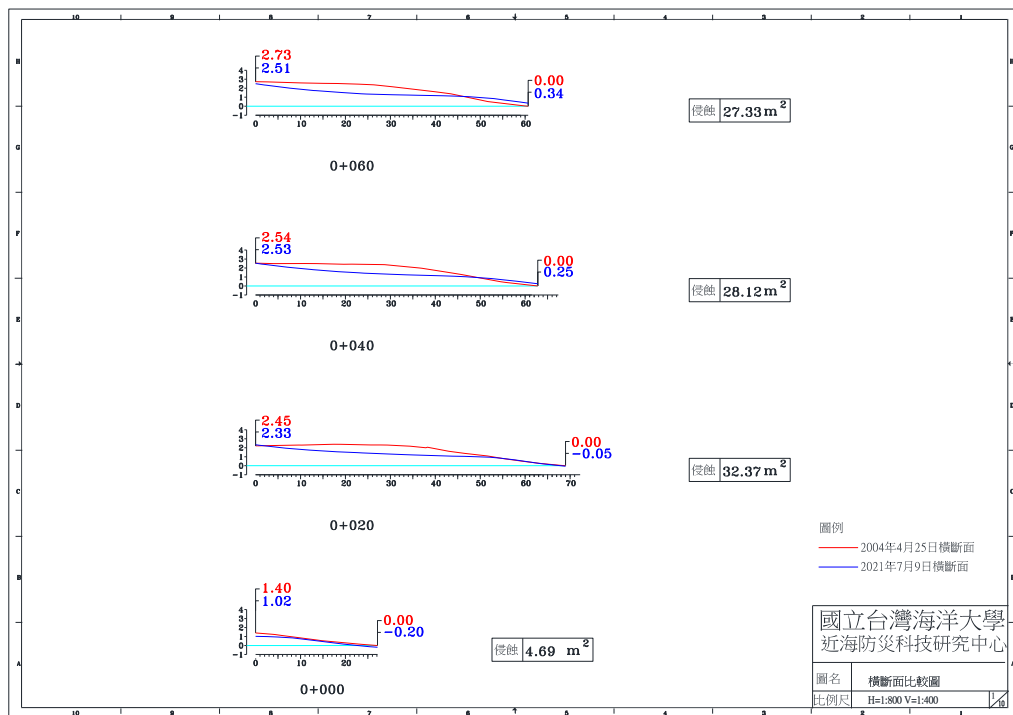
圖 4-4(j) 2021 年 7 月 9 日 A 監測區橫斷面比較圖
