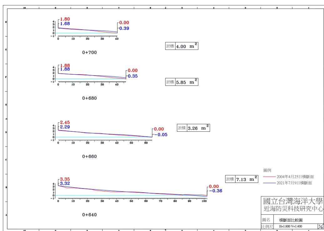
圖 4-4(b) 2021 年 7 月 9 日 A 監測區橫斷面比較圖
