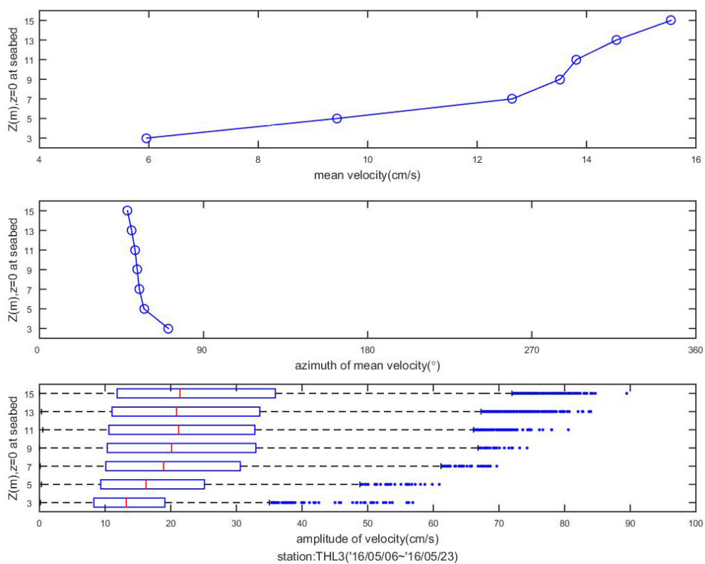
附錄III.11圖-8 THL3分層平均流速、平均流向剖面及流速振幅鬚盒圖
