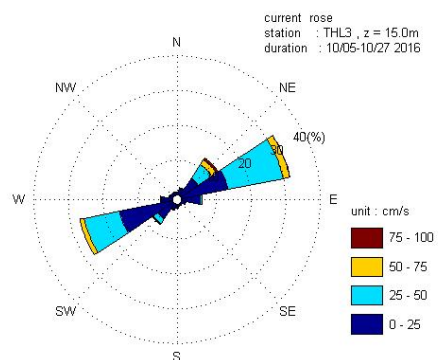
附錄III.11圖-6 THL3流速流向玫瑰圖
