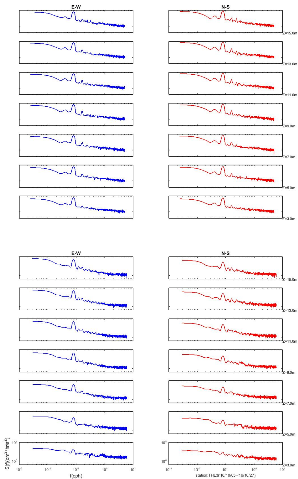
附錄III.11圖-10 流速分量能譜圖
