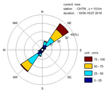
附錄III.11圖-5 CH7W流速流向玫瑰圖
