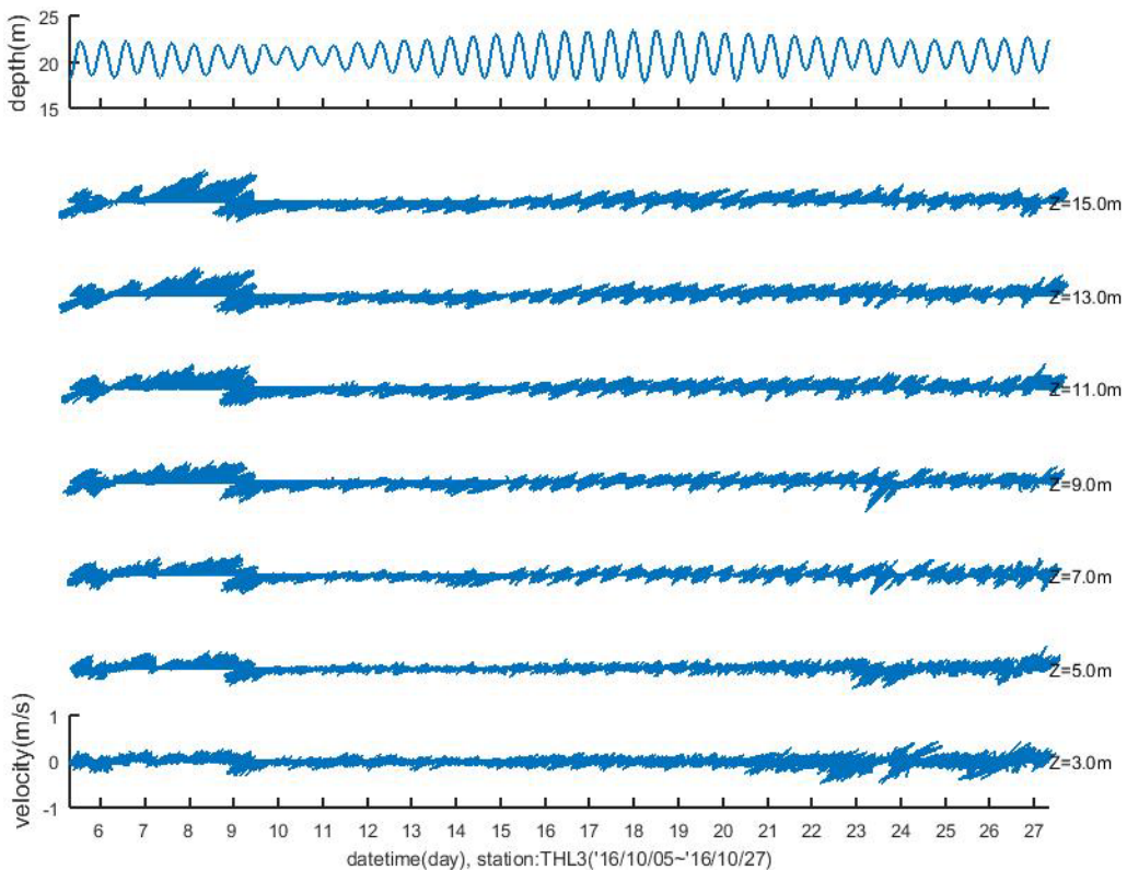
附錄III.11圖-4 THL3分層流矢圖
