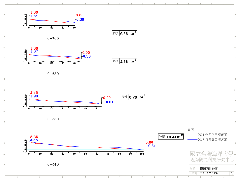
圖 4-4(b) 2017 年 8 月 29 日 A 監測區橫斷面比較圖
