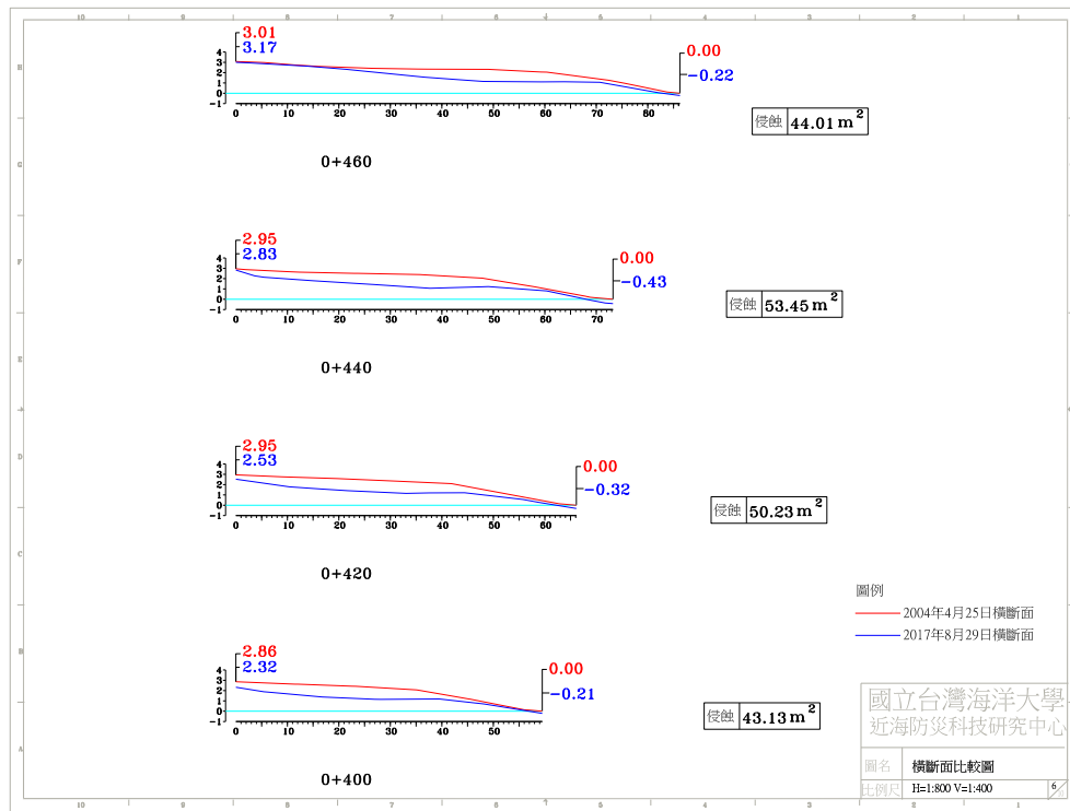
圖 4-4(e) 2017 年 8 月 29 日 A 監測區橫斷面比較圖
