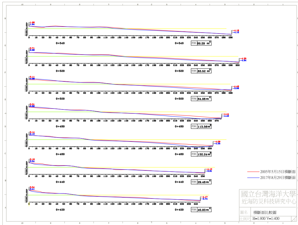
圖 4-5(c) 2017 年 8 月 29 日 B 監測區橫斷面比較圖
