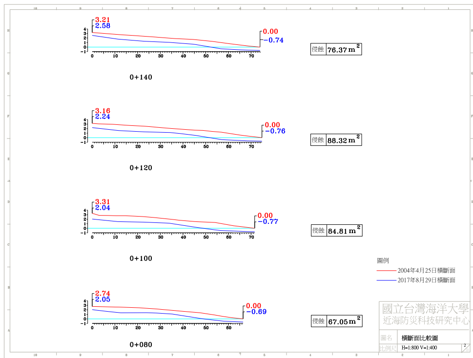
圖 4-4(i) 2017 年 8 月 29 日 A 監測區橫斷面比較圖
