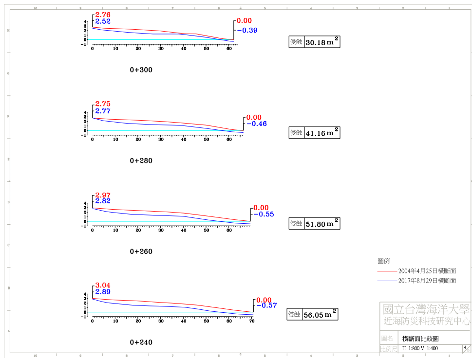
圖 4-4(g) 2017 年 8 月 29 日 A 監測區橫斷面比較圖
