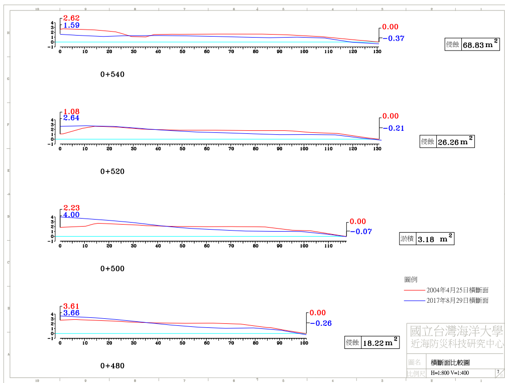
圖 4-4(d) 2017 年 8 月 29 日 A 監測區橫斷面比較圖
