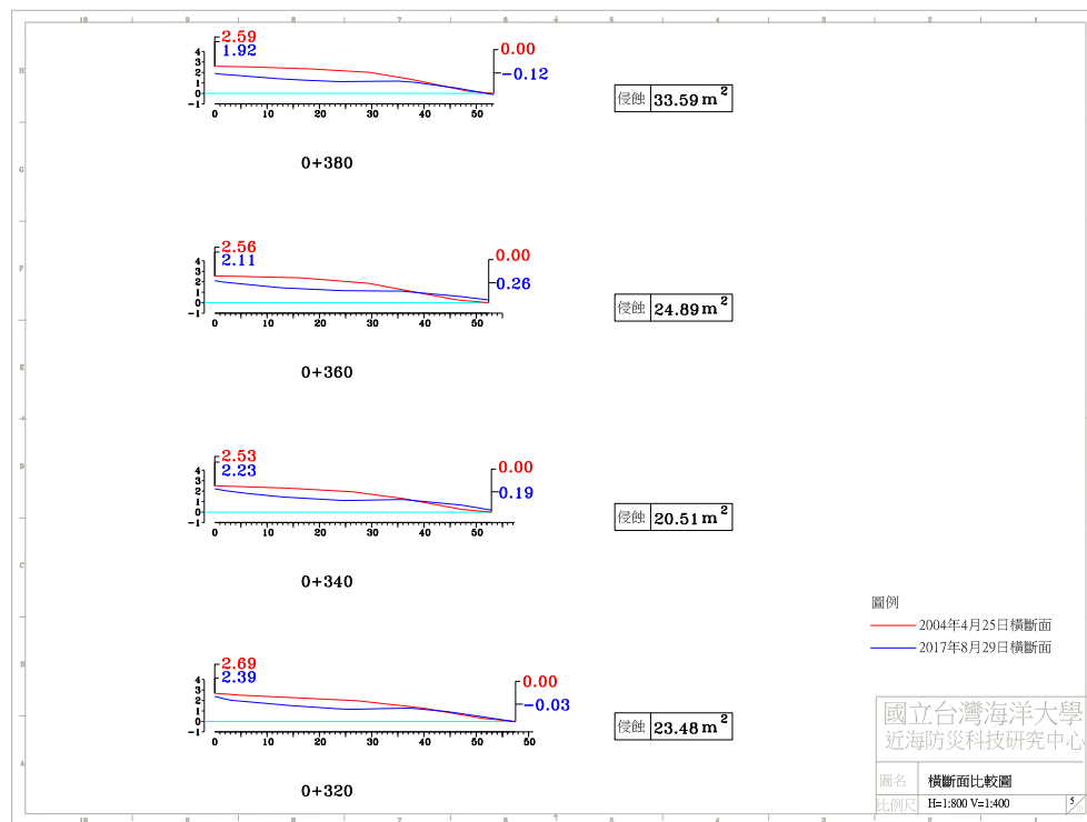
圖 4-4(f) 2017 年 8 月 29 日 A 監測區橫斷面比較圖
