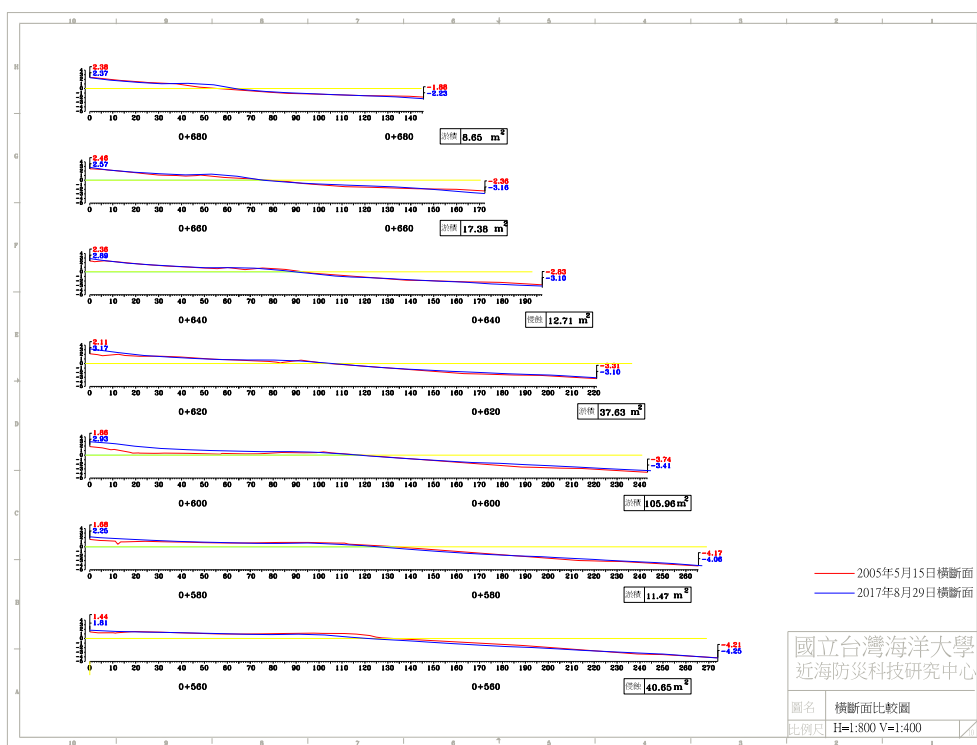
圖 4-5(b) 2017 年 8 月 29 日 B 監測區橫斷面比較圖
