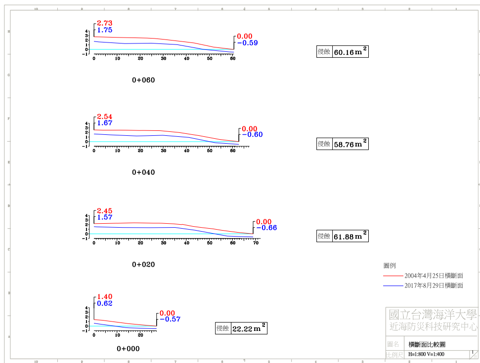
圖 4-4(j) 2017 年 8 月 29 日 A 監測區橫斷面比較圖
