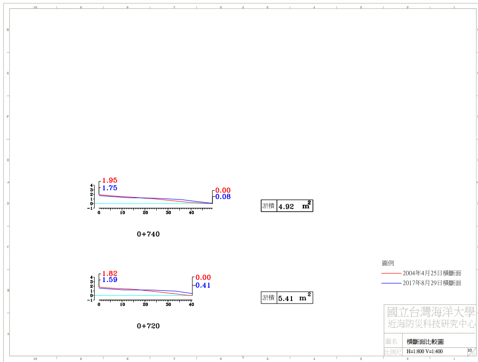
圖 4-4(a) 2017 年 8 月 29 日 A 監測區橫斷面比較圖
