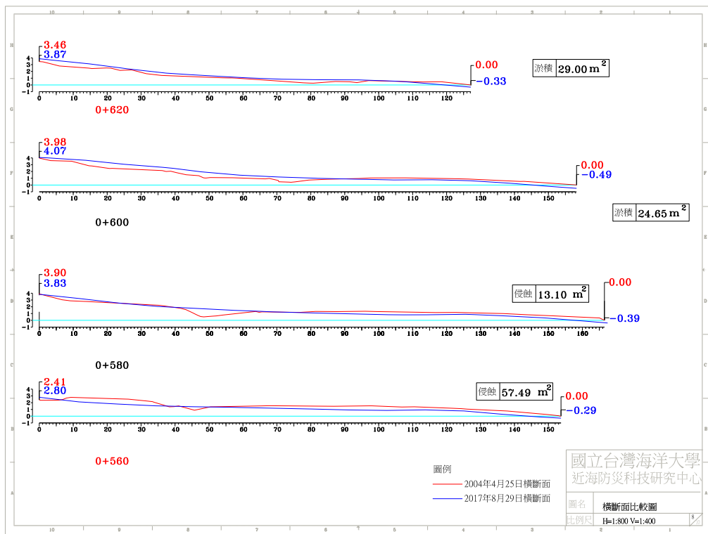
圖 4-4(c) 2017 年 8 月 29 日 A 監測區橫斷面比較圖
