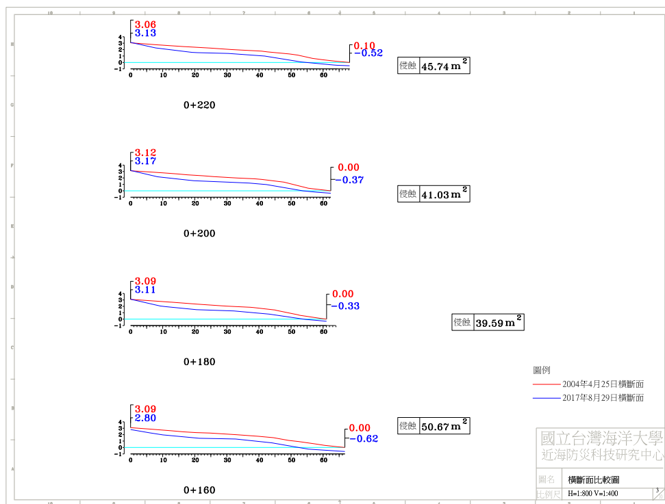
圖 4-4(h) 2017 年 8 月 29 日 A 監測區橫斷面比較圖
