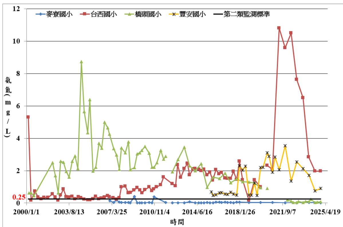
圖3.8 環保單位地下水氮氮濃度歷線圖
