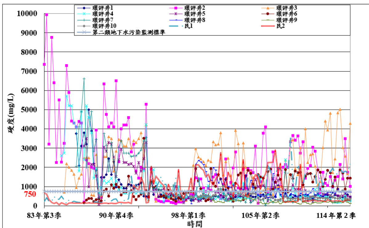
圖3.14 歷季硬度濃度監測結果
