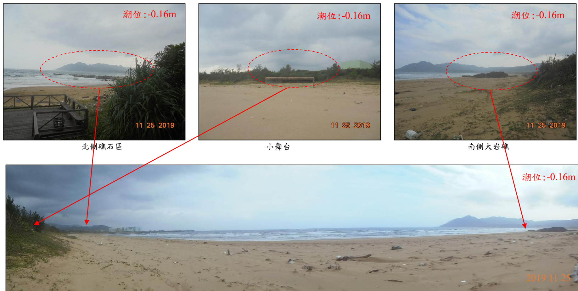
圖 3-6 鹽寮海岸短期性養灘區地形地貌圖(2019/11/25)
