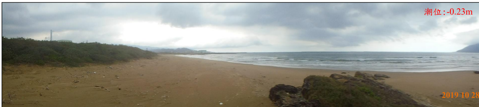
圖 4-7a 監測區南側大岩礁（黑石仔）前沙灘地形(2)（2019/10/28）
