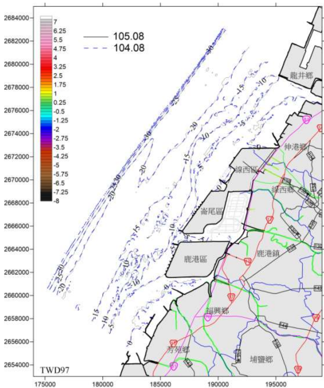
圖 2.11-3(a) 104 年 8 月與 105 年 8 月兩次施測地形等深線比較圖
