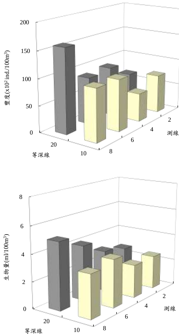
圖 2.10.2-1 民國 105 年 11 月彰化濱海工業區附近海域浮游動物之豐度及生物量分布圖
