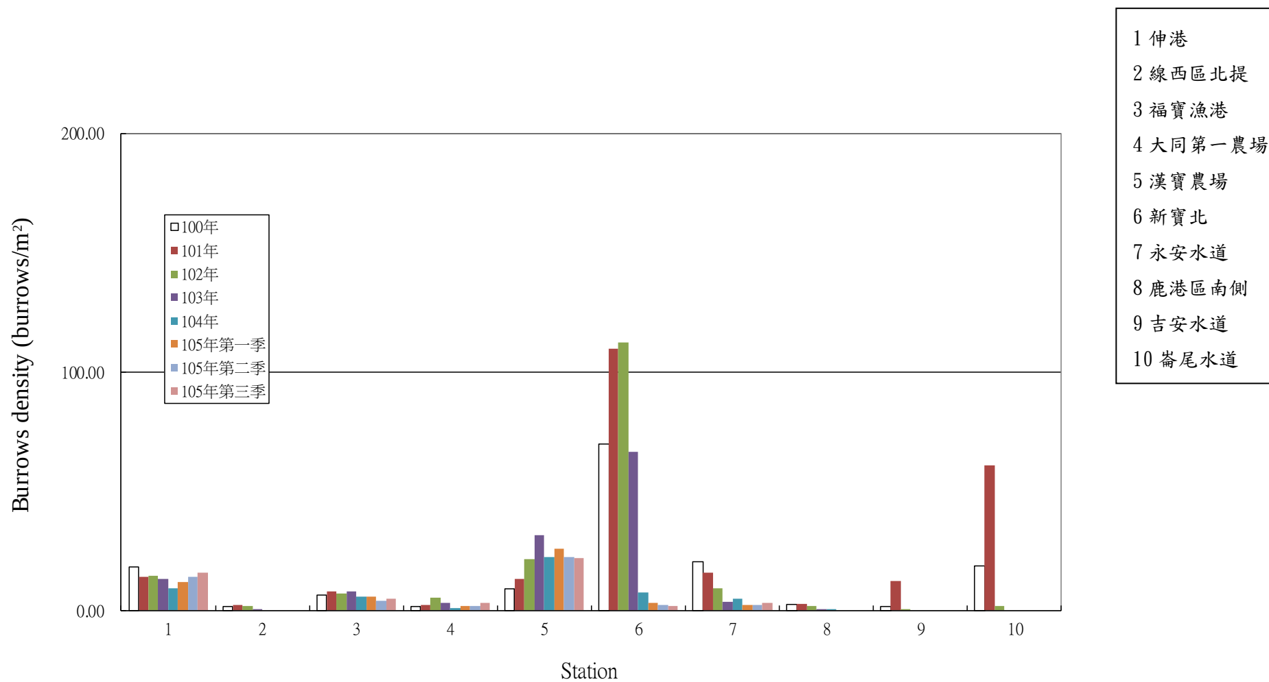
圖 3.1.6-1 各測站螻蛄蝦平均密度(平均洞口數/m²)分布圖
