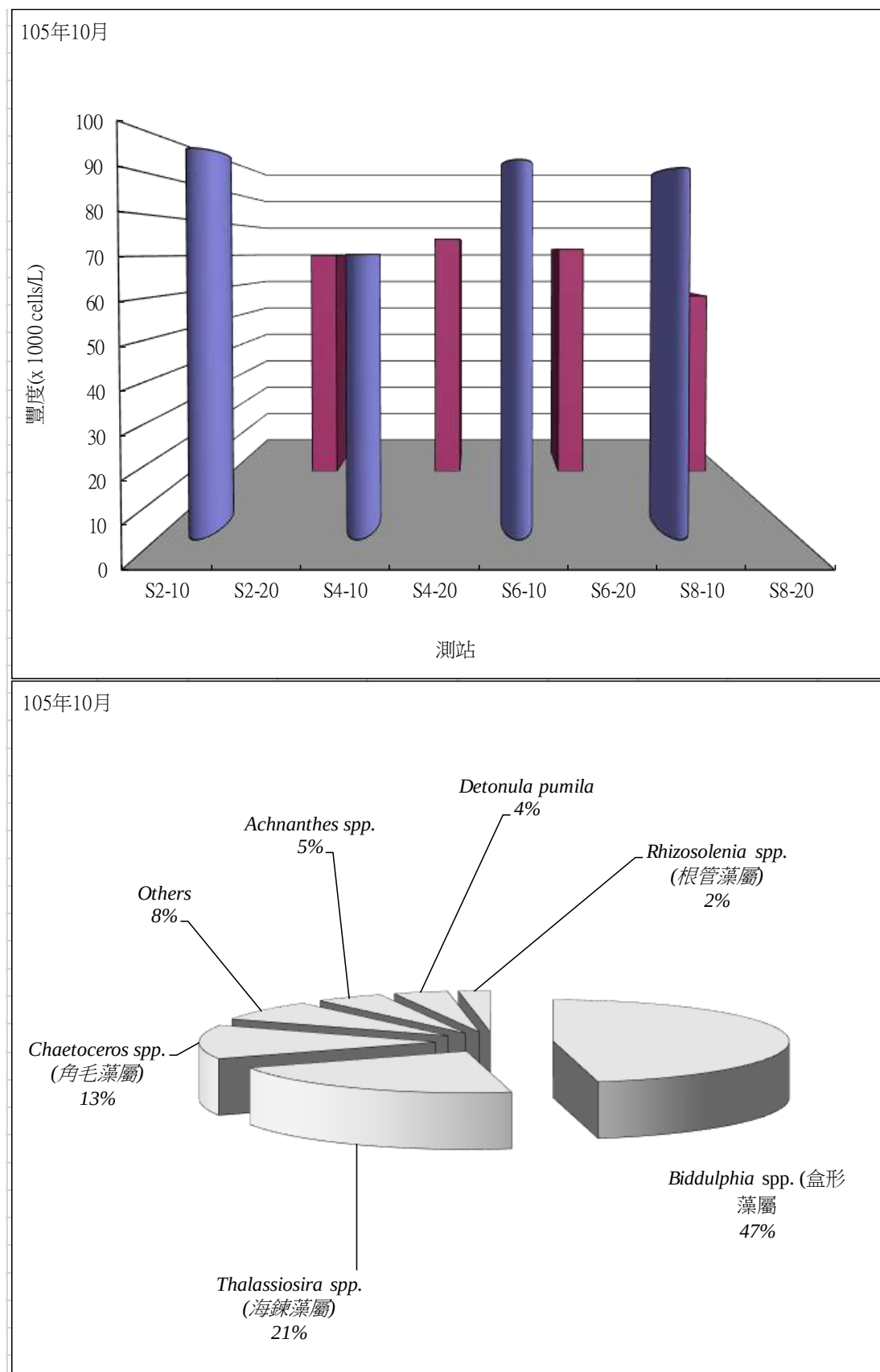
圖 2.10.1-1 民國 105 年 10 月於彰化濱海工業區附近海域各測站之浮游植物
