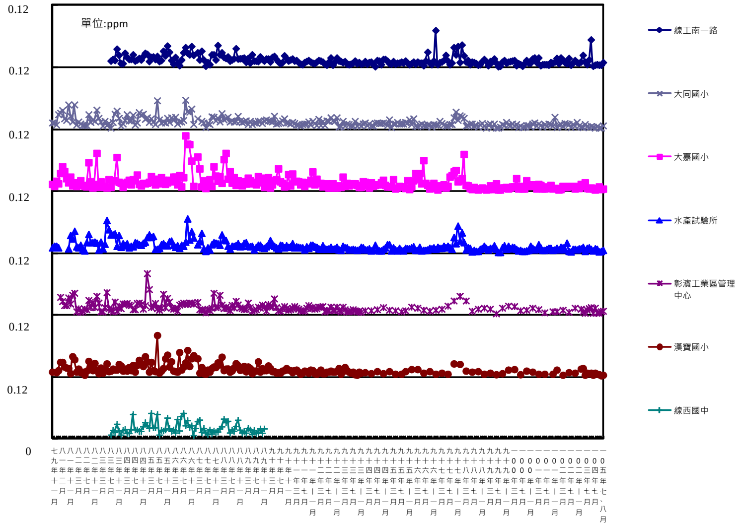
圖 3.1.1-2 彰濱地區歷年二氧化硫最高小時值監測結果分析圖
