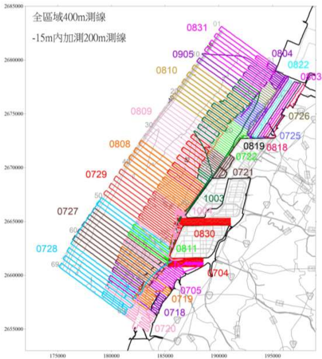
圖 2.11-1 105 年 7 月~10 月地形測量航跡圖
