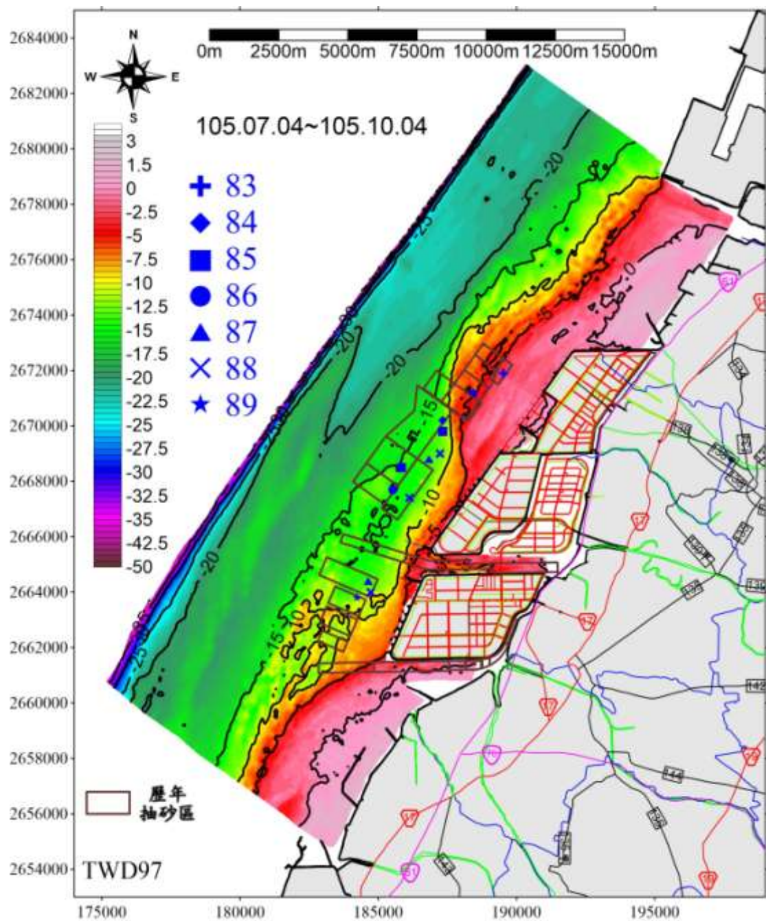
圖 2.11-2 105 年 7 月~10 月海底地形影像圖
