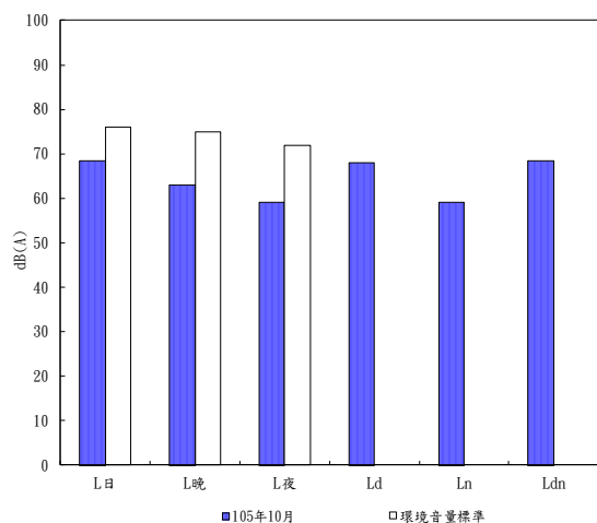
圖 2.2-7 台 17 省道與彰 30 交叉口本季噪音調查結果分析圖
