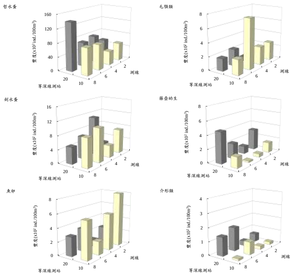
圖 2.10.2-2 民國 105 年 11 月彰化濱海工業區附近海域浮游動物主要優勢類群之豐度分布圖
