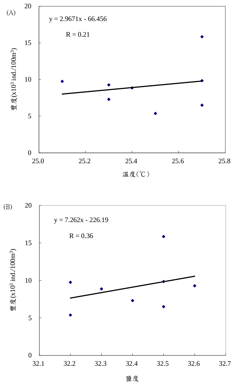
圖 2.10.2-4 民國 105 年 11 月彰濱工業區之浮游動物豐度與(A)溫度 (B)鹽度之相關係數圖
