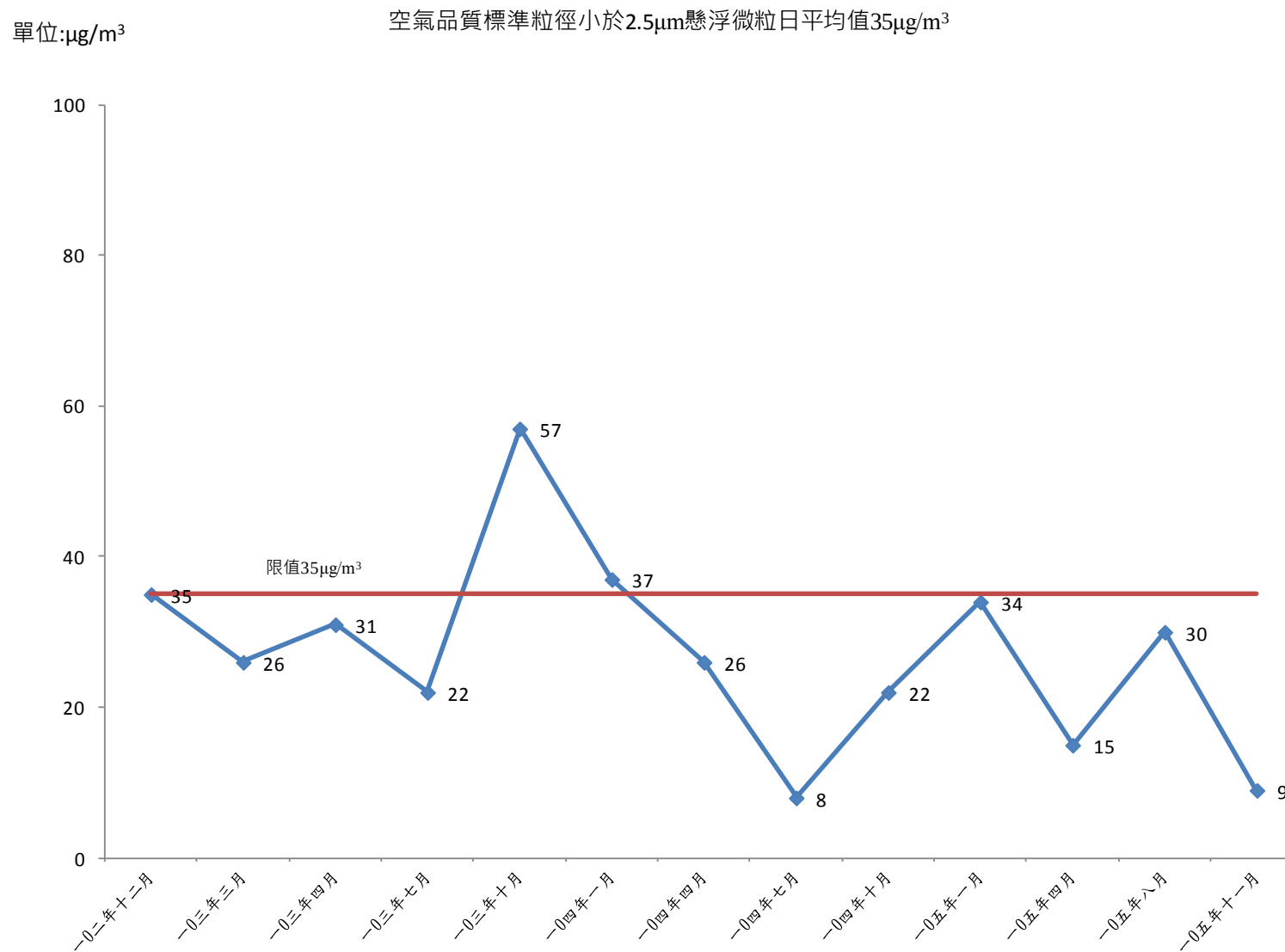
圖 3.1.1-8 彰濱地區-線工南一路歷年粒徑小於 2.5\mu\text{m} 之懸浮微粒日平均值監測結果分析圖
