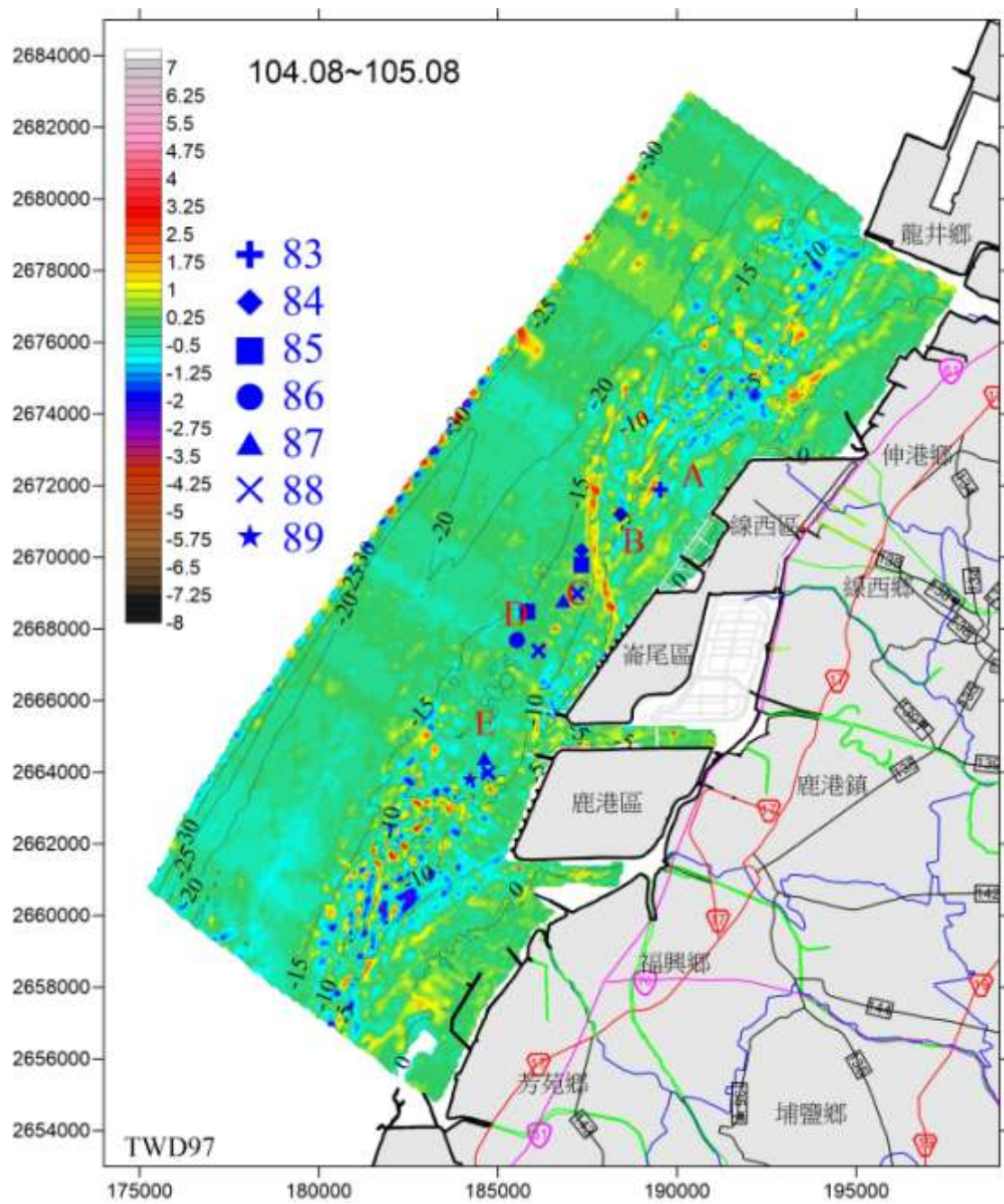
圖 2.11-3(b) 104 年 8 月與 105 年 8 月海底地形侵淤圖
