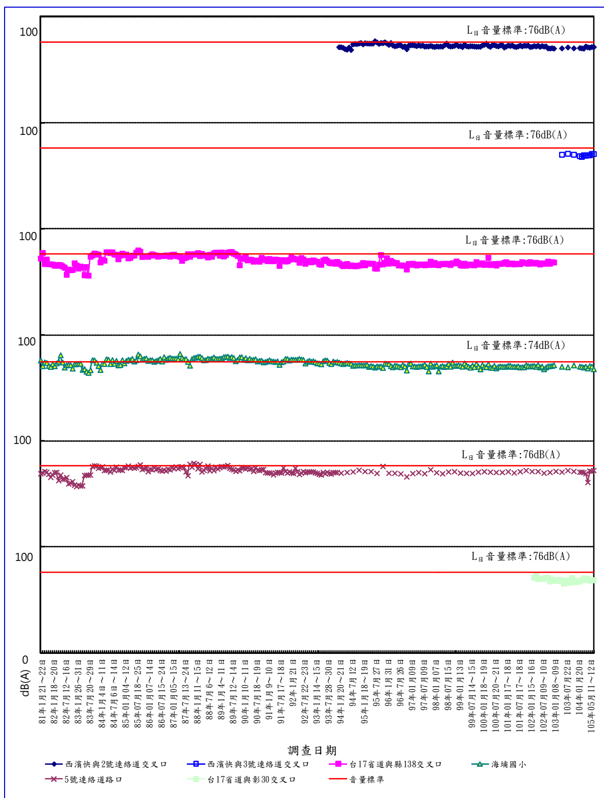
圖 3.1.2-1 彰濱地區歷次噪音 L_d 監測結果
