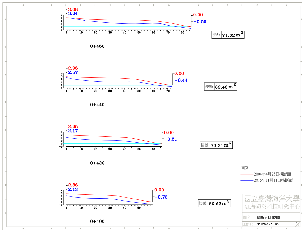
圖 4-4(e) 2015 年 11 月 11 日 A 監測區橫斷面比較圖
