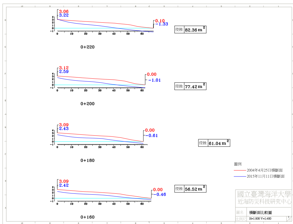
圖 4-4(h) 2015 年 11 月 11 日 A 監測區橫斷面比較圖
