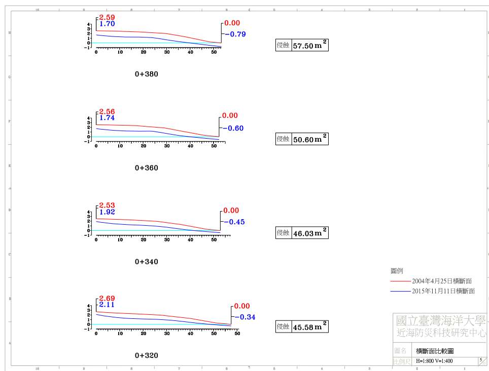
圖 4-4(f) 2015 年 11 月 11 日 A 監測區橫斷面比較圖
