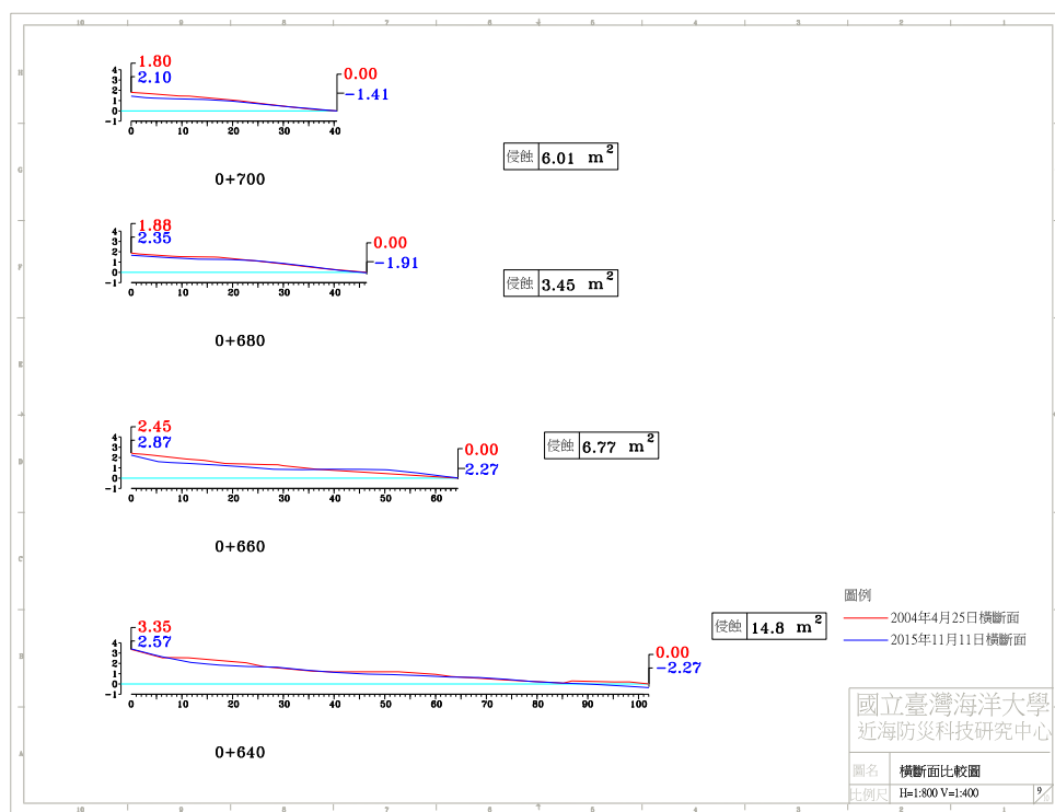
圖 4-4(b) 2015 年 11 月 11 日 A 監測區橫斷面比較圖
