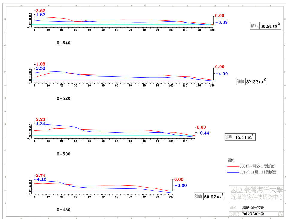
圖 4-4(d) 2015 年 11 月 11 日 A 監測區橫斷面比較圖
