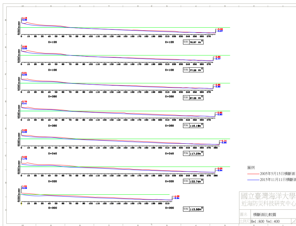
圖 4-5(f) 2015 年 11 月 11 日 B 監測區橫斷面比較圖
