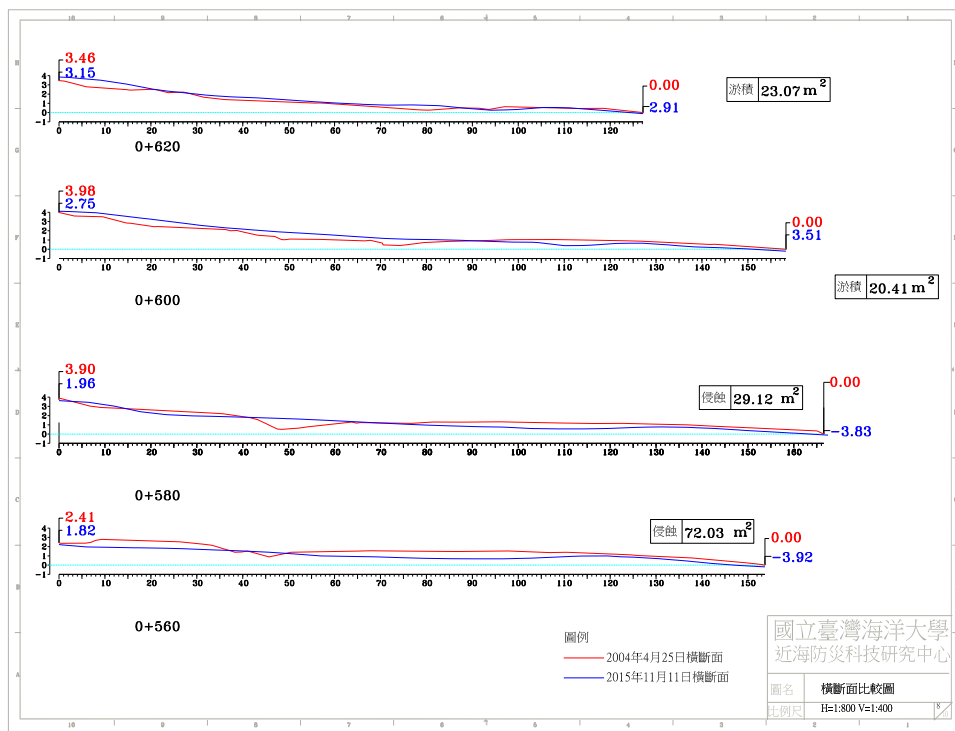
圖 4-4(c) 2015 年 11 月 11 日 A 監測區橫斷面比較圖
