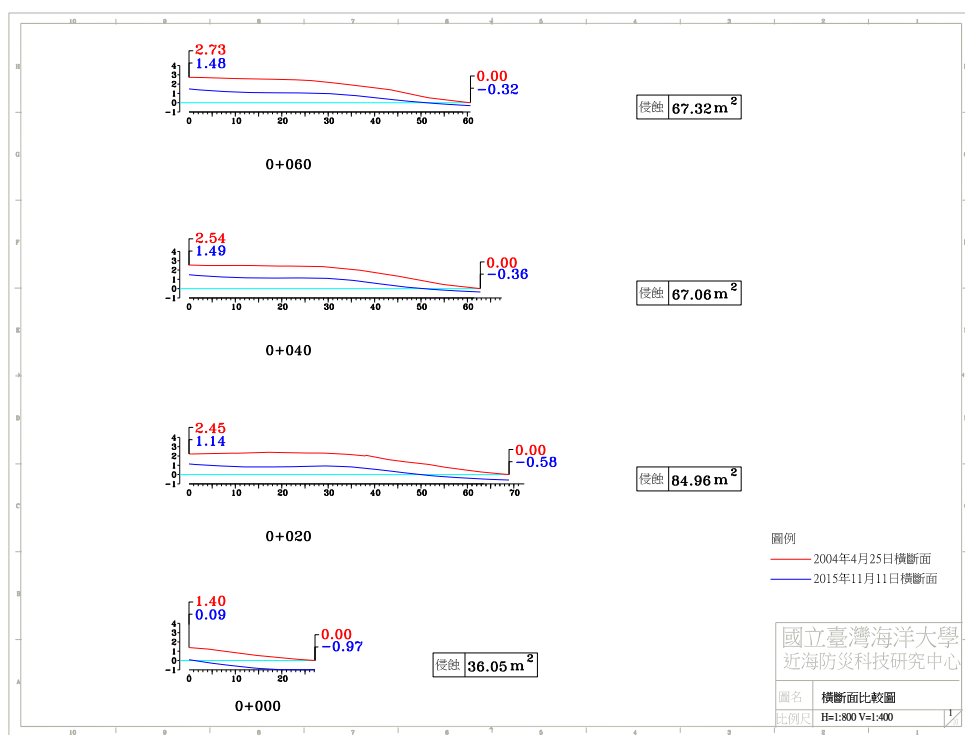
圖 4-4(j) 2015 年 11 月 11 日 A 監測區橫斷面比較圖
