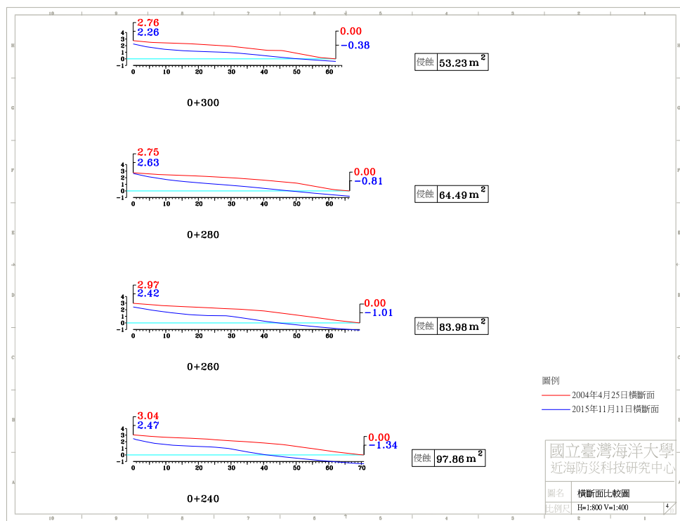
圖 4-4(g) 2015 年 11 月 11 日 A 監測區橫斷面比較圖
