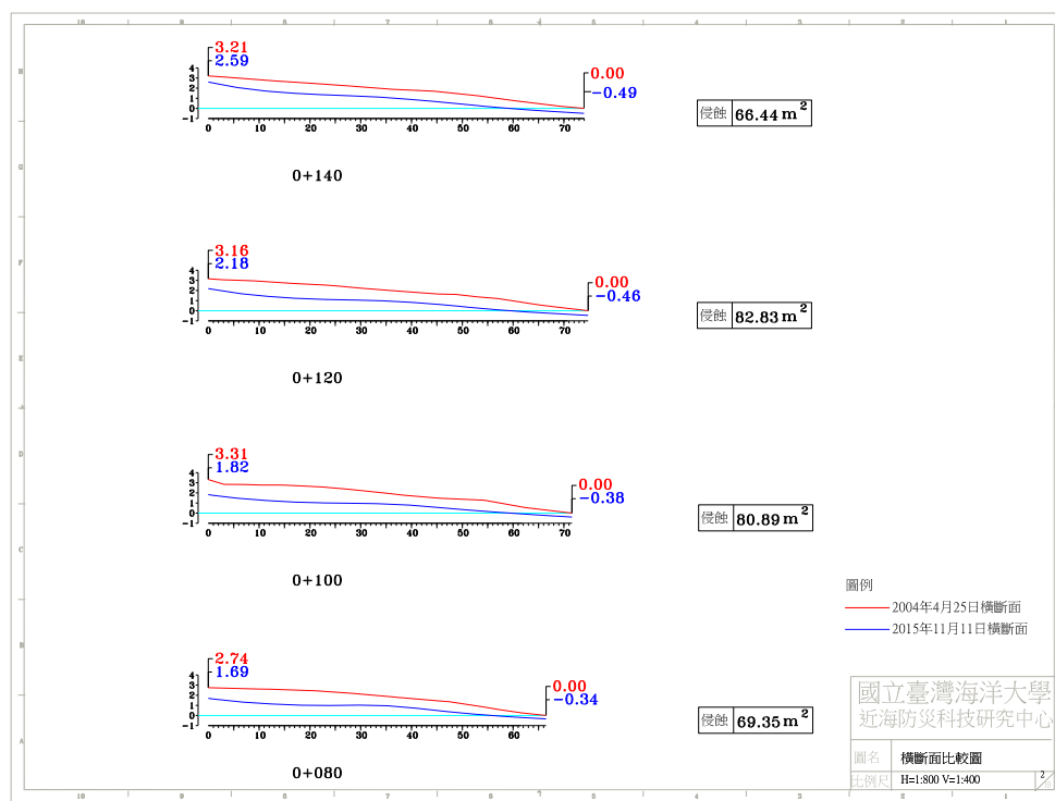
圖 4-4(i) 2015 年 11 月 11 日 A 監測區橫斷面比較圖
