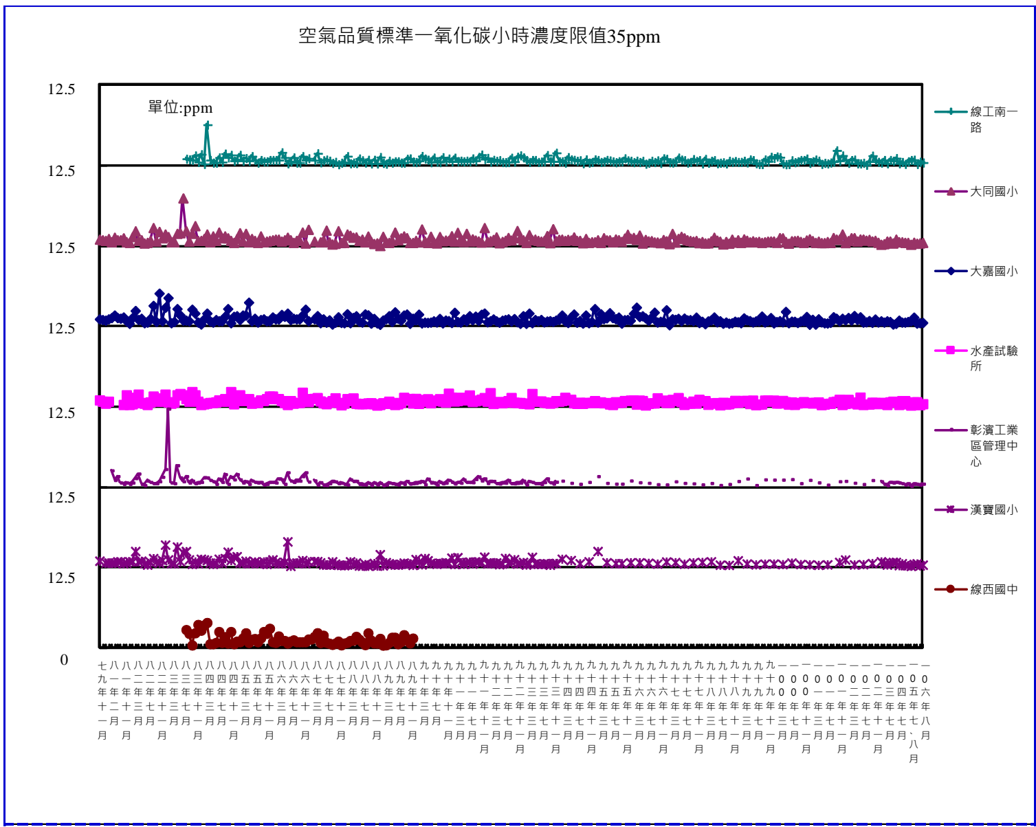
圖 3.1.1-1 彰濱地區歷年一氧化碳最高小時值監測結果分析圖
