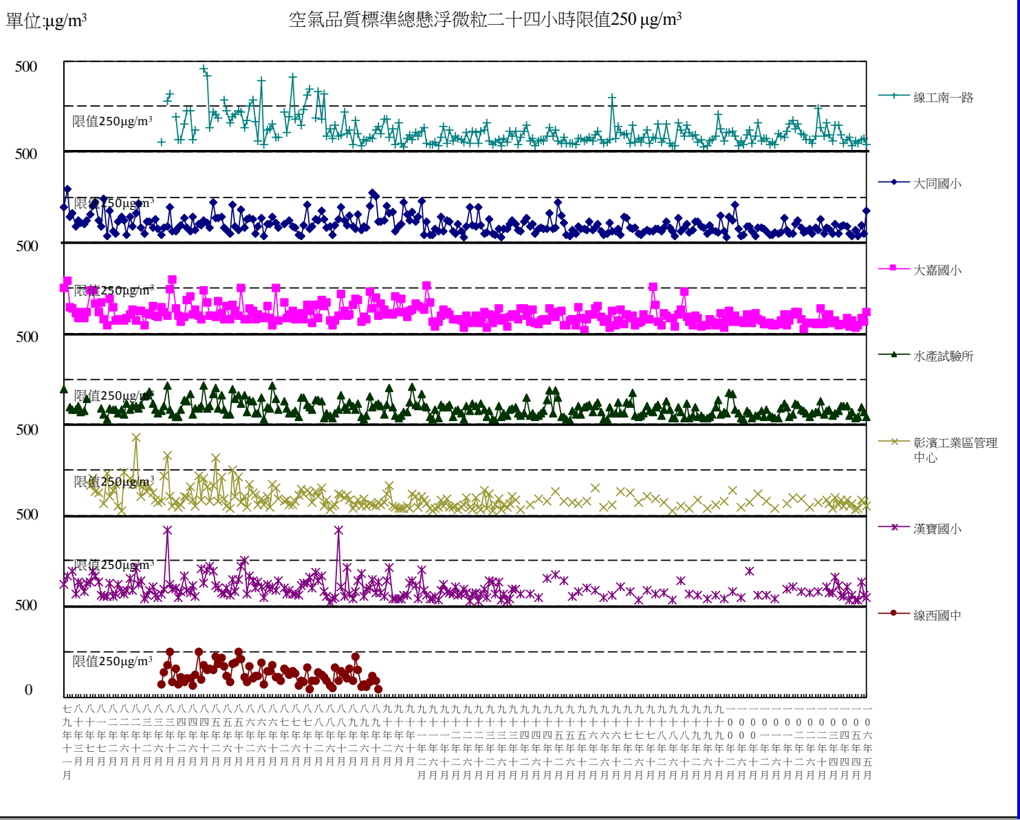
圖 3.1.1-6 彰濱地區歷年總懸浮微粒 24 小時值監測結果分析圖
