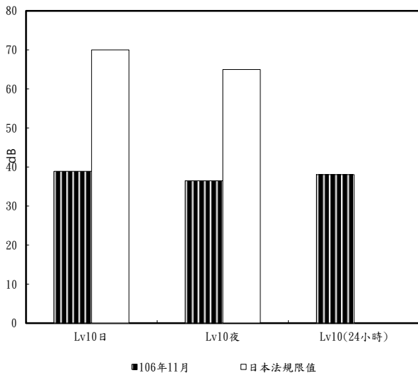
圖 2.3-5 海埔國小本季振動調查結果分析圖
