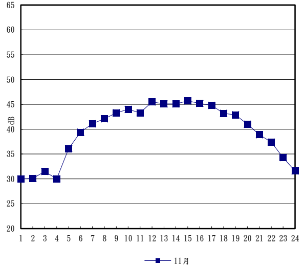
圖 2.3-2 西濱快與 2 號連絡道交叉口本季振動測值逐時變化圖
