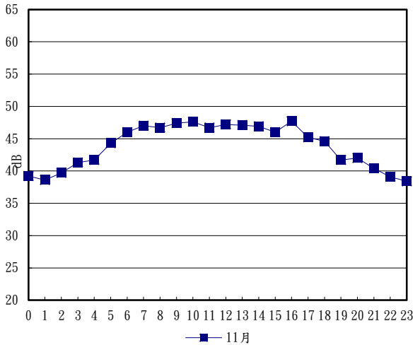
圖 2.3-4 西濱快與 3 號連絡道交叉口本季振動測值逐時變化圖
