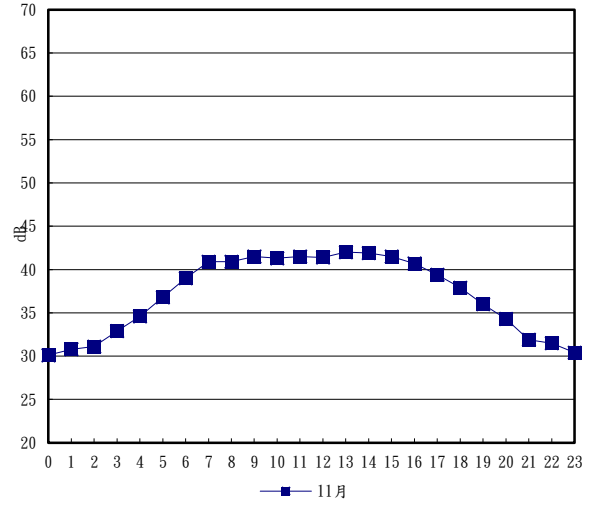
圖 2.3-8 5號連絡道路口本季振動測值逐時變化圖
