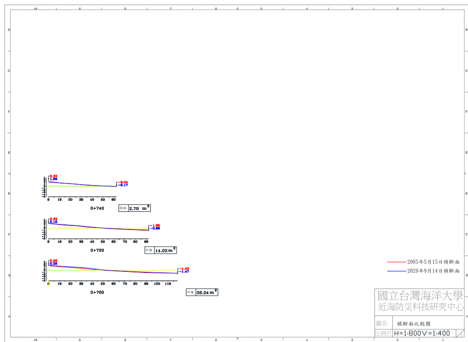
圖 4-7(a) 2020 年 9 月 14 日 B 監測區橫斷面比較圖
