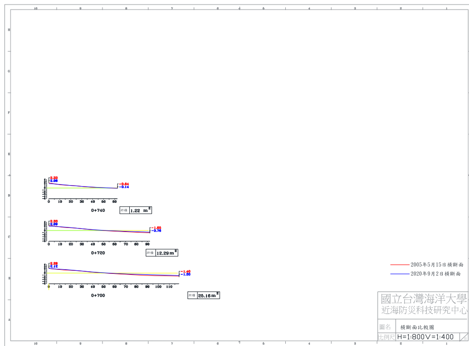
圖 4-5(a) 2020 年 9 月 2 日 B 監測區橫断面比較圖
