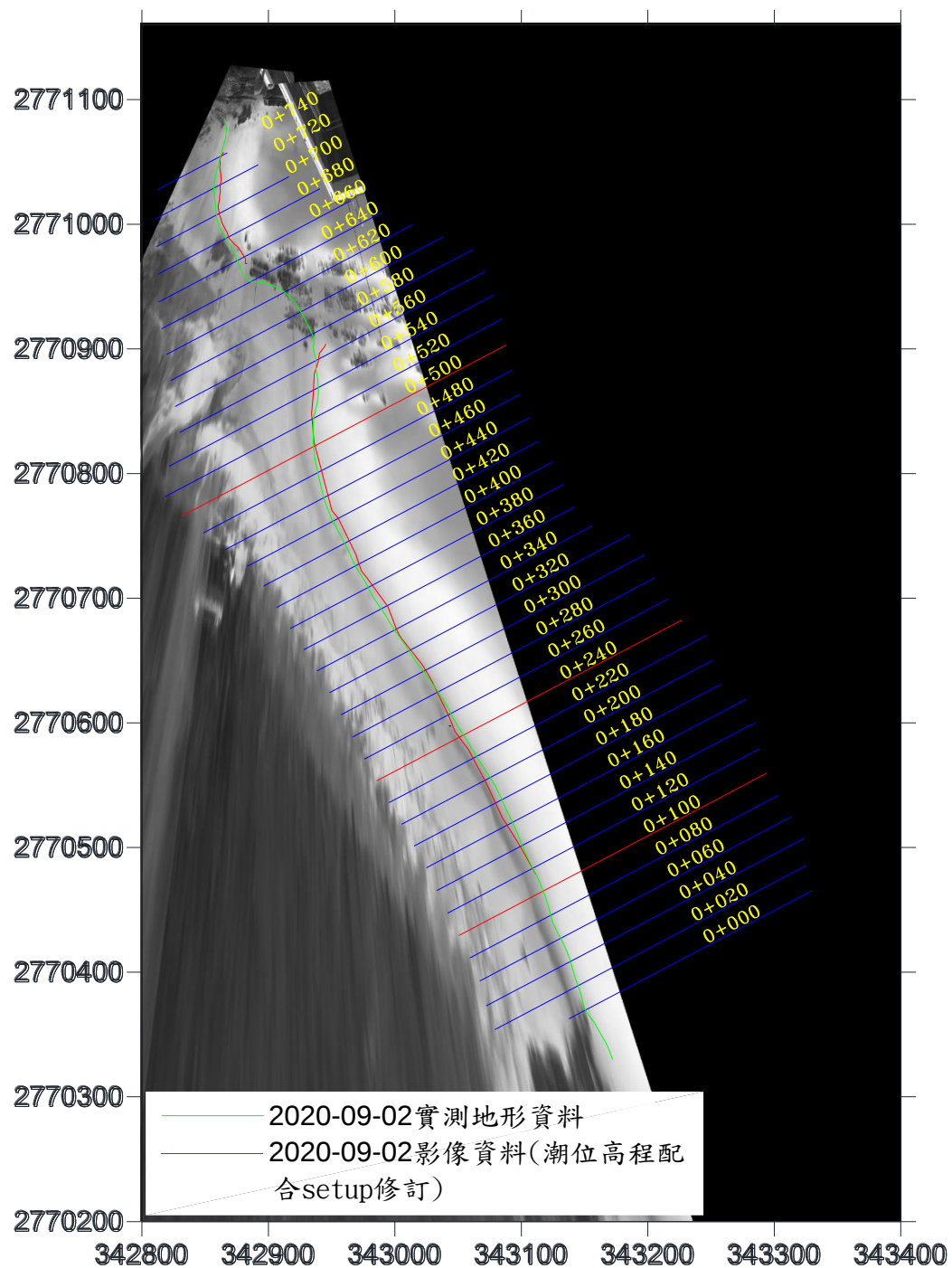
圖 3-22(a) 水位線分析結果圖(2020/9/02)
