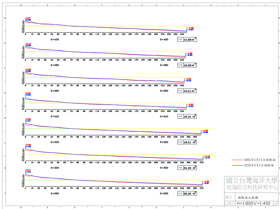
圖 4-5(d) 2020 年 9 月 2 日 B 監測區橫斷面比較圖
