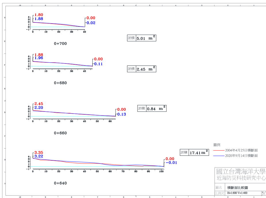
圖 4-6(a) 2020 年 9 月 14 日 A 監測區橫斷面比較圖
