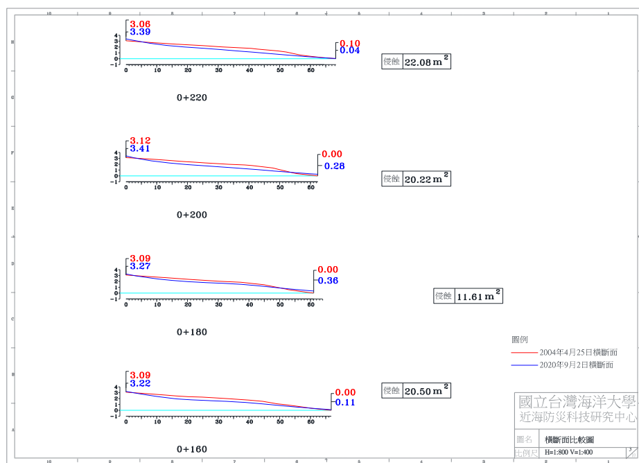
圖 4-4(h) 2020 年 9 月 2 日 A 監測區橫斷面比較圖
