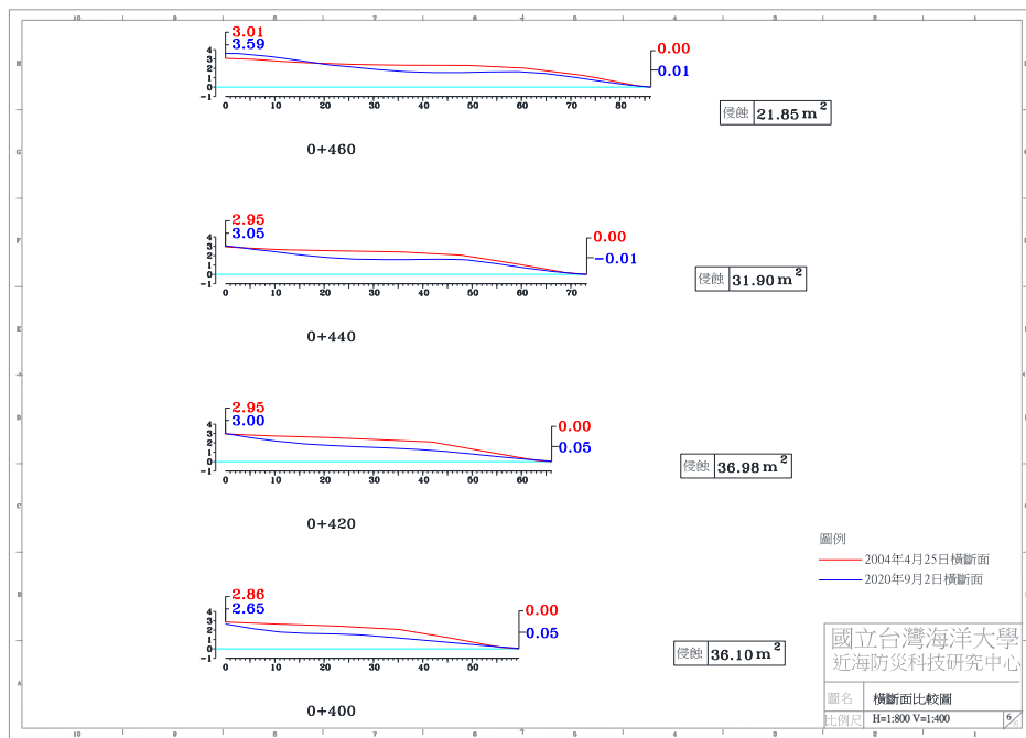
圖 4-4(e) 2020 年 9 月 2 日 A 監測區橫斷面比較圖
