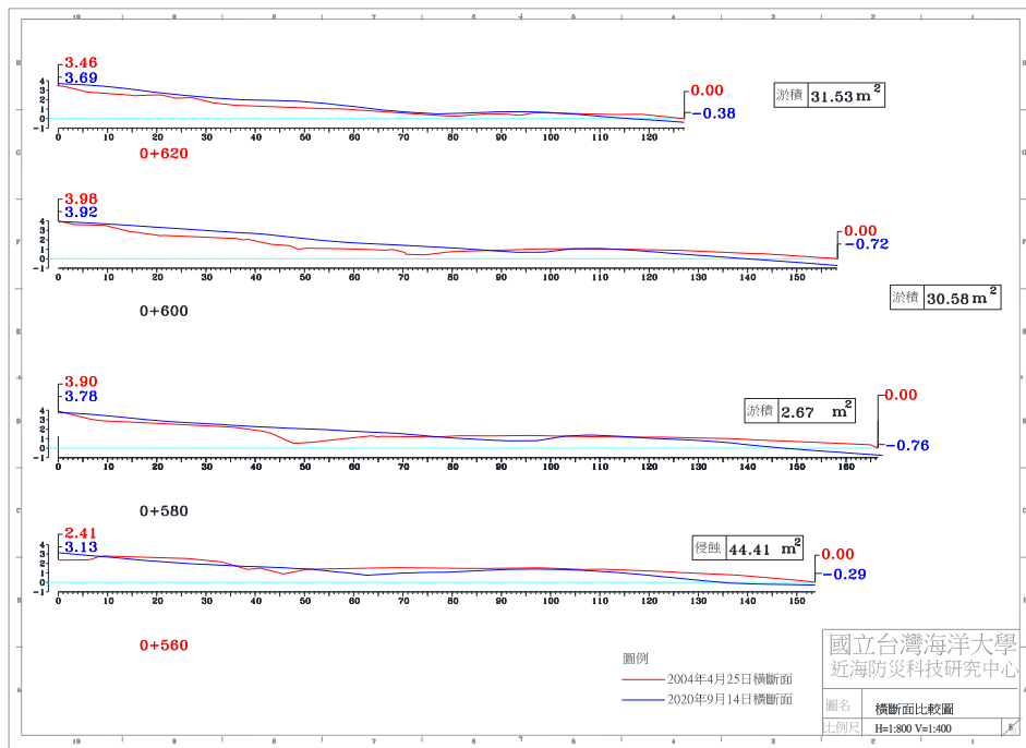
圖 4-6(c) 2020 年 9 月 14 日 A 監測區橫斷面比較圖
