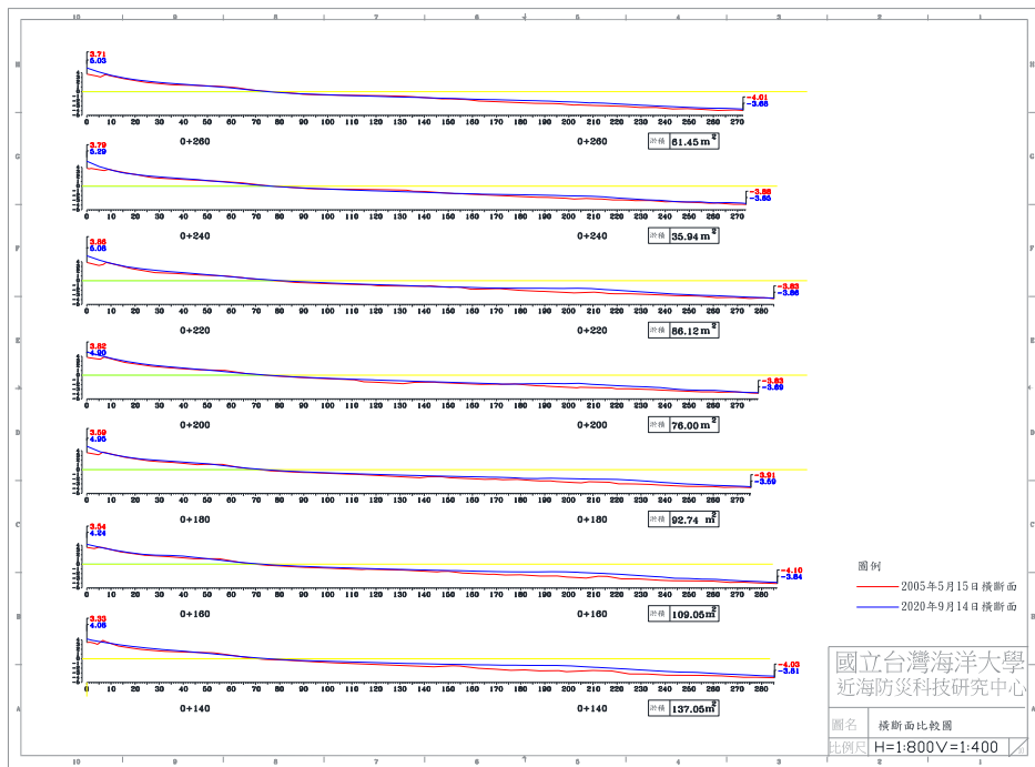
圖 4-7(e) 2020 年 9 月 14 日 B 監測區橫断面比較圖
