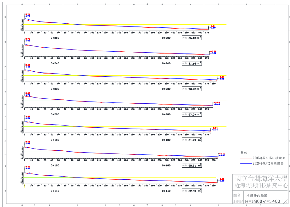
圖 4-5(e) 2020 年 9 月 2 日 B 監測區橫斷面比較圖
