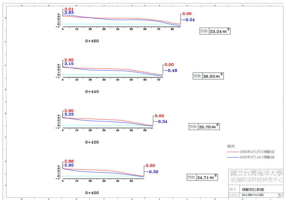
圖 4-6(e) 2020 年 9 月 14 日 A 監測區橫斷面比較圖
