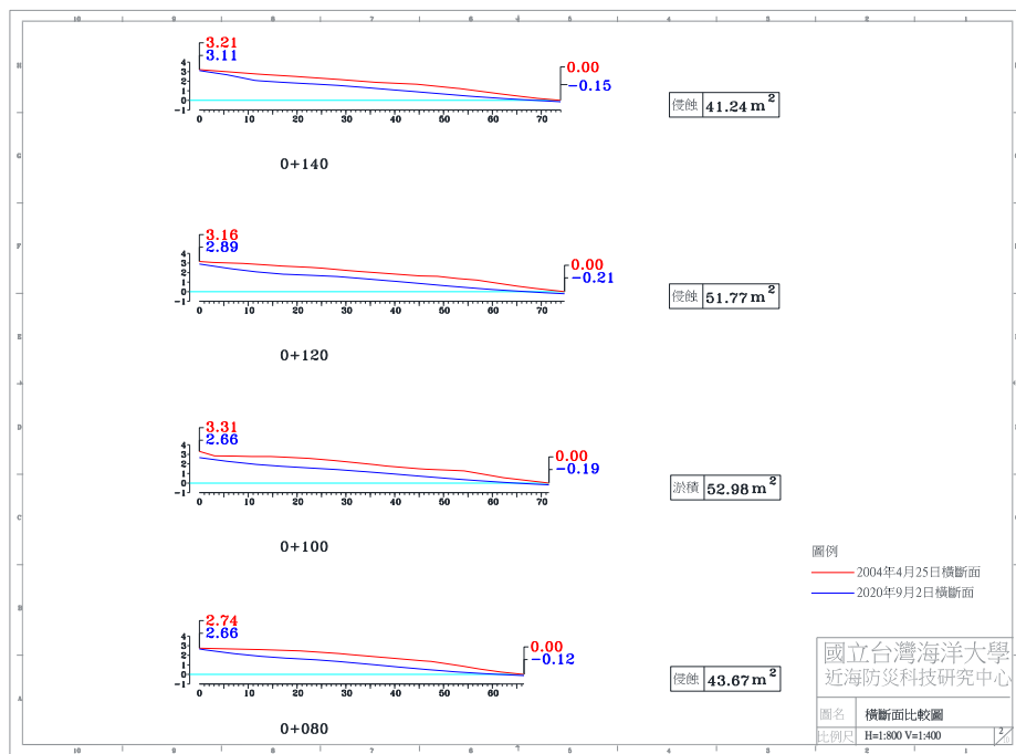
圖 4-4(i) 2020 年 9 月 2 日 A 監測區橫斷面比較圖
