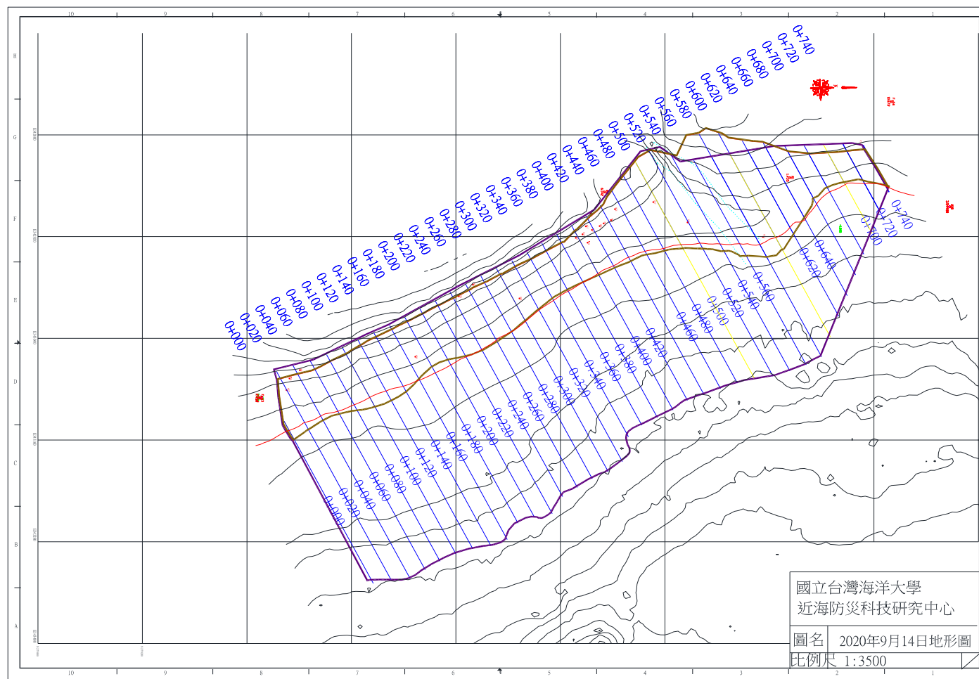
圖 4-1(b) 2020 年 9 月 14 日監測地形圖
