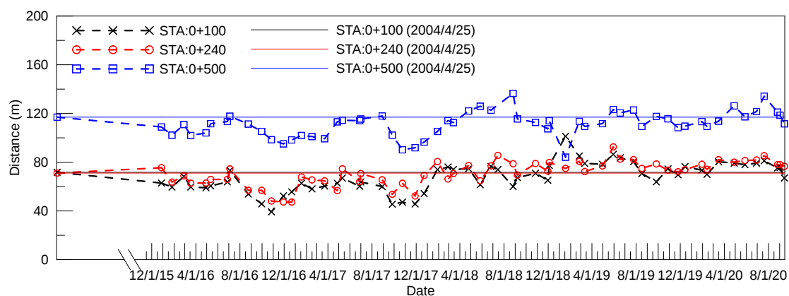
圖 4-23 岸線斷面沙灘寬度變化圖(斷面編號：0+100、0+240、0+500)
