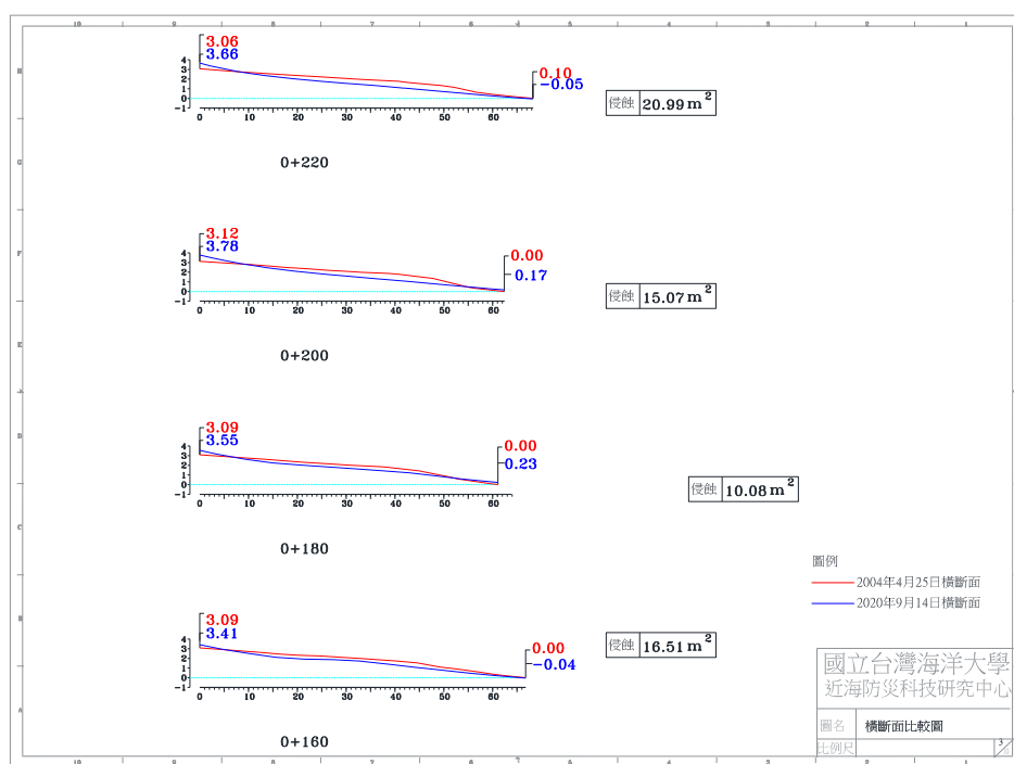
圖 4-6(h) 2020 年 9 月 14 日 A 監測區橫斷面比較圖
