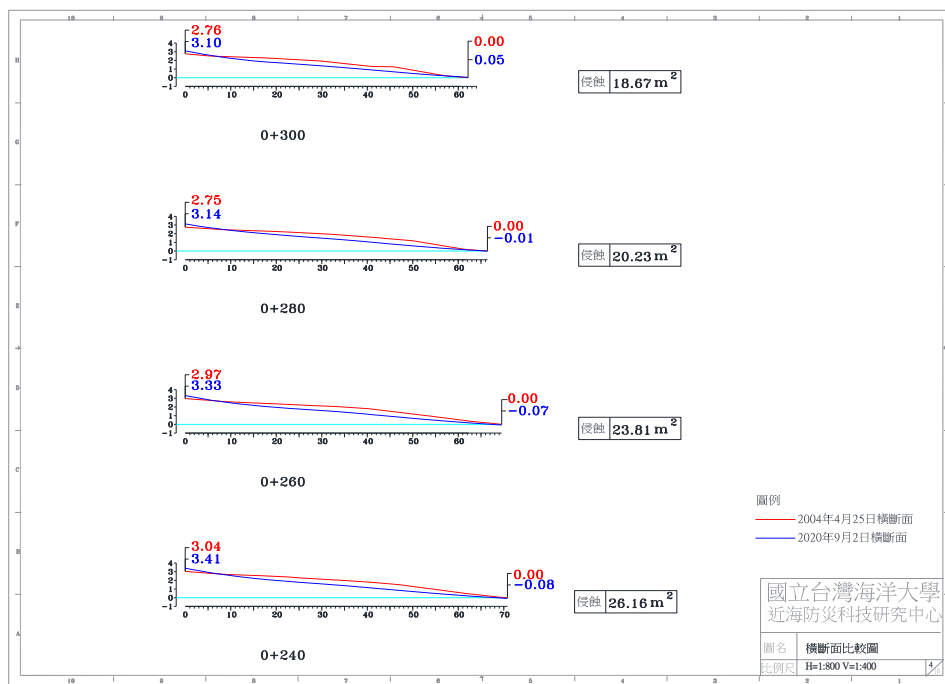
圖 4-4(g) 2020 年 9 月 2 日 A 監測區橫斷面比較圖
