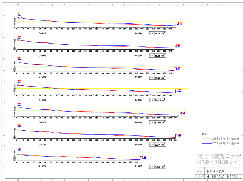
圖 4-7(f) 2020 年 9 月 14 日 B 監測區橫断面比較圖
