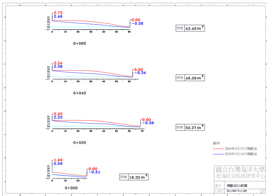
圖 4-6(j) 2020 年 9 月 14 日 A 監測區橫斷面比較圖
