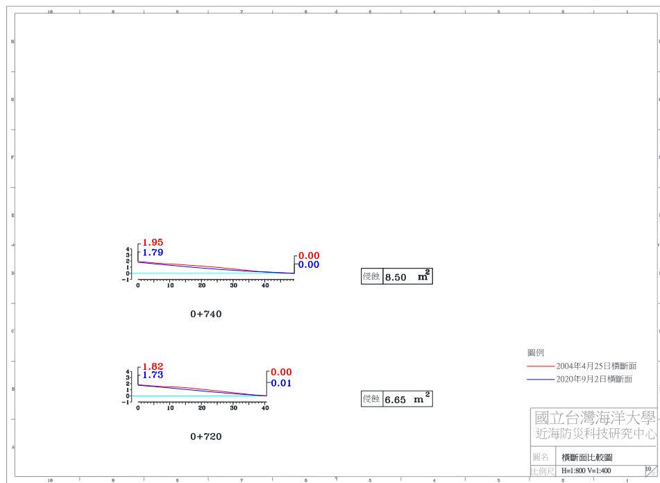
圖 4-4(a) 2020 年 9 月 2 日 A 監測區橫斷面比較圖
