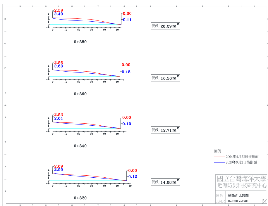
圖 4-4(f) 2020 年 9 月 2 日 A 監測區橫斷面比較圖
