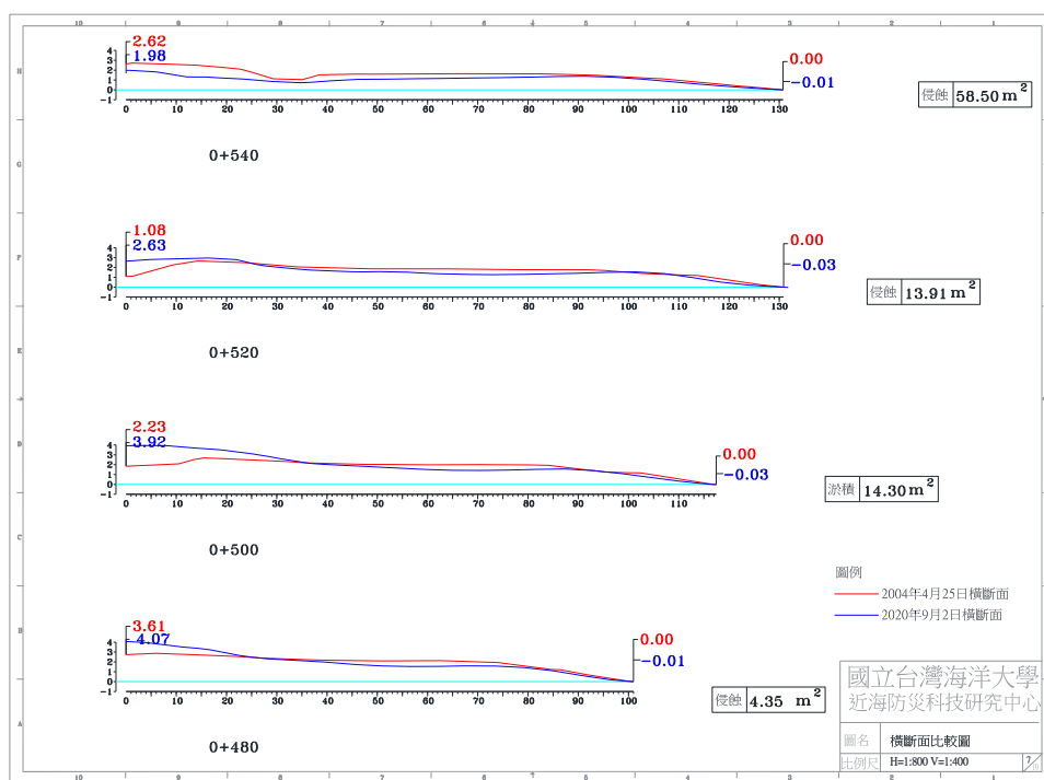
圖 4-4(d) 2020 年 9 月 2 日 A 監測區橫斷面比較圖
