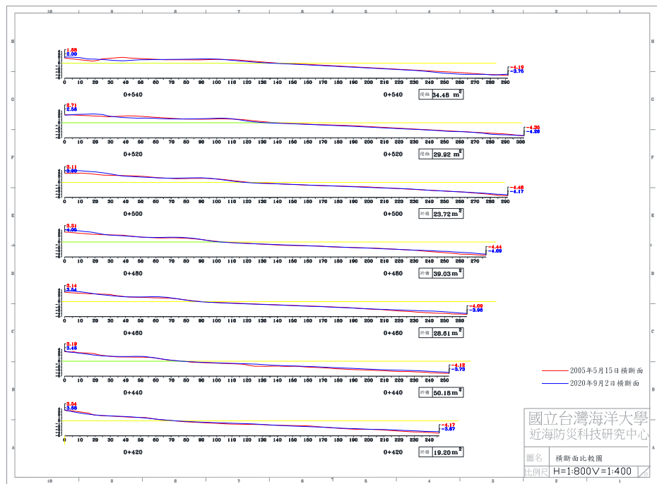
圖 4-5(c) 2020 年 9 月 2 日 B 監測區橫斷面比較圖
