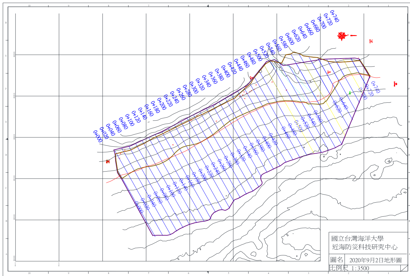
圖 4-1(a) 2020 年 9 月 2 日監測地形圖
