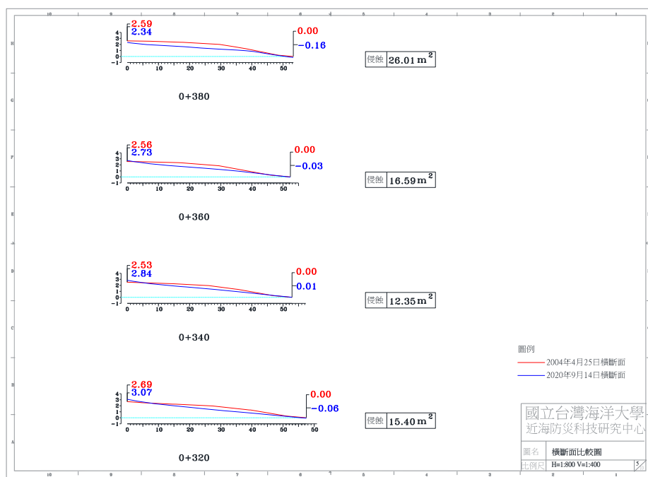
圖 4-6(f) 2020 年 9 月 14 日 A 監測區橫斷面比較圖
