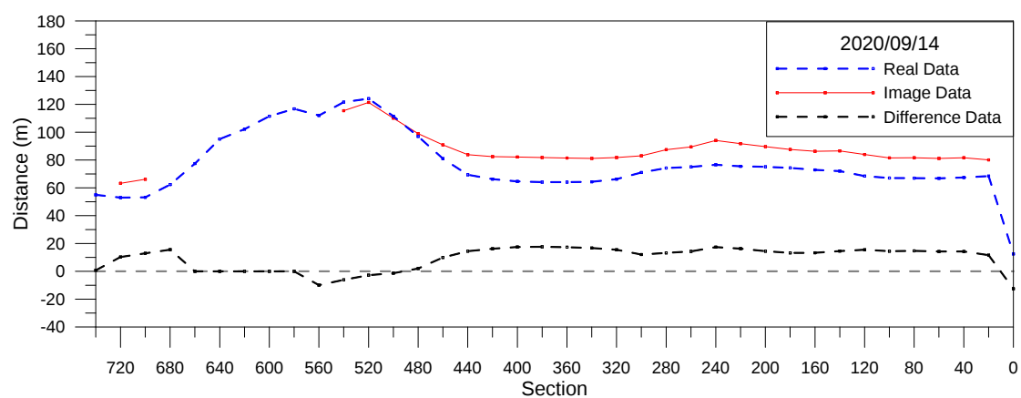
圖 3-23(b) 海岸線分析比較圖(2020/9/14)
