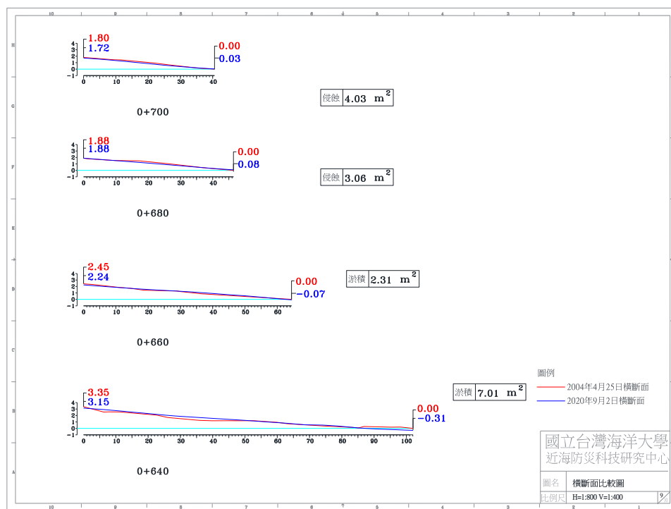
圖 4-4(b) 2020 年 9 月 2 日 A 監測區橫斷面比較圖
