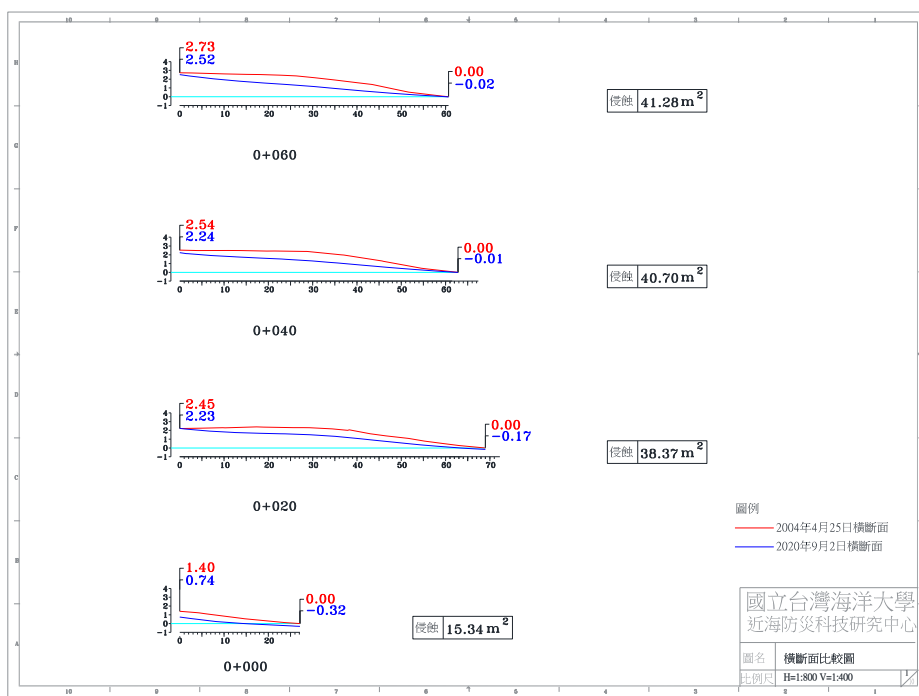
圖 4-4(j) 2020 年 9 月 2 日 A 監測區橫斷面比較圖
