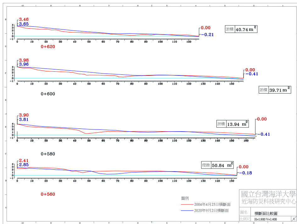
圖 4-4(c) 2020 年 9 月 2 日 A 監測區橫斷面比較圖
