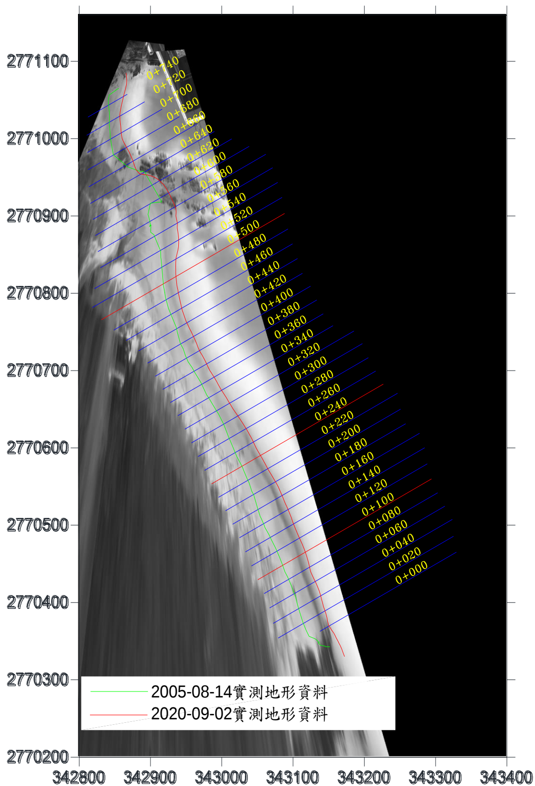
圖 4-24(a) 實測地形水位線分析結果圖(2020/09/02)
