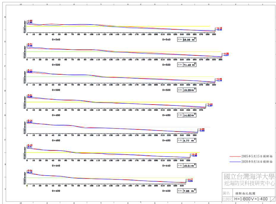
圖 4-7(c) 2020 年 9 月 14 日 B 監測區橫斷面比較圖
