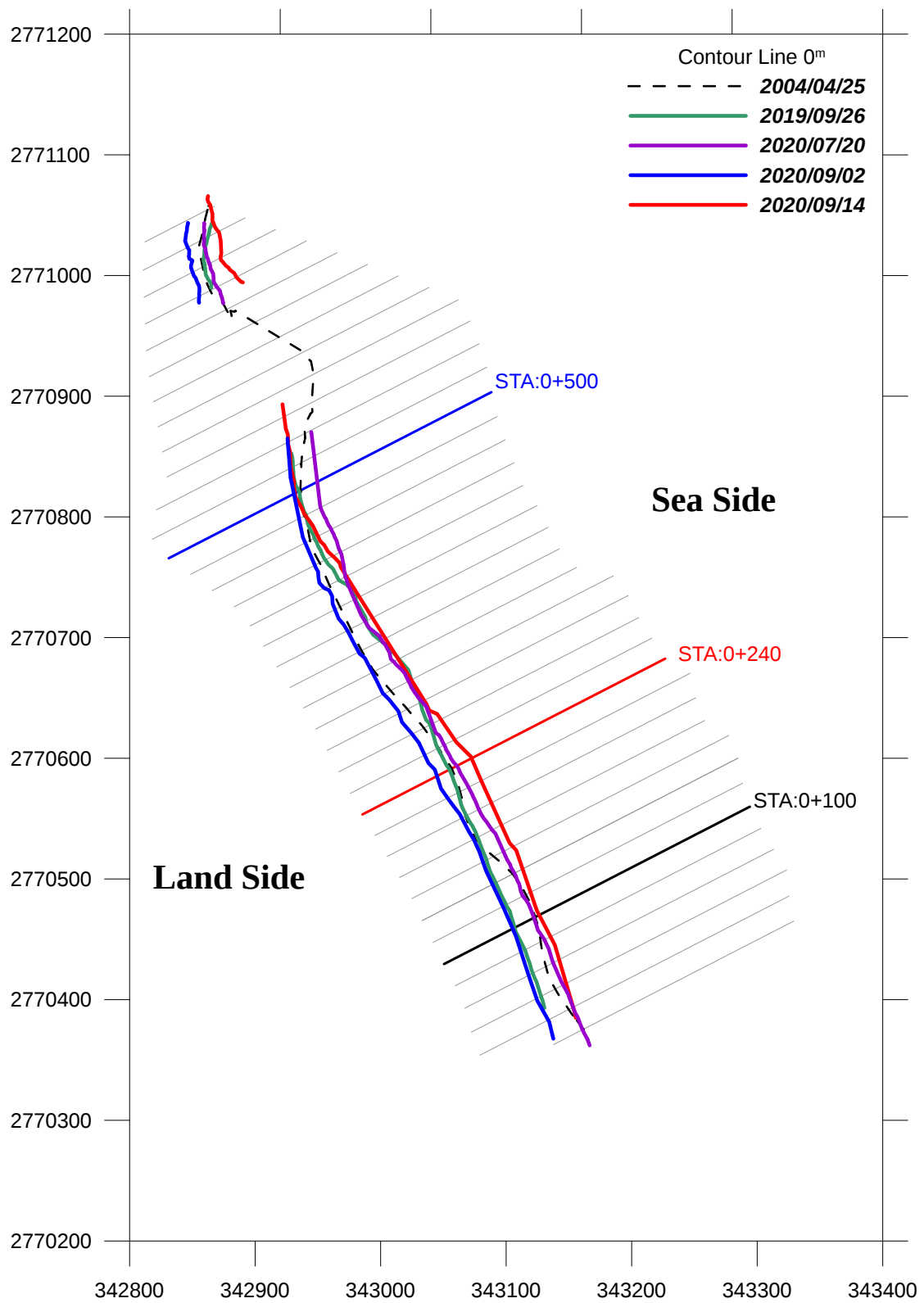
圖 4-22 鹽寮岸線變遷分析比較圖
