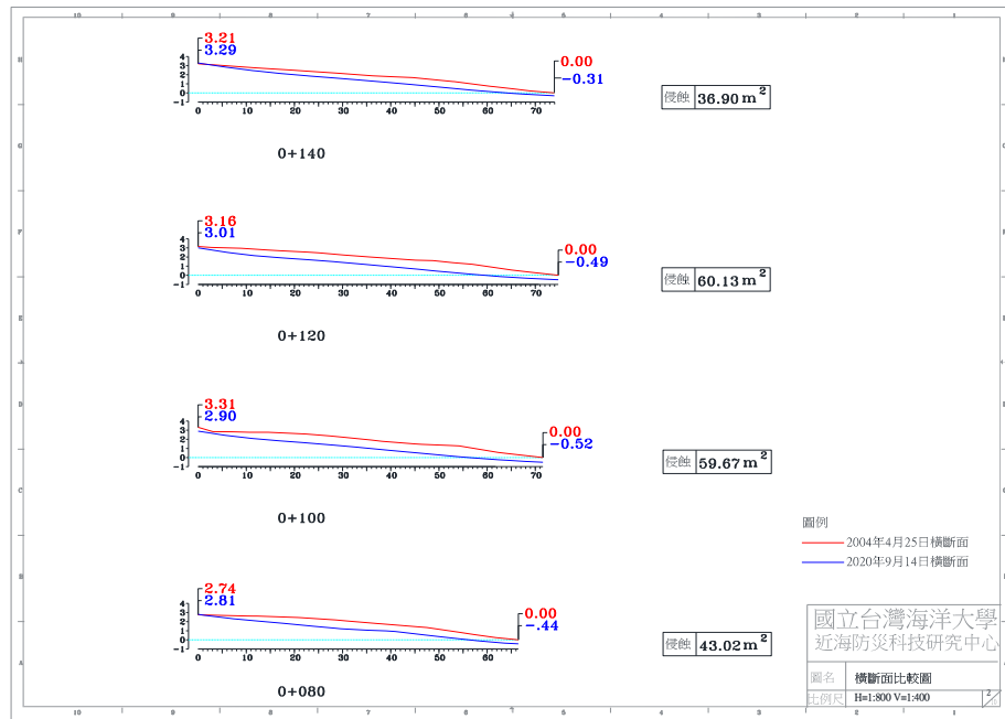
圖 4-6(i) 2020 年 9 月 14 日 A 監測區橫斷面比較圖
