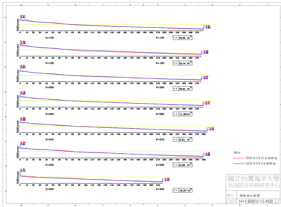
圖 4-5(e) 2020 年 9 月 2 日 B 監測區橫斷面比較圖
