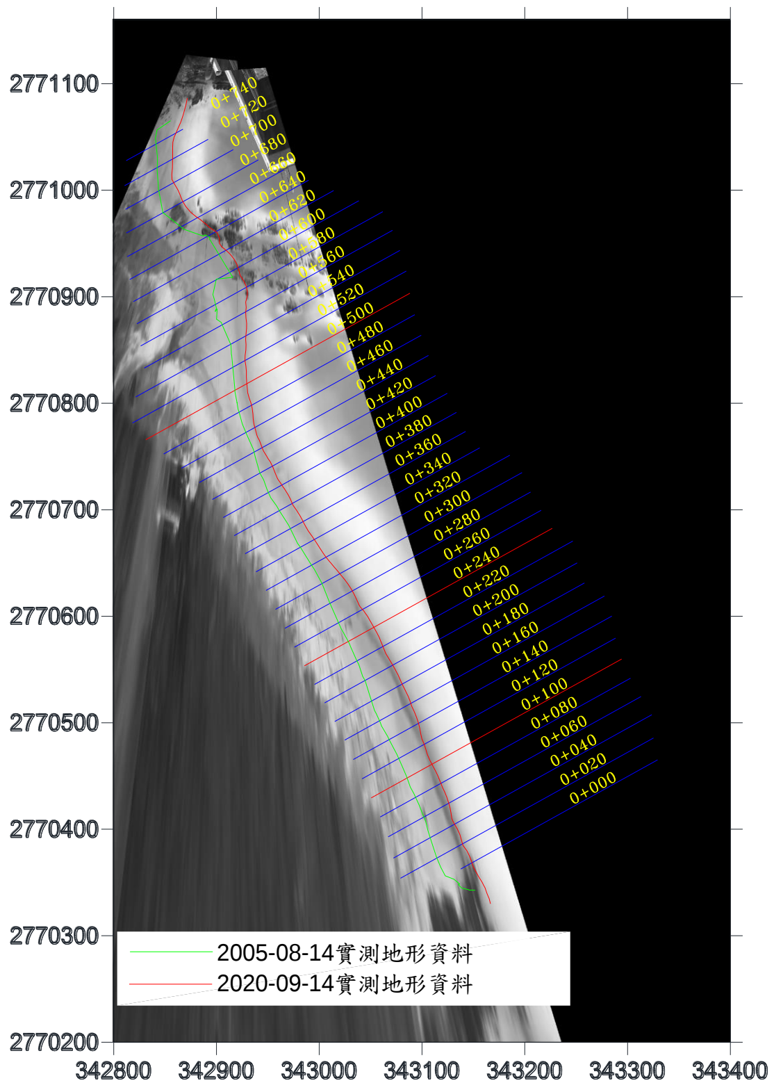
圖 4-24(b) 實測地形水位線分析結果圖(2020/09/14)
