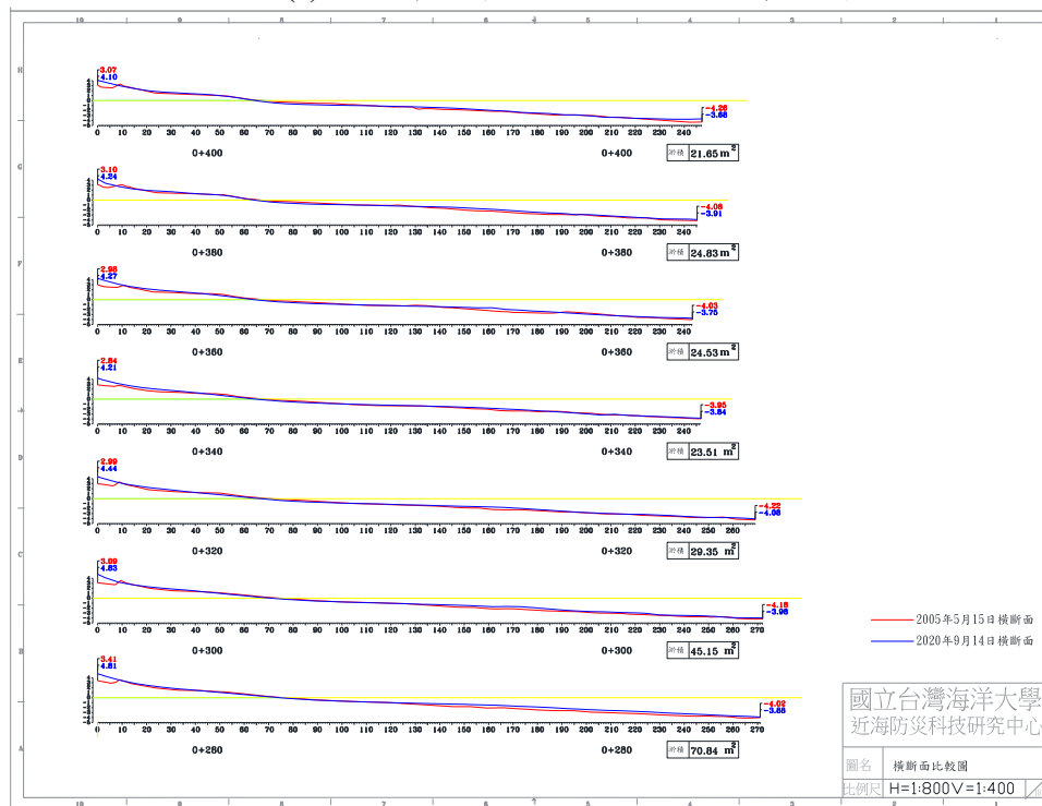
圖 4-7(d) 2020 年 9 月 14 日 B 監測區橫斷面比較圖
