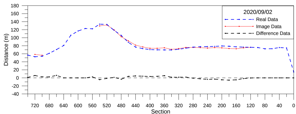
圖 3-23(a) 海岸線分析比較圖(2020/9/02)
