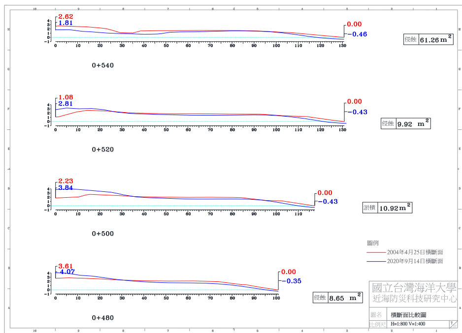
圖 4-6(d) 2020 年 9 月 14 日 A 監測區橫斷面比較圖
