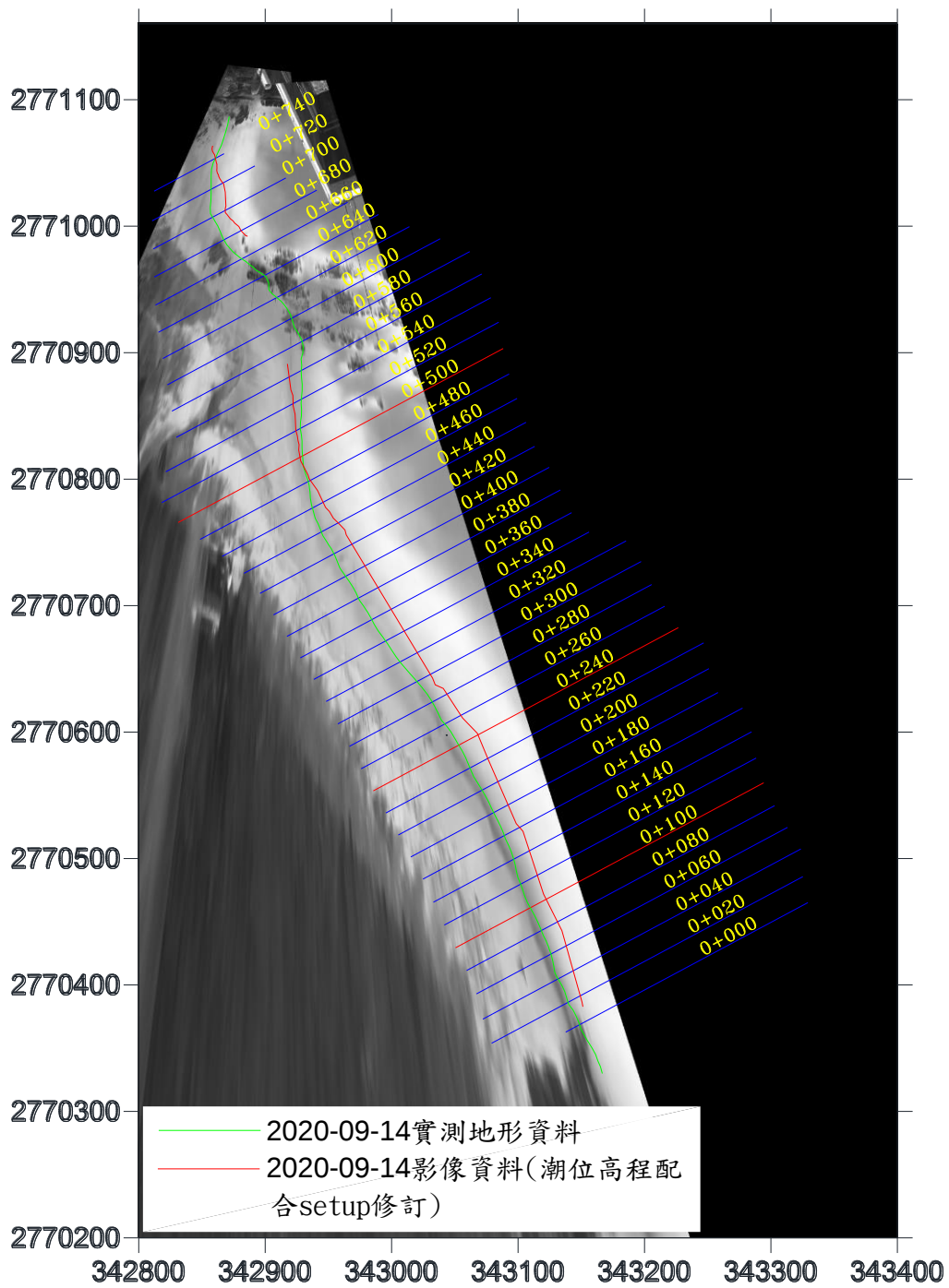
圖 3-22(b) 水位線分析結果圖(2020/9/14)
