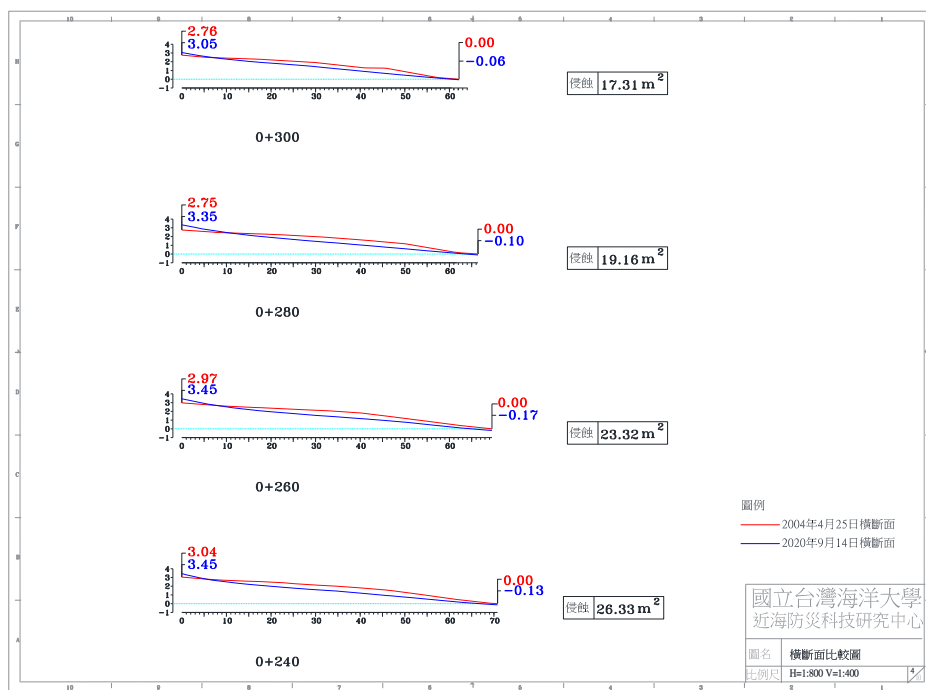
圖 4-6(g) 2020 年 9 月 14 日 A 監測區橫斷面比較圖
