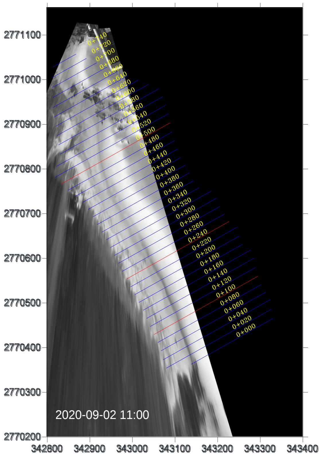
圖 4-21(a)鹽寮海岸地形影像全景圖(2020/09/02 11:00)
