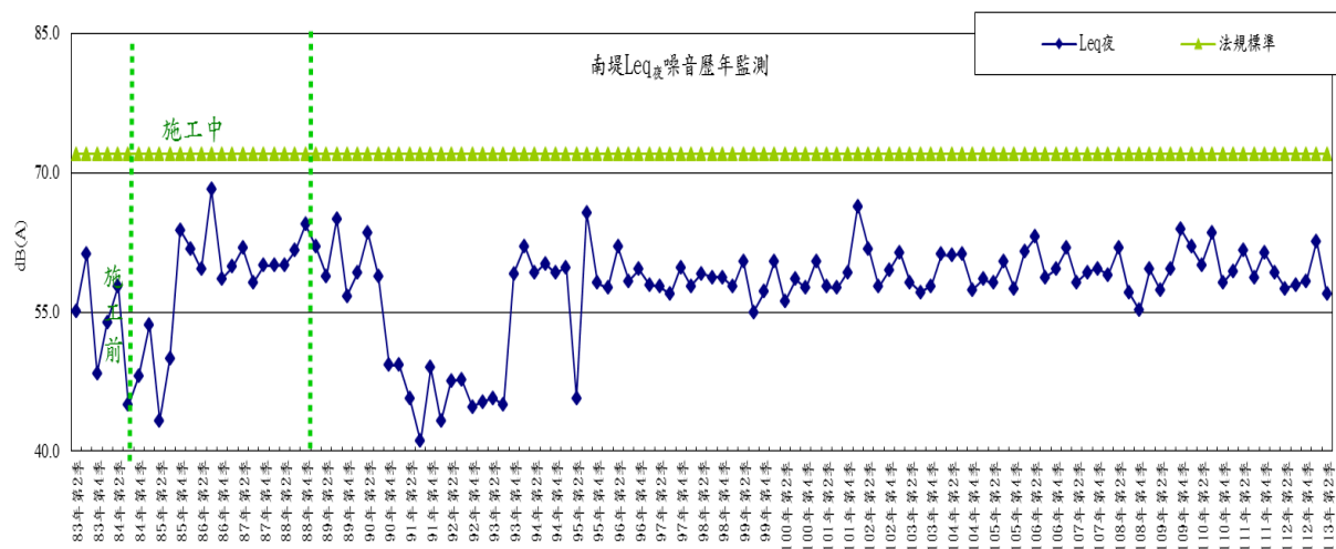
圖 2-6 南堤測點噪音(夜間)歷年監測變化趨勢圖
