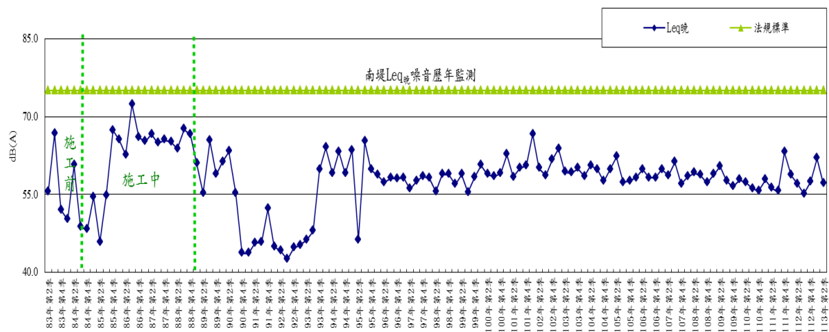
圖 2-5 南堤測點噪音(晚間)歷年監測變化趨勢圖
