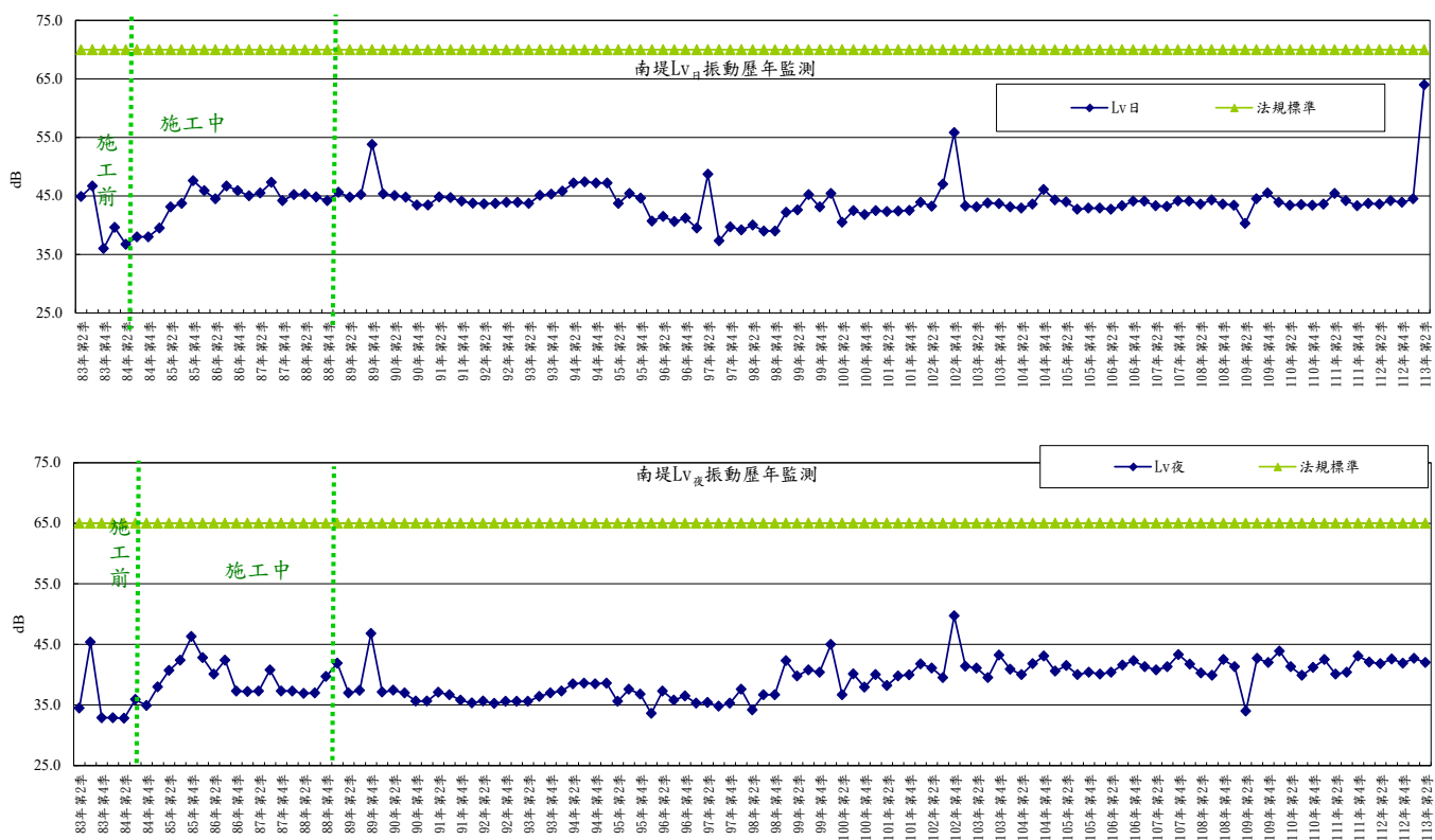
圖2-35 南堤測點振動歷年監測變化趨勢圖
