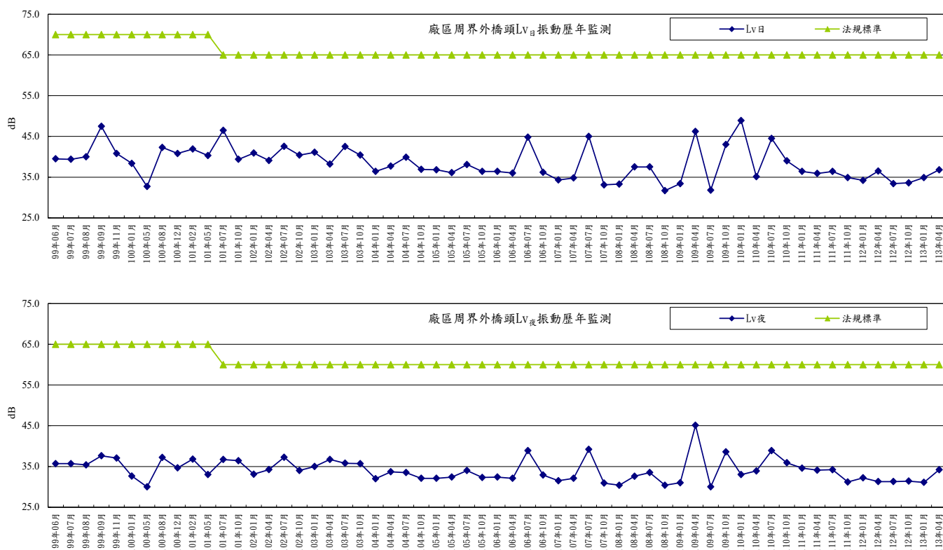
圖2-43 廠區周界外橋頭測點振動歷年監測變化趨勢圖
