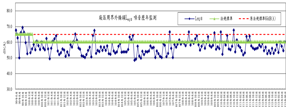
圖2-28 廠區周界外橋頭測點噪音(日間)歷年監測變化趨勢圖
