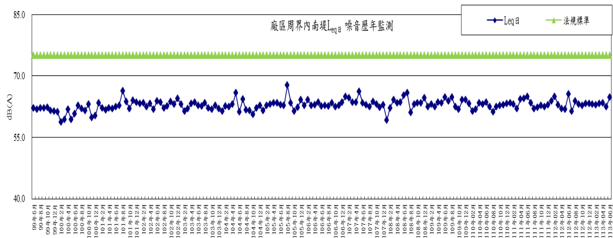
圖2-22 廠區周界內南堤測點噪音(日間)歷年監測變化趨勢圖
