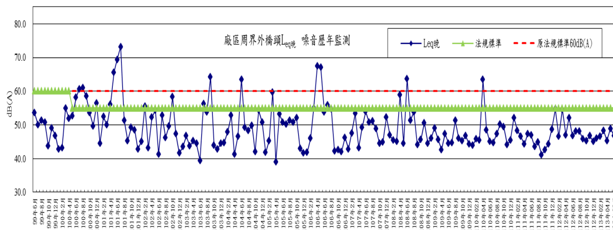
圖 2-29 廠區周界外橋頭測點噪音(晚間)歷年監測變化趨勢圖
