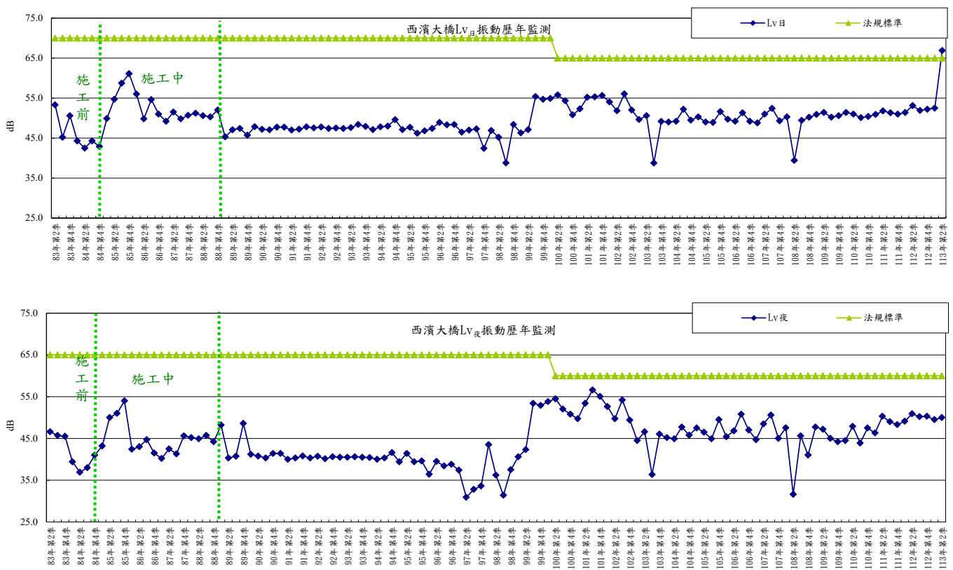
圖2-39 西濱大橋測點振動歷年監測變化趨勢圖
