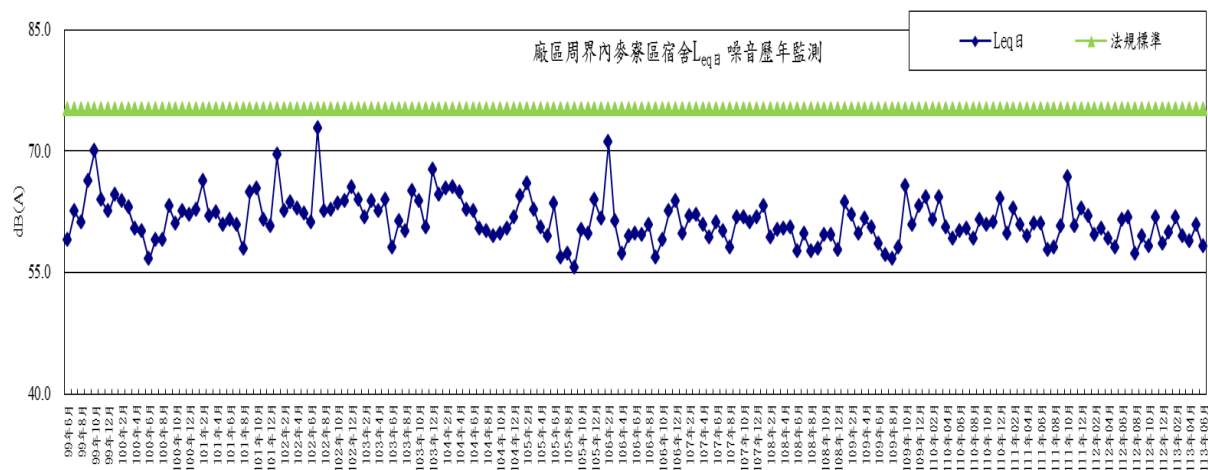
圖 2-25 廠區周界內麥寮區宿舍測點噪音(日間)歷年監測變化趨勢圖
