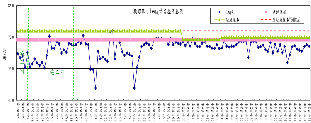
圖 2-8 橋頭國小測點噪音(晚間)歷年監測變化趨勢圖
