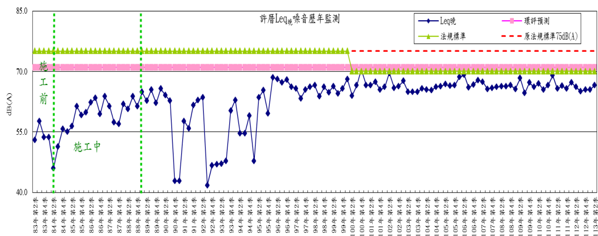
圖 2-11 許厝測點噪音(晚間)歷年監測變化趨勢圖
