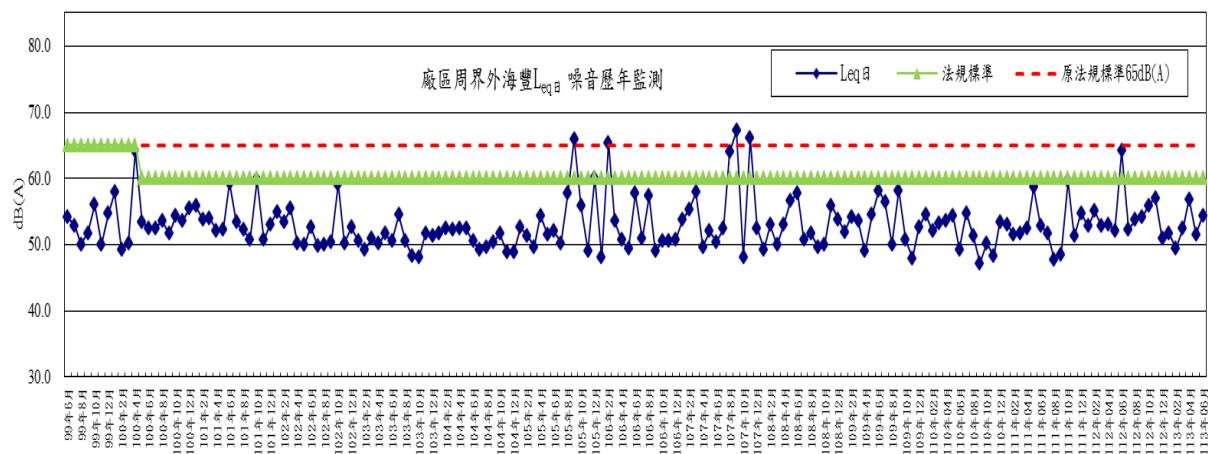
圖 2-31 廠區周界外海豐測點噪音(日間)歷年監測變化趨勢圖
