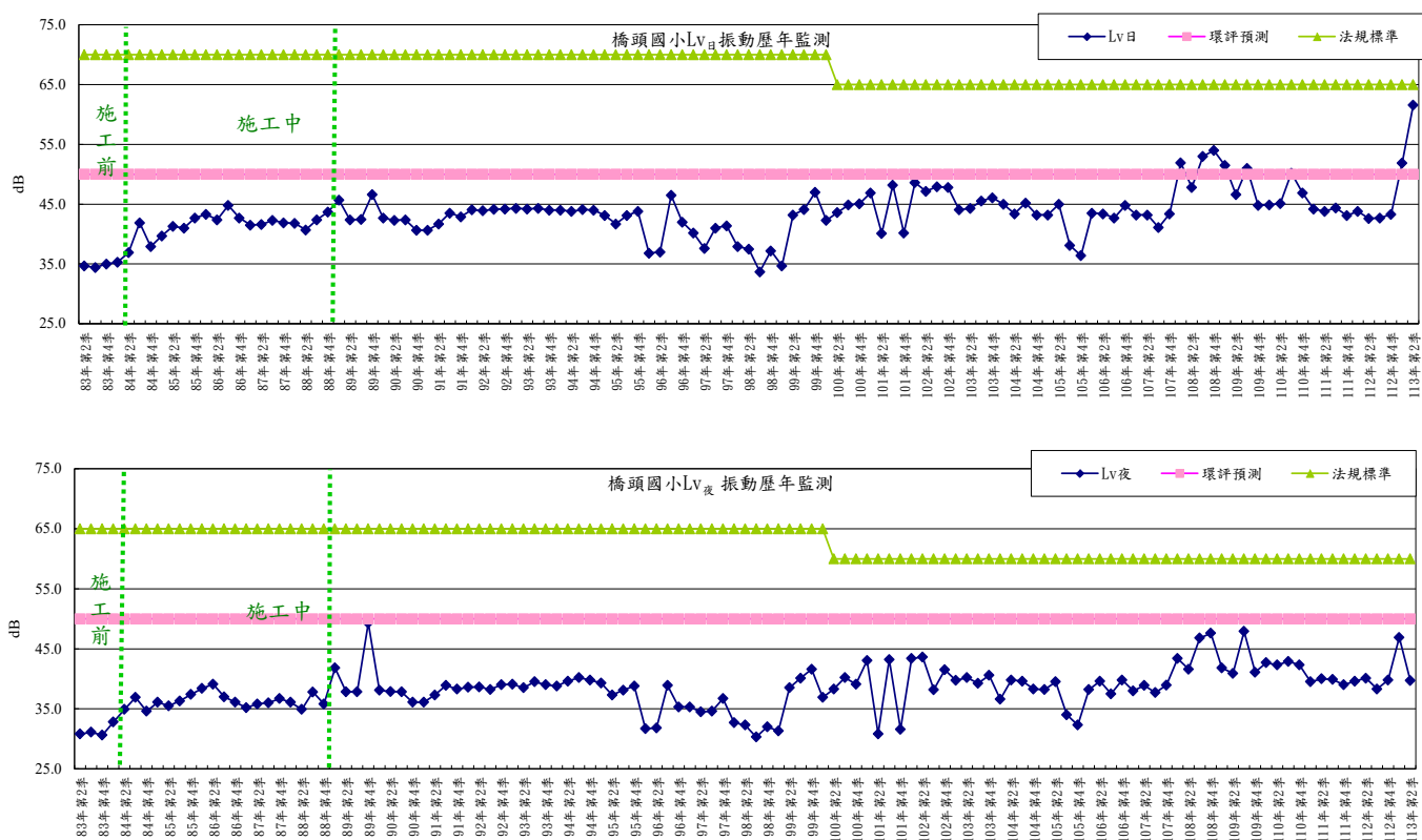
圖2-36 橋頭國小測點振動歷年監測變化趨勢圖
