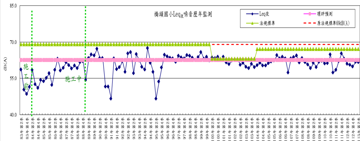
圖2-9 橋頭國小測點噪音(夜間)歷年監測變化趨勢圖
