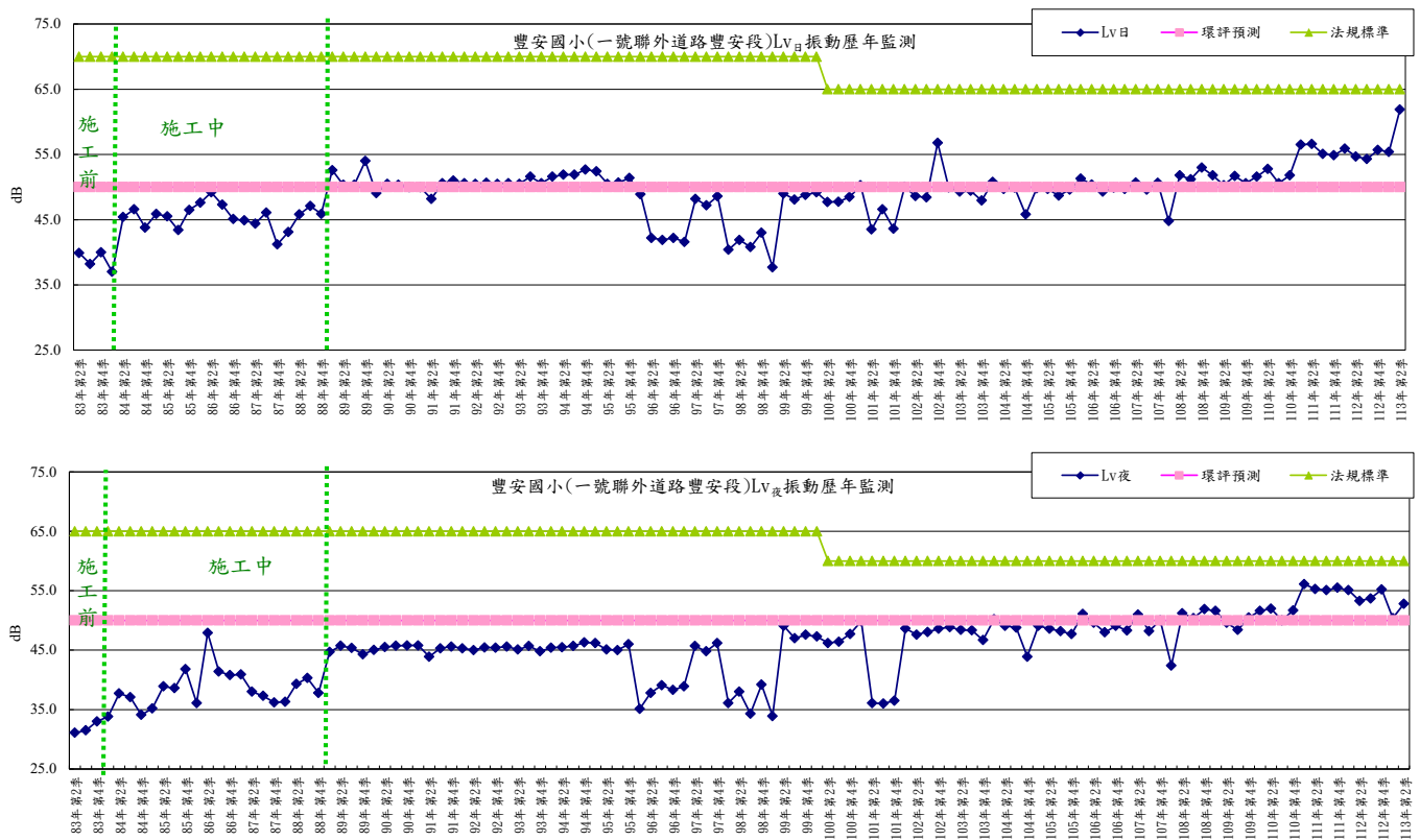
圖 2-38 豐安國小(一號聯外道路豐安段)測點振動歷年監測變化趨勢圖
