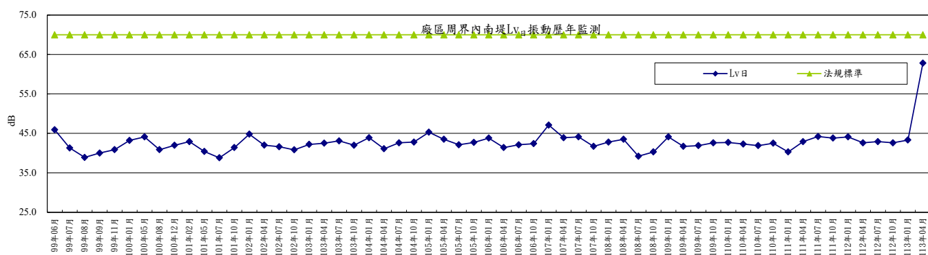
圖2-40 廠區周界內北堤測點振動歷年監測變化趨勢圖
