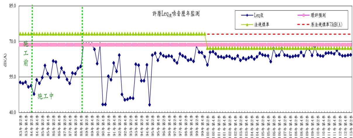
圖2-12 許厝測點噪音(夜間)歷年監測變化趨勢圖
