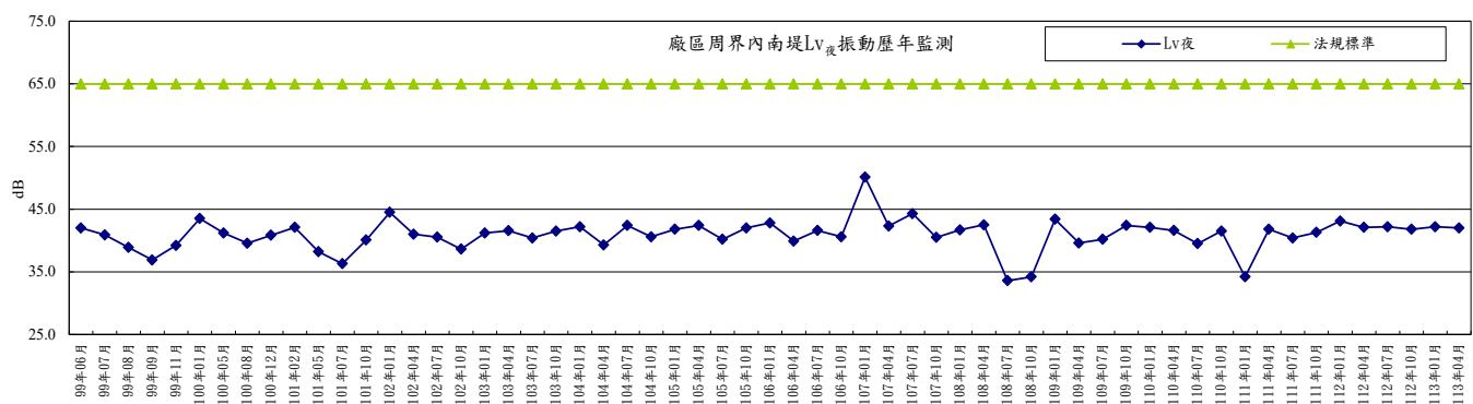
圖2-41 廠區周界內南堤測點振動歷年監測變化趨勢圖
