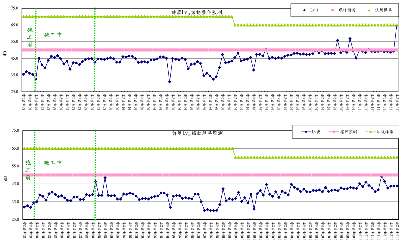
圖2-37 許厝測點振動歷年監測變化趨勢圖
