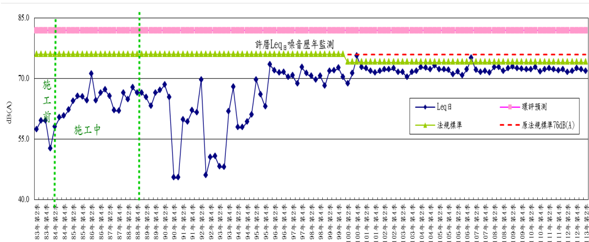
圖2-10 許厝測點噪音(日間)歷年監測變化趨勢圖
