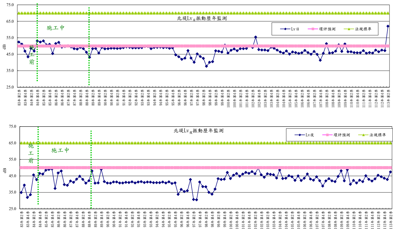
圖2-34 北堤測點振動歷年監測變化趨勢圖
