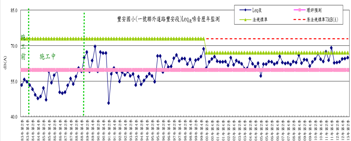
圖 2-15 豐安國小(一號聯外道路豐安段)測點噪音(夜間)歷年監測變化趨勢圖
