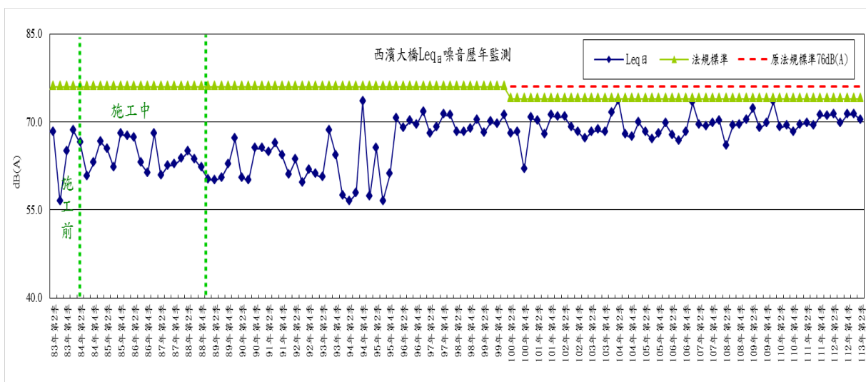
圖2-16 西濱大橋測點噪音(日間)歷年監測變化趨勢圖
