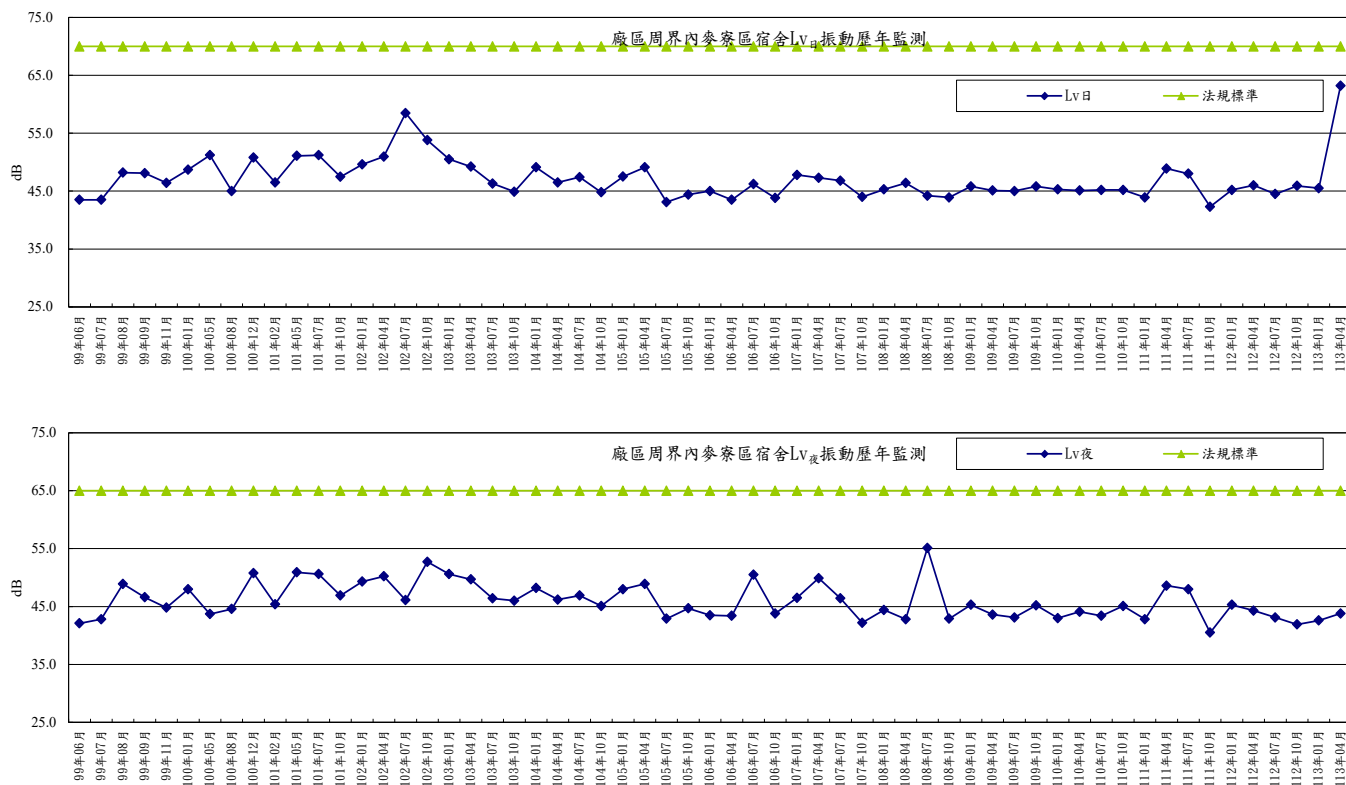
圖2-42 廠區周界內麥寮區宿舍測點振動歷年監測變化趨勢圖
