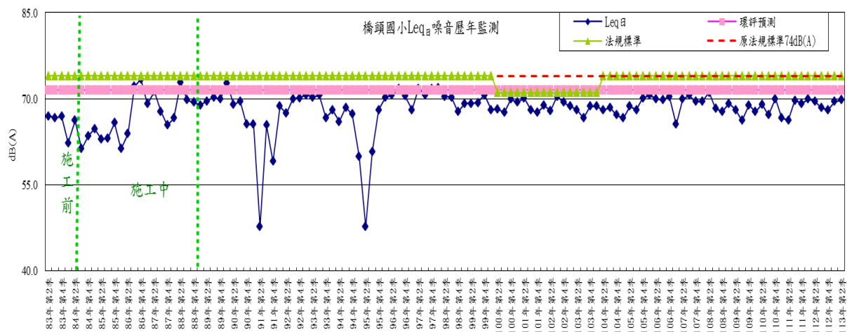
圖2-7 橋頭國小測點噪音(日間)歷年監測變化趨勢圖
