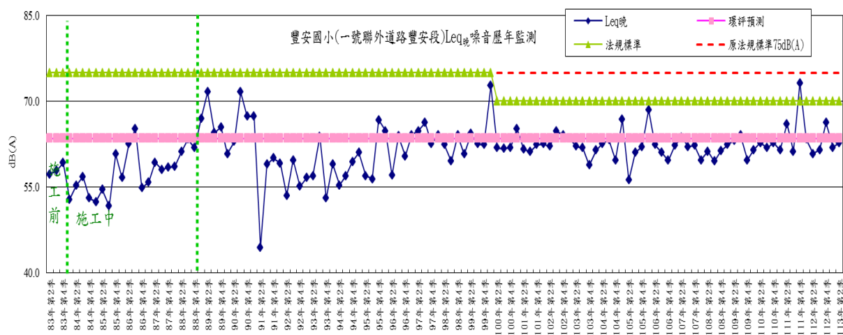
圖 2-14 豐安國小(一號聯外道路豐安段)測點噪音(晚間)歷年監測變化趨勢圖
