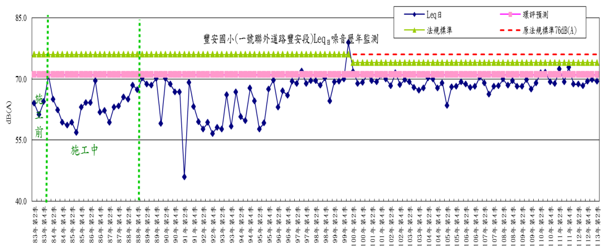
圖 2-12 豐安國小(一號聯外道路豐安段)測點噪音(日間)歷年監測變化趨勢圖
