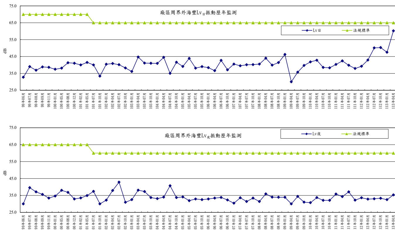
圖2-44 廠區周界外海豐測點振動歷年監測變化趨勢圖
