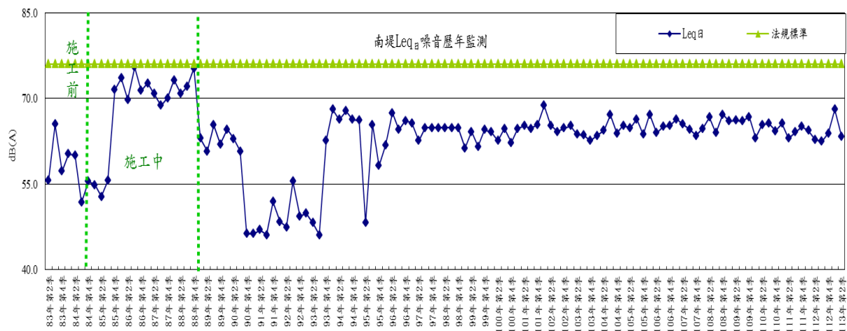
圖2-4 南堤測點噪音(日間)歷年監測變化趨勢圖
