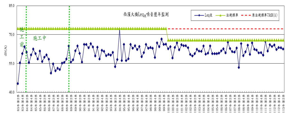
圖 2-18 西濱大橋測點噪音(夜間)歷年監測變化趨勢圖
