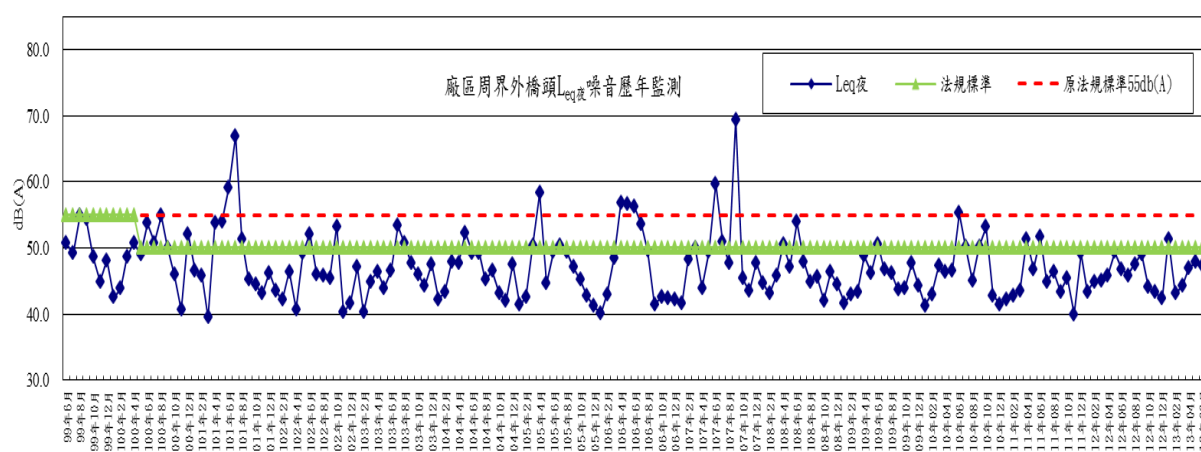
圖2-30 廠區周界外橋頭測點噪音(夜間)歷年監測變化趨勢圖
