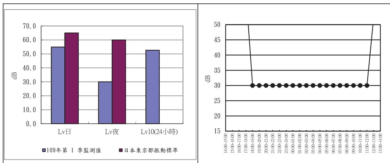
圖 2.3-5 五條港出入管制 109 年度第 1 季振動監測成果分析圖及逐時變化圖
