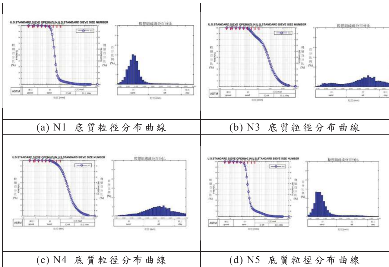
圖 2.9.2-2 海域潮間帶底質粒徑分布曲線
