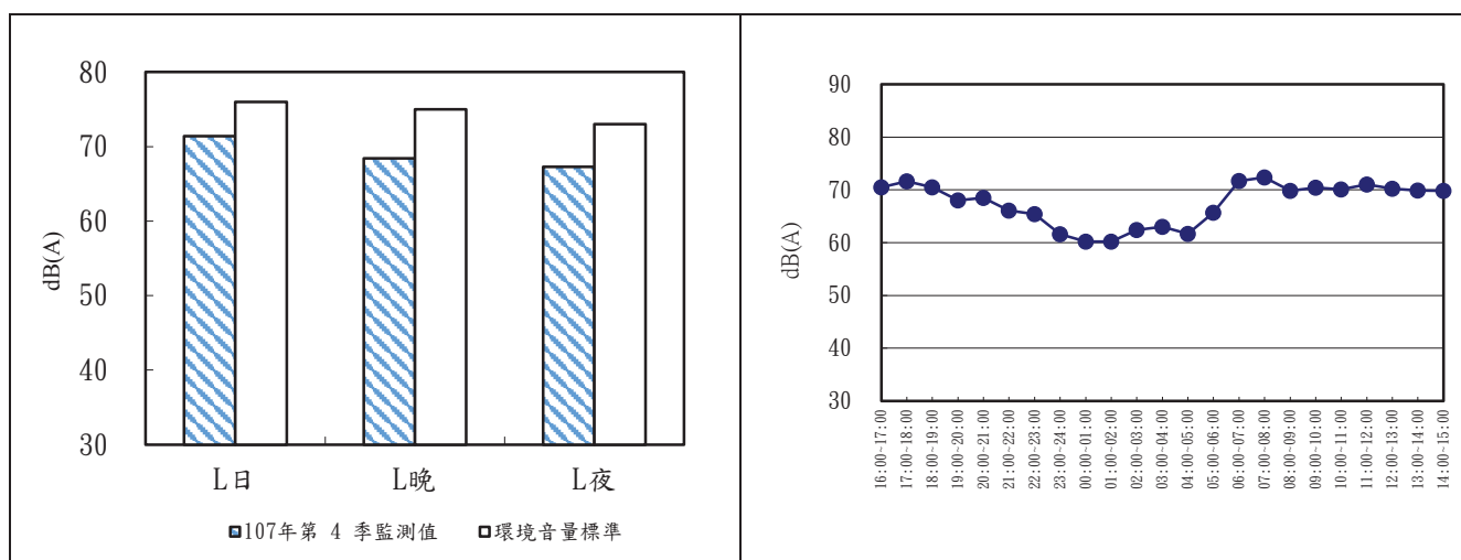
圖 2.2-2 海豐橋 109 年第 1 季噪音監測成果分析圖及逐時變化圖
