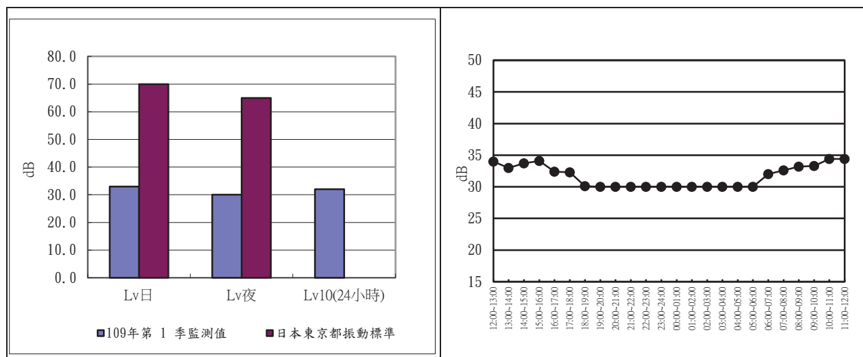
圖 2.3-4 海口橋 109 年度第 1 季振動監測成果分析圖及逐時變化圖
