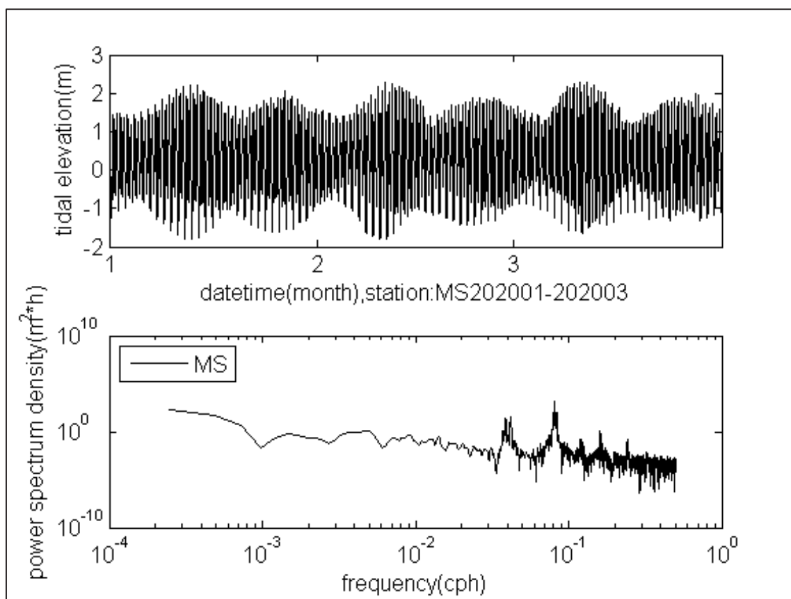
圖 2.13-3 MS 測站 2020 年 01~03 月實測潮位頻譜與逐時變化圖
