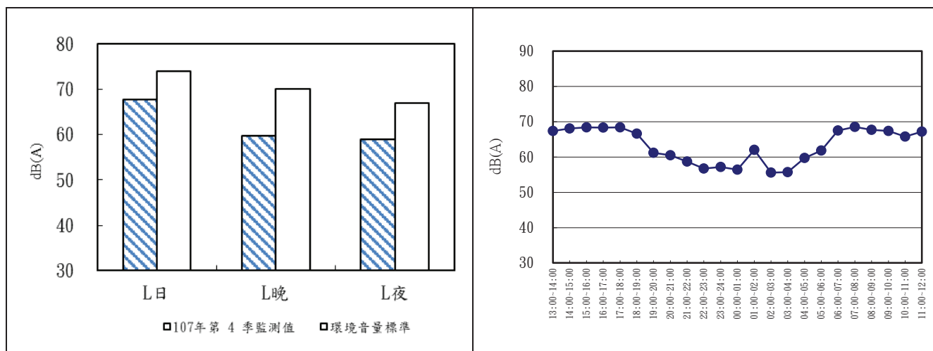
圖 2.2-1 安西府 109 年第 1 季噪音監測成果分析圖及逐時變化圖
