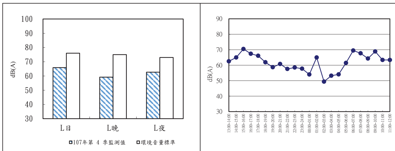
圖 2.2-4 海口橋 109 年第 1 季噪音監測成果分析圖及逐時變化圖
