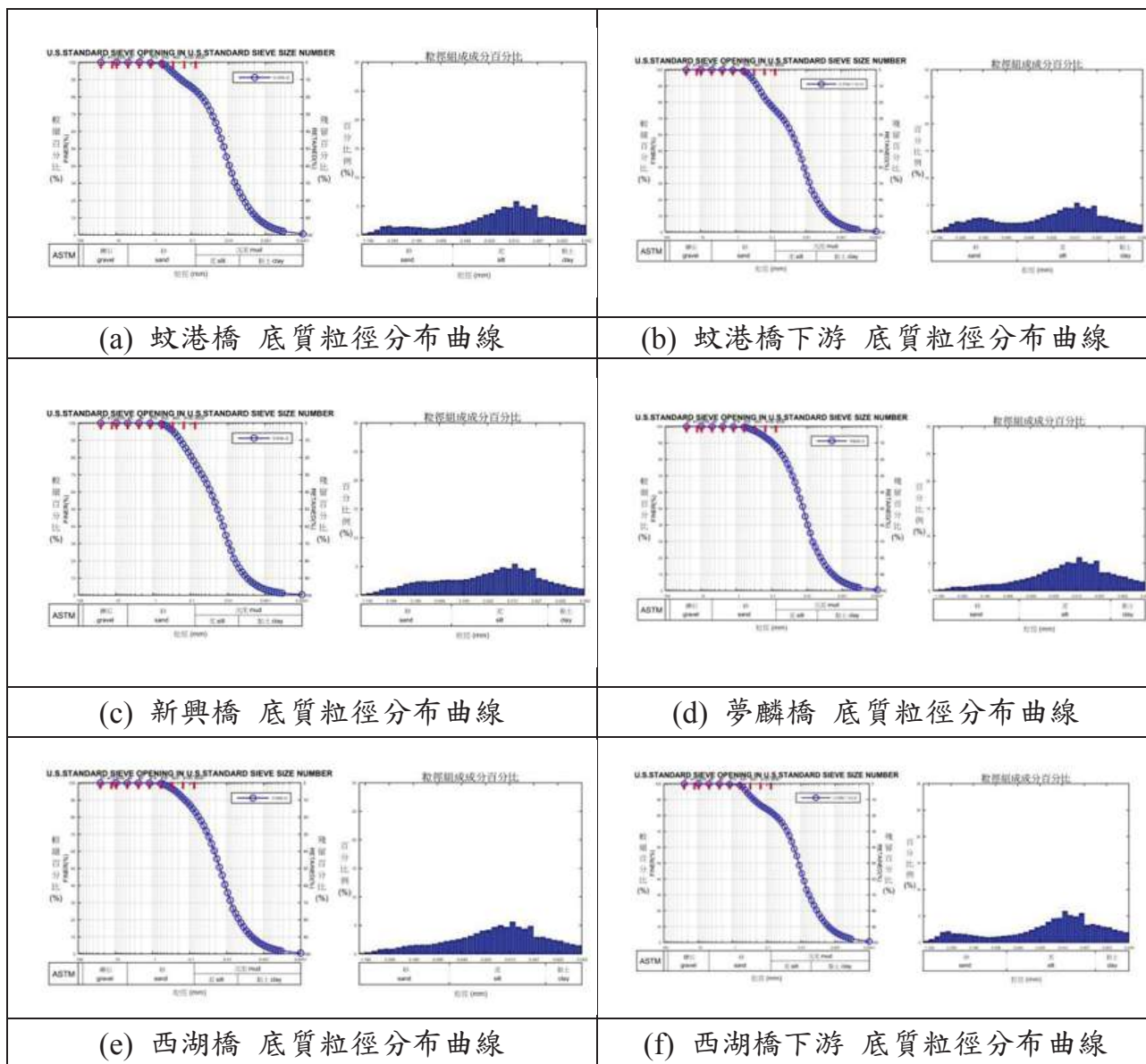
圖 2.9.2-3 陸域底質粒徑分布曲線
