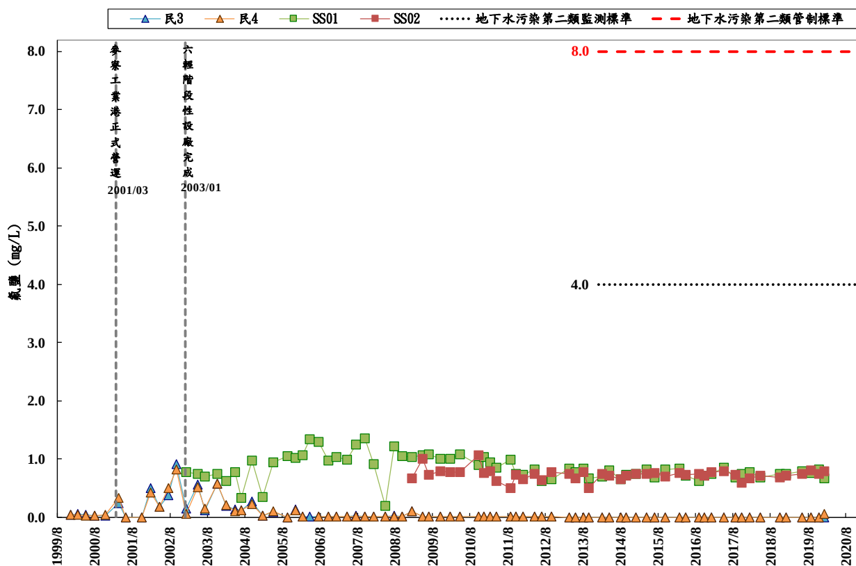
圖 3.1.6-4 氯鹽歷年濃度測值變化
