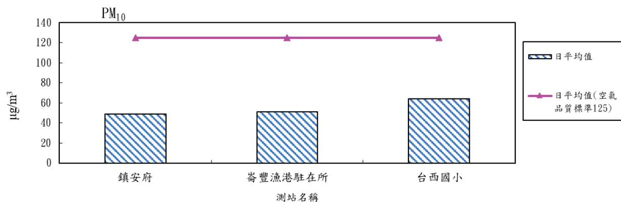
圖 2.1-9 109 年度第 1 季各測站 PM 10 日平均值比較分析圖
