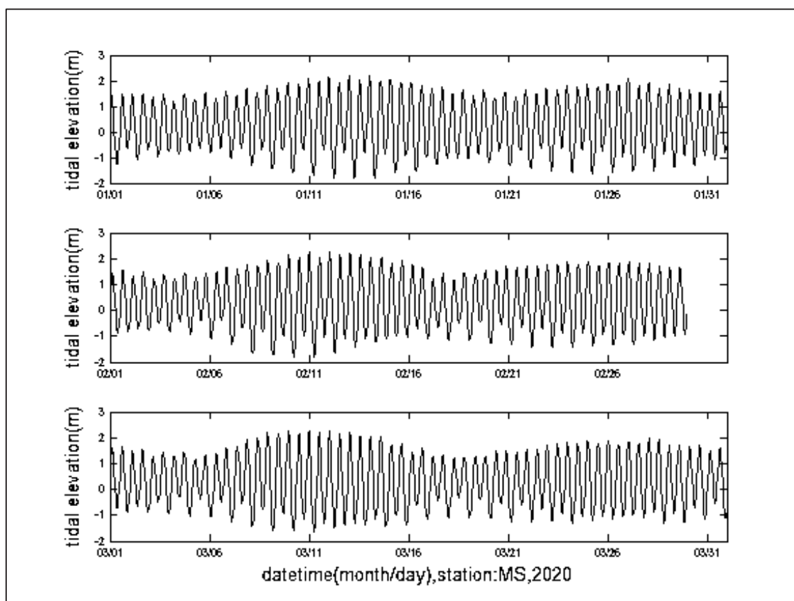
圖 2.13-1 MS 測站 2020 年 01~03 月各月實測潮位逐時變化圖
