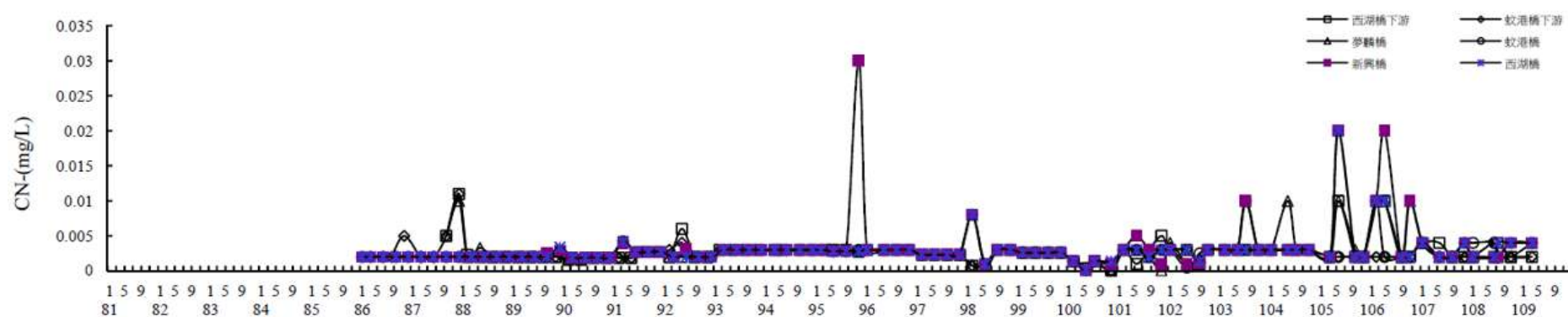
圖 3.1.8-1 離島工業區陸域河口歷年水質變化圖(續 25)
