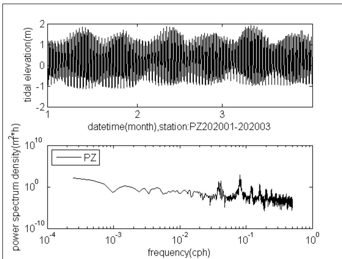
圖 2.13-4 PZ 測站 2020 年 01~03 月實測潮位頻譜與逐時變化圖
