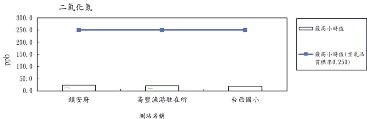
圖 2.1-4 109 年度第 1 季各測站二氧化氮(NO 2 )最高小時值比較分析圖
