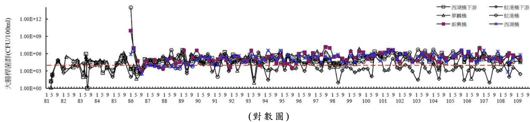
圖 3.1.8-1 離島工業區陸域河口歷年水質變化圖(續 7)
