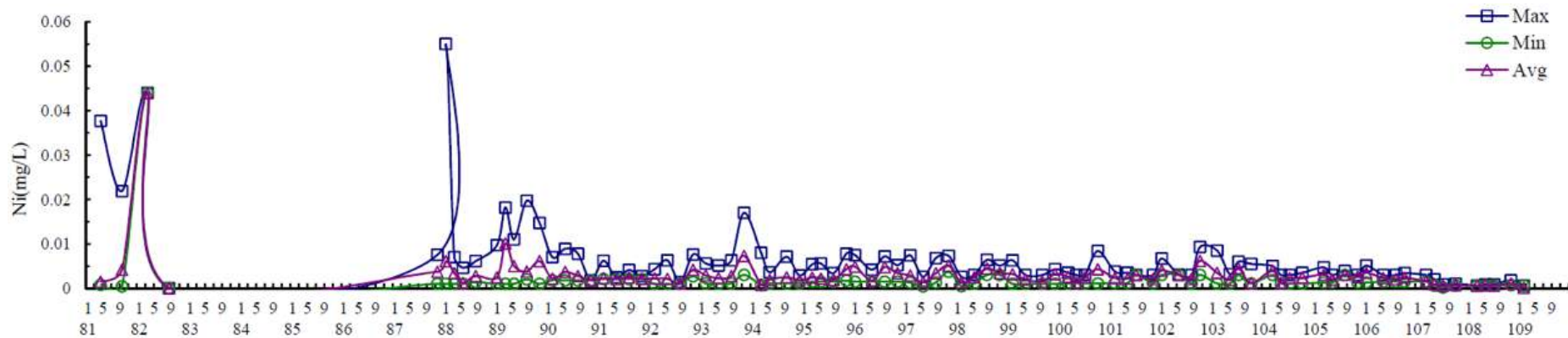
圖 3.1.9-20 離島工業區海域歷年水質變化圖(Ni)
