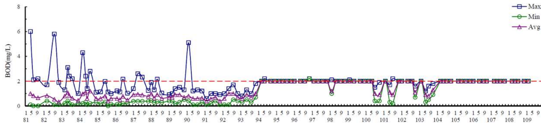
圖 3.1.9-4 離島工業區海域歷年水質變化圖(BOD)
