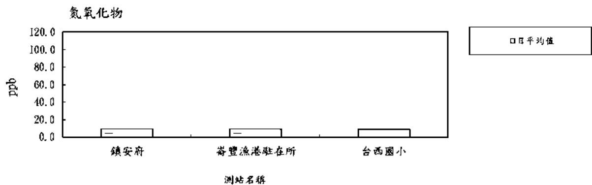
圖 2.1-3 109 年度第 1 季各測站氮氧化物(NO x )日平均值比較分析圖
