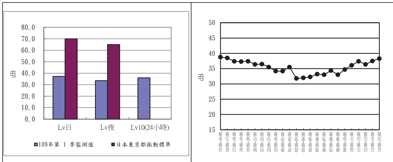
圖 2.3-2 海豐橋 109 年度第 1 季振動監測成果分析圖及逐時變化圖
