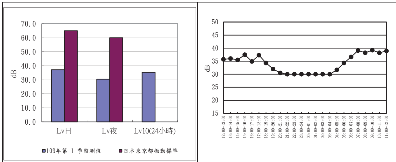
圖 2.3-1 安西府 109 年度第 1 季振動監測成果分析圖及逐時變化圖
