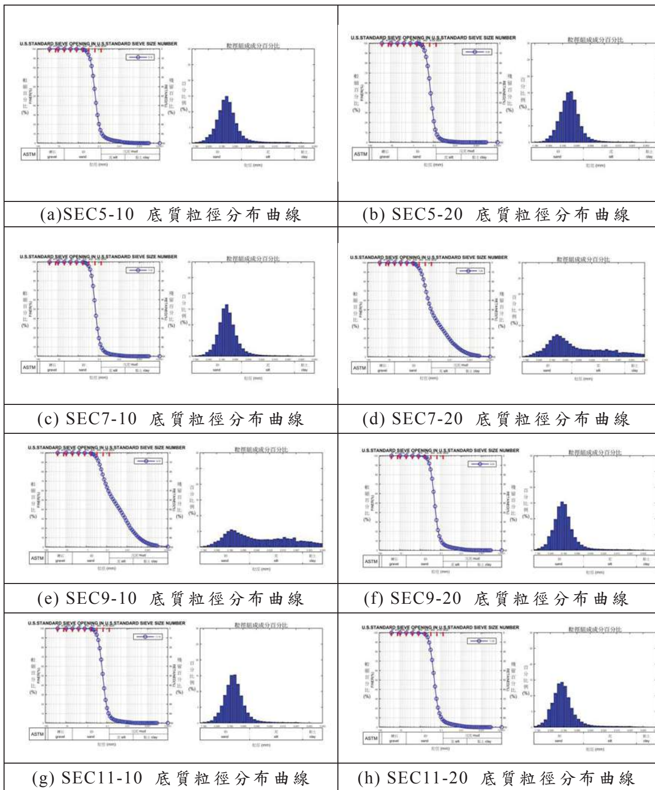
圖 2.9.2-1 海域潮間帶底質粒徑分布曲線
