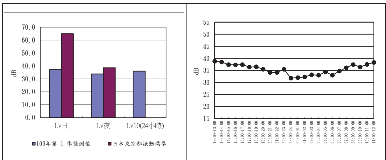
圖 2.3-3 崙豐國小 109 年度第 1 季振動監測成果分析圖及逐時變化圖
