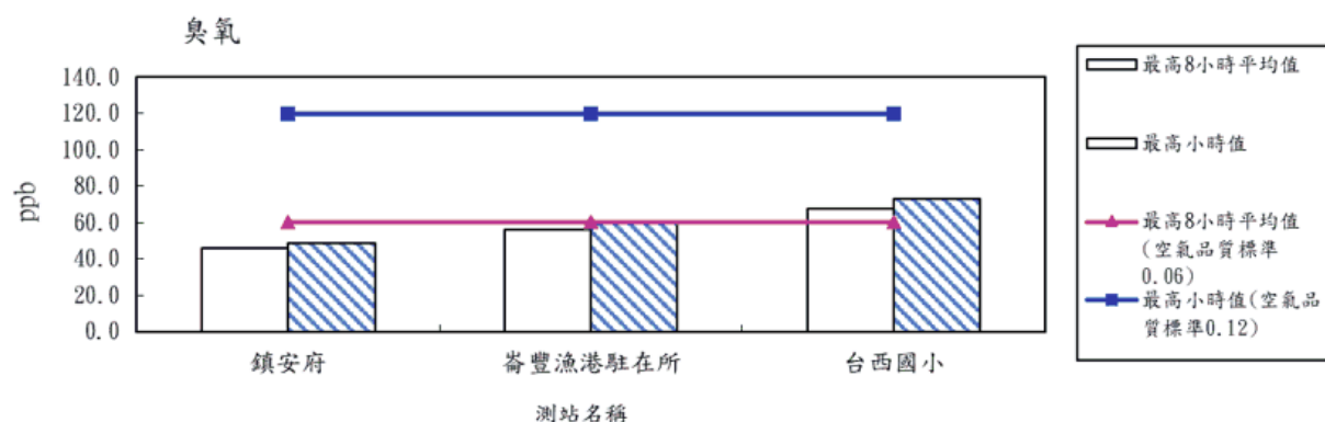
圖 2.1-5 109 年度第 1 季各測站臭氧(O 3 )最高 8 小時平均值及最高小時值比較分析圖
