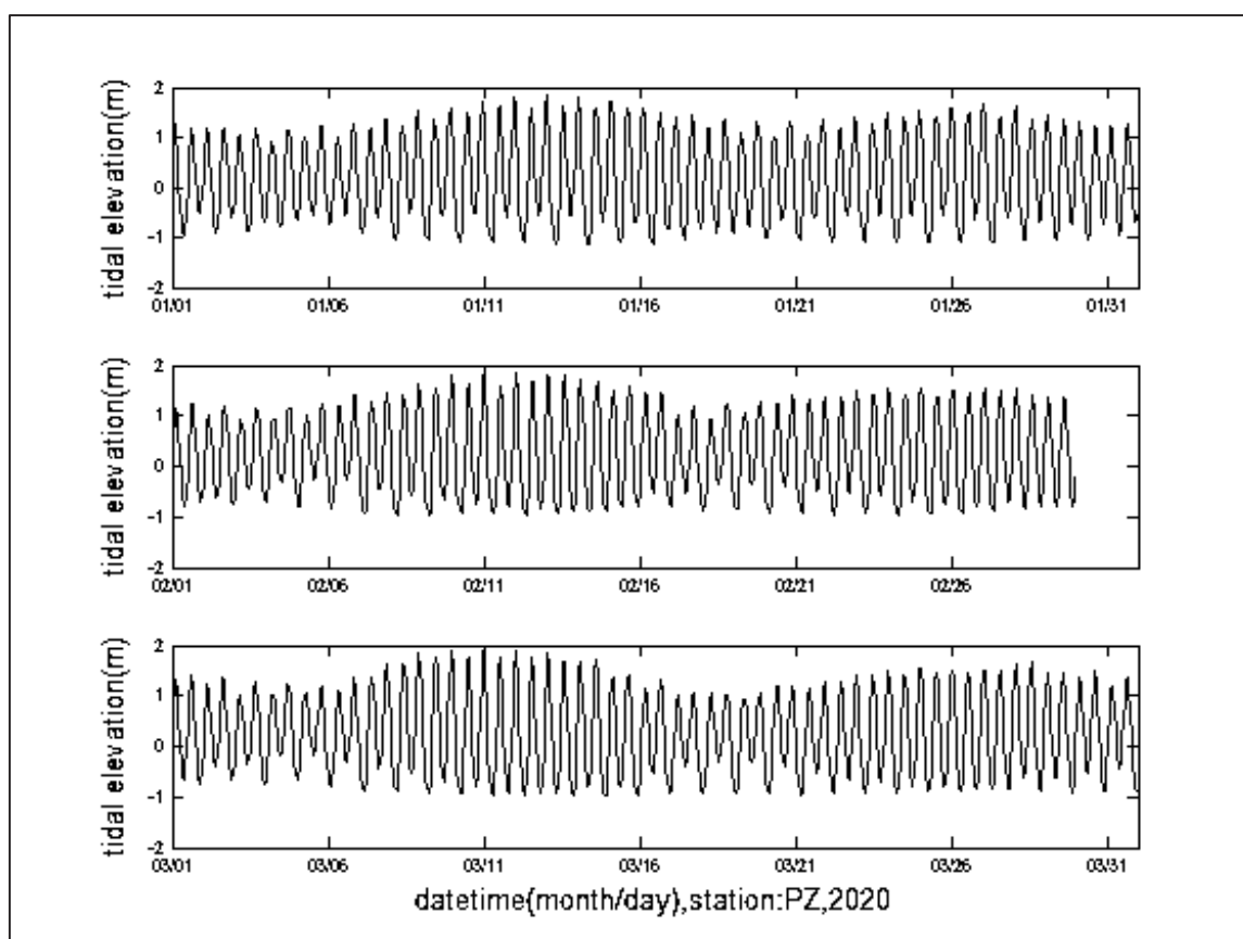
圖 2.13-2 PZ 測站 2020 年 01~03 月各月實測潮位逐時變化圖
