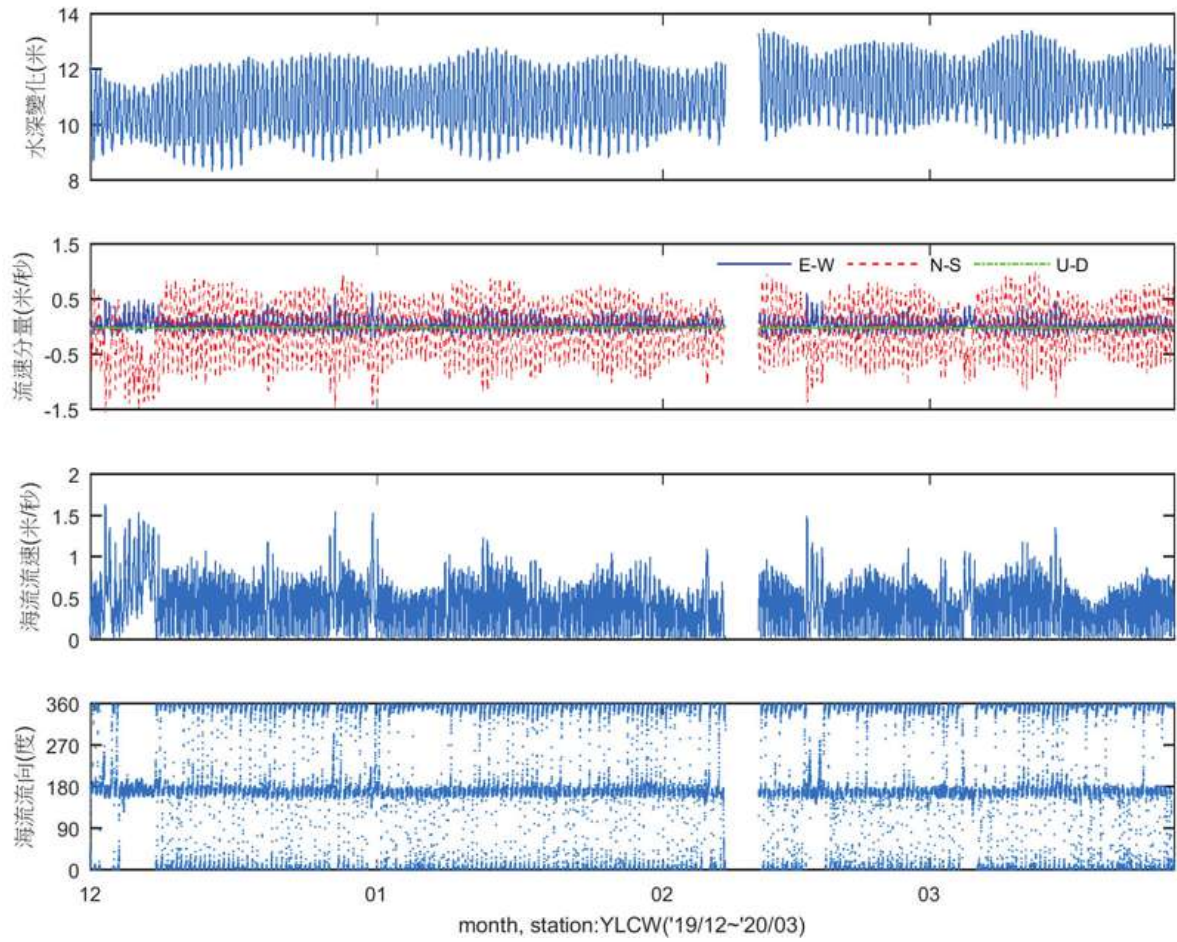
圖 2.13-10 YLCW 測站 2019 年 12 月~2020 年 3 月海流分量與流速流向時序列
