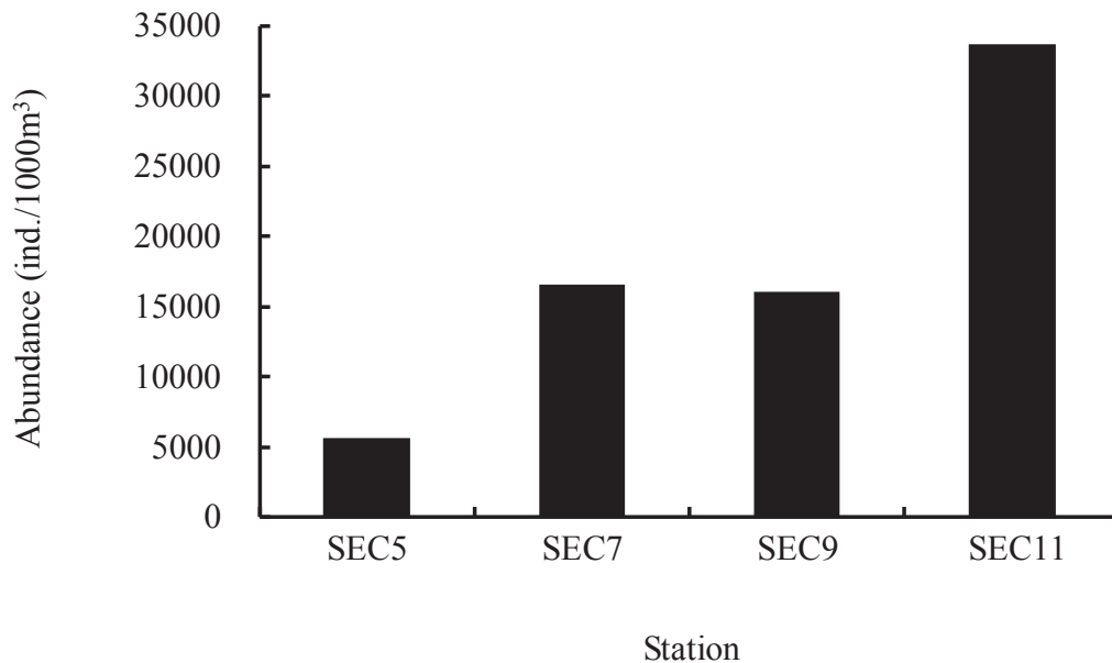
圖 2.10.6-8 雲林縣離島式基礎工業區沿海蟹幼生豐度 (109 年 03 月 25 日)
