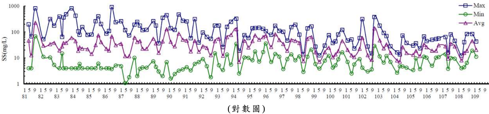
圖 3.1.9-5 離島工業區海域歷年水質變化圖(SS)
