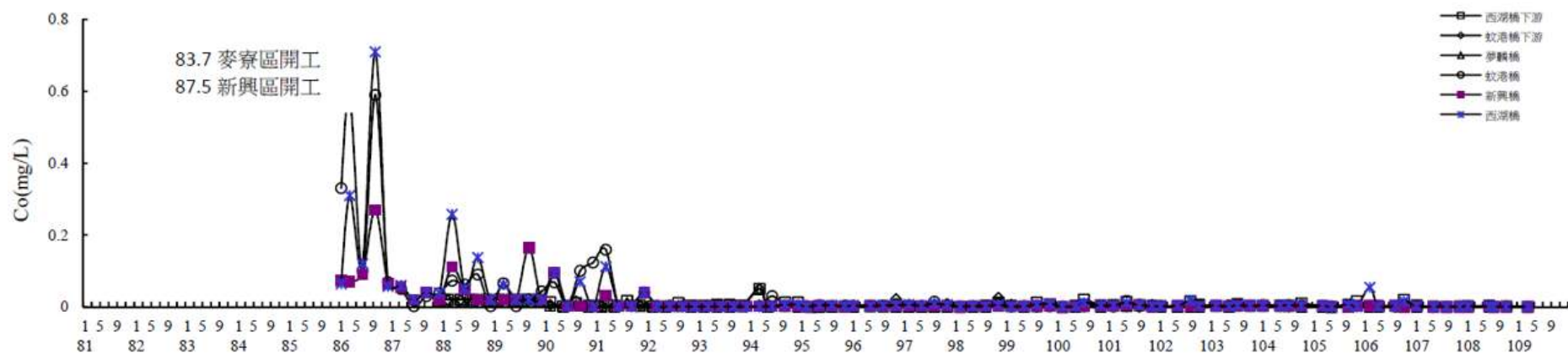
圖 3.1.8-1 離島工業區陸域河口歷年水質變化圖(續 24)
