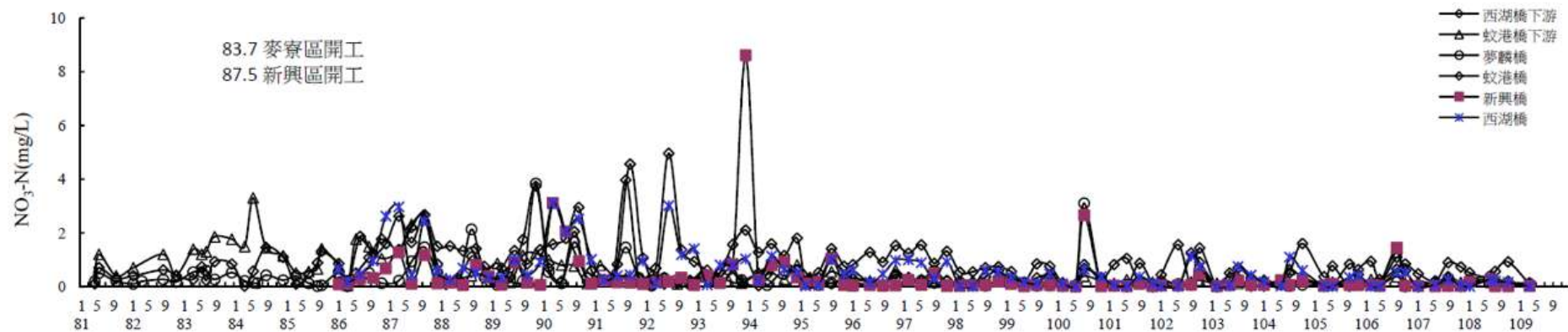
圖 3.1.8-1 離島工業區陸域河口歷年水質變化圖(續 8)
