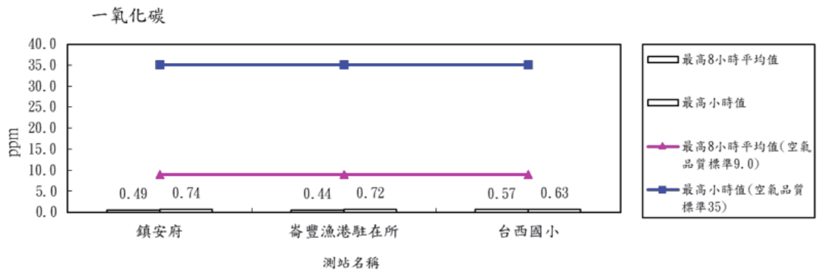
圖 2.1-1 109 年度第 1 季各測站一氧化碳(CO)最高 8 小時平均值及最高小時值比較分析圖
