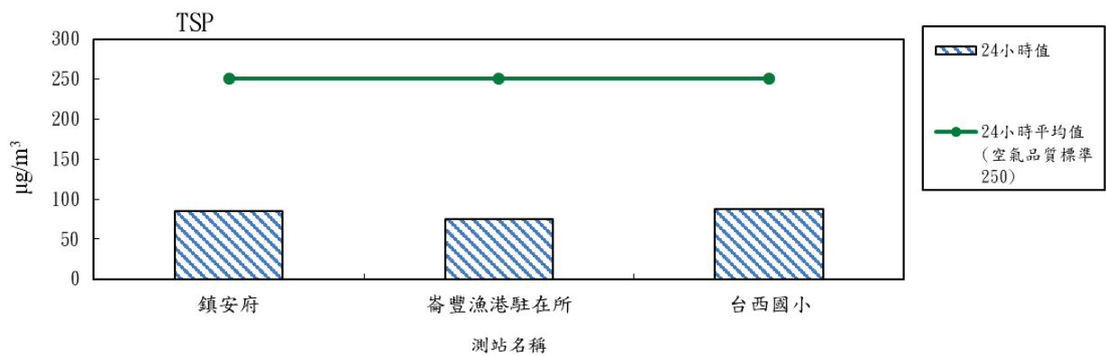
圖 2.1-8 109 年度第 1 季各測站 TSP 24 小時值比較分析圖
