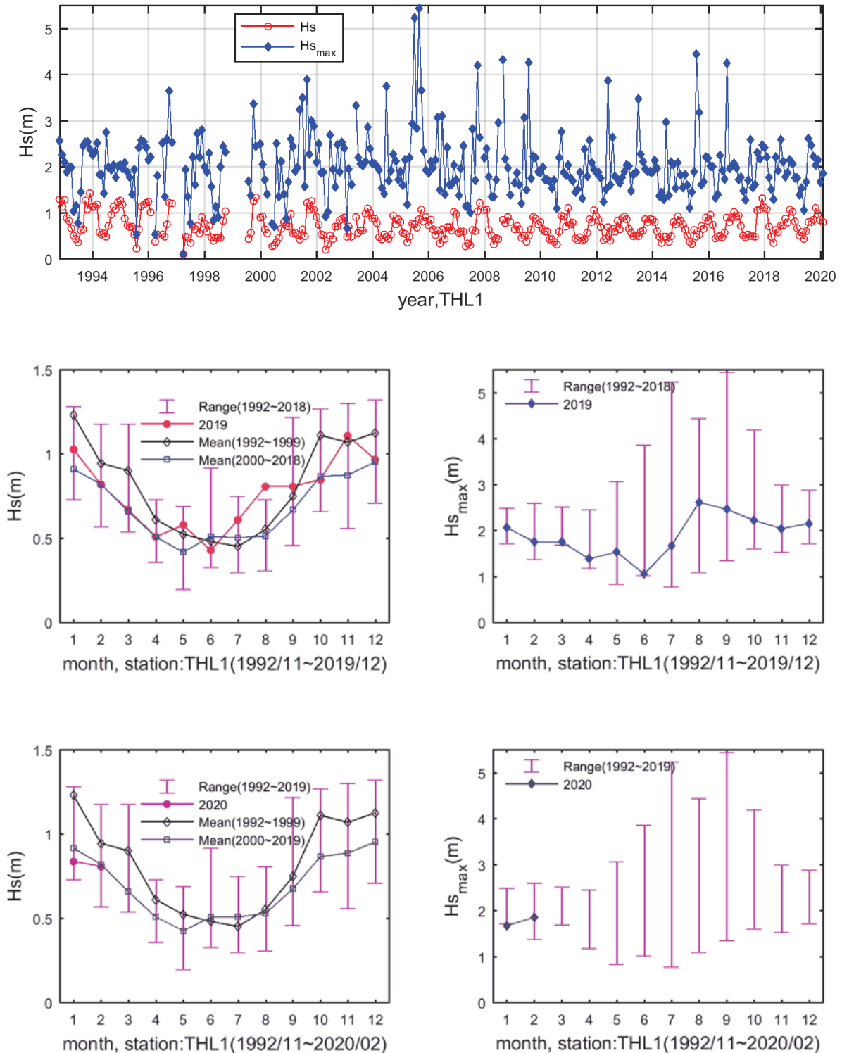
圖 2.13-8 歷年月平均及月最大示性波高時序列與分布範圍
