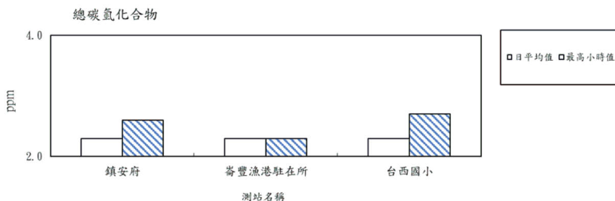
圖 2.1-6 109 年度第 1 季各測站總碳氫化合物(THC)日平均值及最高小時值比較分析圖
