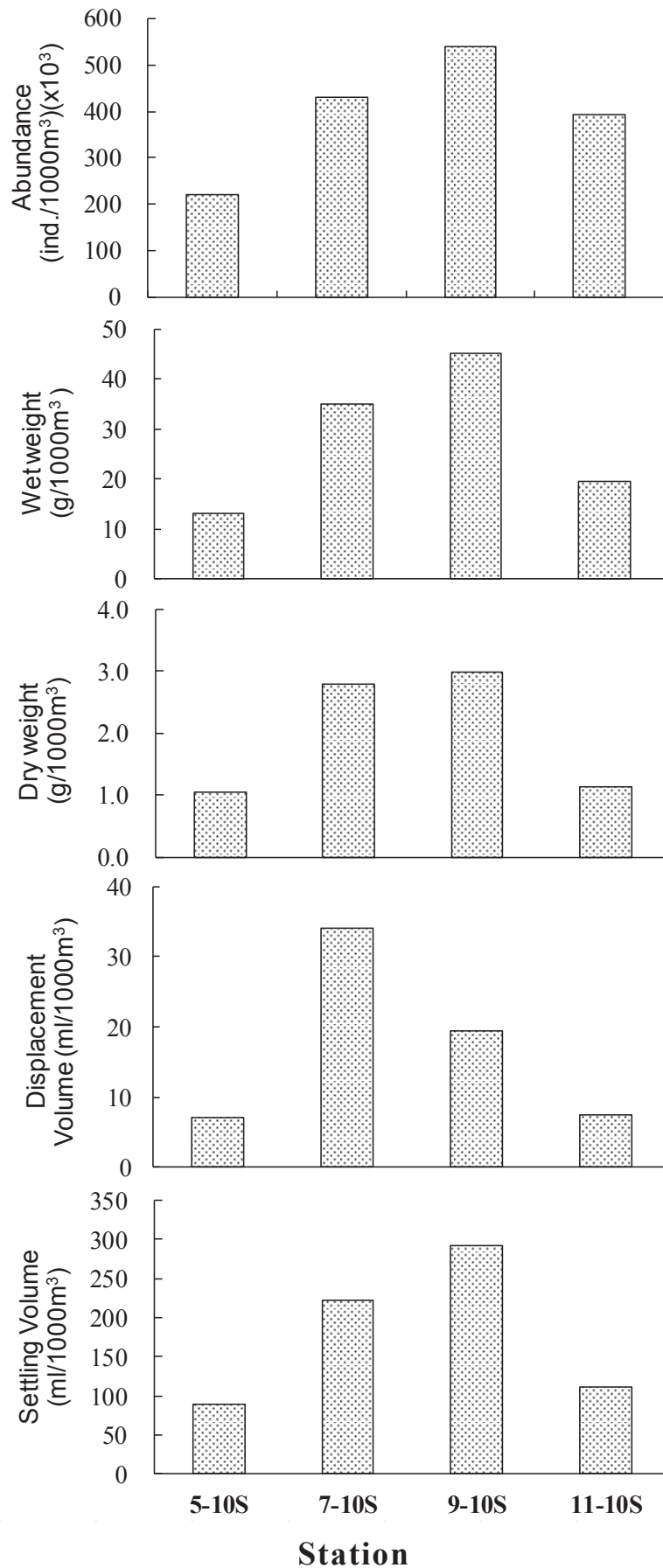
圖 2.10.1-1 民國 109 年 3 月 26 日雲林縣台西鄉 10 米水深表層各測站中浮游動物之豐度及生物量的變化圖
