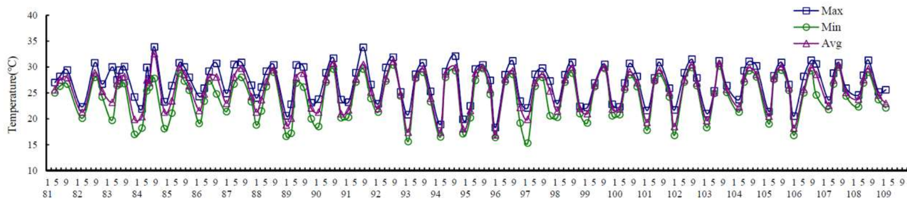
圖 3.1.9-2 離島工業區海域歷年水質變化圖(溫度)
