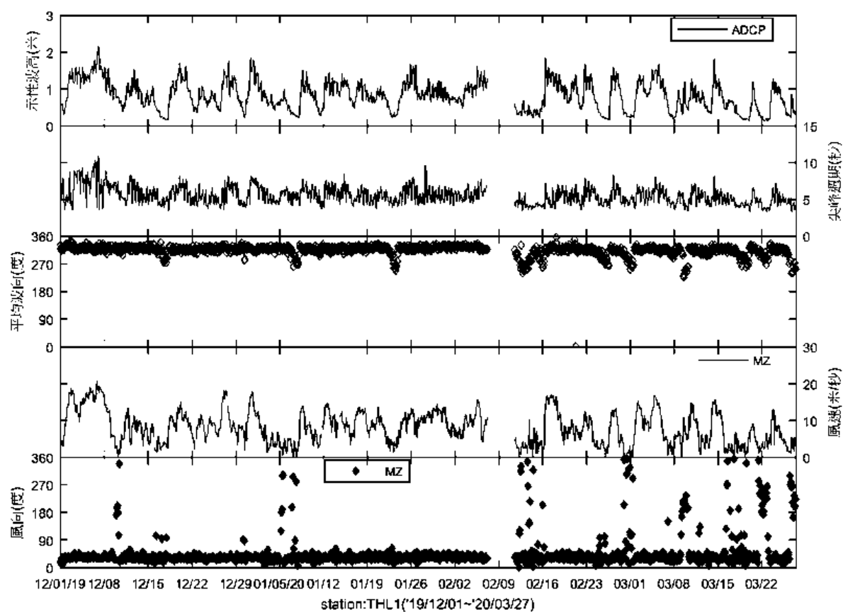
圖 2.13-6 THL1 測站 2019 年 12 月~2020 年 3 月波浪與風速風向時序列
