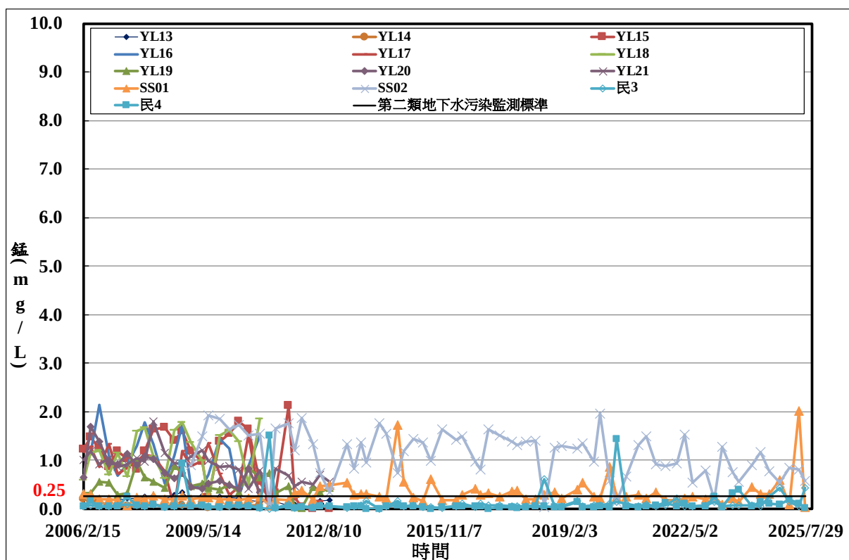
圖3.3 雲林離島計畫地下水錳濃度歷線圖
