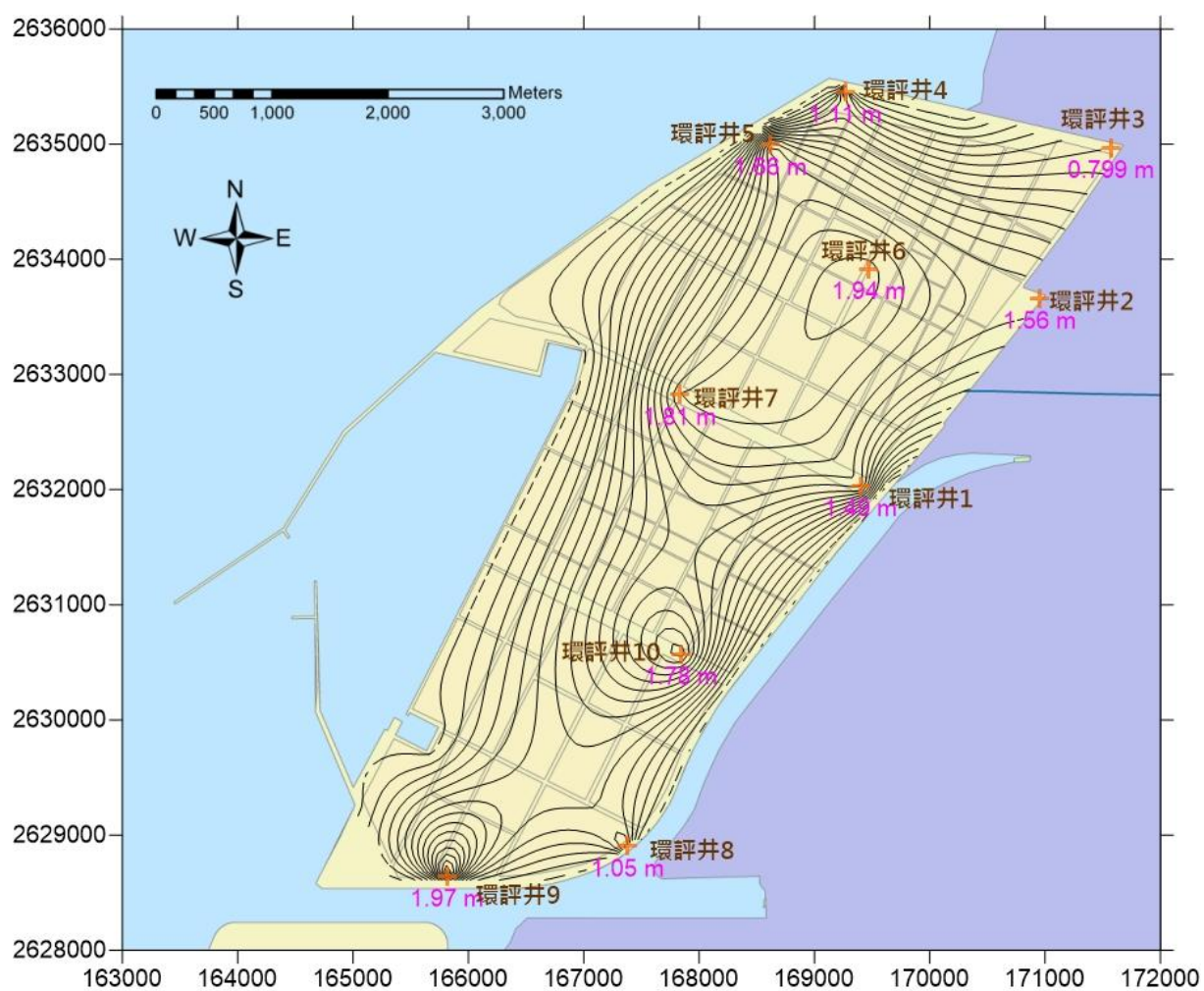
圖2.1 本季(7月至9月)採樣時地下水水位高程等值圖
