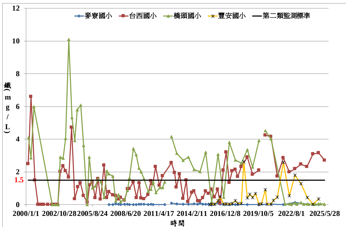
圖3.6 環保單位地下水鐵濃度歷線圖
