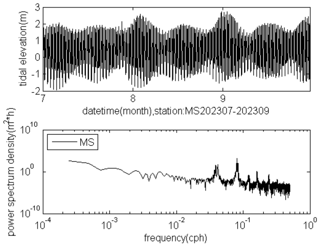
圖 2.13-3 MS 測站 2023 年 7~9 月實測潮位頻譜與逐時變化圖
