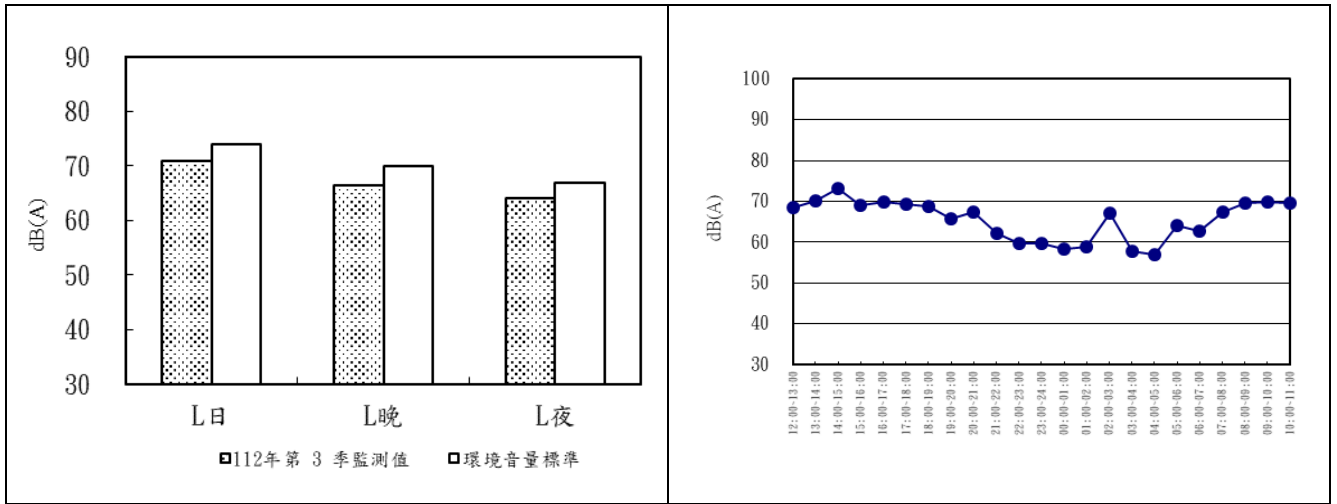
圖 2.2-1 安西府 112 年第 3 季噪音監測成果分析圖及逐時變化圖
