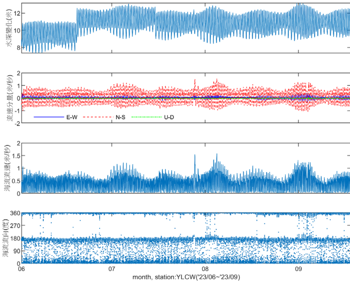
圖 2.13-10 YLCW 測站 2023 年 6 月~2023 年 9 月海流分量與流速流向時序列
