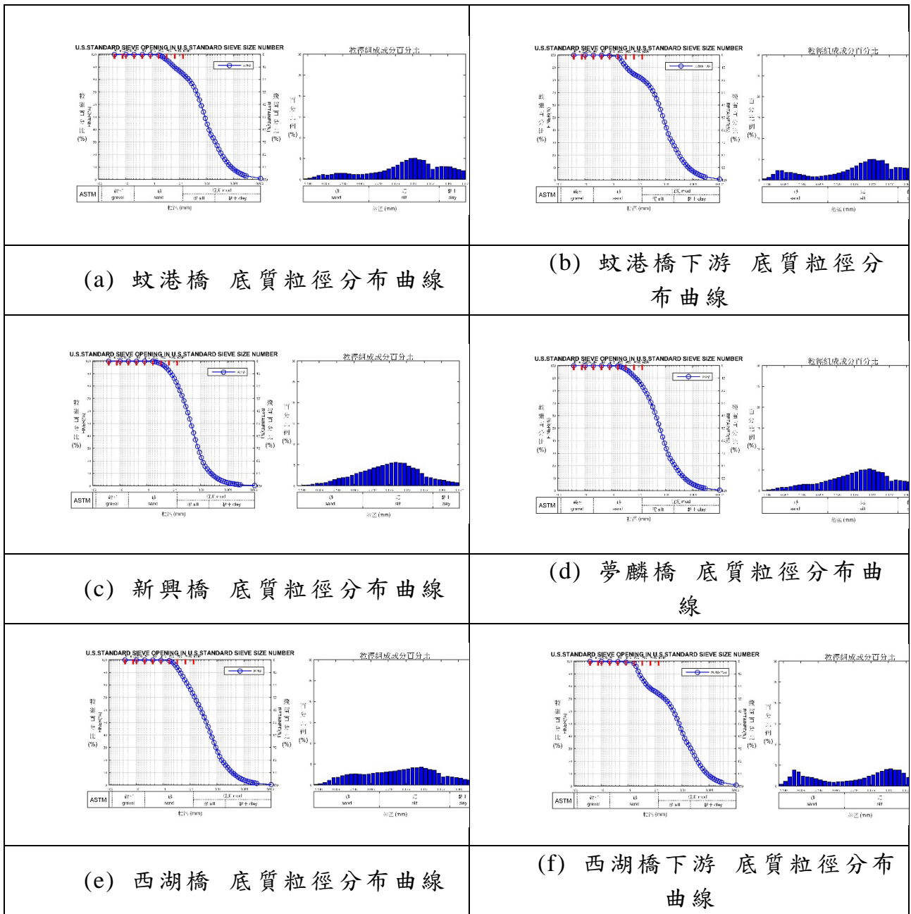
圖 2.9.2-4 陸域底質粒徑分布曲線
