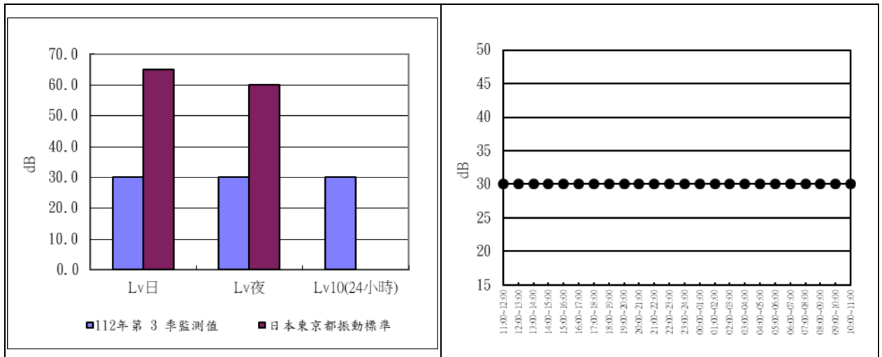
圖 2.3-5 五條港出入管制 112 年度第 3 季振動監測成果分析圖及逐時變化圖
