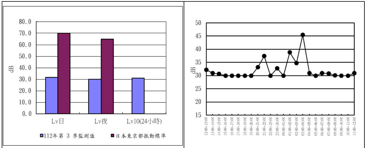
圖 2.3-4 海口橋 112 年度第 3 季振動監測成果分析圖及逐時變化圖
