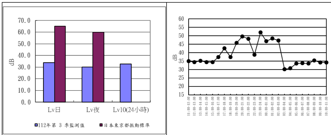
圖 2.3-1 安西府 112 年度第 3 季振動監測成果分析圖及逐時變化圖
