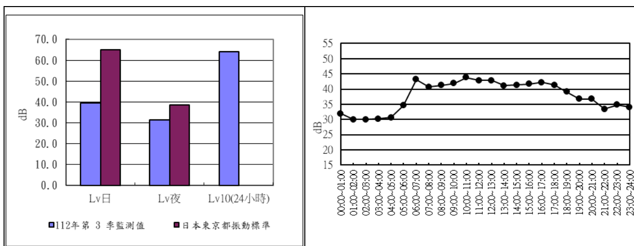
圖 2.3-3 崙豐國小 112 年度第 3 季振動監測成果分析圖及逐時變化圖
