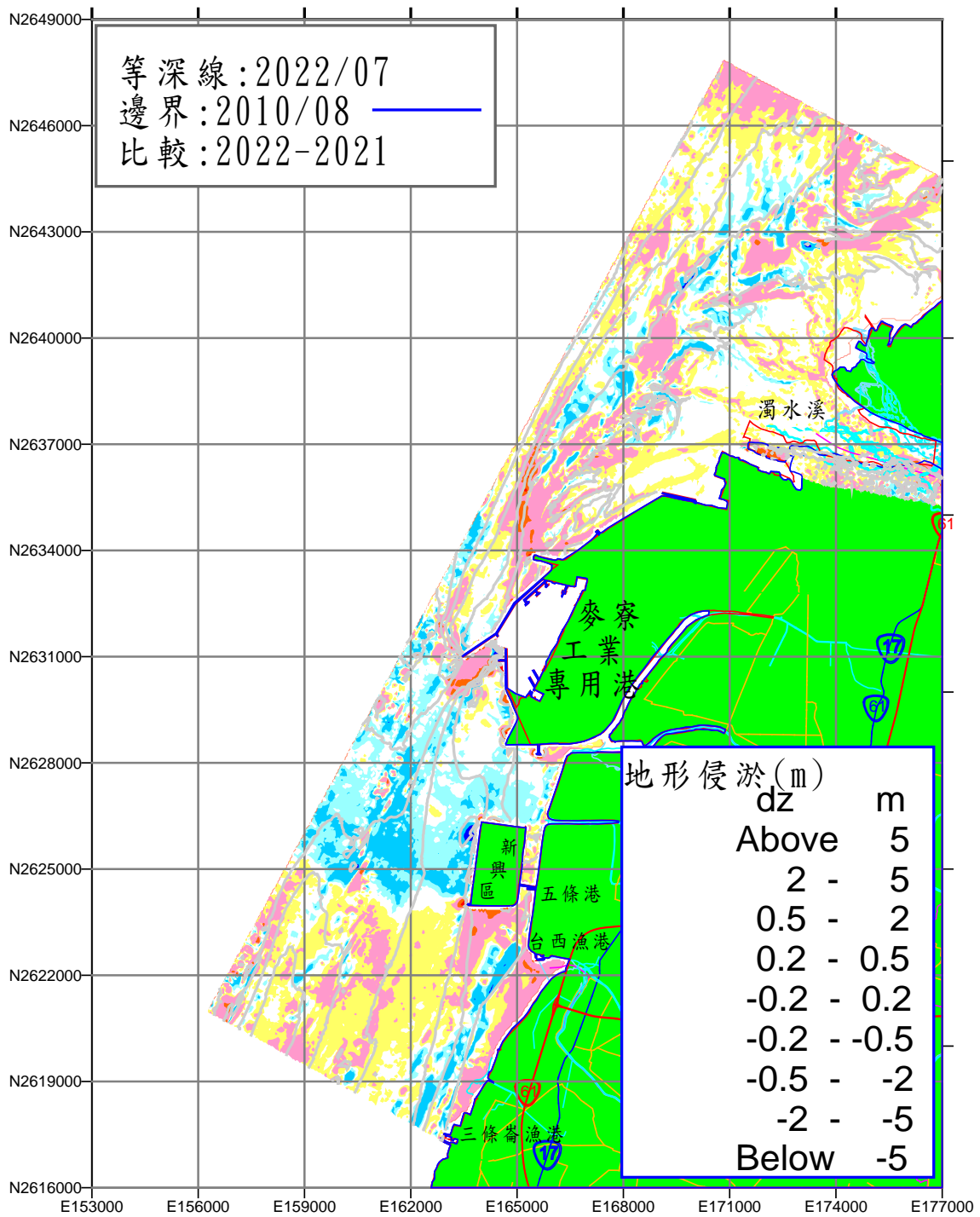
圖 2.12-2 本區地形測量變動量計算圖(2021~2022)
