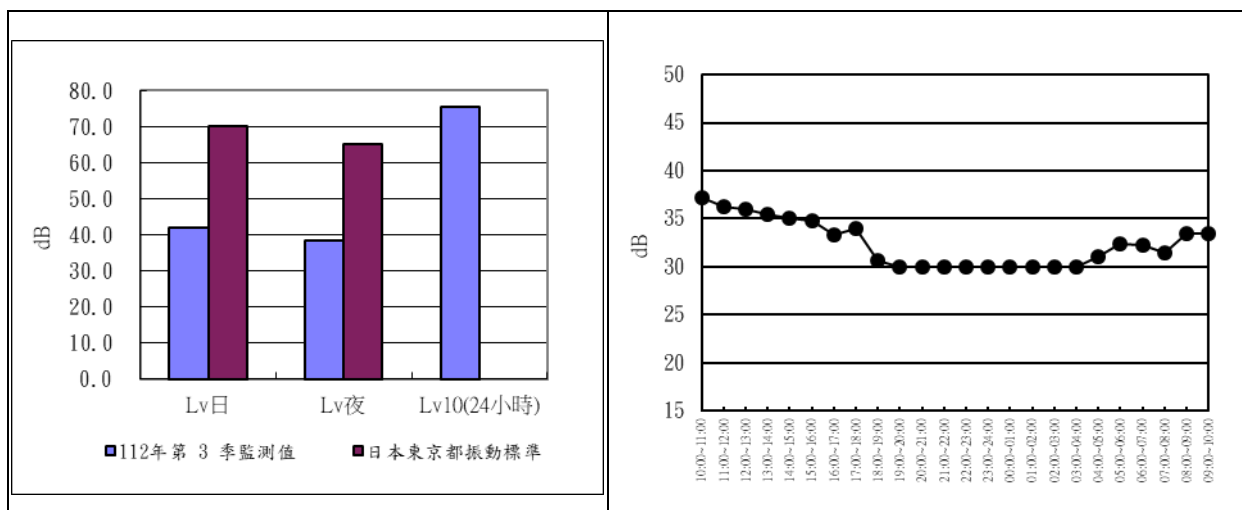
圖 2.3-2 海豐橋 112 年度第 3 季振動監測成果分析圖及逐時變化圖
