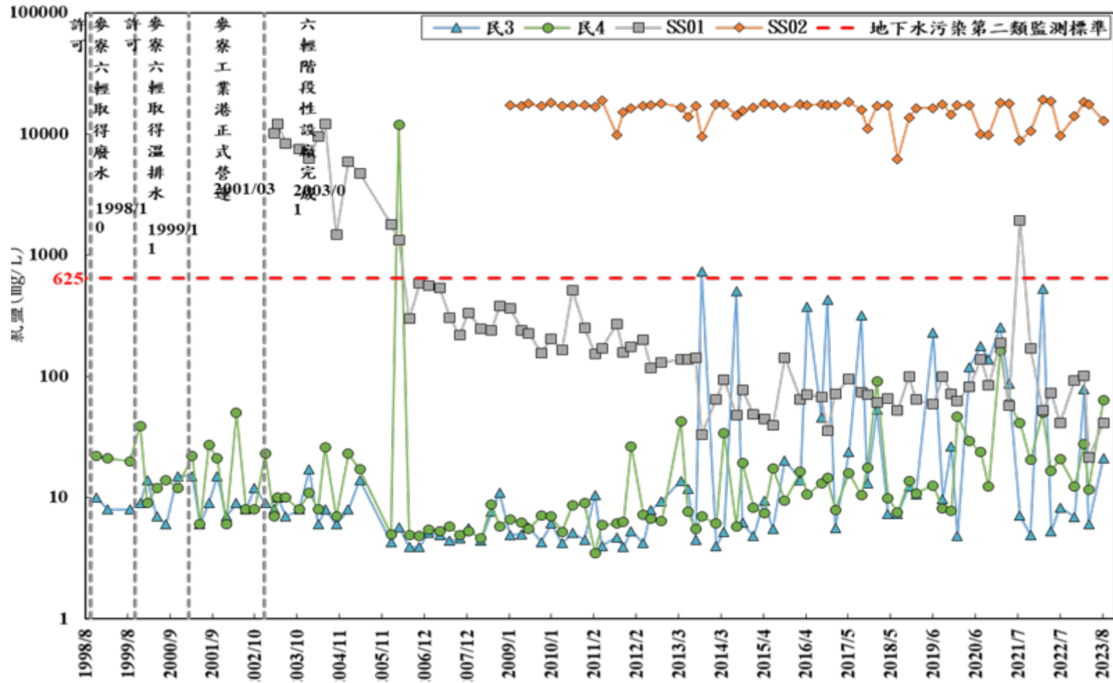
圖 3.1.6-3 氯鹽歷年濃度測值變化
