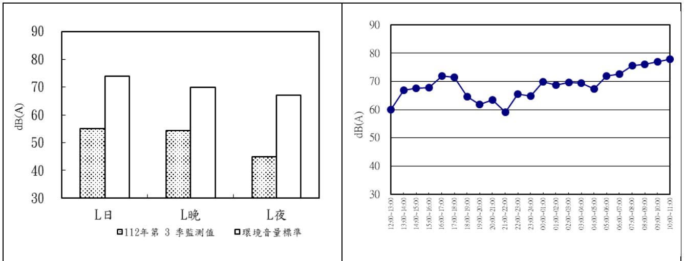
圖 2.2-5 五條港出入管制站 112 年第三季噪音監測成果分析圖及逐時變化圖
