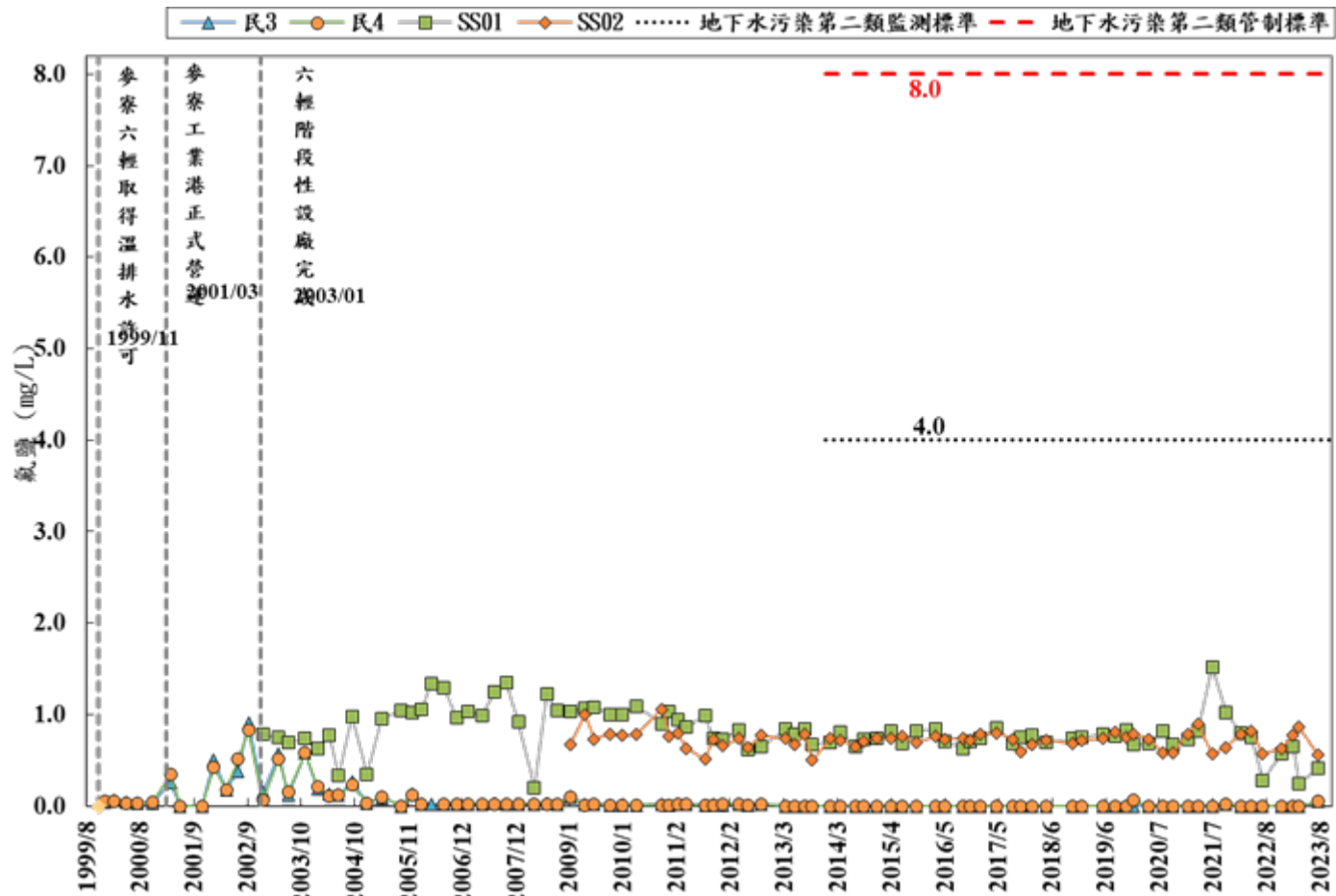
圖 3.1.6-4 氟鹽歷年濃度測值變化
