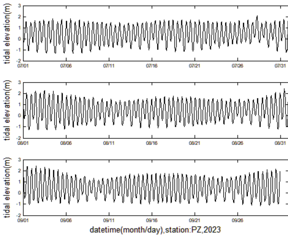
圖 2.13-2 PZ 測站 2023 年 7~9 月各月實測潮位逐時變化圖
