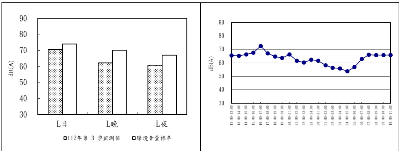
圖 2.2-3 崙豐國小 112 年第 3 季噪音監測成果分析圖及逐時變化圖
