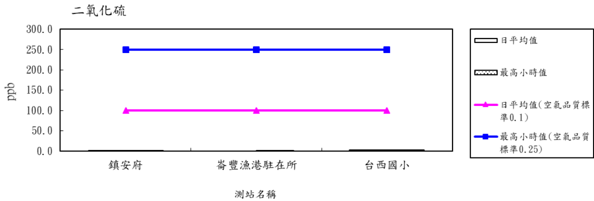
圖 2.1-2 112 年度第 3 季各測站二氧化硫(SO 2 )日平均值及最高小時值比較分析圖
