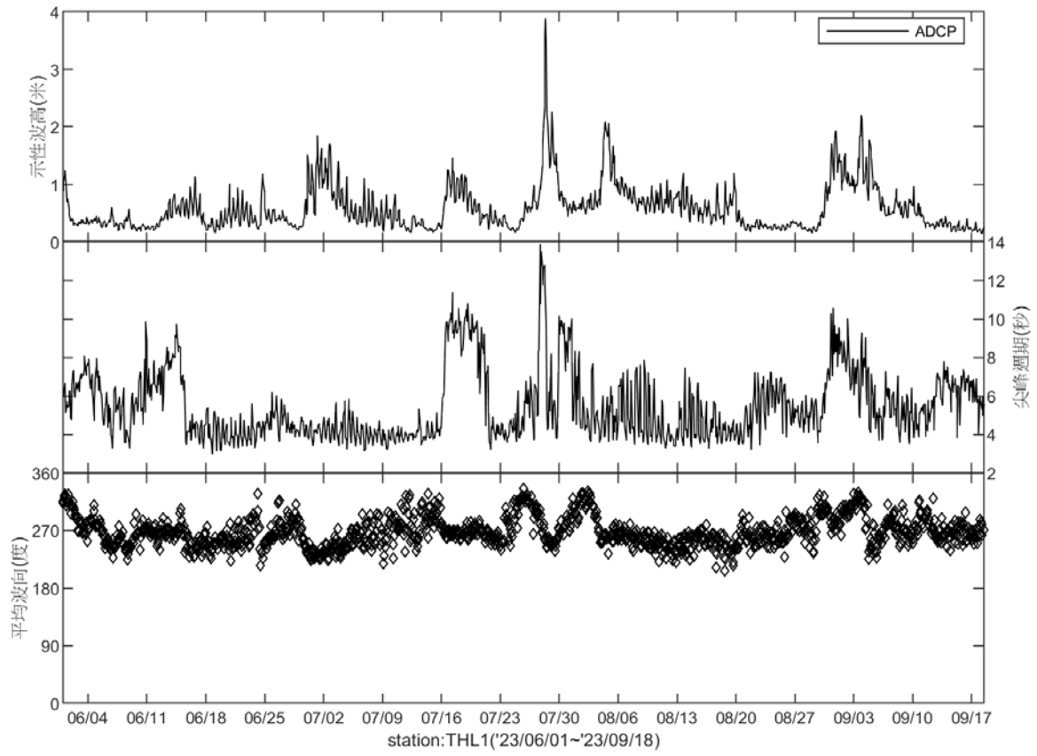
圖 2.13-6 THL1 測站 2023 年 6 月~2023 年 9 月波浪時序列
