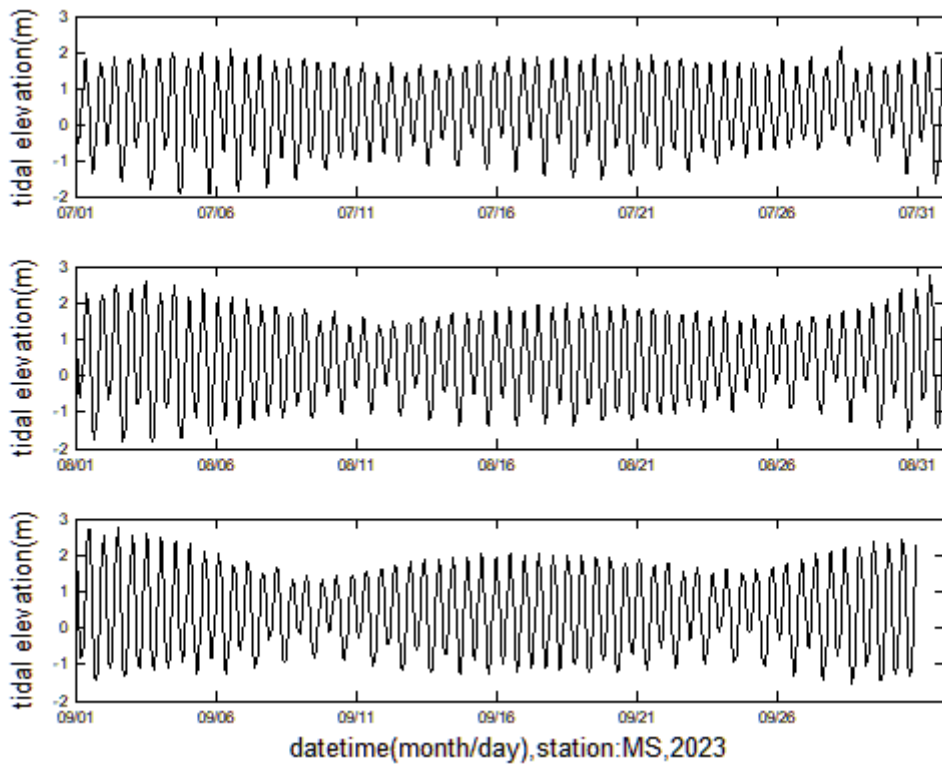
圖 2.13-1 MS 測站 2023 年 7~9 月各月實測潮位逐時變化圖
