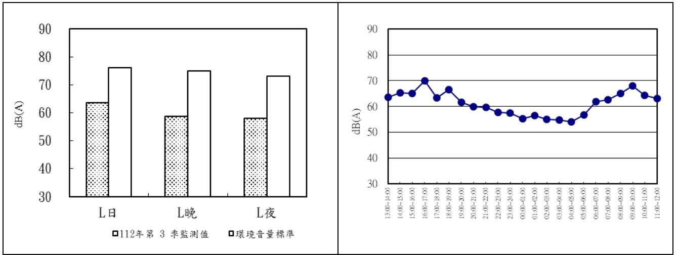
圖 2.2-4 海口橋 112 年第三季噪音監測成果分析圖及逐時變化圖
