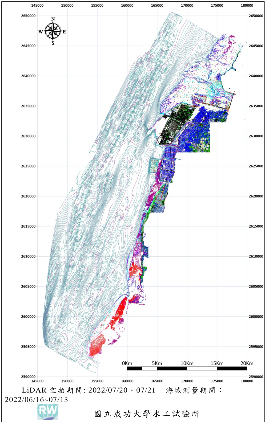
圖 2.12-1 本區海域 2022 年海域地形圖
