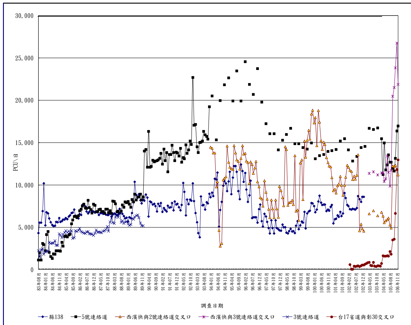
圖 3.1.4-1 彰濱地區歷次交通流量監測結果(續)
