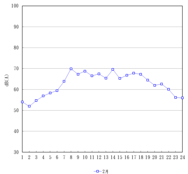
圖 2.2-10 台 17 省道與彰 30 交叉口本季噪音測值逐時變化圖
