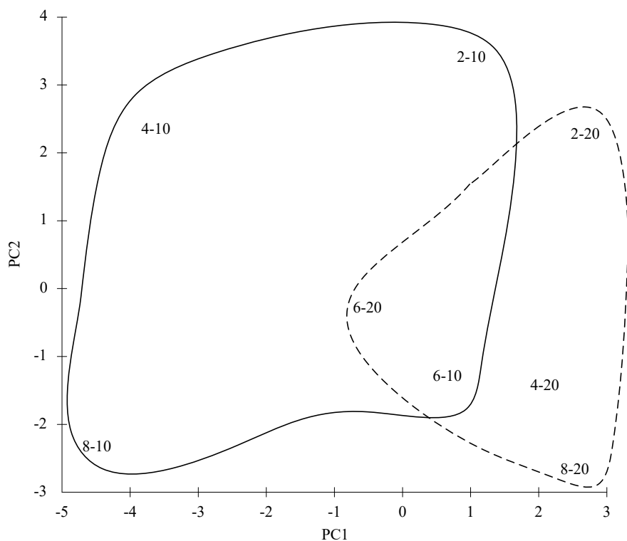
圖 2.10.2-3 民國 107 年 3 月彰濱工業區附近海域各測站浮游動物群聚分析圖圖(圖中第一個數字代表測站，第二個數字代表深度)
