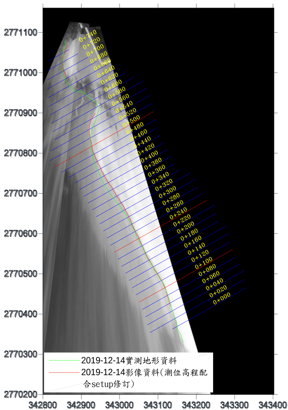
圖 3-22 水位線分析結果圖(2019/12/14)
