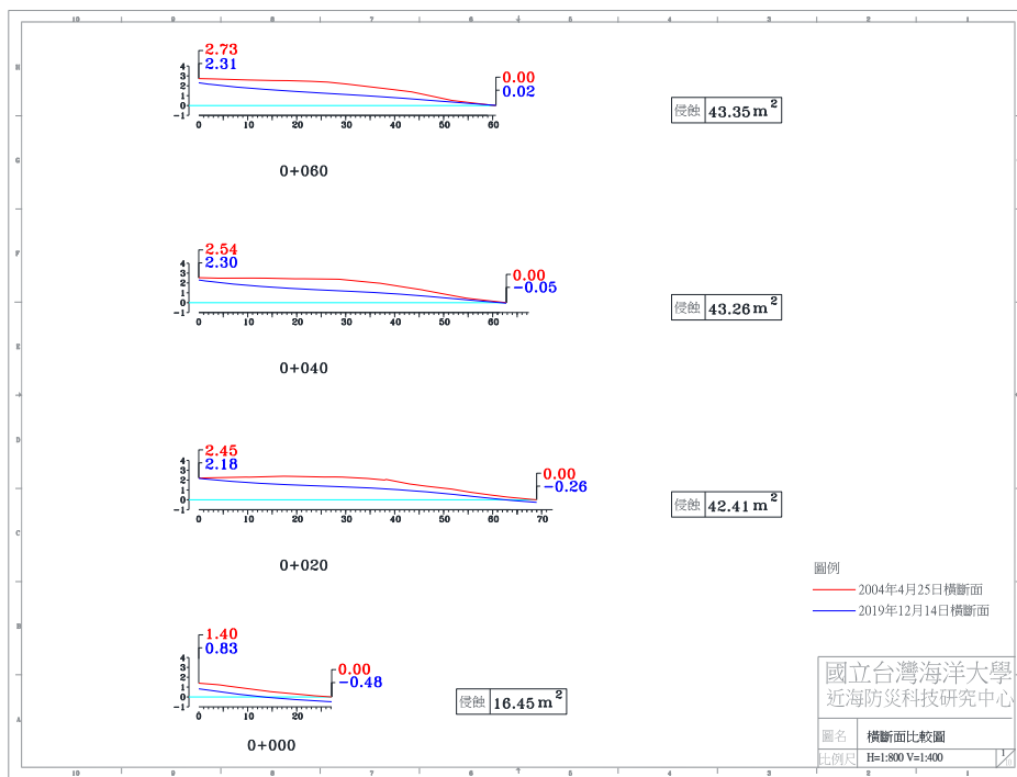
圖 4-4(j) 2019 年 12 月 14 日 A 監測區橫斷面比較圖
