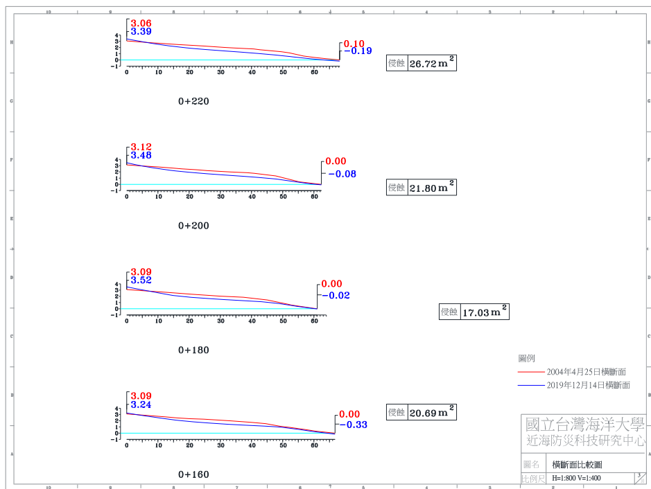
圖 4-4(h) 2019 年 12 月 14 日 A 監測區橫斷面比較圖
