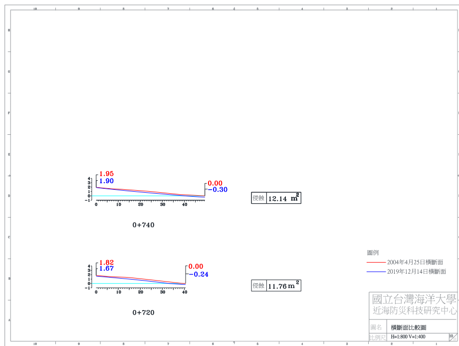
圖 4-4(a) 2019 年 12 月 14 日 A 監測區橫斷面比較圖
