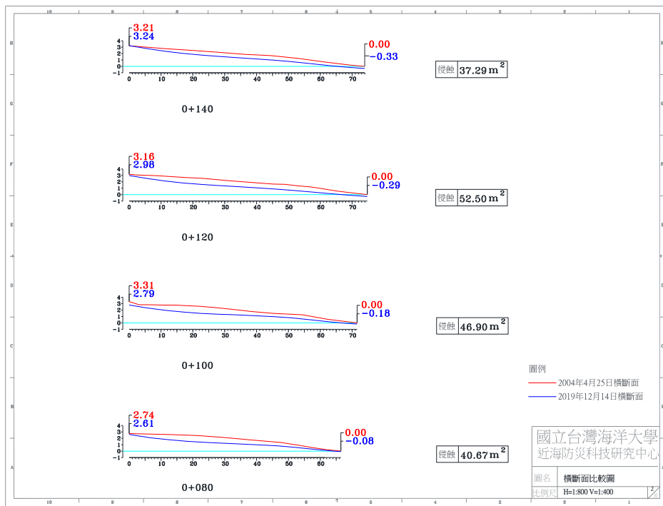
圖 4-4(i) 2019 年 12 月 14 日 A 監測區橫斷面比較圖
