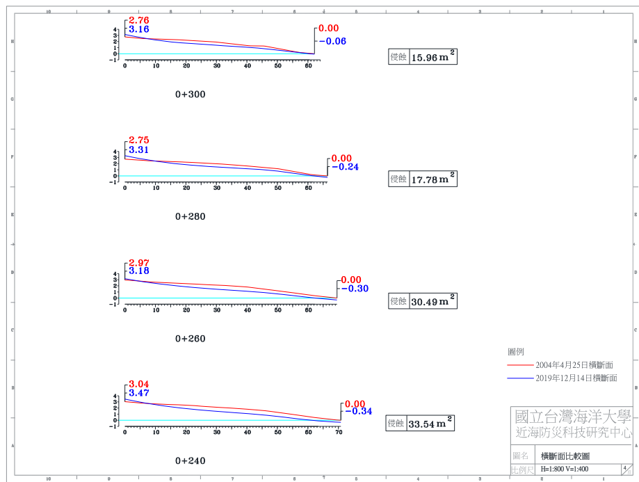
圖 4-4(g) 2019 年 12 月 14 日 A 監測區橫斷面比較圖
