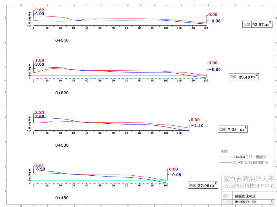
圖 4-4(d) 2019 年 12 月 14 日 A 監測區橫斷面比較圖
