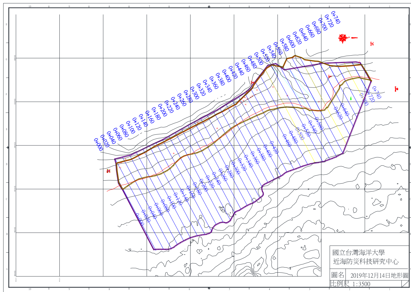
圖 4-1 2019 年 12 月 14 日監測地形圖
