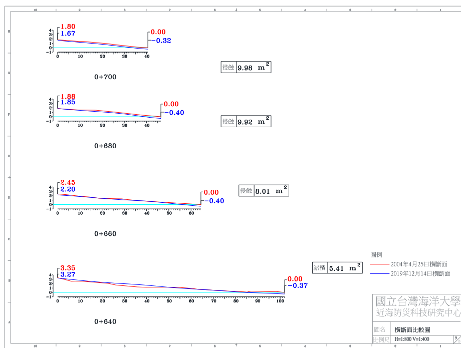
圖 4-4(b) 2019 年 12 月 14 日 A 監測區橫斷面比較圖
