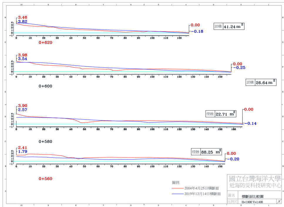
圖 4-4(c) 2019 年 12 月 14 日 A 監測區橫斷面比較圖
