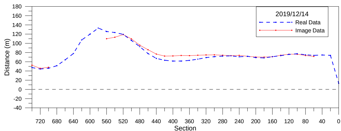
圖 3-23 海岸線分析比較圖(2019/12/14)
