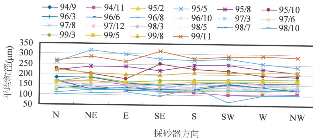
圖3.1-38 各測站各方向各採樣期平均粒徑比較圖
