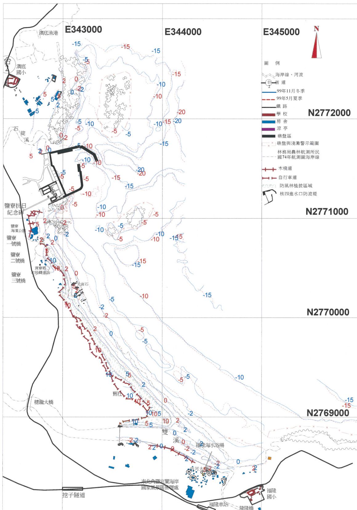
圖 3.1-39 核四施工環境監測海岸地形 99 年 11 月（冬季）與 99 年 5 月（夏季）監測結果比較（半年變化比較）
