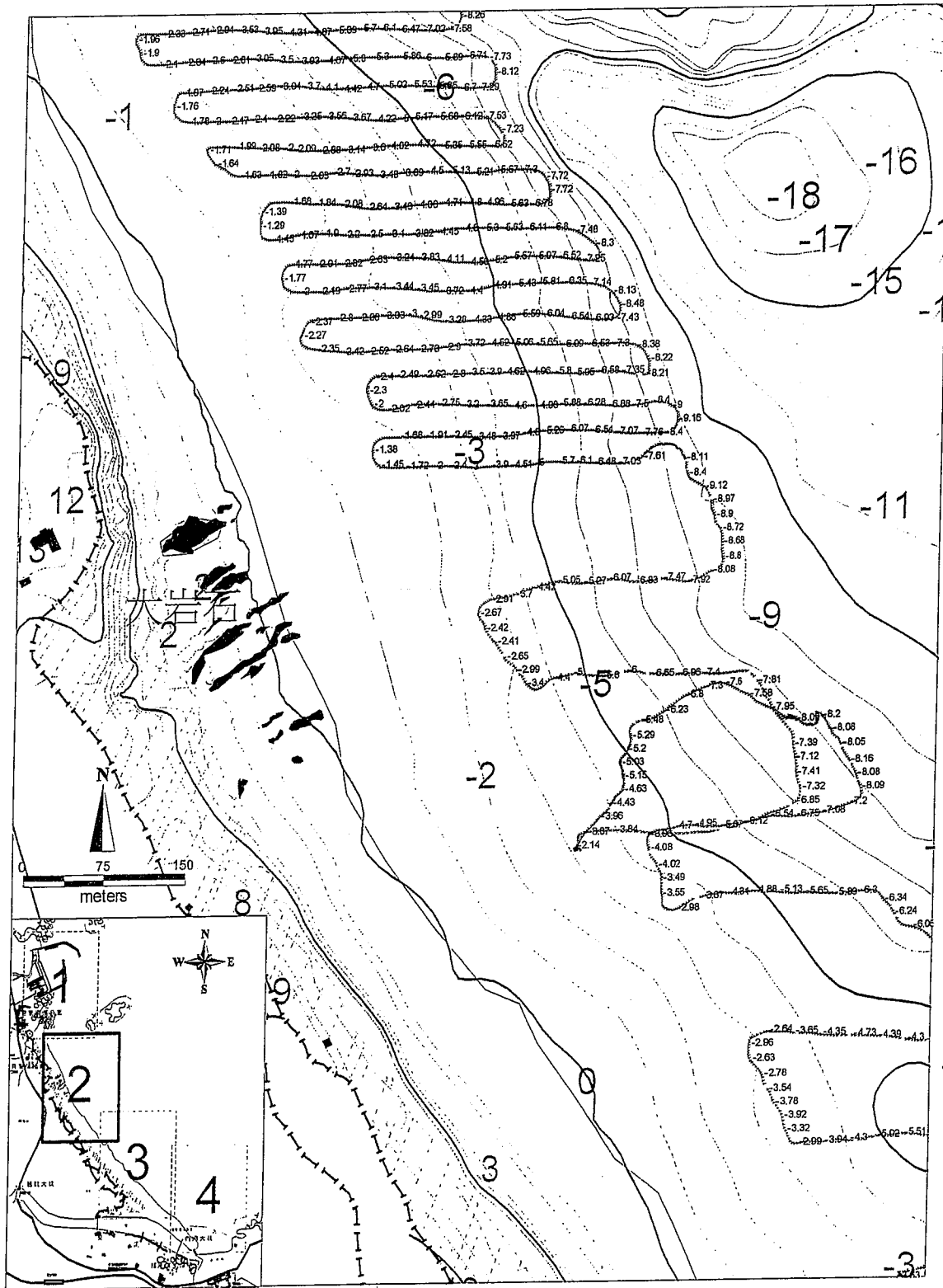
圖 2.16-4 海岸地形 99 年 11 月(冬季)海岸地形監測路徑(續 4)
