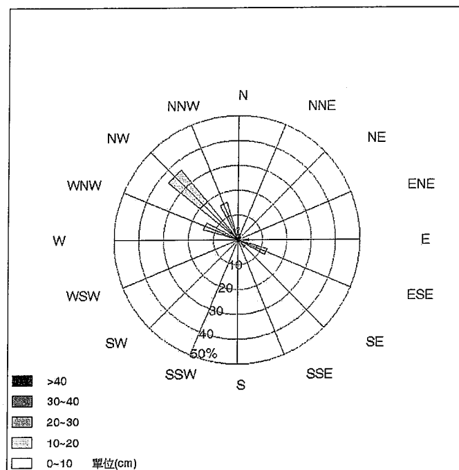
圖2.15-2 本季（99年第4季）海流儀實測流速流向玫瑰圖
