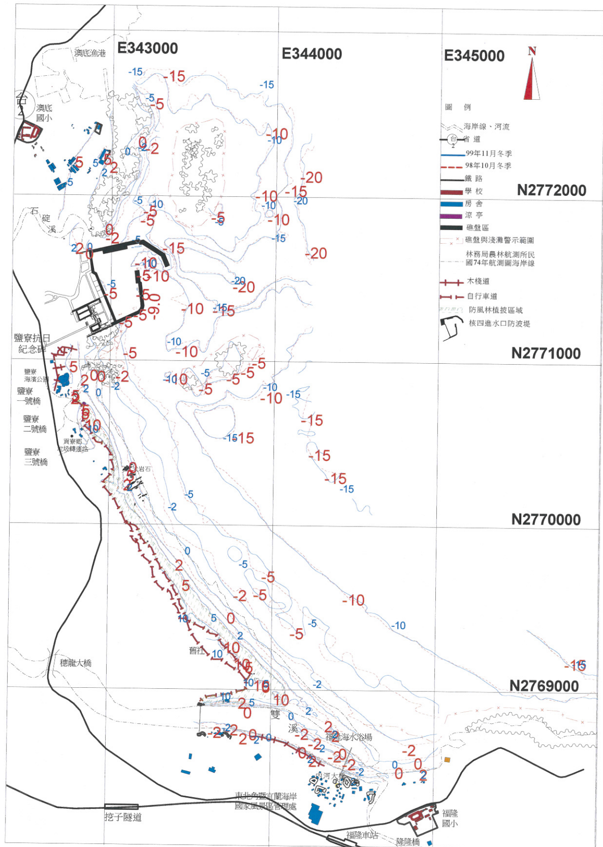
圖 3.1-40 核四施工環境監測海岸地形 99 年 11 月（冬季）與 98 年 10 月（冬季）監測結果比較（同季比較）
