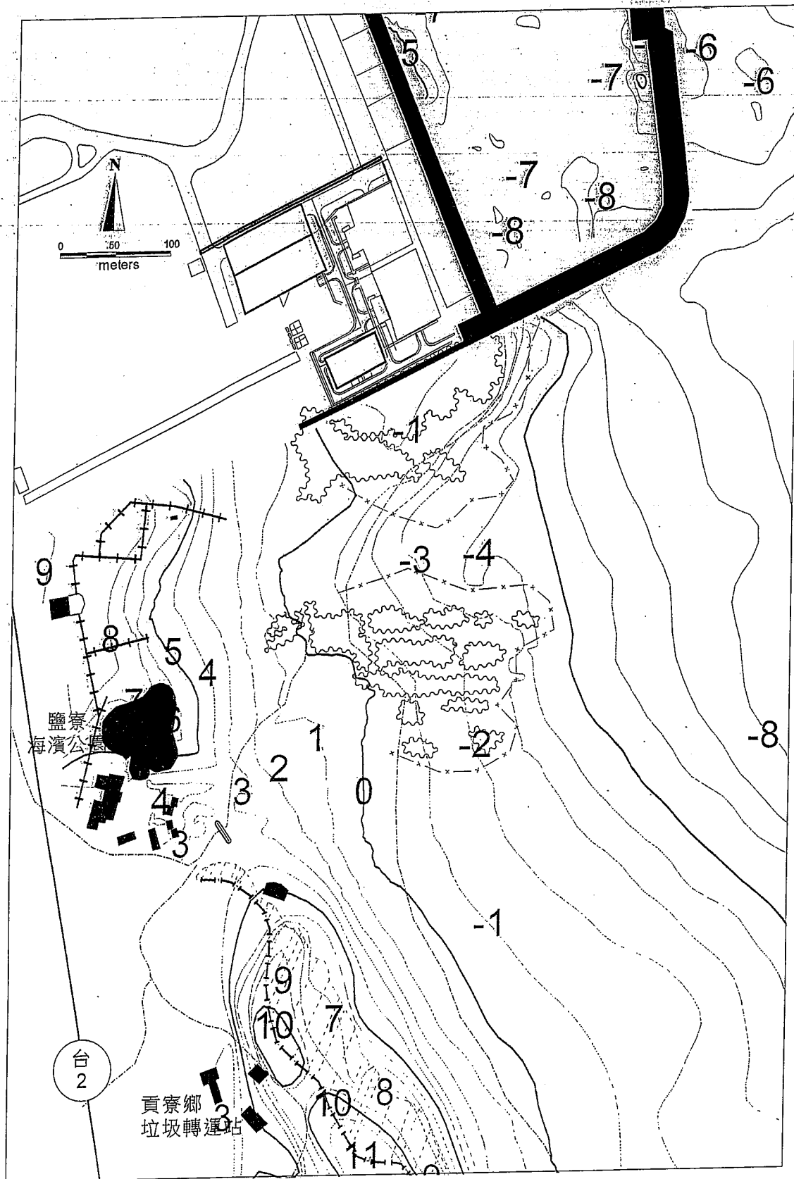
圖 2.16-3 鹽寮公園附近 99 年 11 月（冬季）海岸地形監測結果
