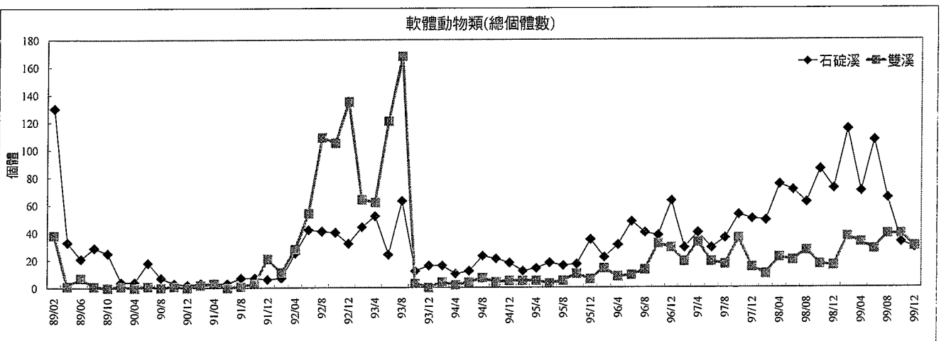
圖3.1-26 核四施工期間環境監測河域生態長期趨勢分析 (續)
