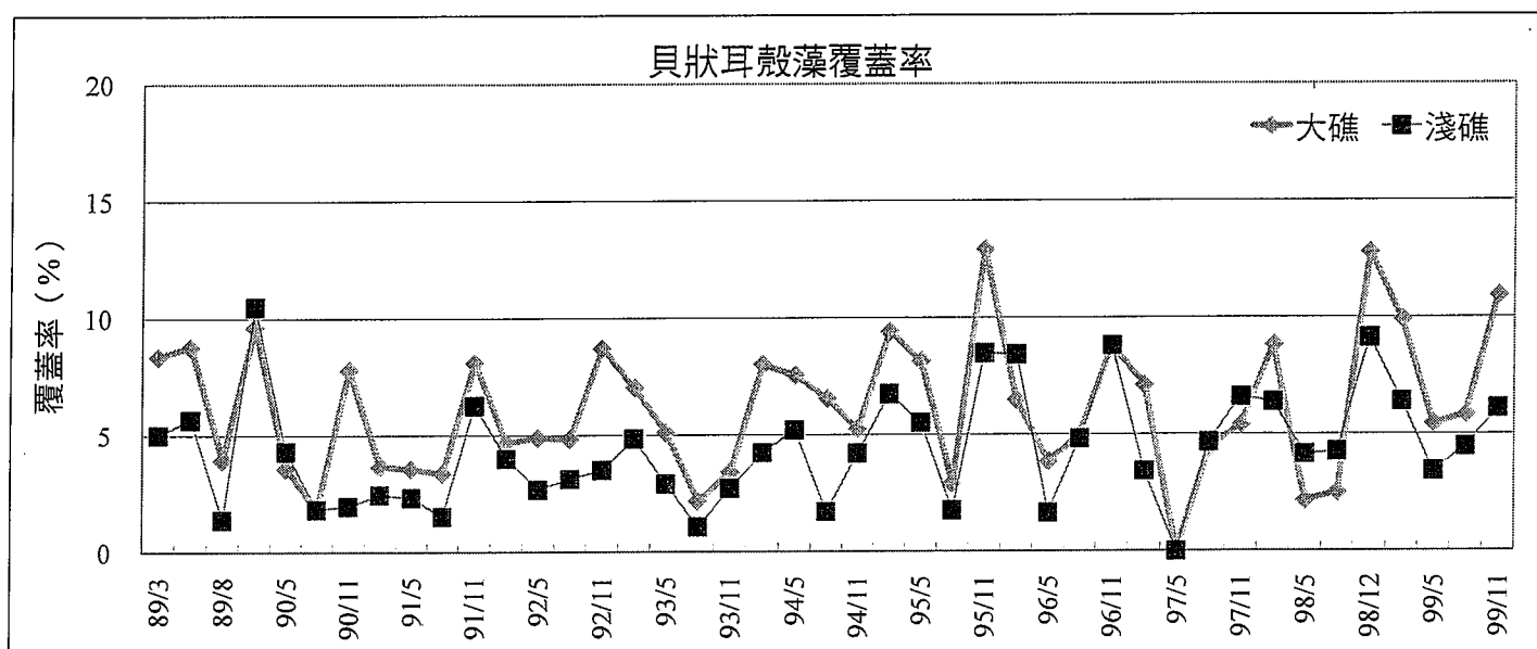
圖3.1-33 核四施工期間環境監測調查海域大型藻類指標物種長期變動趨勢
