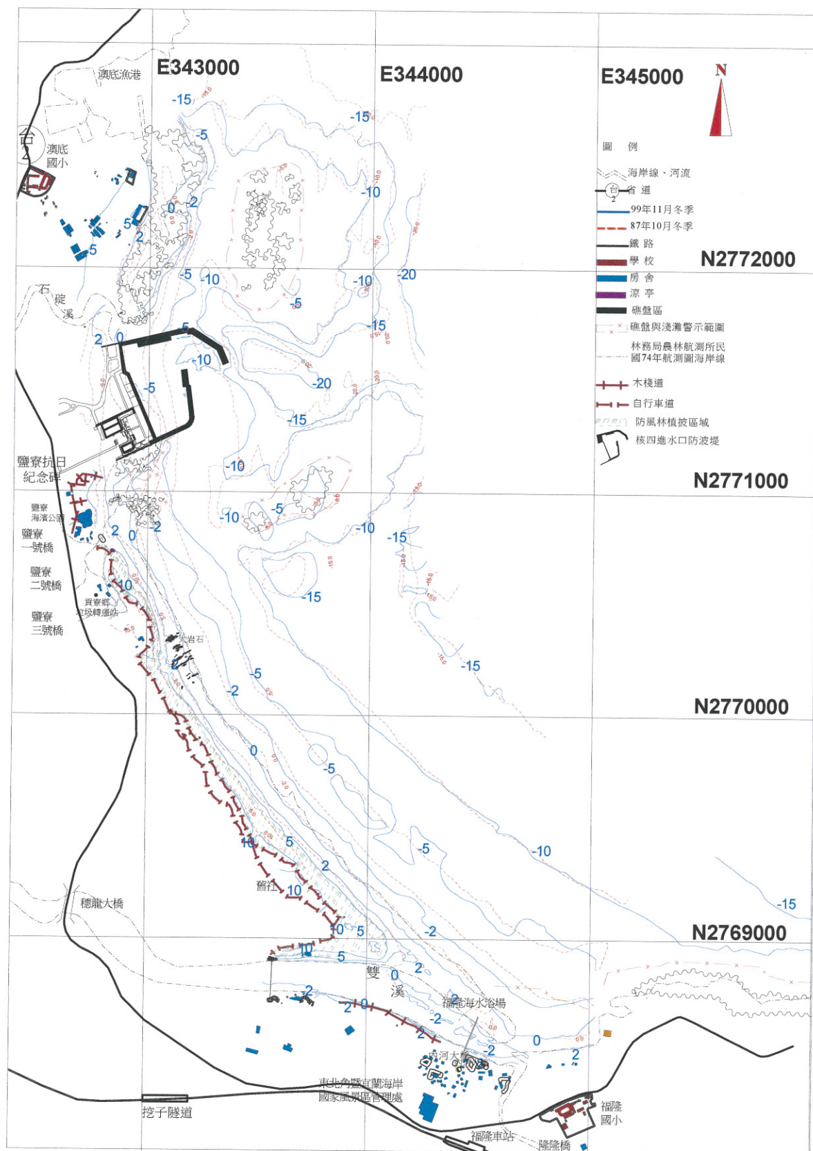
圖 3.1-41 核四施工環境監測海岸地形 99 年 11 月（冬季）與 87 年 10 月（冬季）監測結果比較（海事工程施工前後比較）
