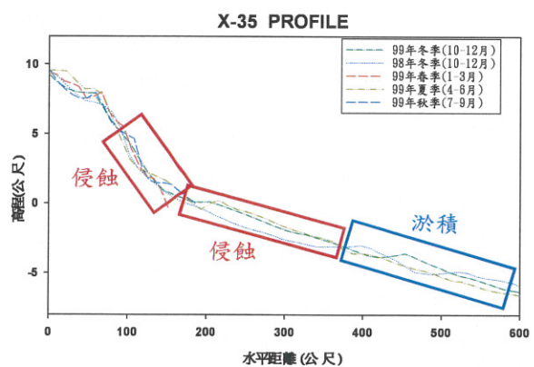
圖3.1-50 核四附近海岸地形監測各剖面水深變化比較 (續1)
