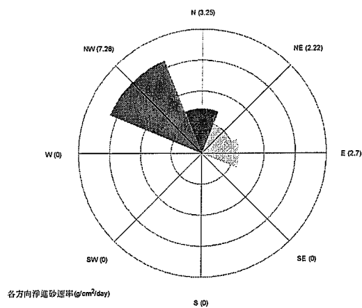
S4測站各方向淨進砂速率雷達圖
