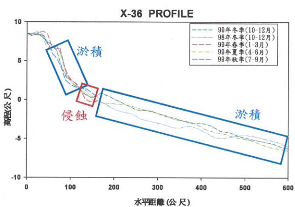
圖3.1-50 核四附近海岸地形監測各剖面水深變化比較 (續1)
