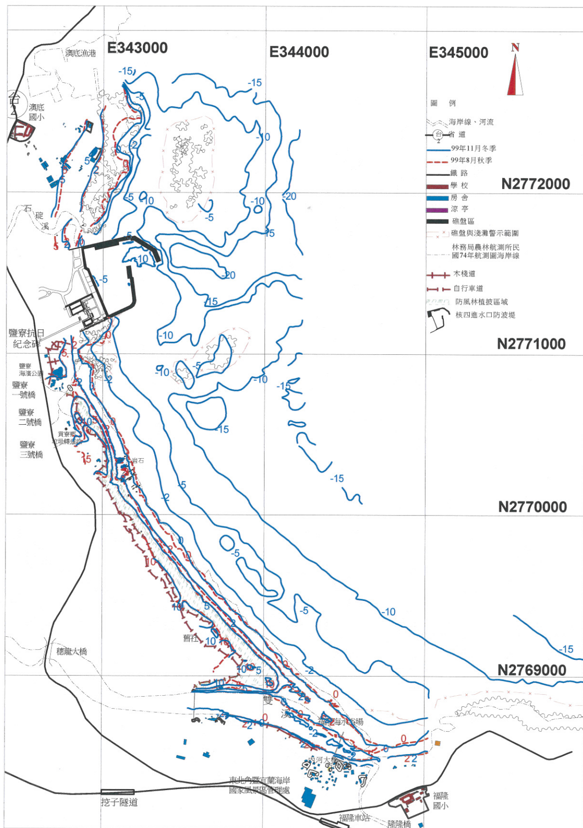
圖 2.16-5 核四施工環境監測海岸地形 99 年 11 月（冬季）與 99 年 8 月（秋季）監測結果比較
