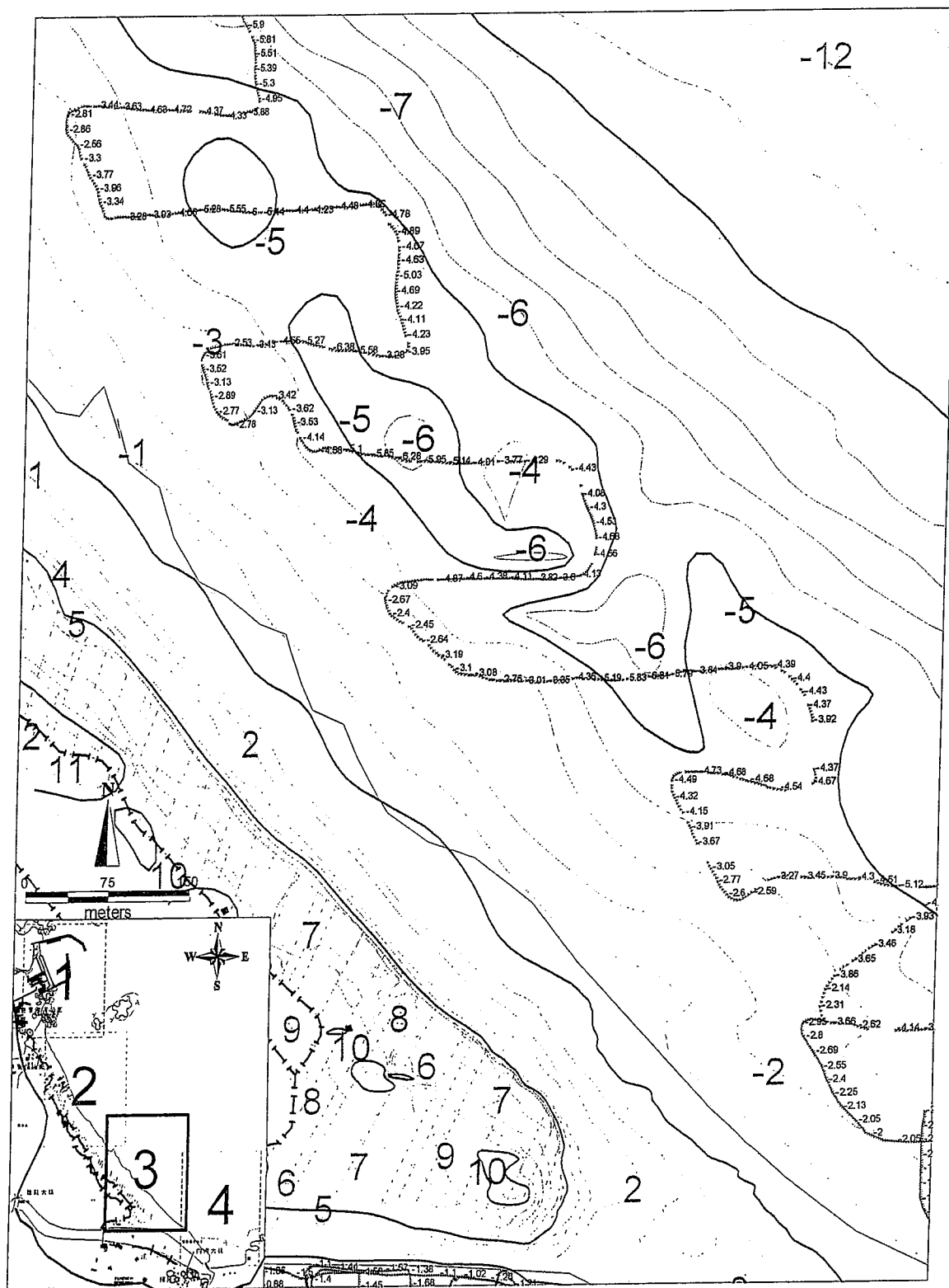
圖 2.16-4 海岸地形 99 年 11 月(冬季)海岸地形監測路徑(續 5)
