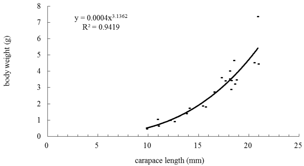
圖III.6-13 本季螞蛄雌蝦頭胸甲長(cl)與體重(bw濕重)之關係
