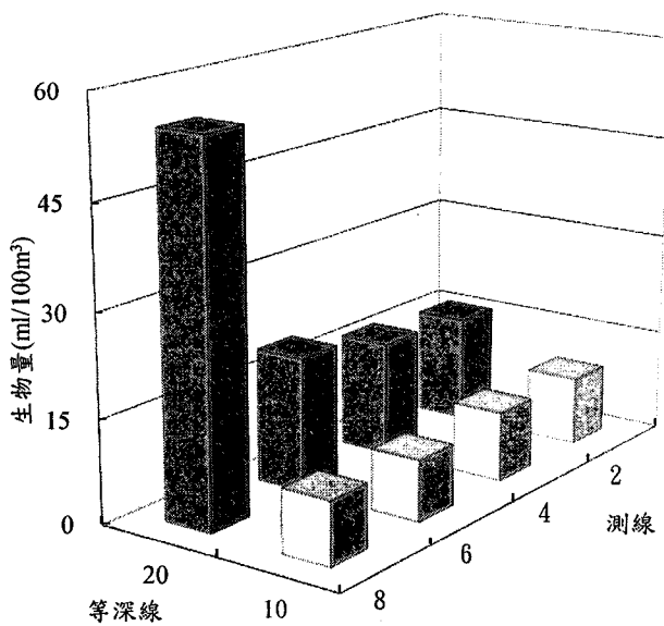
圖 2.10.2-1 民國 108 年 7 月彰化濱海工業區附近海域浮游動物之豐度及生物量分布圖
