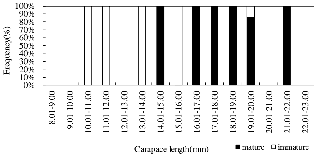
圖III.6-19 本季成熟雌蝦與未成熟雌蝦之比例
