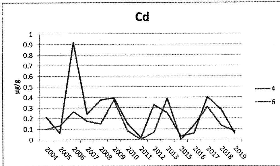
附錄 III.10-2 圖 19. 2004~2019 年 7 月測站 4 及 6 漁舟蜆螺體內鎘含量之測站比較圖
