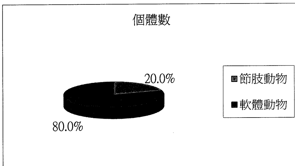
附錄III.10-1圖6 民國108年7月潮間帶各大類生物之個體數百分比
