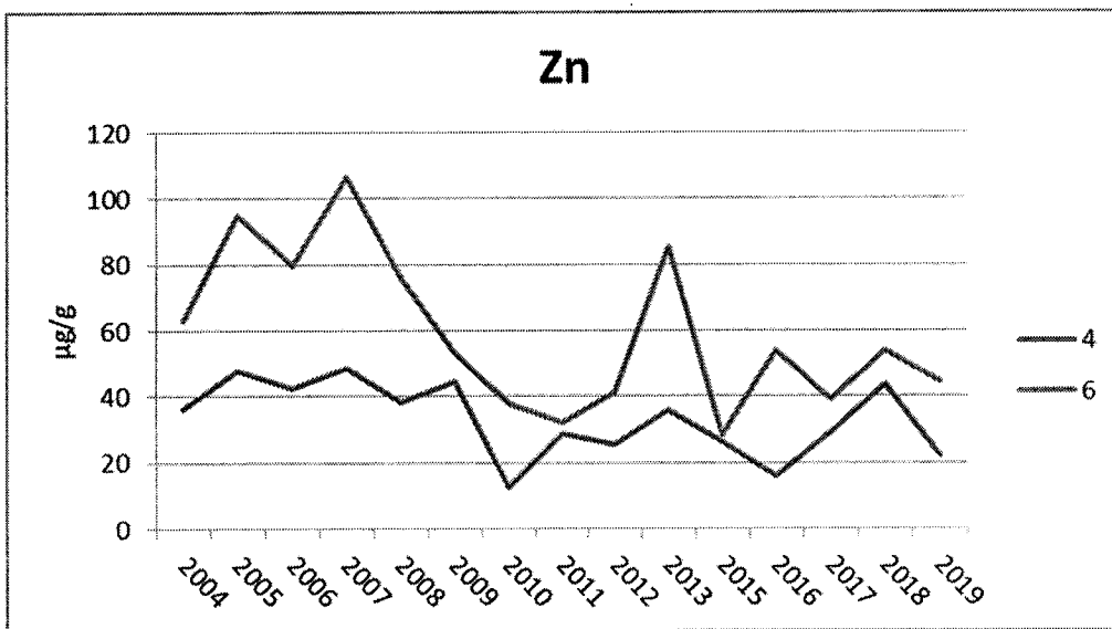
附錄 III.10-2 圖 20. 2004~2019 年 7 月測站 4 及 6 漁舟蜆螺體內鋅含量之測站比較圖
