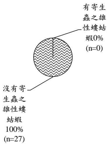
圖III.6-26 本季雄性螻蛄蝦被等足目寄生的百分率 (n=27)。
