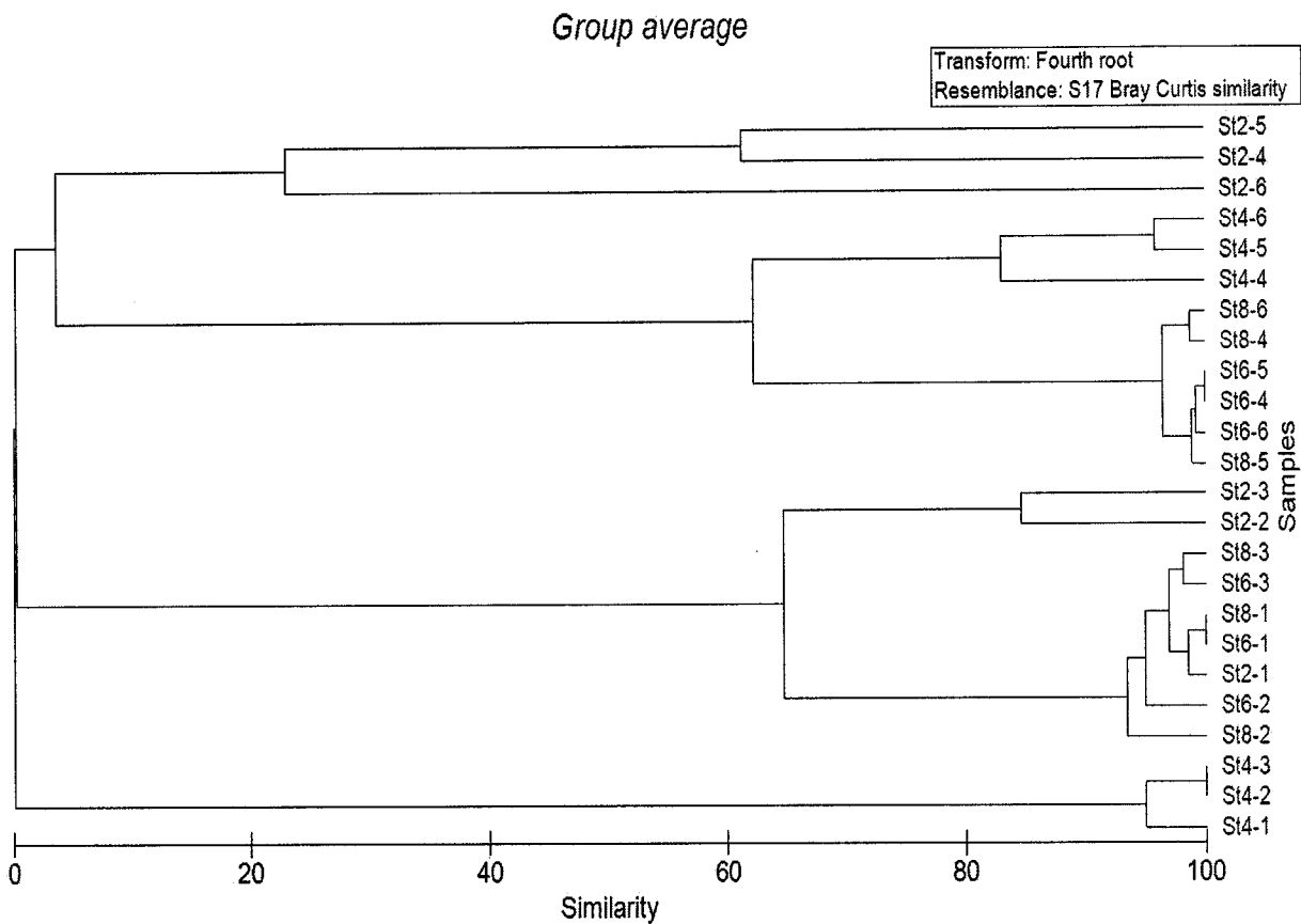
附錄III.10-2圖3 民國108年7月於彰濱工業區附近海域潮間帶各測站之群聚分析樹狀圖。
