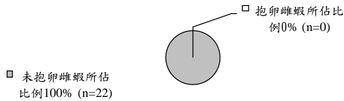
圖III.6-20 本季伸港地區螻蛄蝦抱卵母蝦佔雌蝦之百分比(n=22)。
