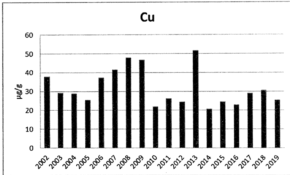
附錄 III.10-2 圖 5. 2002 至 2019 年 7 月短指和尚蟹體內銅含量之年度比較圖
