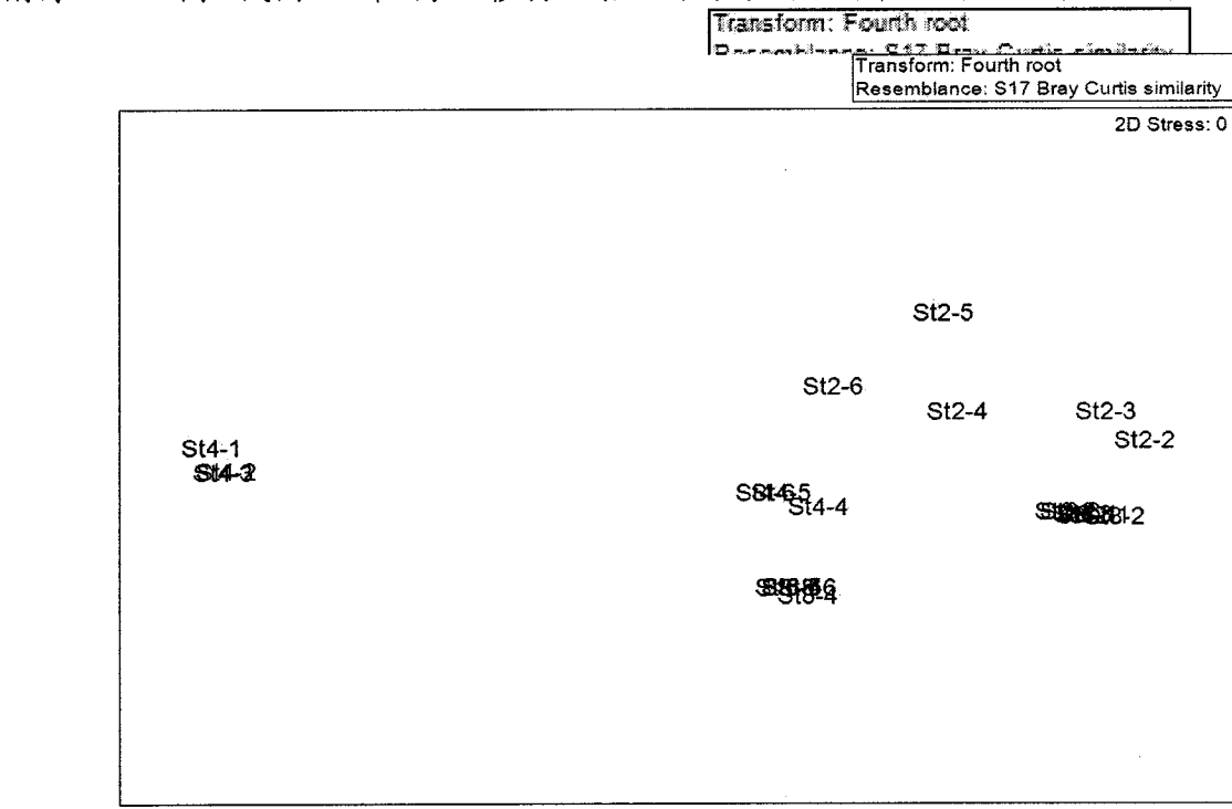
附錄III.10-2圖4 民國108年7月於彰濱工業區附近海域潮間帶各測站之群聚MDS圖。
