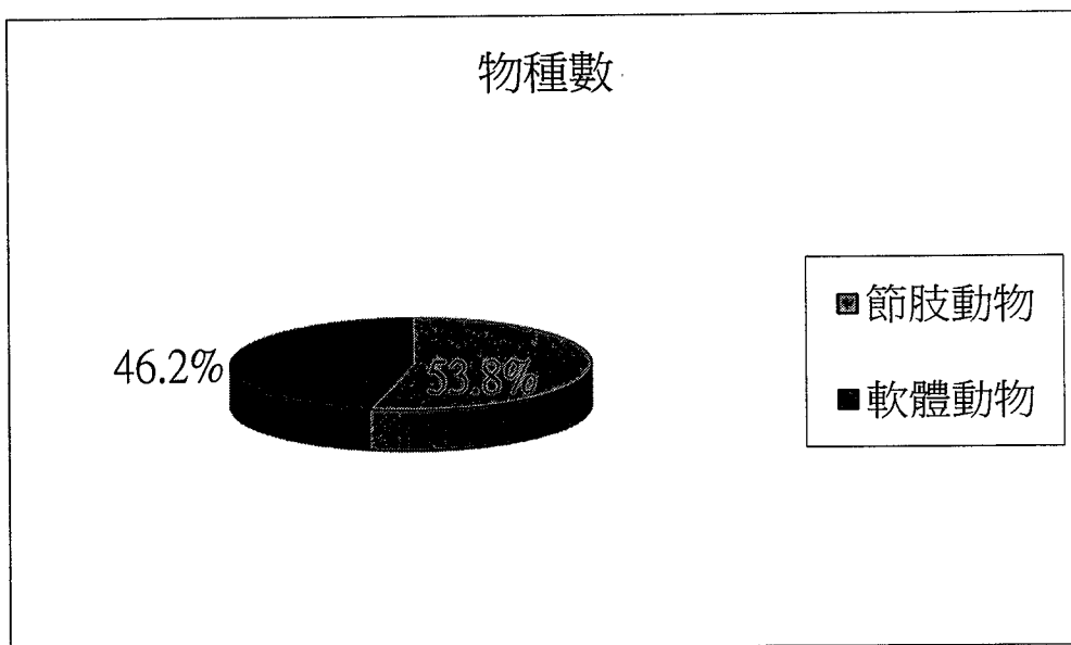
附錄III.10-1圖5 民國108年7月潮間帶各大類生物之物種數百分比
