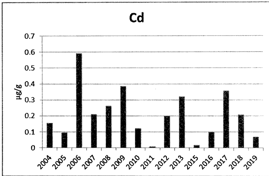
附錄 III.10-2 圖 11. 2004 至 2019 年 7 月漁舟蜆螺體內鎘含量之年度比較圖
