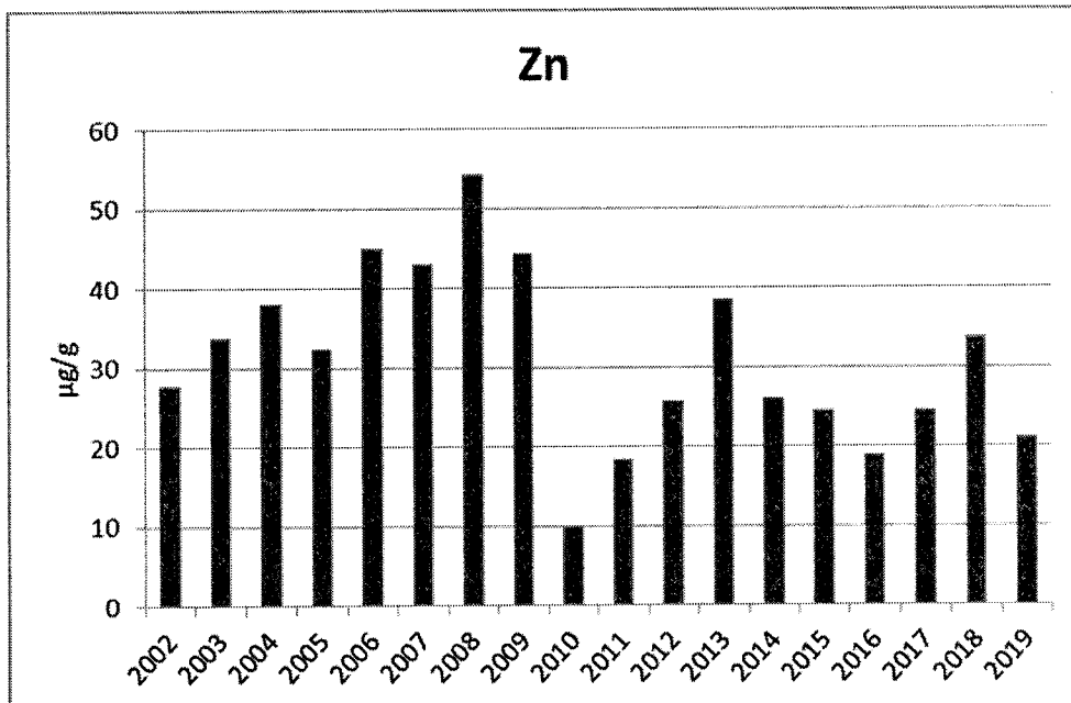
附錄 III.10-2 圖 8. 2002 至 2019 年 7 月短指和尚蟹體內鋅含量之年度比較圖
