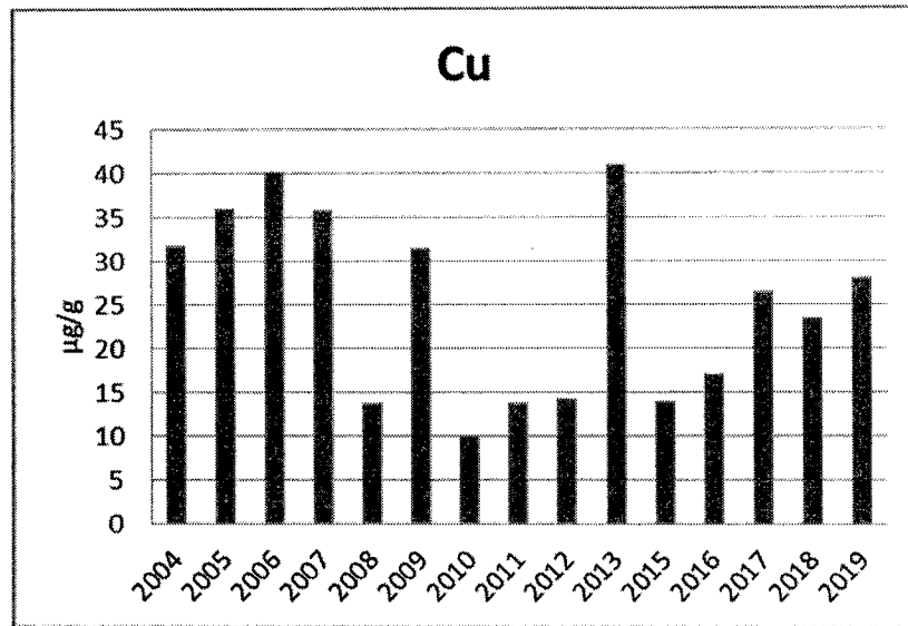
附錄 III.10-2 圖 9. 2004 至 2019 年 7 月漁舟蜆螺體內銅含量之年度比較圖
