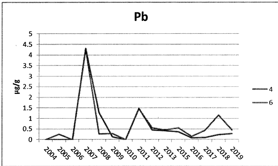
附錄 III.10-2 圖 18. 2004~2019 年 7 月測站 4 及 6 漁舟蜆螺體內鉛含量之測站比較圖
