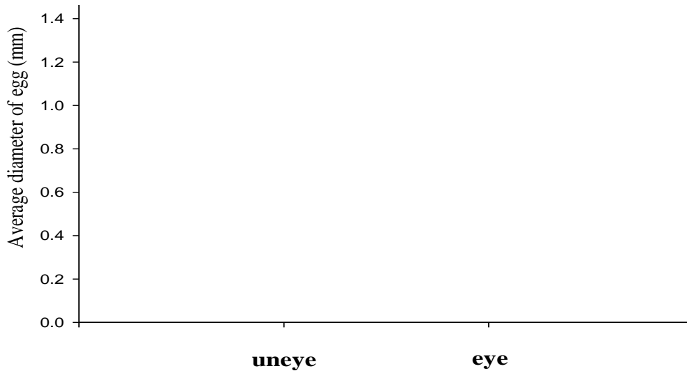
圖 III. 6-21 本季伸港地區螻蛄蝦發眼卵與未發眼卵之平均卵徑(本季未發現發眼母蝦)。
