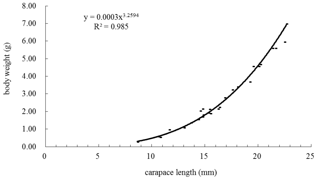
圖III.6-12 本季螞蛄雄蝦頭胸甲長(cl)與體重(bw濕重)之關係
