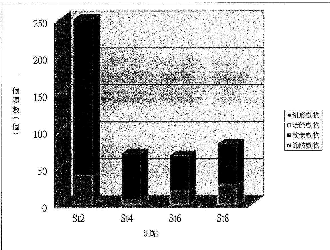
附錄III.10-1圖8 民國108年7月於彰濱工業區附近海域潮間帶各測站各大類生物之個體數比較圖
