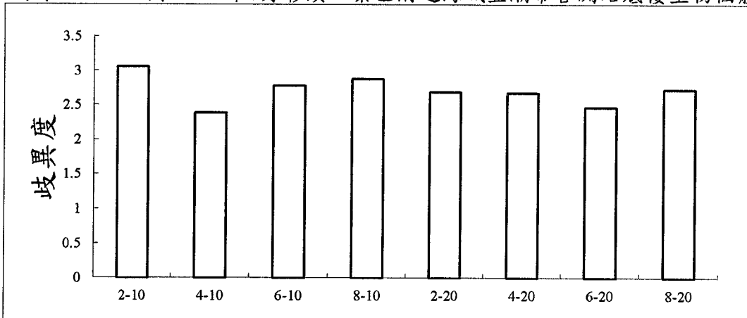
附錄III.10-1圖3 108年7月彰濱工業區附近海域亞潮帶各測站底棲生物歧異度之比較
