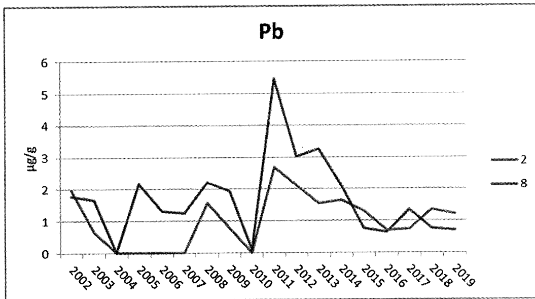
附錄 III.10-2 圖 14. 2002~2019 年 7 月測站 2 及 8 短指和尚蟹體內鉛含量之測站比較圖
