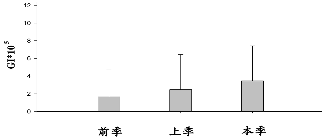
圖 III.6-18 本季與前兩季螻蛄蝦卵巢指數之比較
