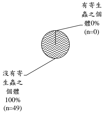
圖III.6-24 本季螻蛄蝦被等足目寄生的百分率(n=49)。
