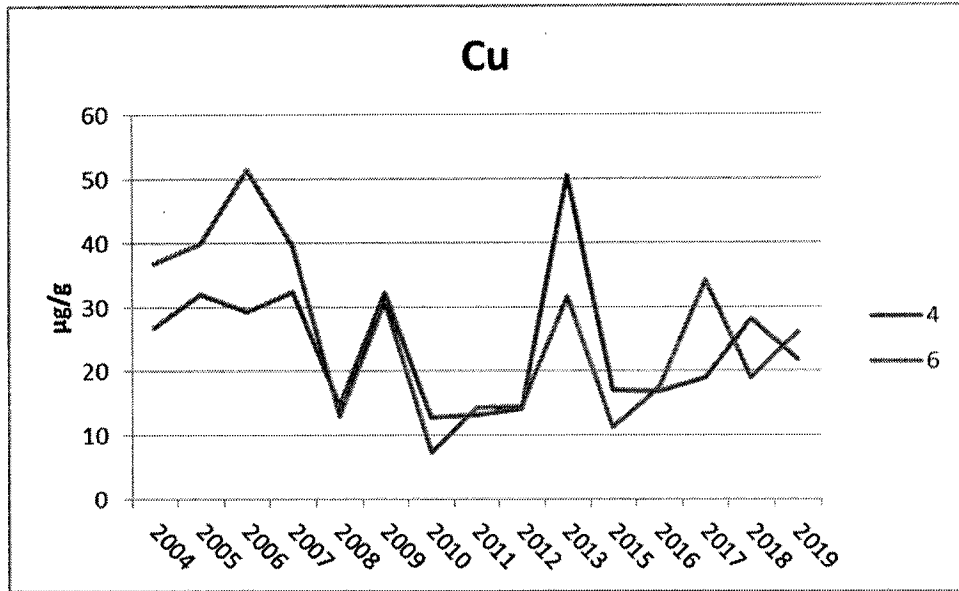
附錄 III.10-2 圖 17. 2004~2019 年 7 月測站 4 及 6 漁舟蜆螺體內銅含量之測站比較圖
