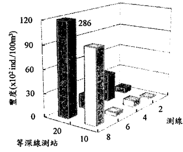
圖 2.10.2-2 民國 108 年 7 月彰化濱海工業區附近海域浮游動物主要優勢類群之豐度分布圖
