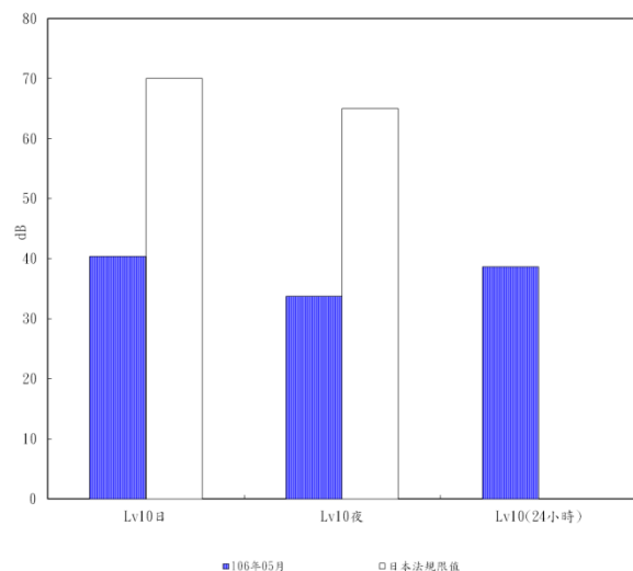
圖 2.3-5 海埔國小日本季振動調查結果分析圖
