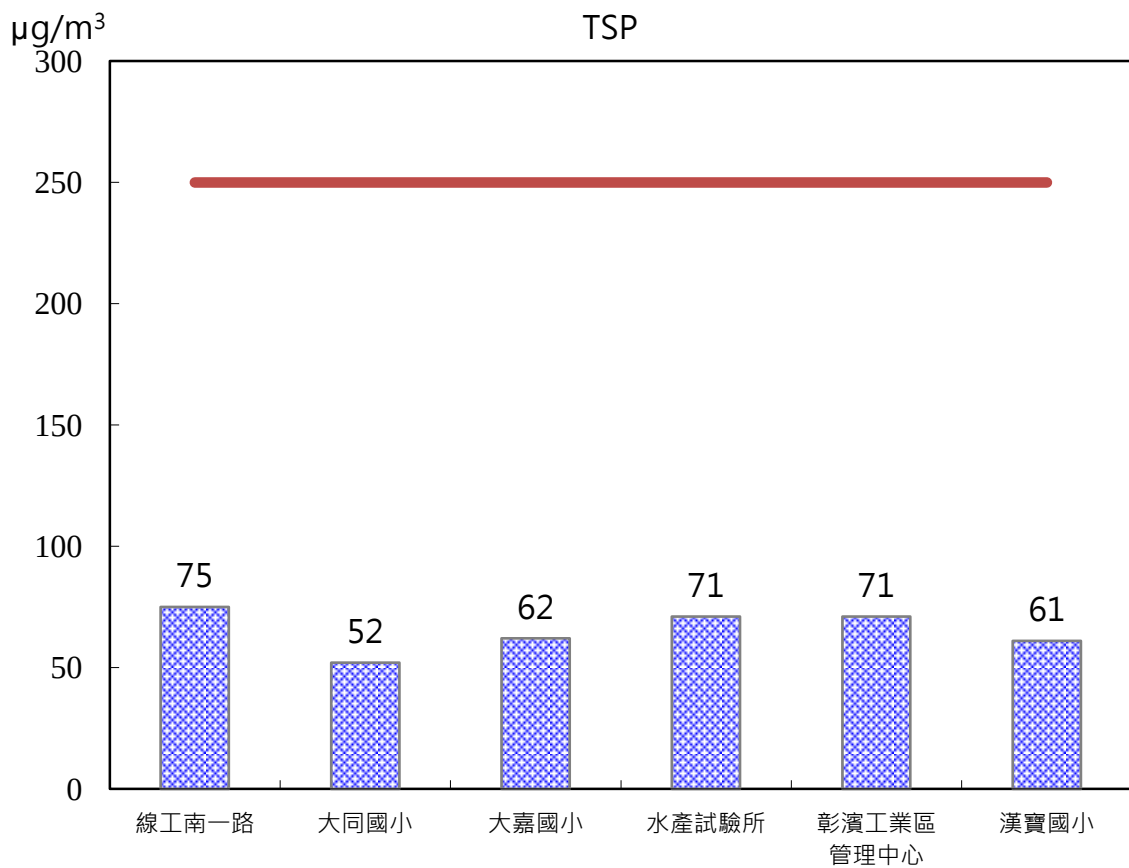
圖 2.1-8 本季各測站 TSP24 小時值監測結果比較分析圖
