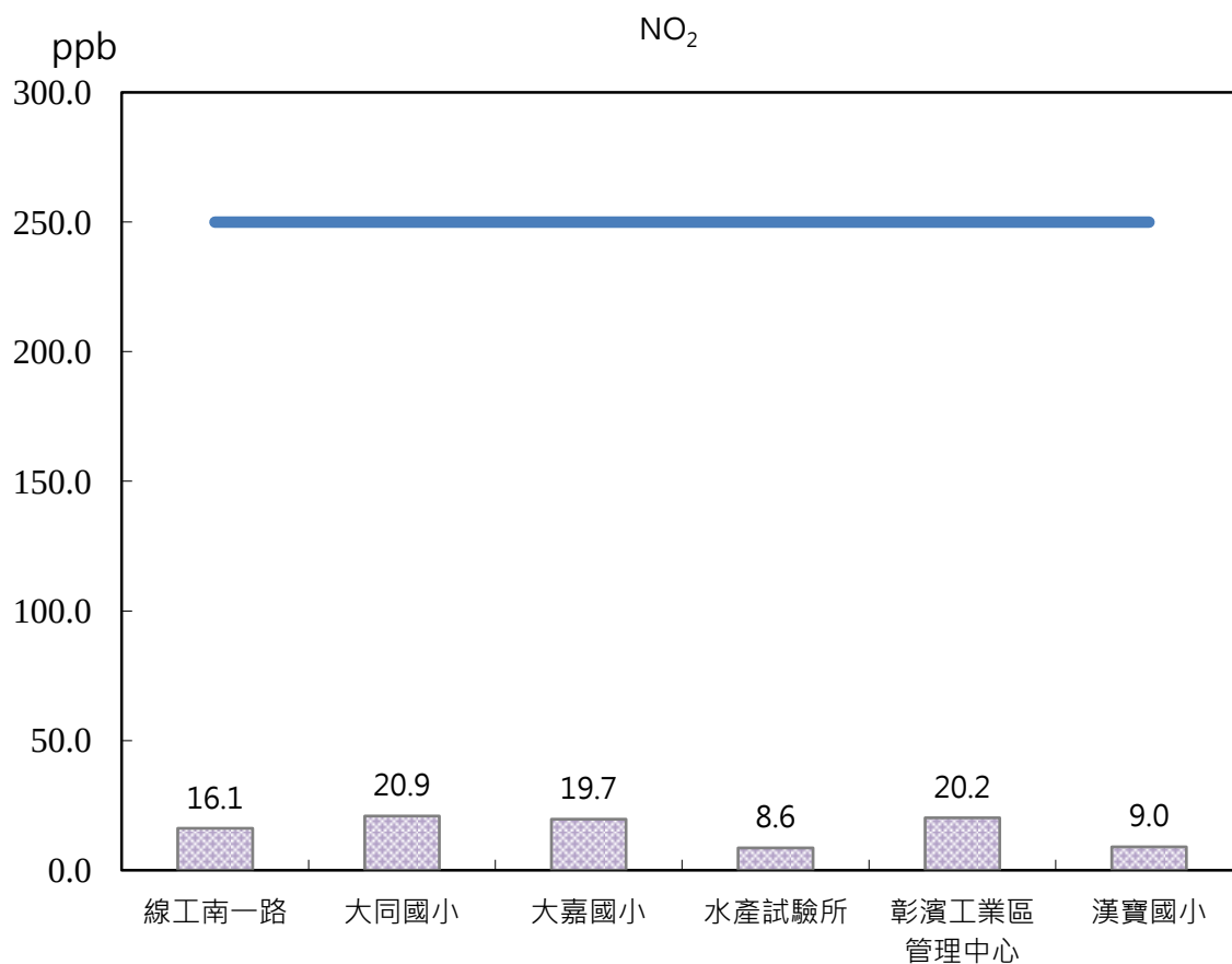
圖 2.1-5 本季各測站 NO 2 最高小時值監測結果比較分析圖
