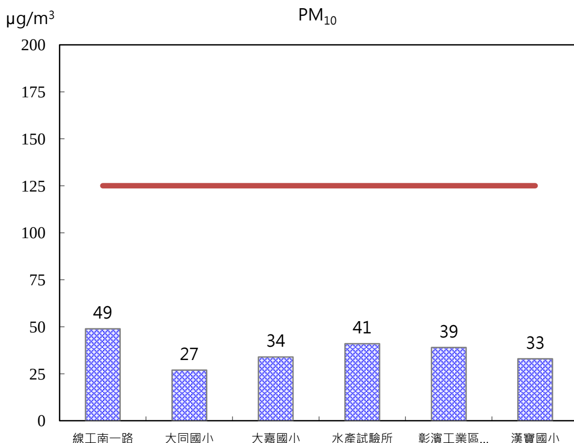
圖 2.1-9 本季各測站 PM 10 日平均值監測結果比較分析圖
