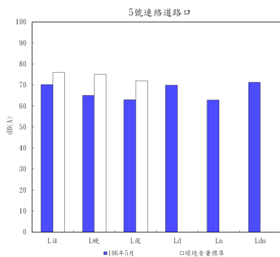
圖 2.2-7 5 號連絡道路口本季噪音調查結果分析圖
