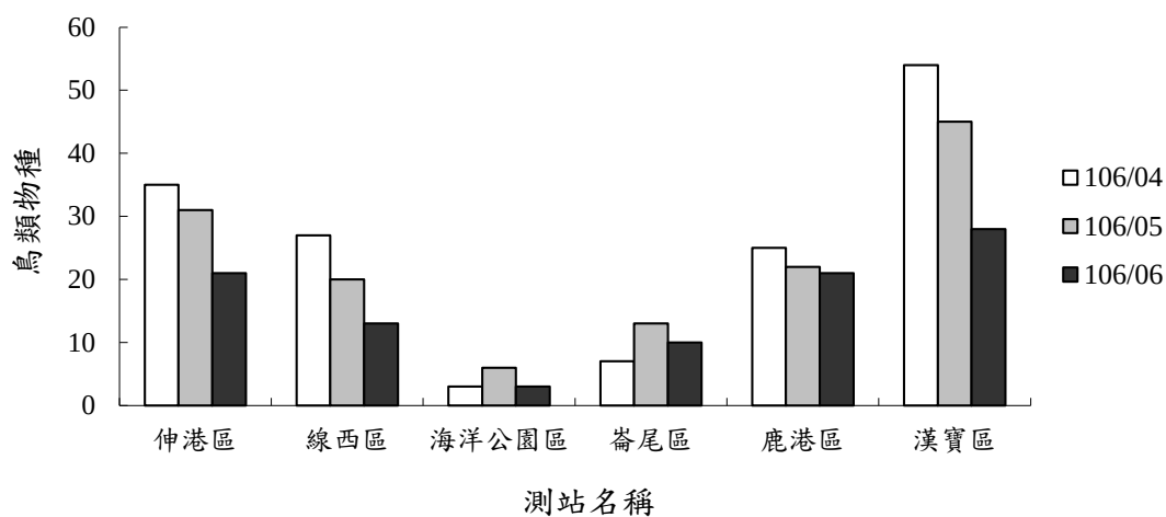
圖 2.5-1 本季各測站鳥類種數分布圖
