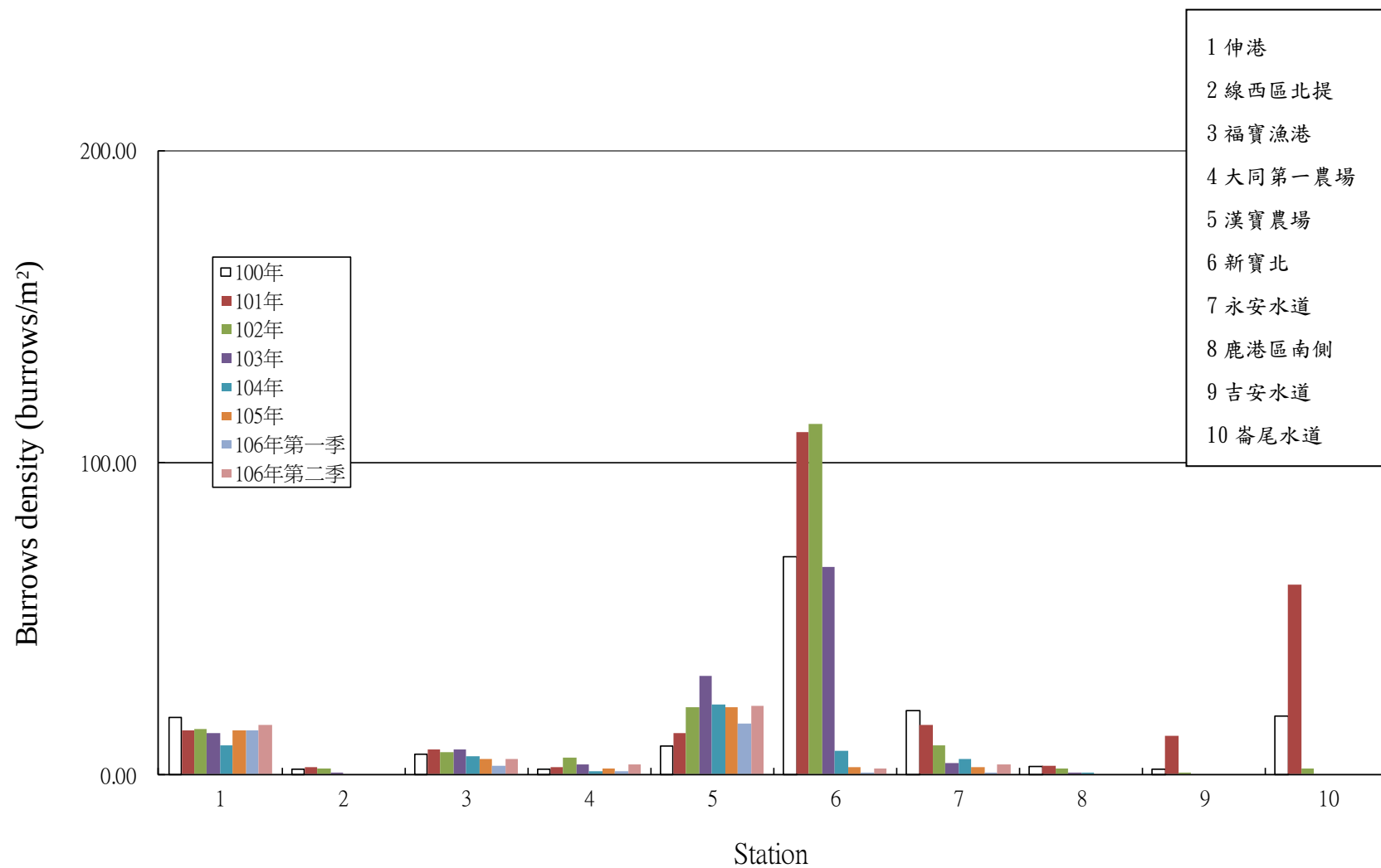
圖 3.1.6-1 各測站螻蛄蝦平均密度(平均洞口數/m²)分布圖
