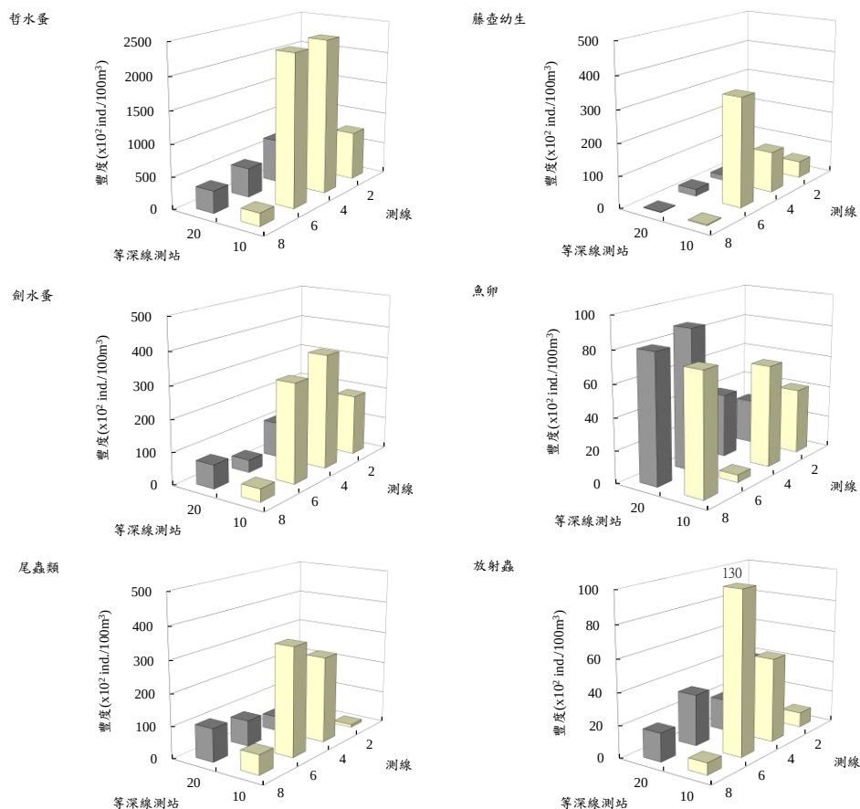
圖 2.10.2-2 民國 106 年 5 月彰化濱海工業區附近海域浮游動物主要優勢類群之豐度分布圖
