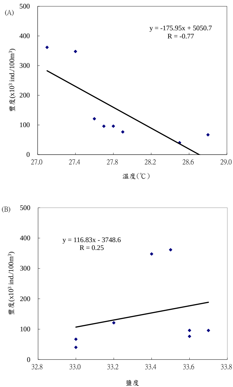
圖 2.10.2-4 民國 106 年 5 月彰濱工業區之浮游動物豐度與(A)溫度 (B)鹽度之相關係數圖
