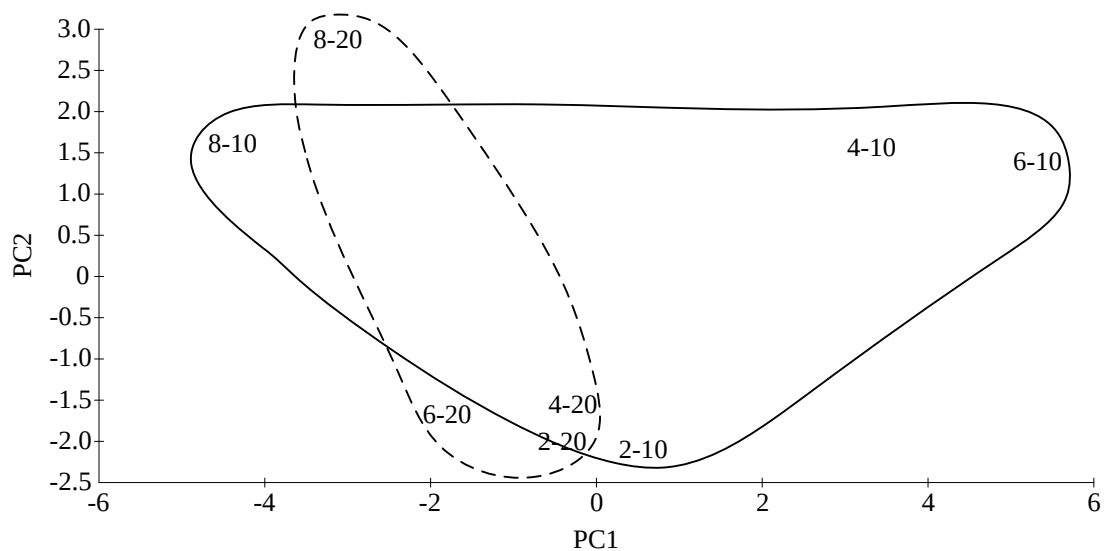
圖 2.10.2-3 民國 106 年 5 月彰濱工業區附近海域各測站浮游動物群聚分析圖(圖中第一個數字代表測站，第二個數字代表深度)
