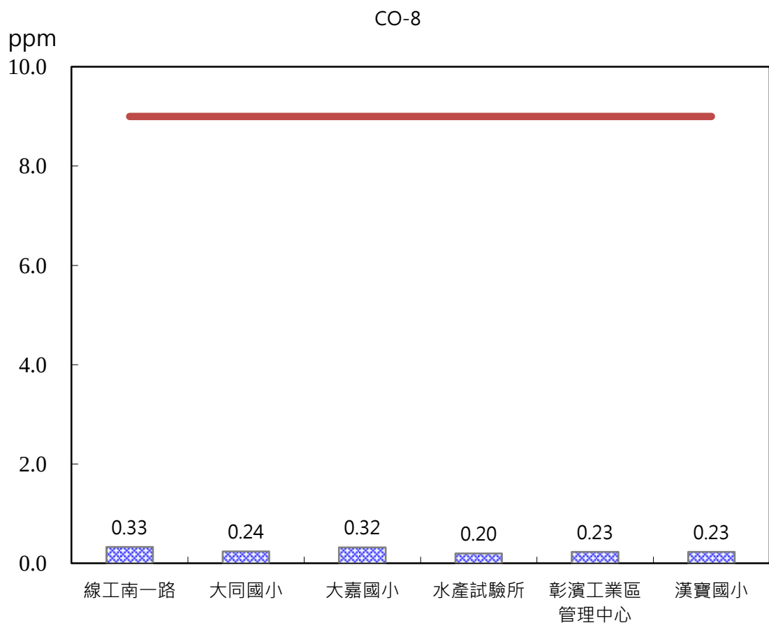
圖 2.1-1 本季各測站 CO 最高 8 小時平均值監測結果比較分析圖
