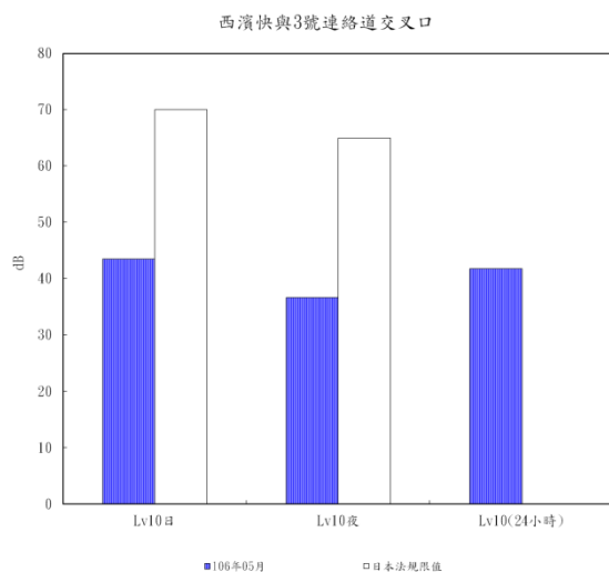
圖 2.3-3 西濱快與3號連絡道交叉口日本季振動調查結果分析圖
