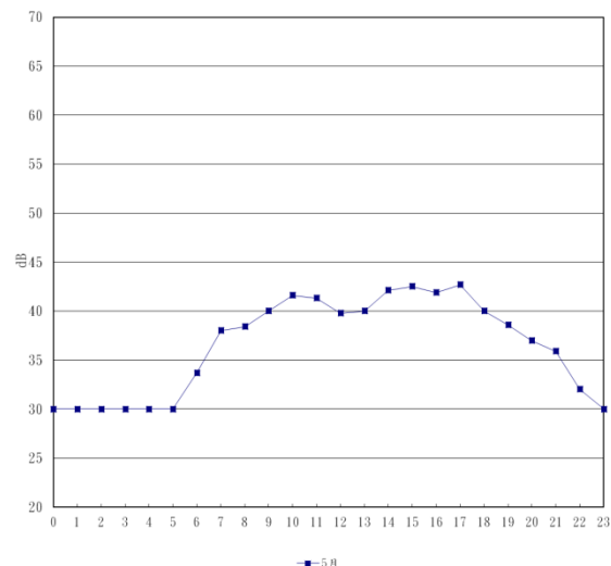
圖 2.3-6 海埔國小日本季振動測值逐時變化圖
