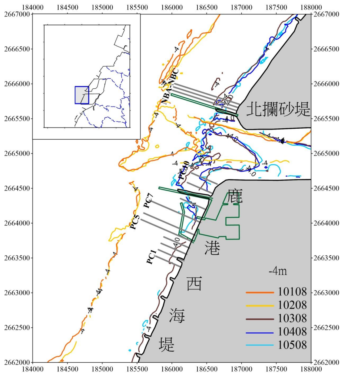
圖 2.11-4 鹿港區西海堤突堤群-4m 等深線位置比較
