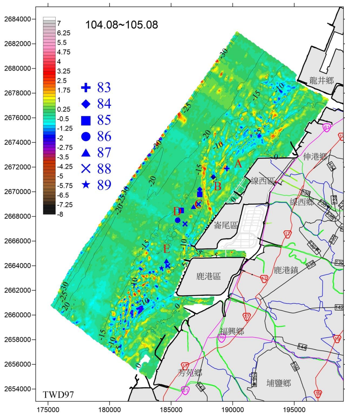
圖 2.11-3 104 年 8 月與 105 年 8 月海底地形侵淤圖
