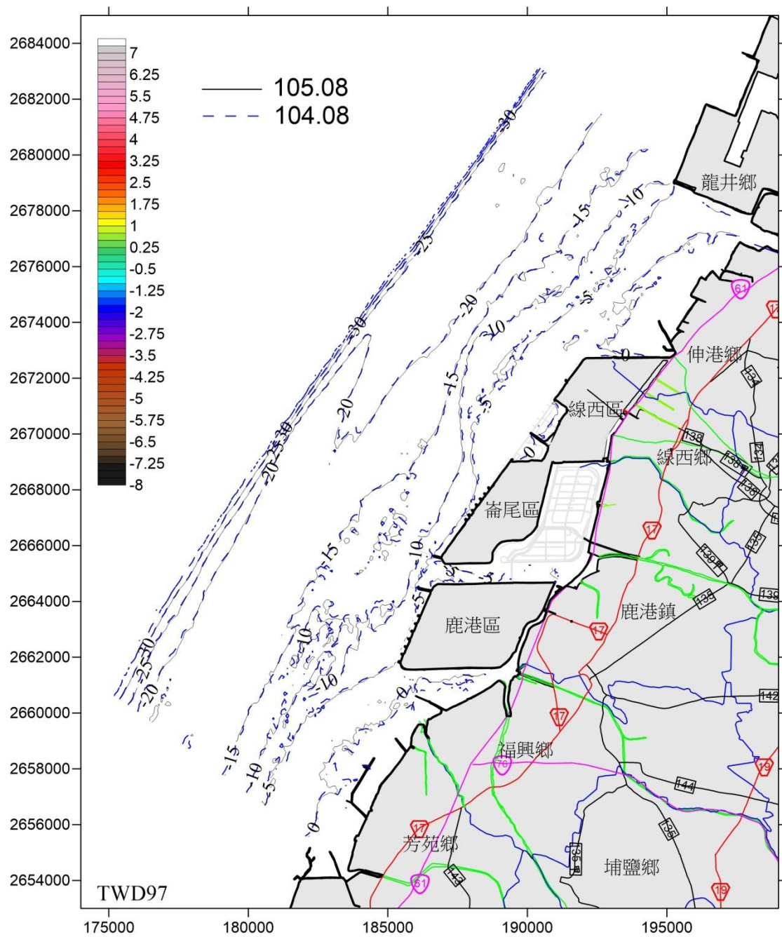
圖 2.11-2 104 年 8 月與 105 年 8 月兩次施測地形等深線比較圖
