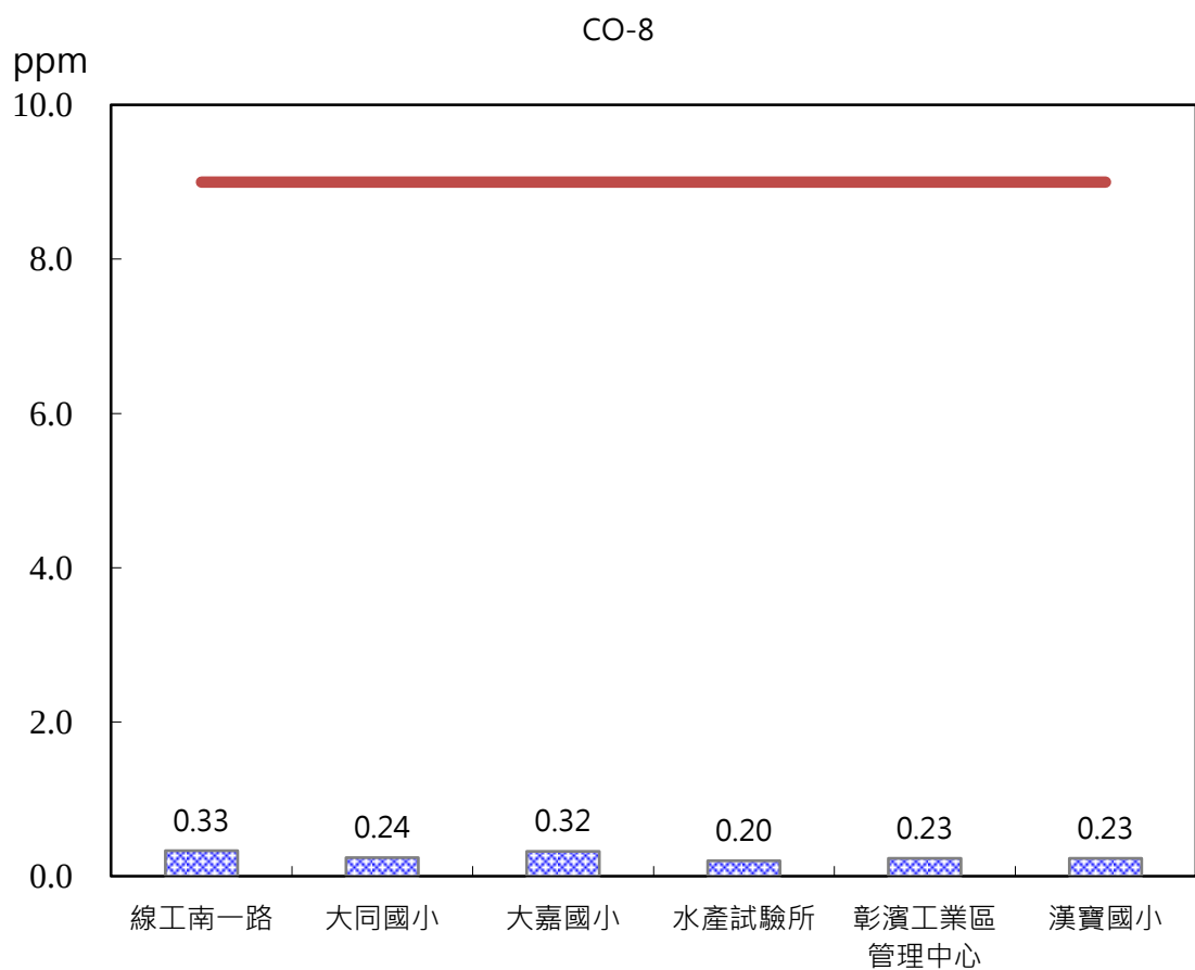
圖 2.1-2 本季各測站 CO 最高小時值監測結果比較分析圖
