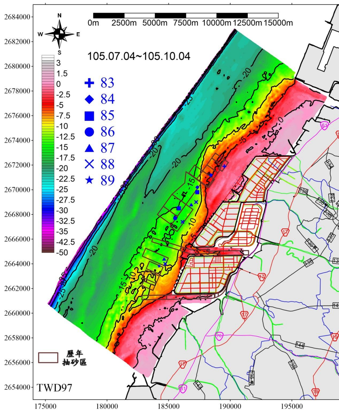
圖 2.11-1 105 年 7 月~10 月海底地形影像圖
