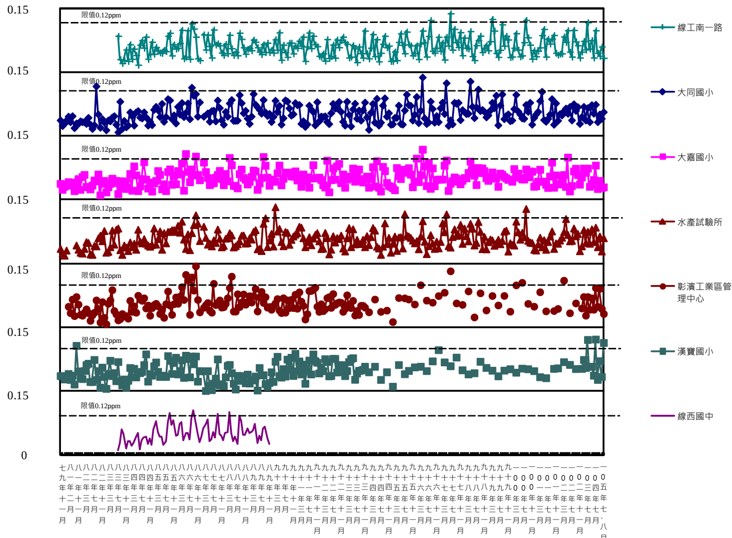
圖 3.1.1-4 彰濱地區歷年臭氧最高小時值監測結果分析圖
