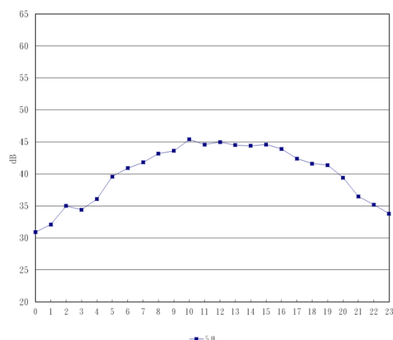
圖 2.3-4 西濱快與3號連絡道交叉口日本季振動測值逐時變化圖
