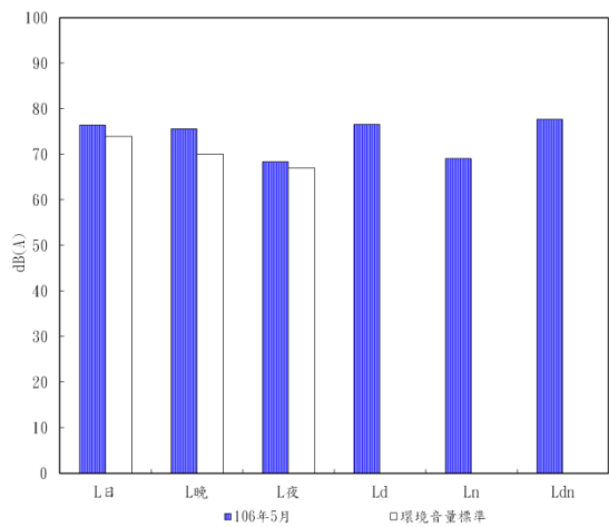
圖 2.2-5 海埔國小本季噪音調查結果分析圖
