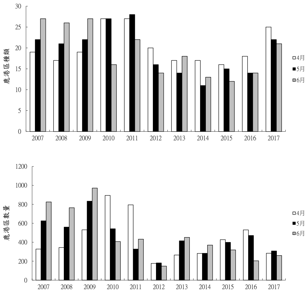
圖 3.1.5-5 鹿港區北測海堤歷年同期鳥類種類與數量調查結果比較
