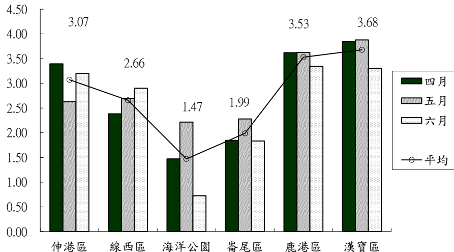
圖 2.5-3 本季各樣區歧異度指數值
