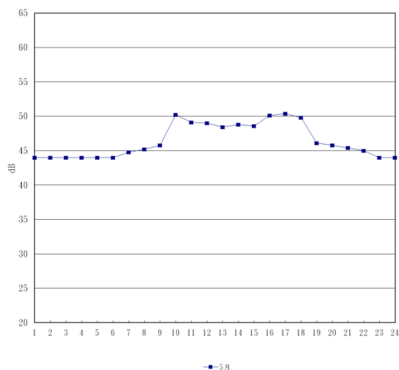
圖 2.3-2 西濱快與2號連絡道交叉口日本季振動測值逐時變化圖
