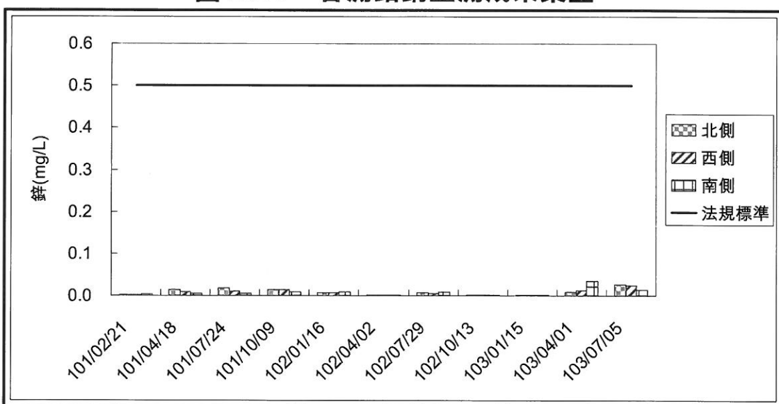
圖 2.2-8 各測站鋅監測成果彙整
