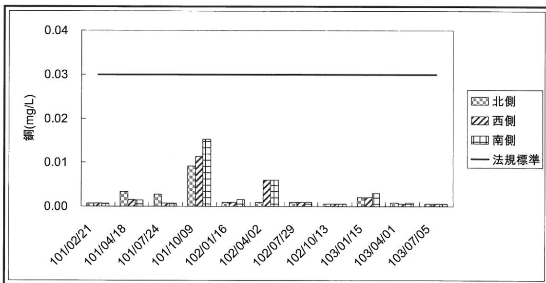
圖 2.2-7 各測站銅監測成果彙整
