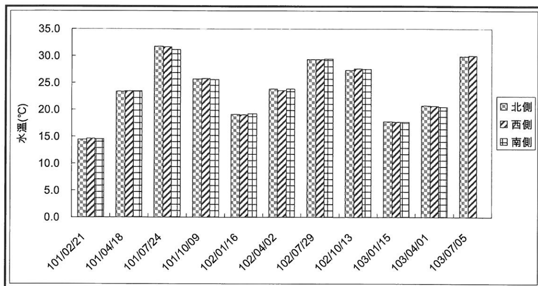
圖 2.2-1 各測站水温監測成果彙整
