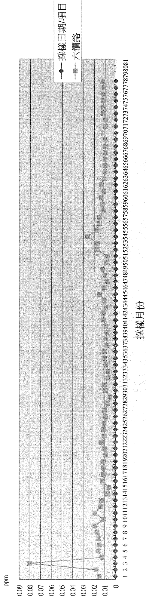
圖3.1.4.3.4 麥寮附近海域歷年來生物體內六價鉻採樣分析結果變化圖
