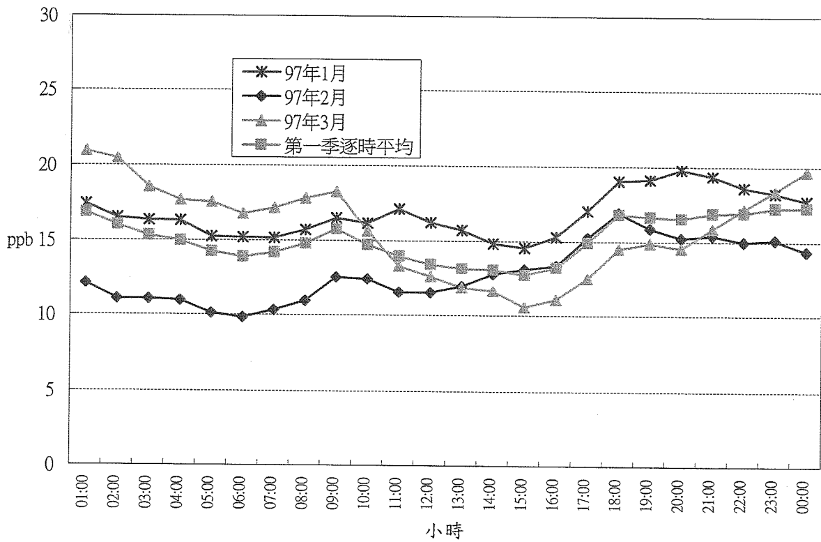
圖 3.1.1.5 土庫測站97年第1季 NO 2 逐時平均濃度變化圖(4/7)
