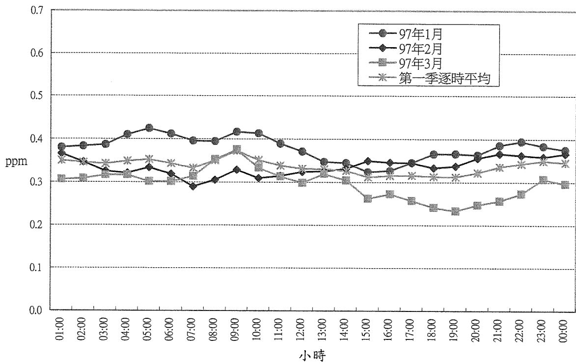
圖 3.1.1.3 麥寮測站 97年第1季CO逐時平均濃度變化圖(5/7)
