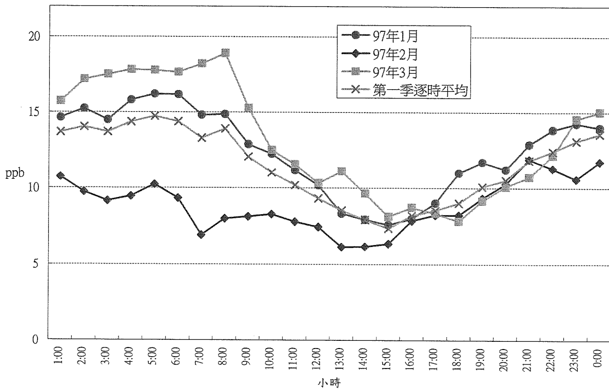
圖 3.1.1.3 麥寮測站97年第1季 NO 2 逐時平均濃度變化圖(4/7)
