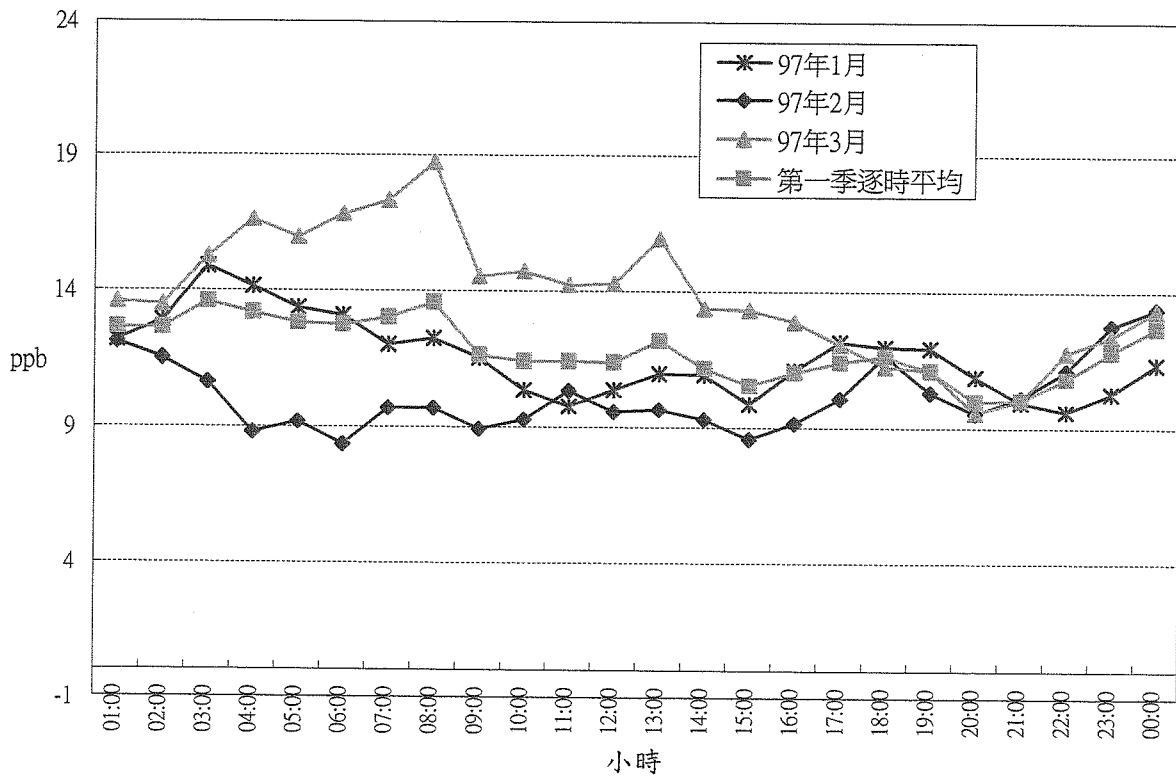
圖 3.1.1.4 台西測站97年第1季 NO 2 逐時平均濃度變化圖(4/7)
