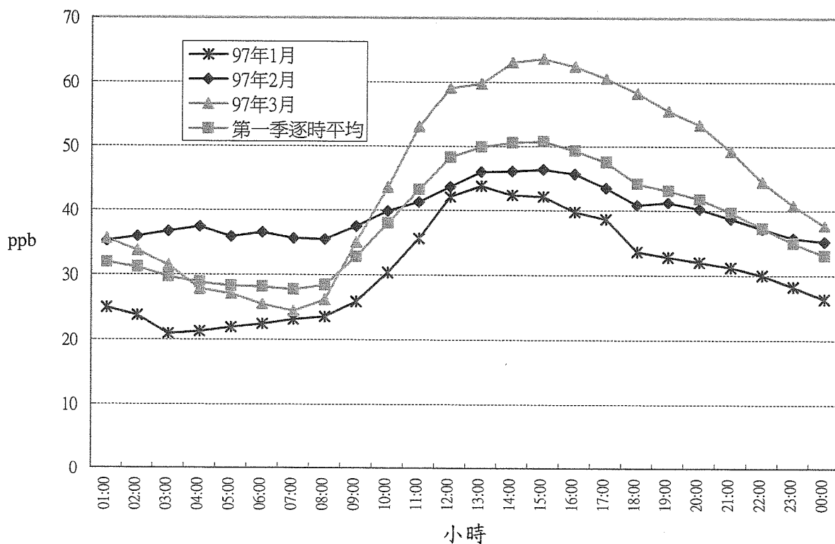
圖 3.1.1.4 台西測站97年第1季O 3 逐時平均濃度變化圖(6/7)
