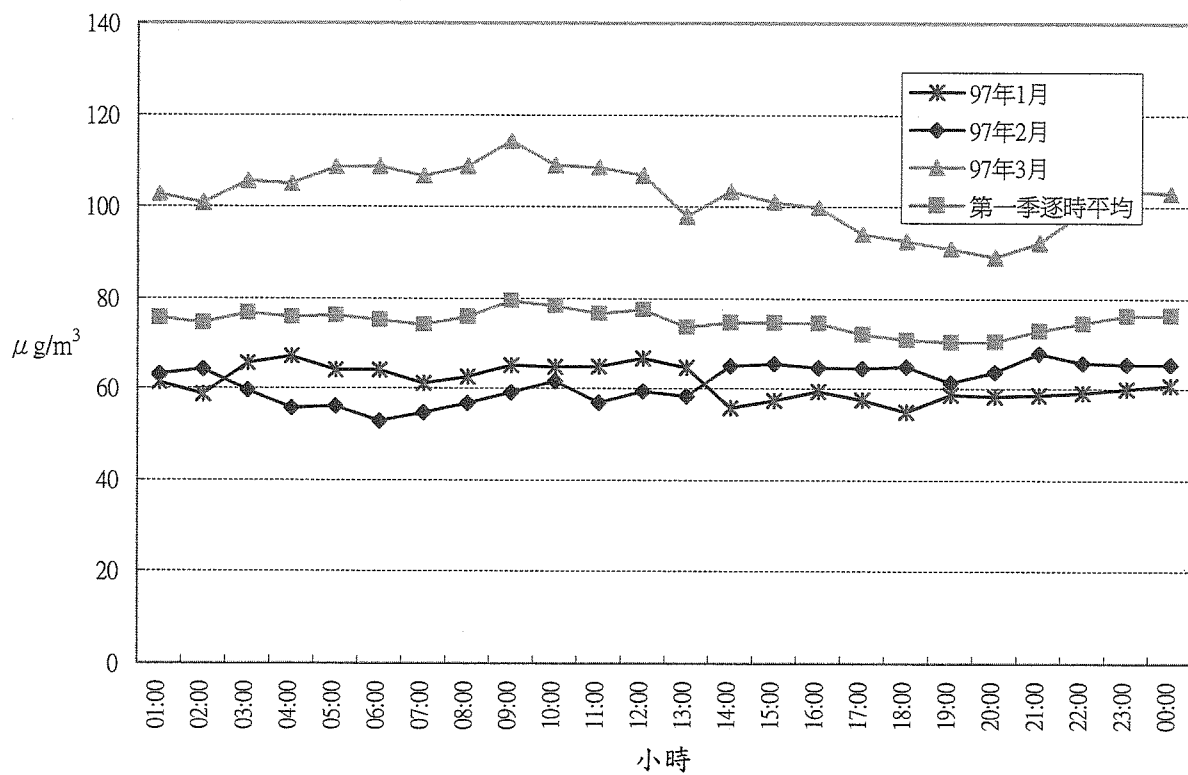
圖 3.1.1.4 台西測站97年第1季 PM10 逐時平均濃度變化圖(1/7)
