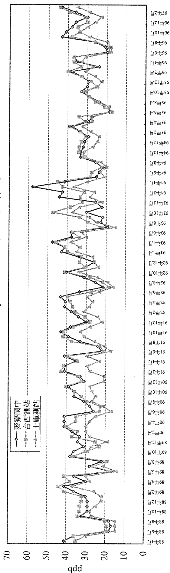
圖 3.1.1.2 O 3 三測站各月月平均比較圖 (6/6)
