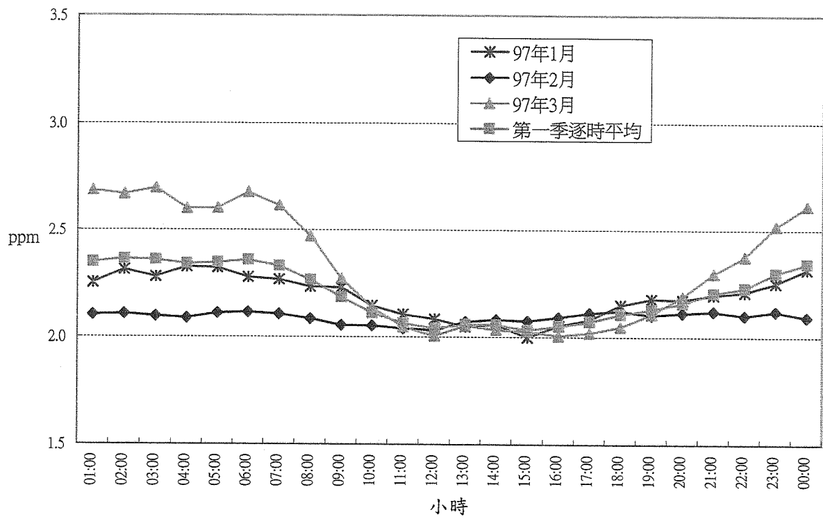
圖 3.1.1.5 土庫測站 97年第1季THC逐時平均濃度變化圖(7/7)
