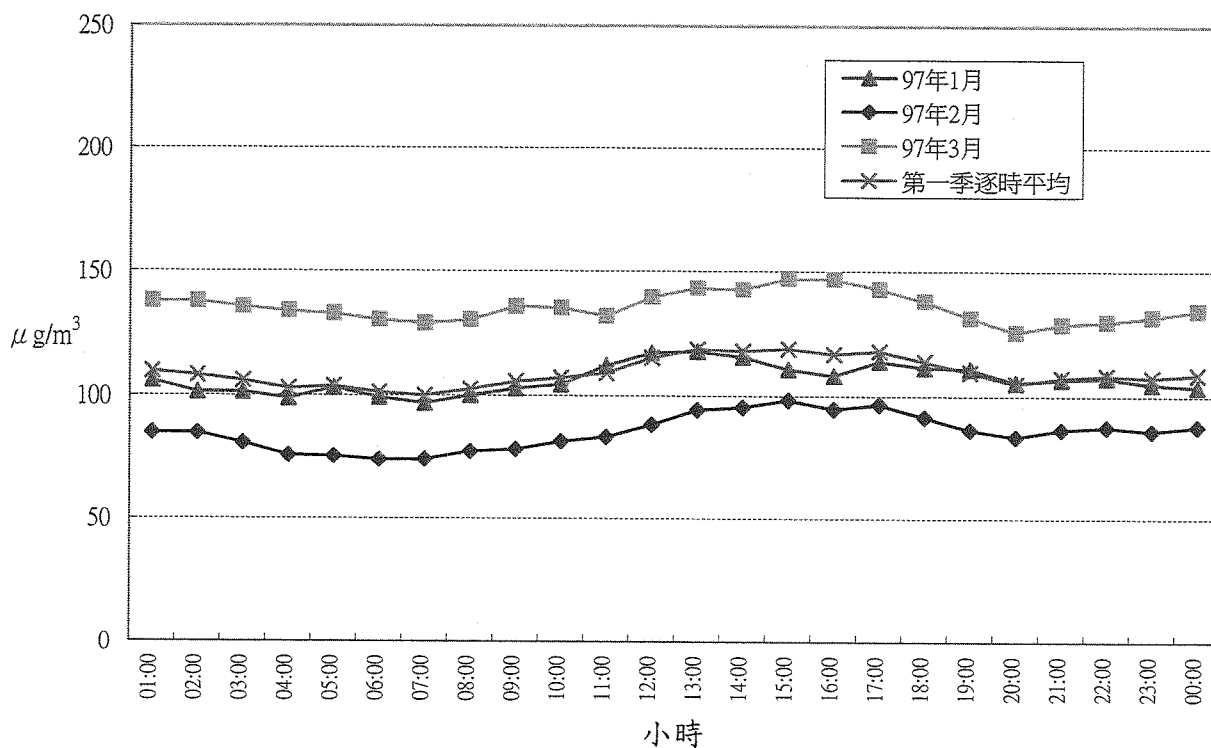
圖 3.1.1.3 麥寮測站 97年第1季 TSP 逐時平均濃度變化圖(2/7)
