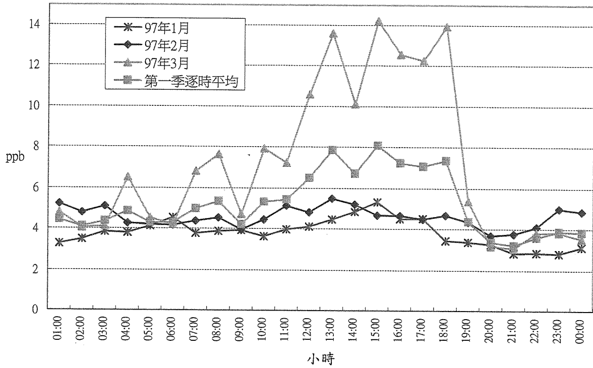
圖 3.1.1.4 台西測站97年第1季SO 2 逐時平均濃度變化圖(3/7)
