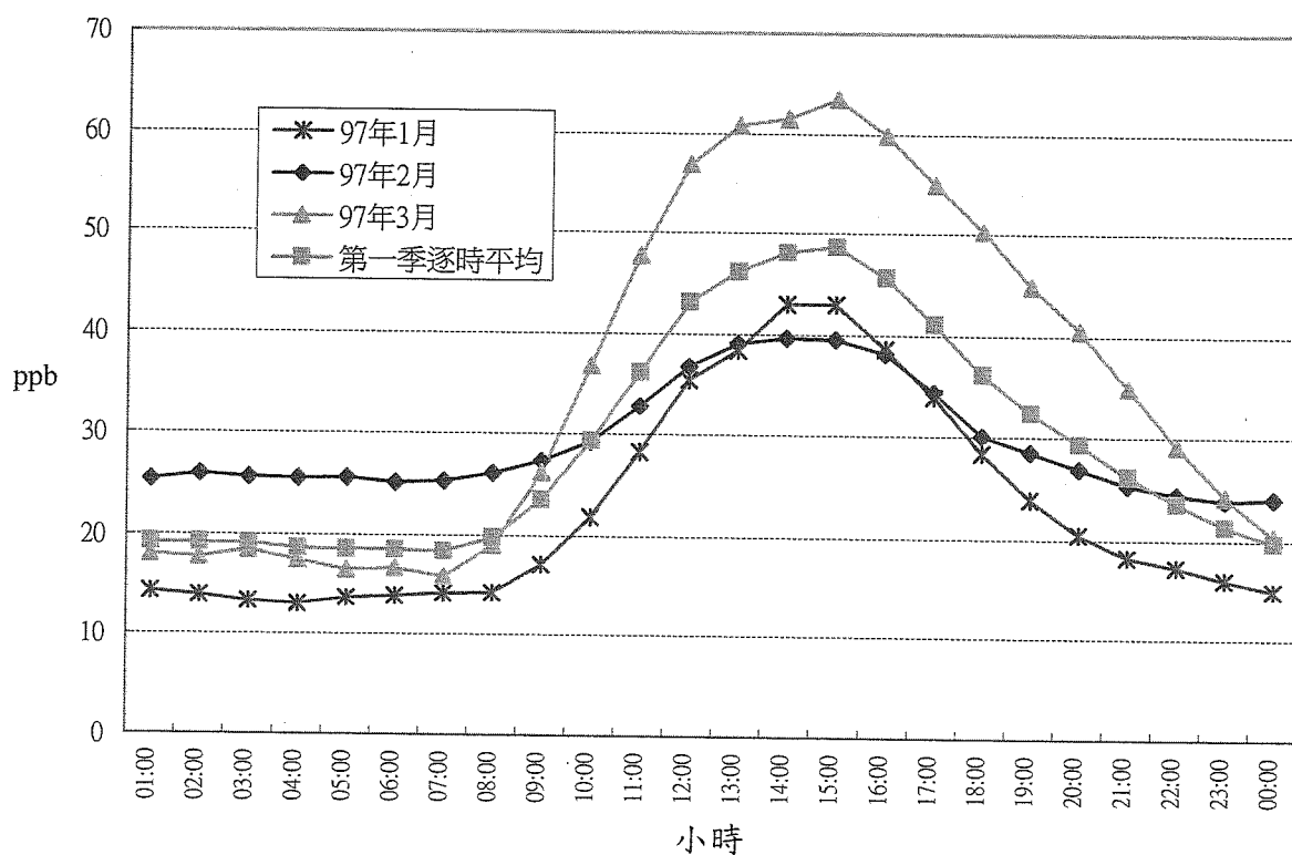
圖 3.1.1.5 土庫測站97年第1季O 3 逐時平均濃度變化圖(6/7)
