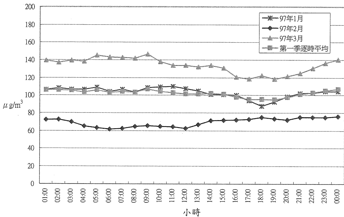
圖 3.1.1.4 台西測站 97年第1季 TSP 逐時平均濃度變化圖(2/7)
