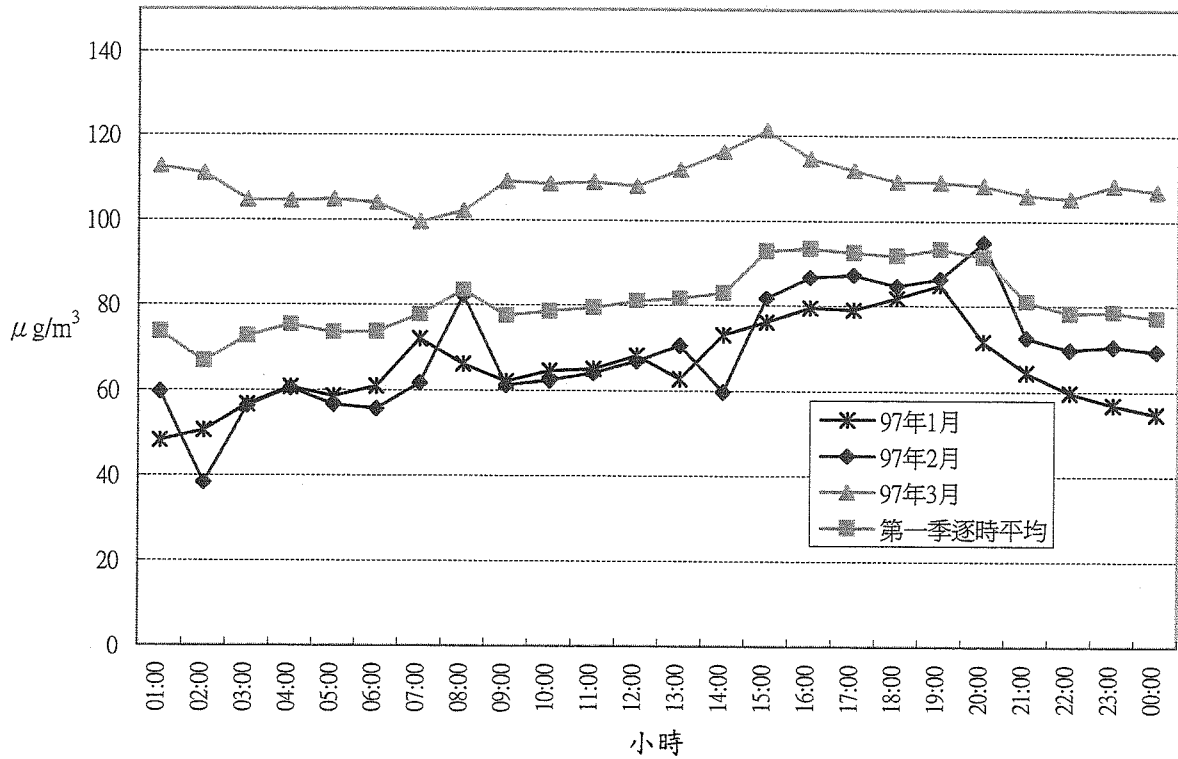
圖 3.1.1.5 土庫測站97年第1季 PM 10 逐時平均濃度變化圖(1/7)
