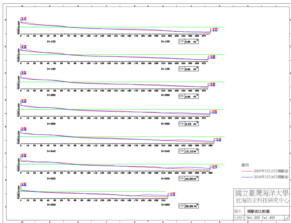
圖 4-5(f) 2016 年 3 月 18 日 B 監測區橫断面比較圖
