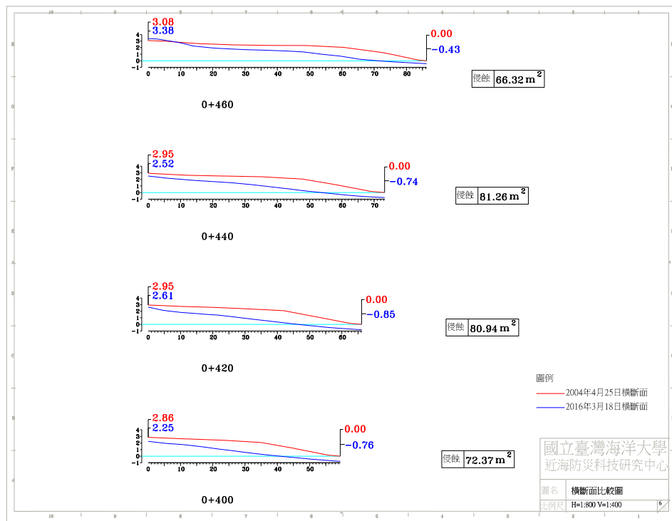
圖 4-4(e) 2016 年 3 月 18 日 A 監測區橫斷面比較圖
