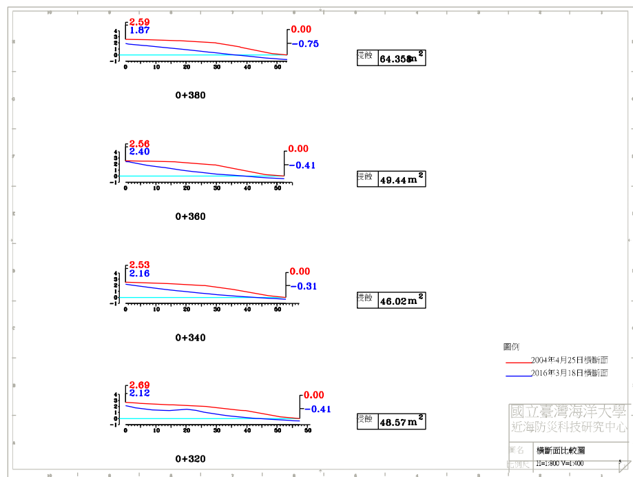
圖 4-4(f) 2016 年 3 月 18 日 A 監測區橫斷面比較圖
