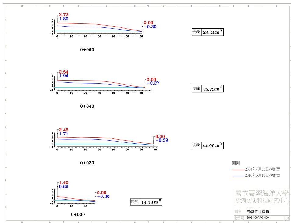
圖 4-4(j) 2016 年 3 月 18 日 A 監測區橫斷面比較圖
