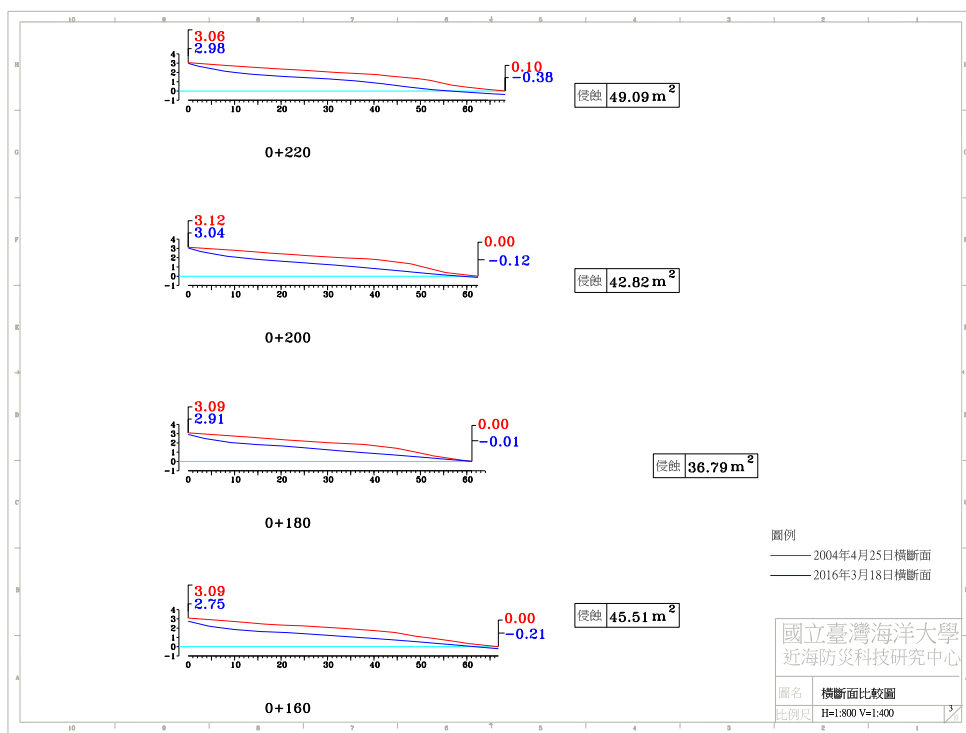
圖 4-4(h) 2016 年 3 月 18 日 A 監測區橫斷面比較圖
