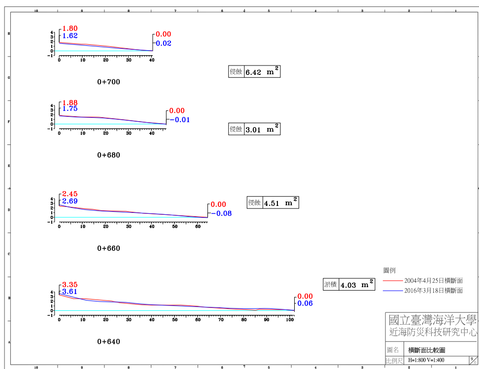
圖 4-4(b) 2016 年 3 月 18 日 A 監測區橫斷面比較圖
