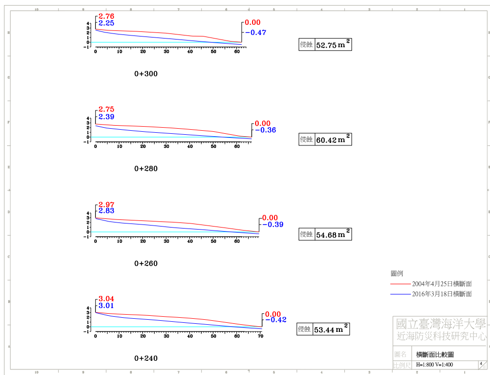
圖 4-4(g) 2016 年 3 月 18 日 A 監測區橫斷面比較圖
