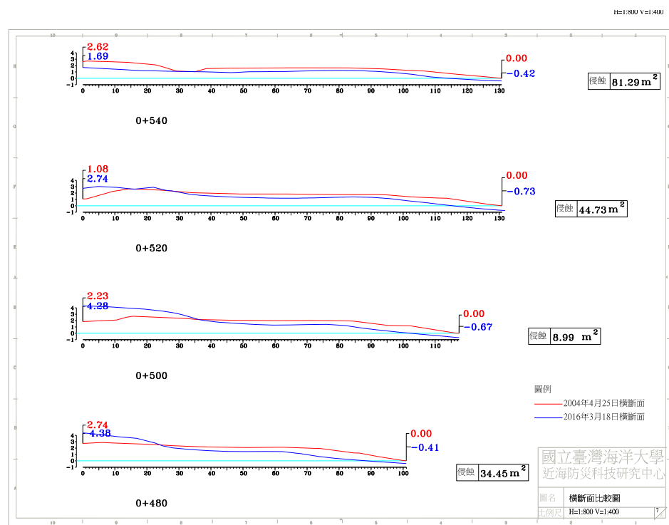
圖 4-4(d) 2016 年 3 月 18 日 A 監測區橫斷面比較圖
