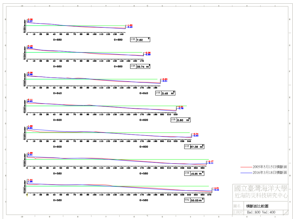
圖 4-5(b) 2016 年 3 月 18 日 B 監測區橫斷面比較圖
