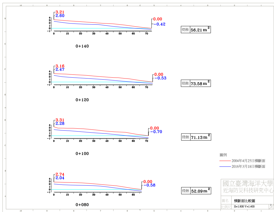
圖 4-4(i) 2016 年 3 月 18 日 A 監測區橫斷面比較圖
