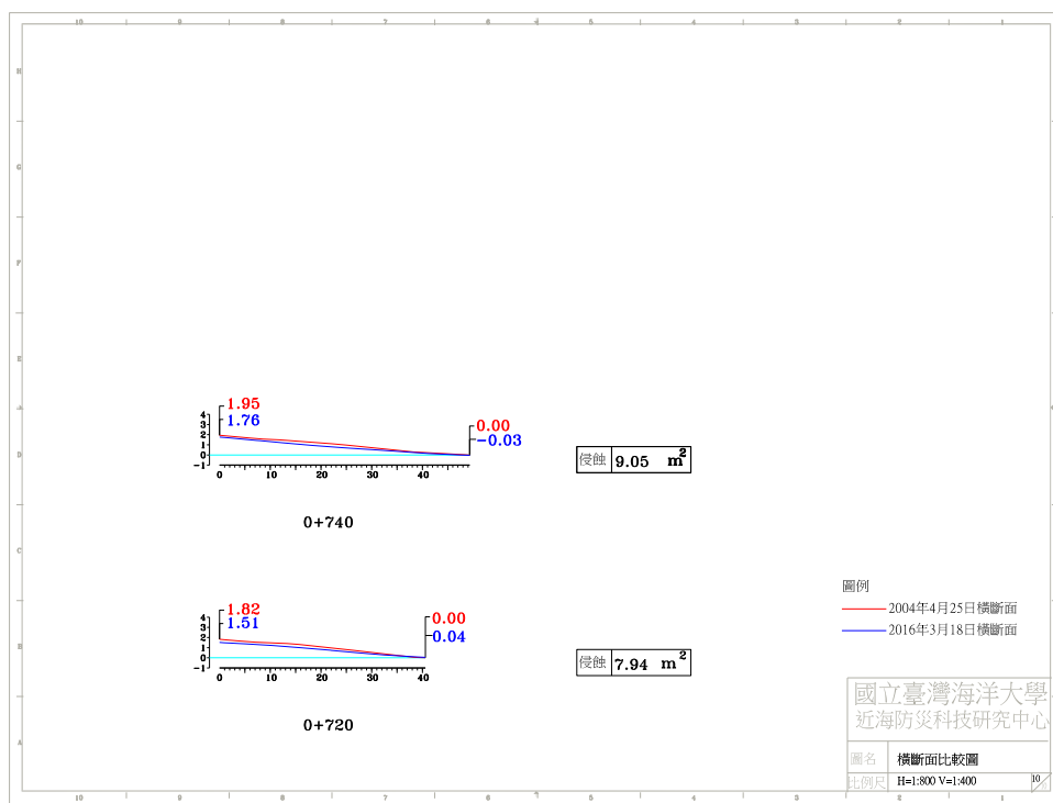
圖 4-4(a) 2016 年 3 月 18 日 A 監測區橫斷面比較圖
