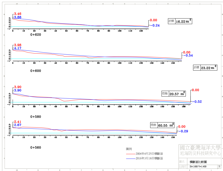
圖 4-4(c) 2016 年 3 月 18 日 A 監測區橫斷面比較圖
