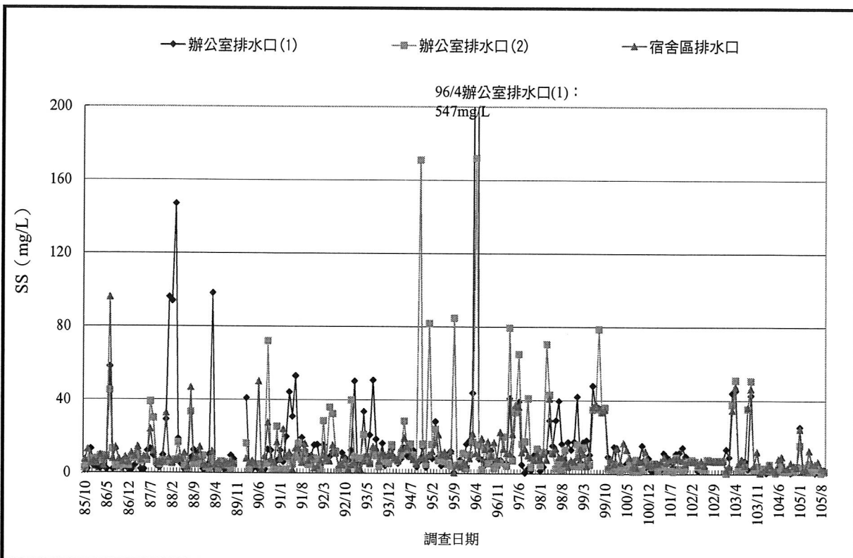
圖3.1-7 核四環境監測廠區水質歷年調查懸浮固體濃度變化圖
