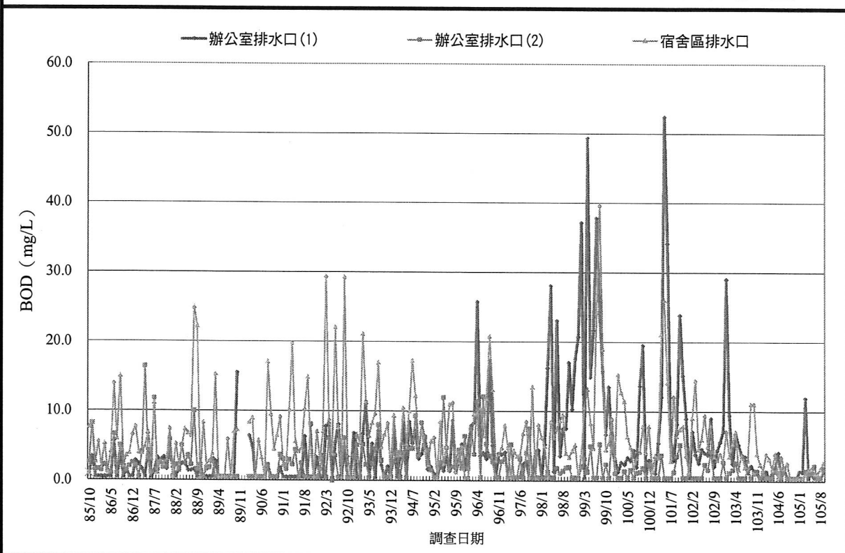
圖3.1-8 核四環境監測廠區水質歷年調查生化需氧量變化圖
