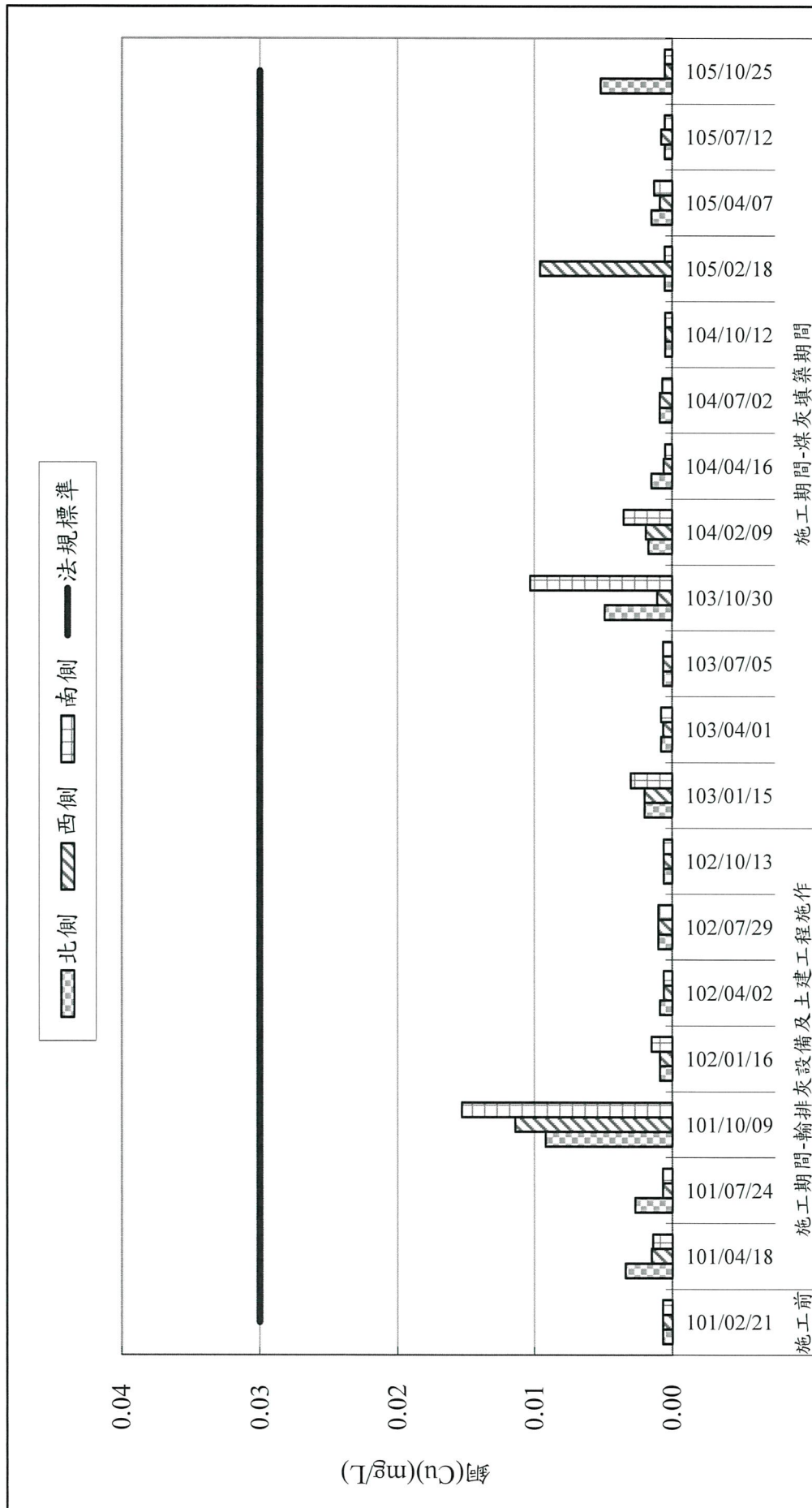
圖 2.2-7 歷季各測站銅(Cu)監測成果彙整
