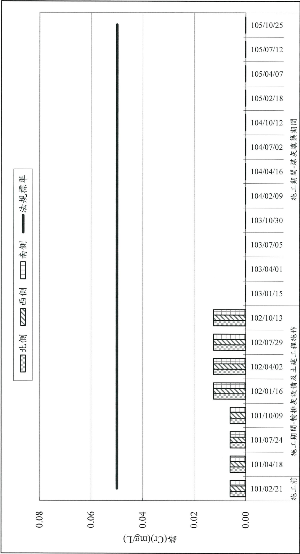
圖 2.2-12 歷季各測站鉻(Cr)監測成果彙整
