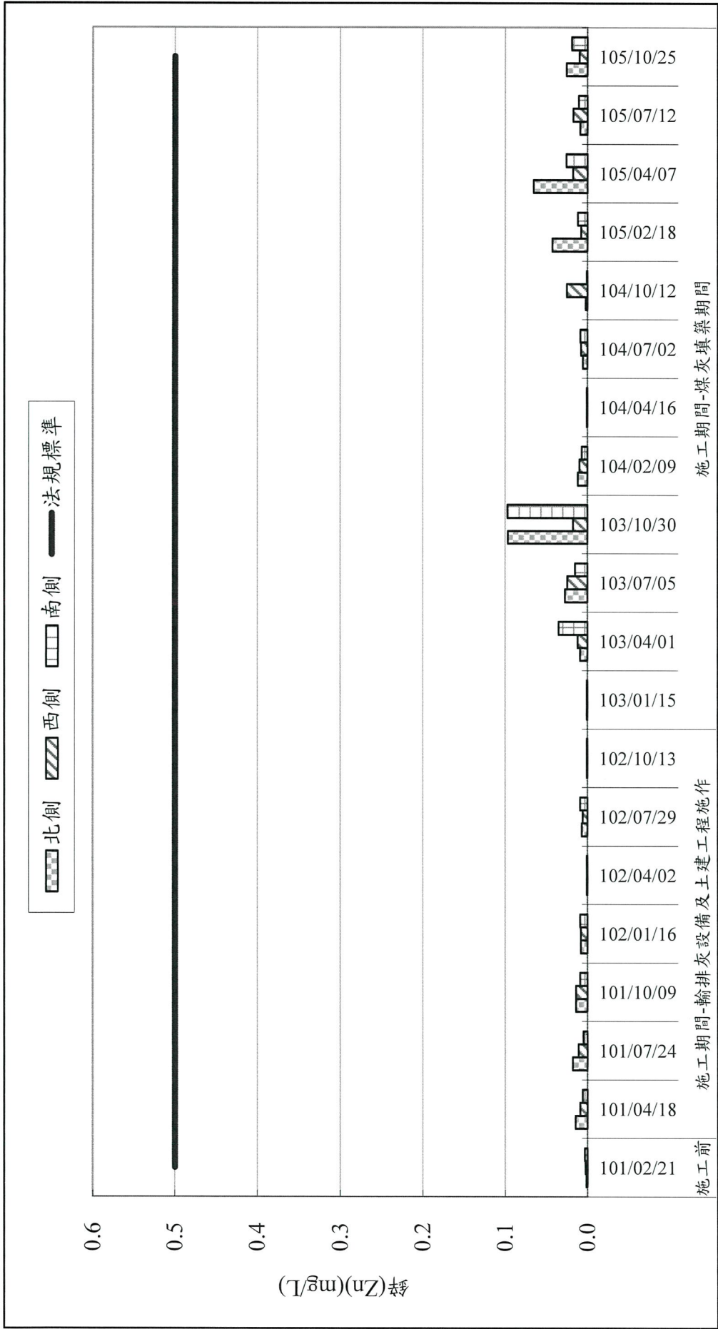
圖 2.2-9 歷季各測站鋅(Zn)監測成果彙整
