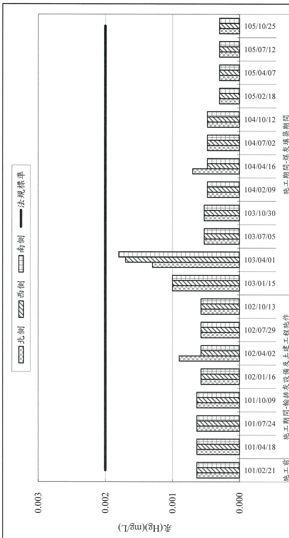
圖 2.2-13 歷季各測站汞(Hg)監測成果彙整
