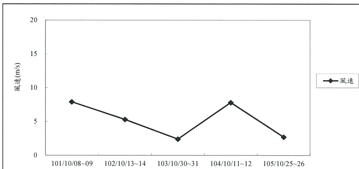
圖 3.1-1 歷年同期風速監測成果彙整
