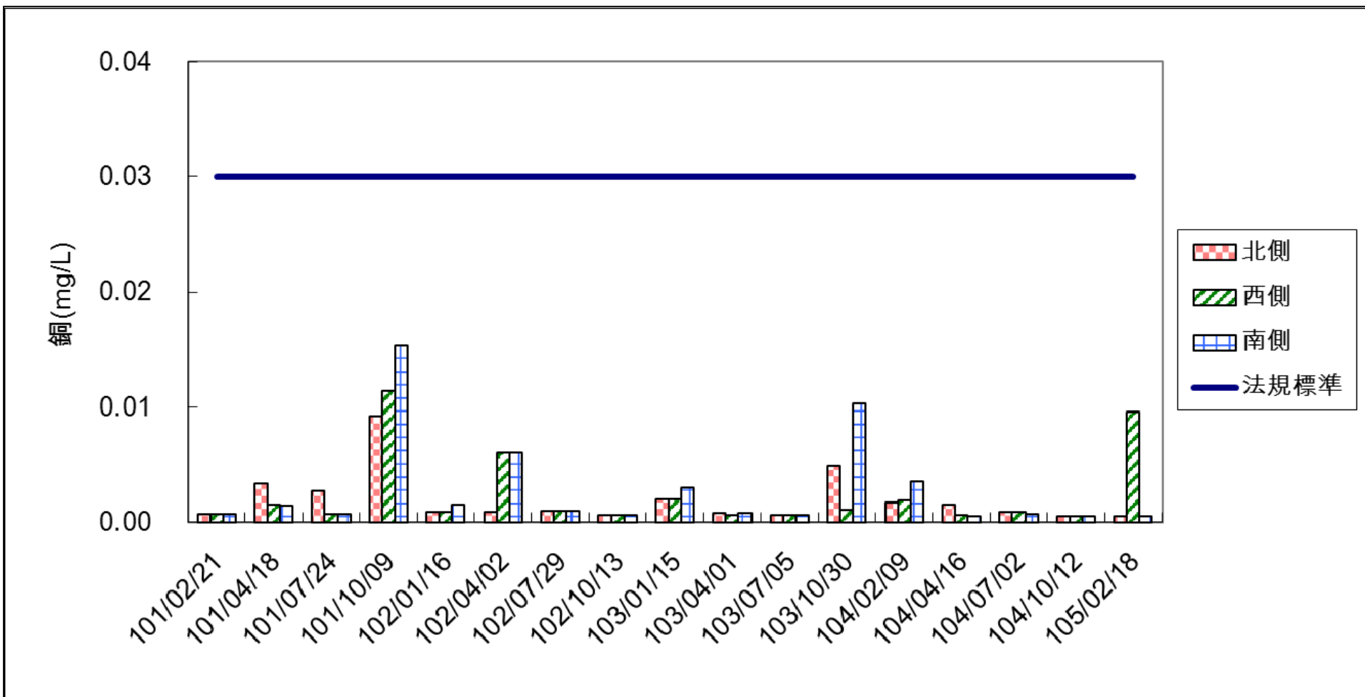
圖 2.2-7 各測站銅監測成果彙整
