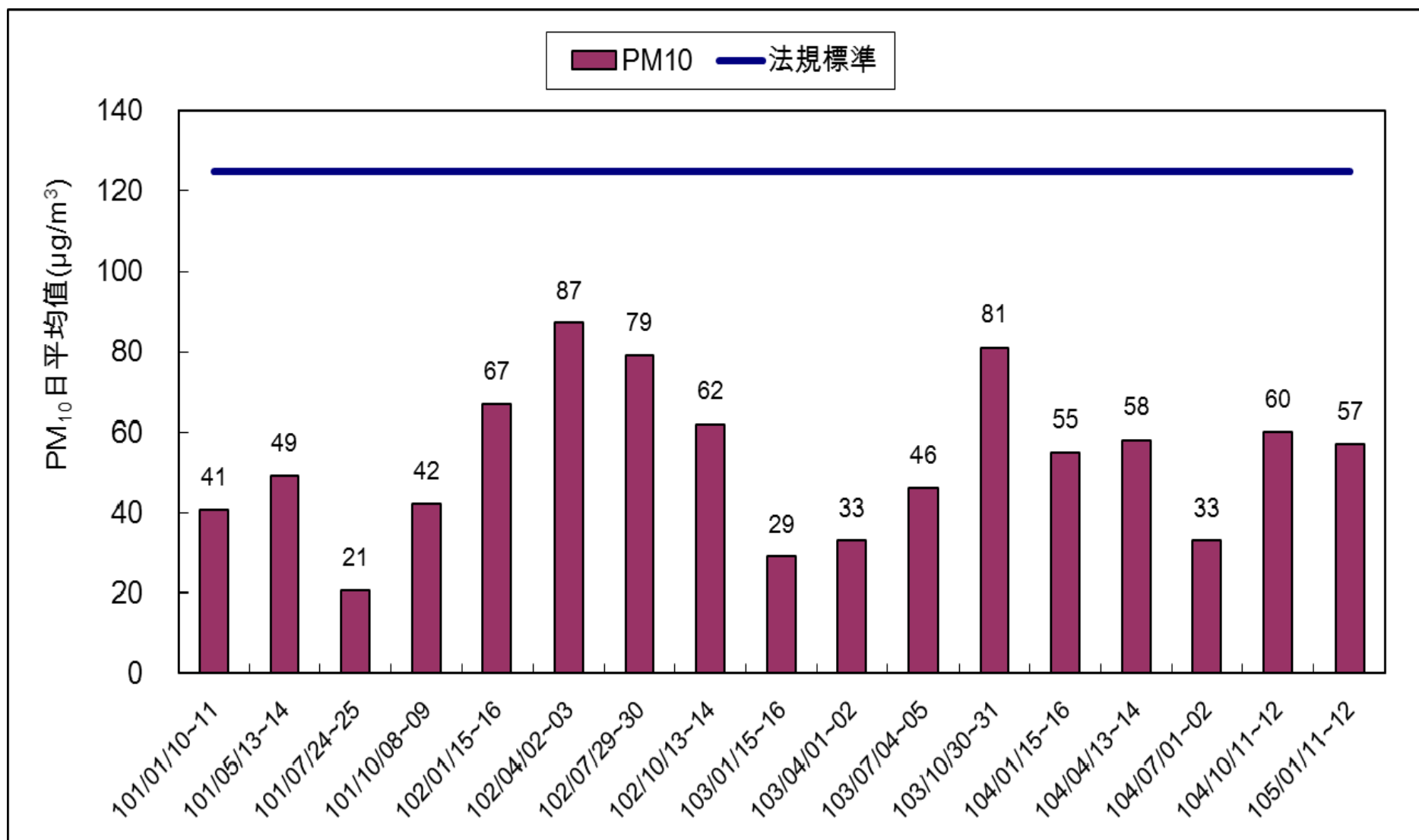
圖 2.1-2 粒徑 \leq 10\mu\text{m} 之懸浮微粒日平均值監測成果彙整
