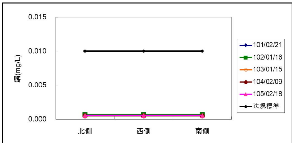
圖 3.1-19 歷年同期各測站鎘監測成果彙整
