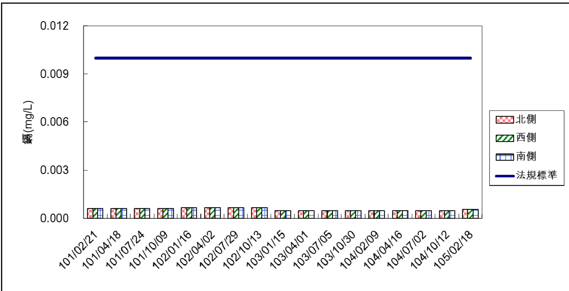
圖 2.2-11 各測站鉛監測成果彙整
