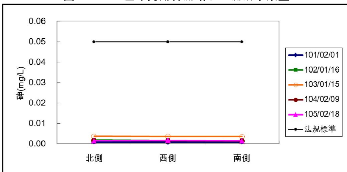
圖 3.1-22 歷年同期各測站砷監測成果彙整
