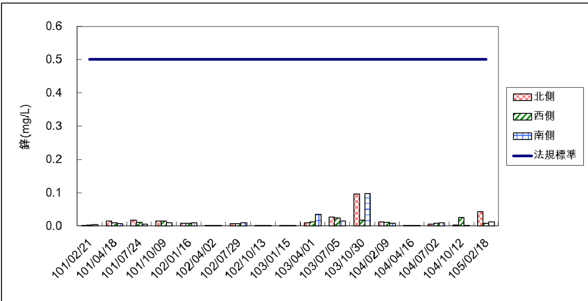
圖 2.2-9 各測站鋅監測成果彙整
