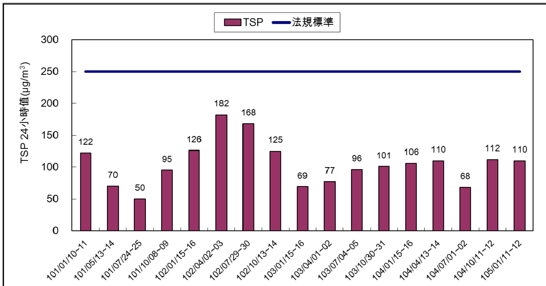
圖 2.1-1 總懸浮微粒 24 小時值監測成果彙整
