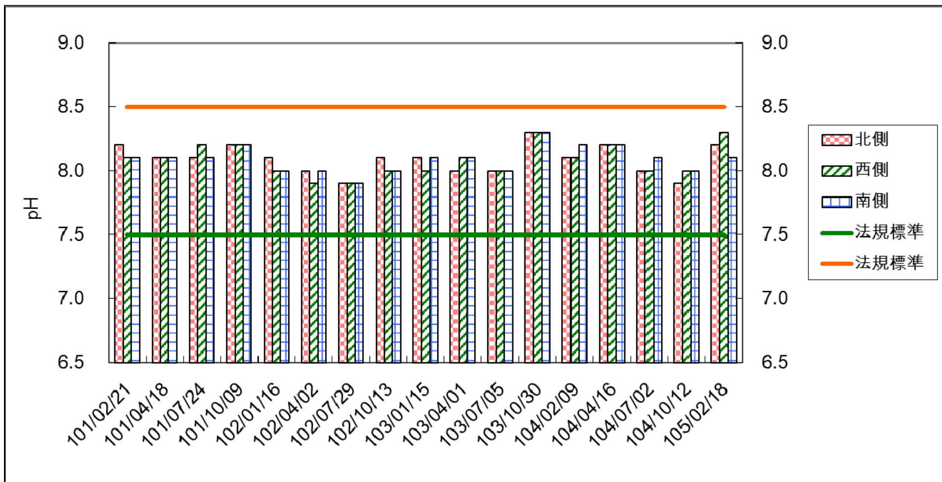
圖 2.2-6 各測站 pH 監測成果彙整
