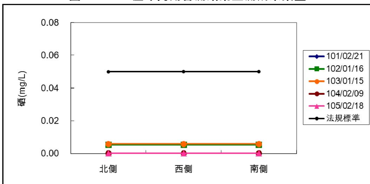
圖 3.1-16 歷年同期各測站硒監測成果彙整
