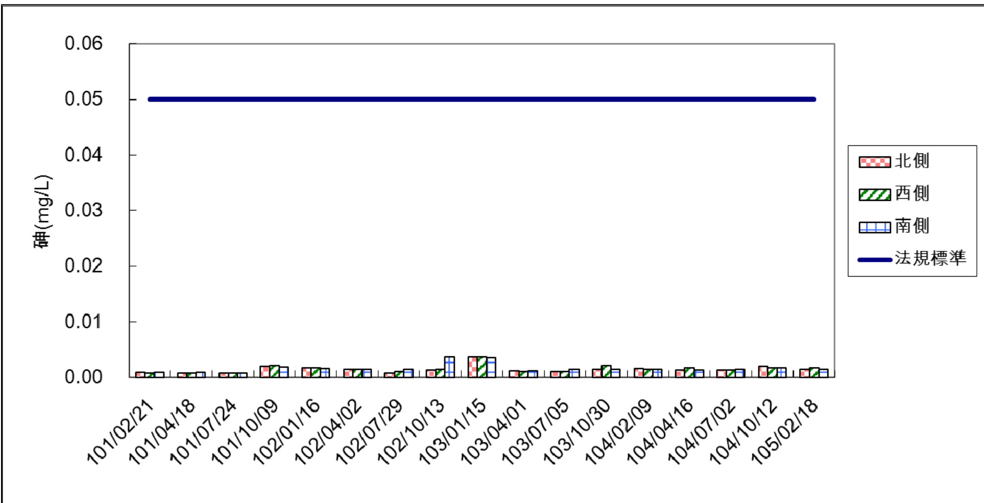
圖 2.2-14 各測站砷監測成果彙整
