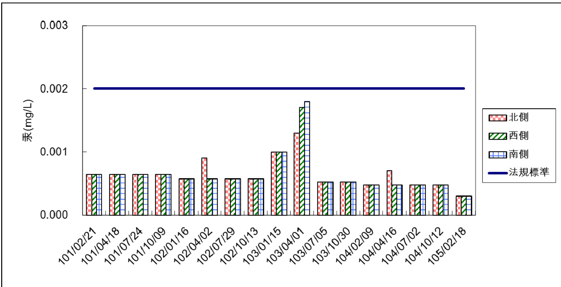
圖 2.2-13 各測站汞監測成果彙整
