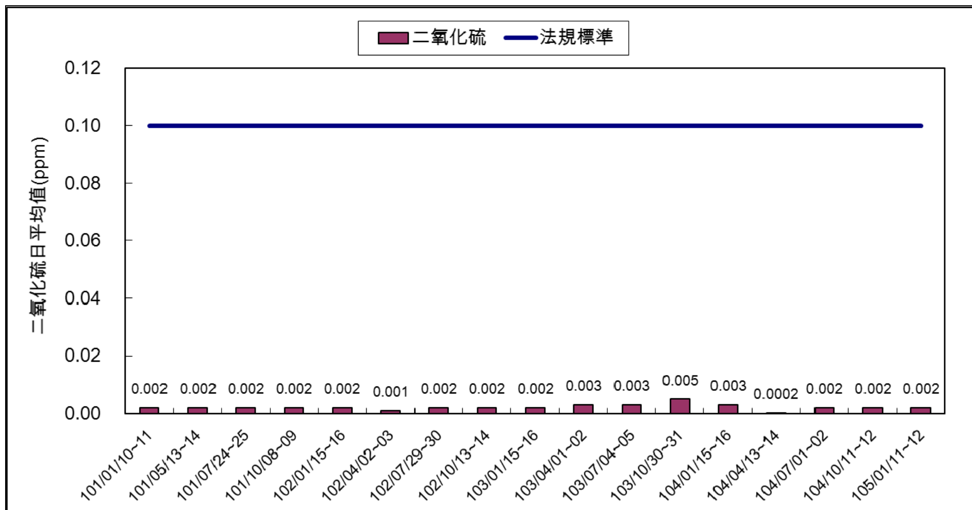
圖 2.1-4 二氧化硫日平均值監測成果彙整
