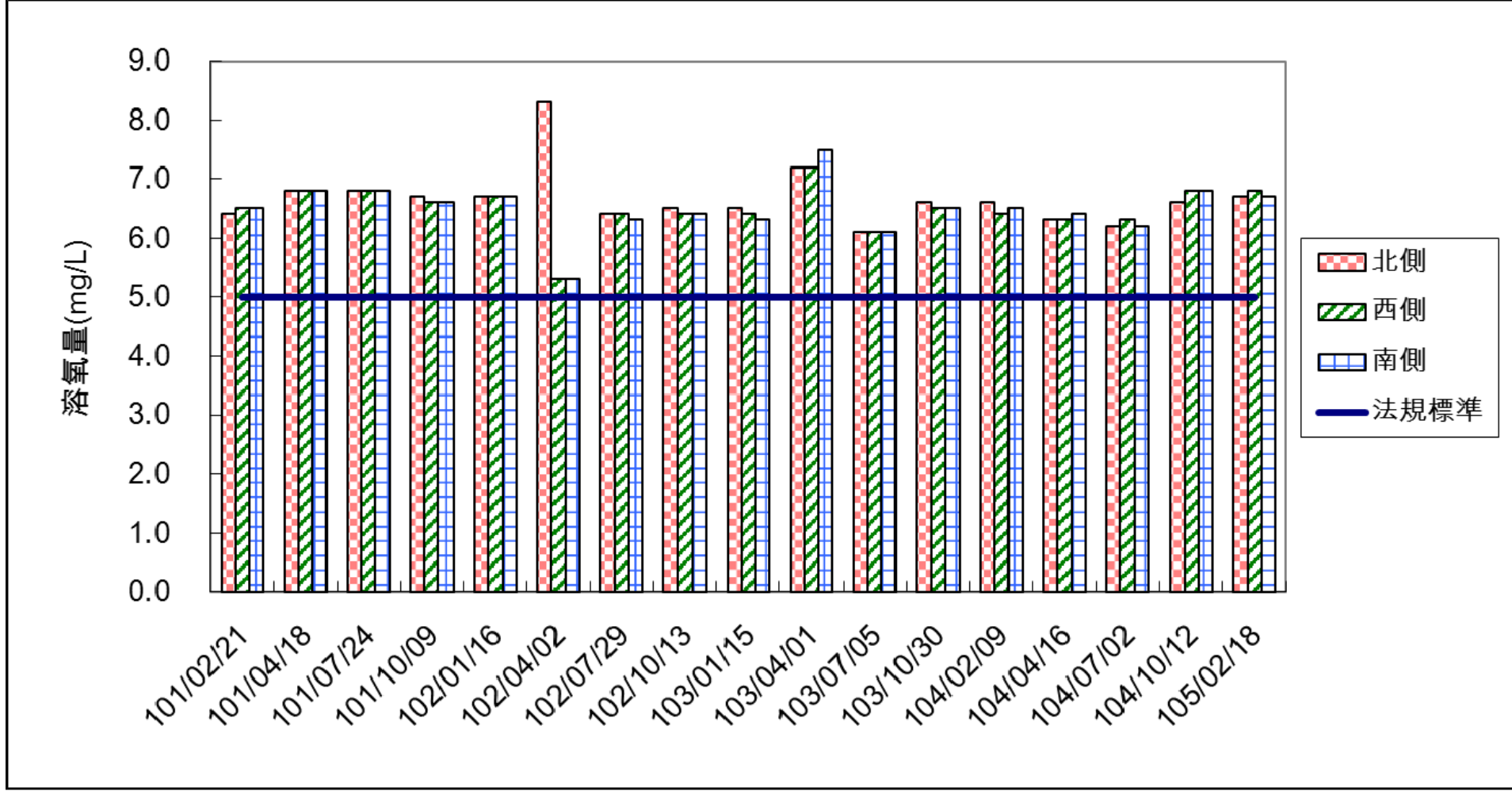
圖 2.2-3 各測站溶氧量監測成果彙整
