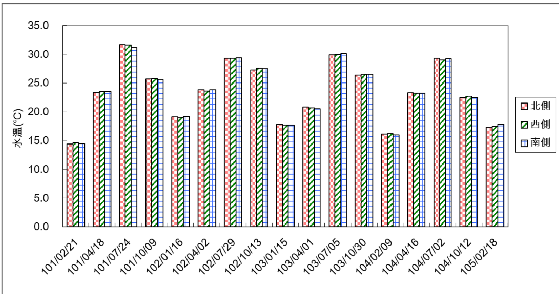
圖 2.2-1 各測站水溫監測成果彙整
