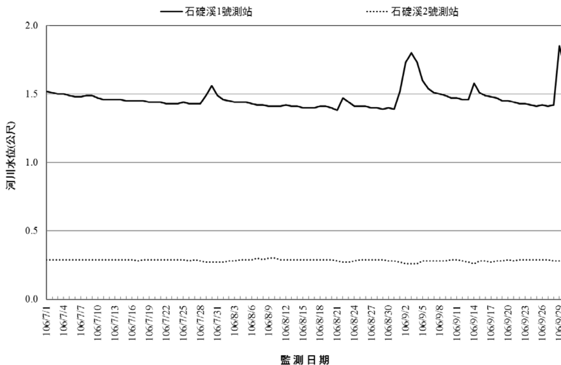
圖 2.2-1 核四封存期間河川水文 106 年 7~9 月水位變化圖
