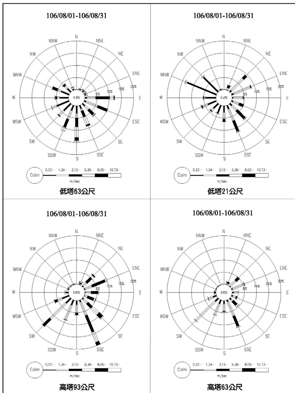
圖 2.1-2 核四封存期間環境監測氣象塔 106 年 8 月風花圖
