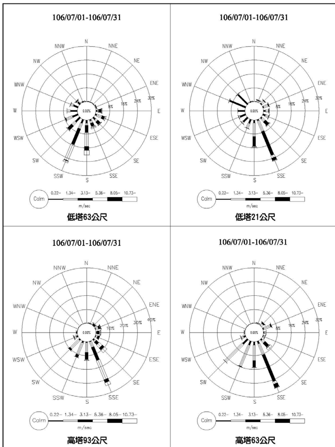
圖 2.1-1 核四封存期間環境監測氣象塔 106 年 7 月風花圖
