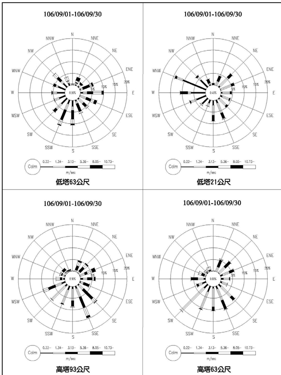
圖 2.1-3 核四封存期間環境監測氣象塔 106 年 9 月風花圖
