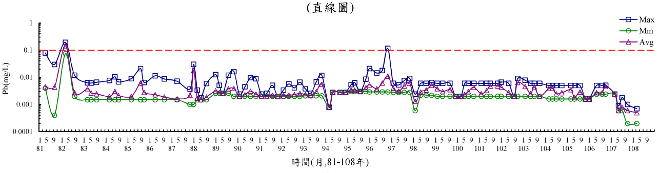
圖3.1.9-16 離島工業區海域歷年水質變化圖(Pb)
