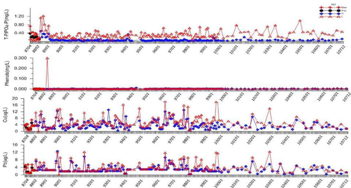
圖 2.9-1 新興區潮間帶水質歷次調查結果(續 6)
