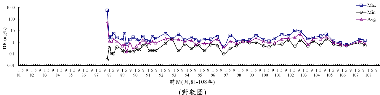
圖3.1.9-24 離島工業區海域歷年水質變化圖(TOC)
