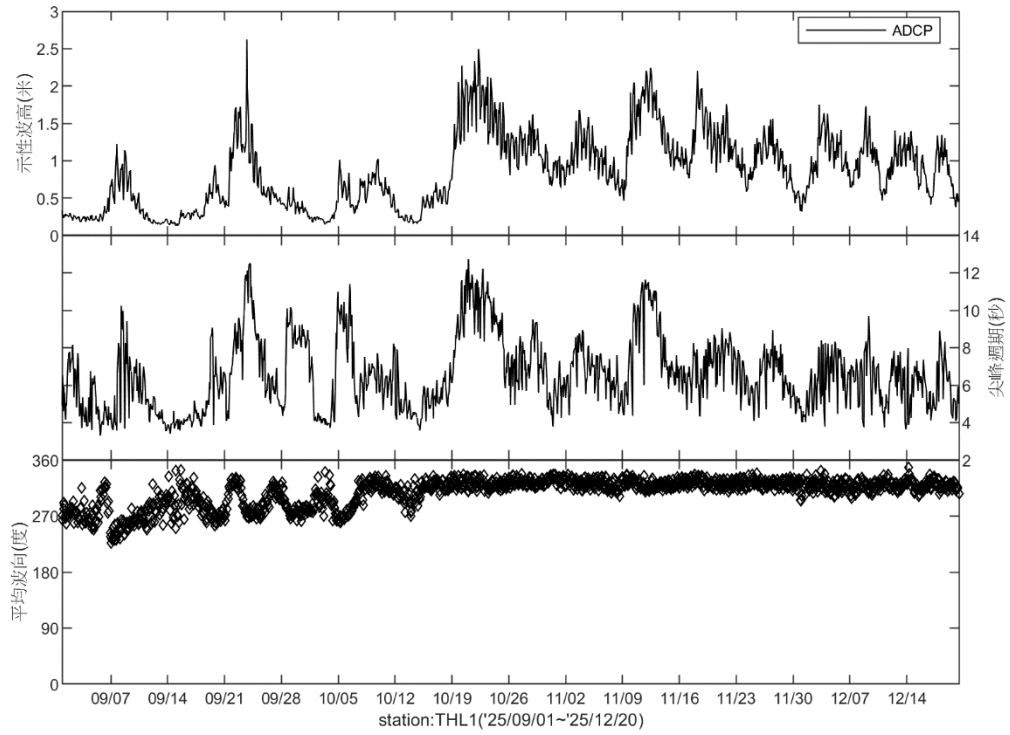
圖 2.13-6 THL1 測站 2025 年 9 月~12 月波浪時序列
