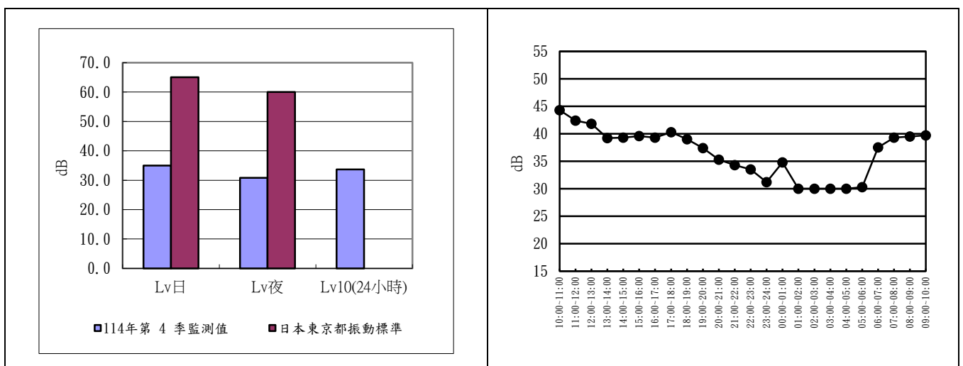
圖 2.3-3 崙豐國小 114 年度第 4 季振動監測成果分析圖及逐時變化圖
