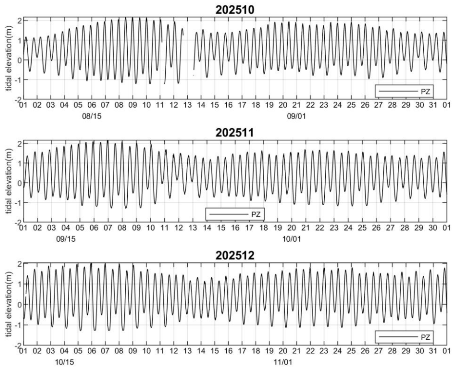
圖 2.13-2 PZ 測站 2025 年 10~12 月各月實測潮位逐時變化圖
