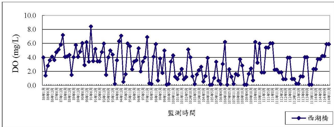
圖 3.1.7-2 陸域水質歷次溶氧比較分析圖
