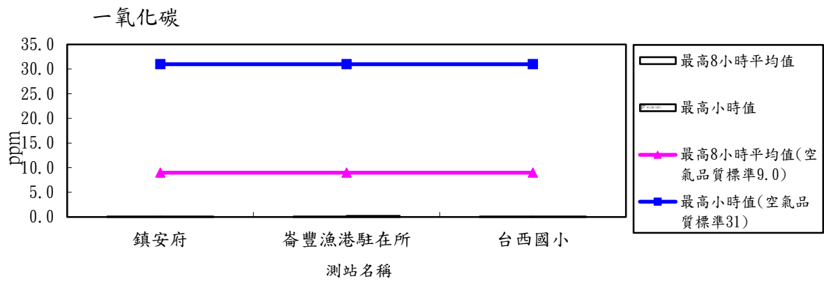
圖 2.1-1 114 年度第 4 季各測站一氧化碳(CO)最高 8 小時平均值及最高小時值比較分析圖
