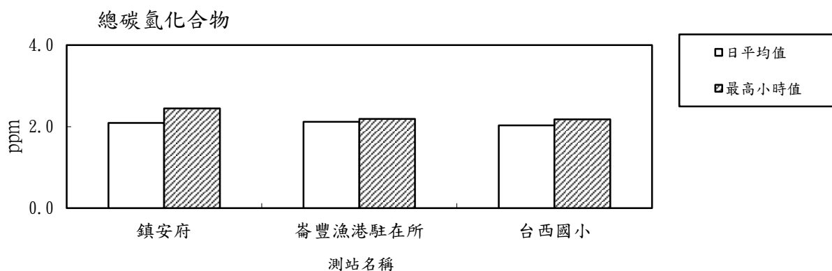
圖 2.1-6 114 年度第 4 季各測站總碳氫化合物(THC)日平均值及最高小時值比較分析圖
