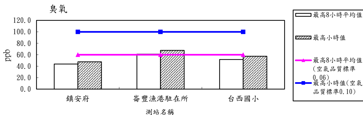
圖 2.1-5 114 年度第 4 季各測站臭氧(O 3 )最高 8 小時平均值及最高小時值比較分析圖
