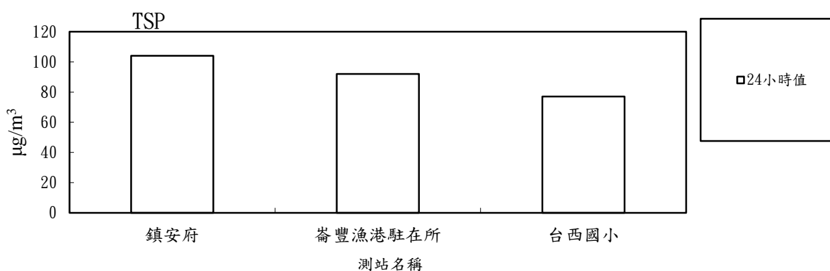
圖 2.1-8 114 年度第 4 季各測站 TSP 24 小時值比較分析圖
