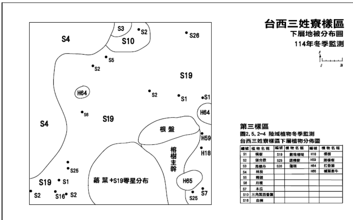
圖 2.5.2-4 陸域植物生態冬季監測台西三姓寮樣區下層植物分布圖
