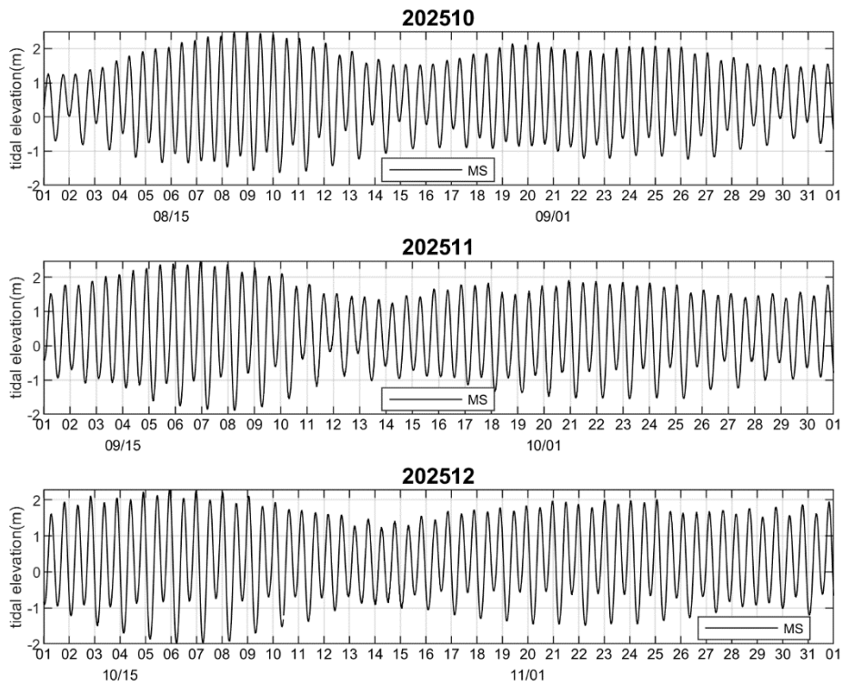
圖 2.13-1 MS 測站 2025 年 10~12 月各月實測潮位逐時變化圖
