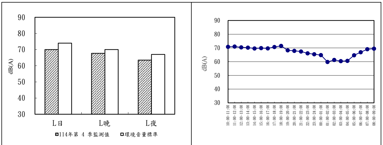
圖 2.2-2 海豐橋 114 年第四季噪音監測成果分析圖及逐時變化圖
