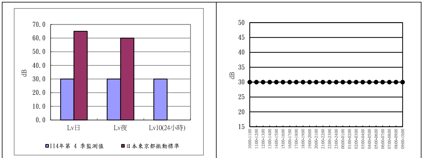
圖 2.3-5 五條港出入管制 114 年度第 4 季振動監測成果分析圖及逐時變化圖
