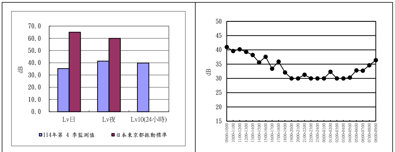
圖 2.3-2 海豐橋 114 年度第 4 季振動監測成果分析圖及逐時變化圖
