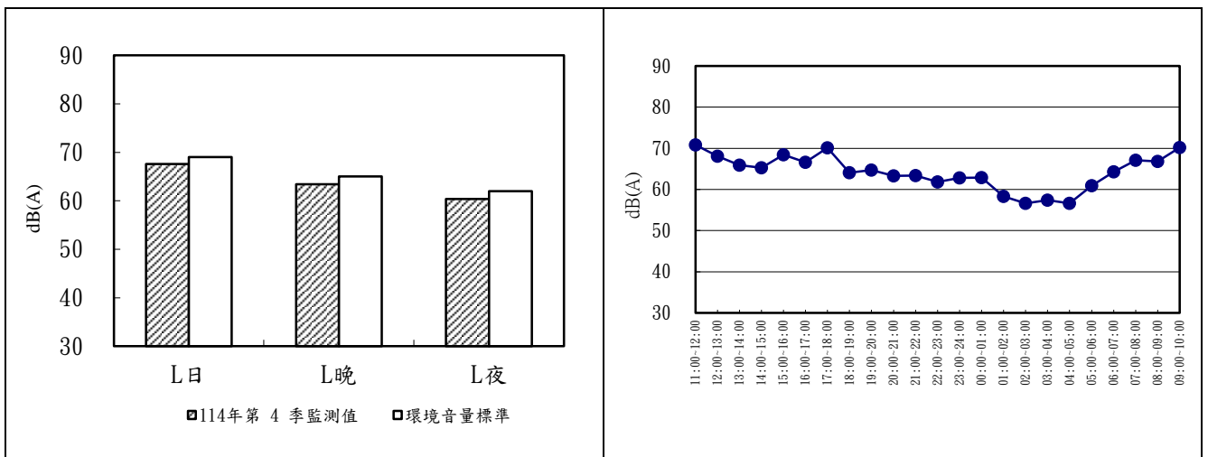
圖 2.2-3 崙豐國小 114 年第四季噪音監測成果分析圖及逐時變化圖
