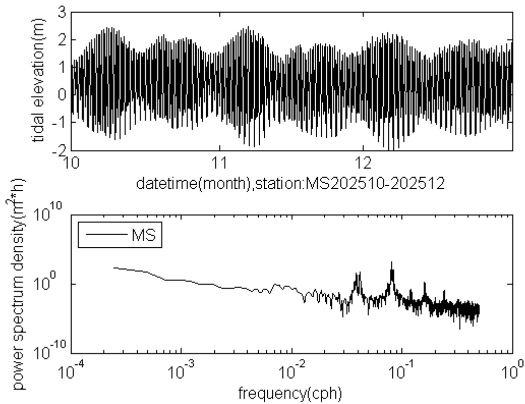
圖 2.13-3 MS 測站 2025 年 10~12 月實測潮位頻譜與逐時變化圖
