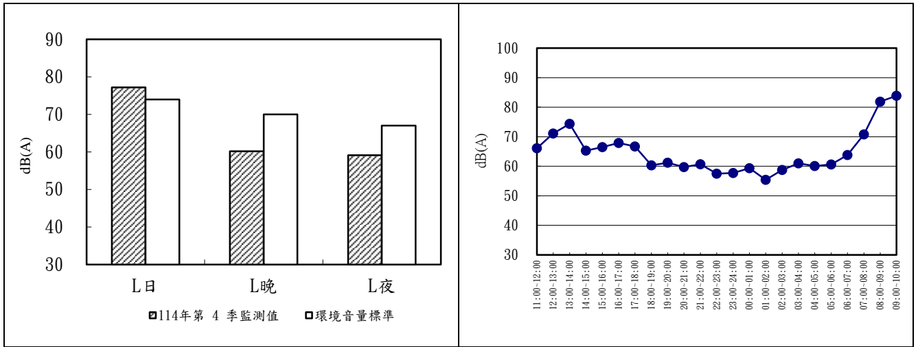
圖 2.2-1 安西府 114 年第四季噪音監測成果分析圖及逐時變化圖
