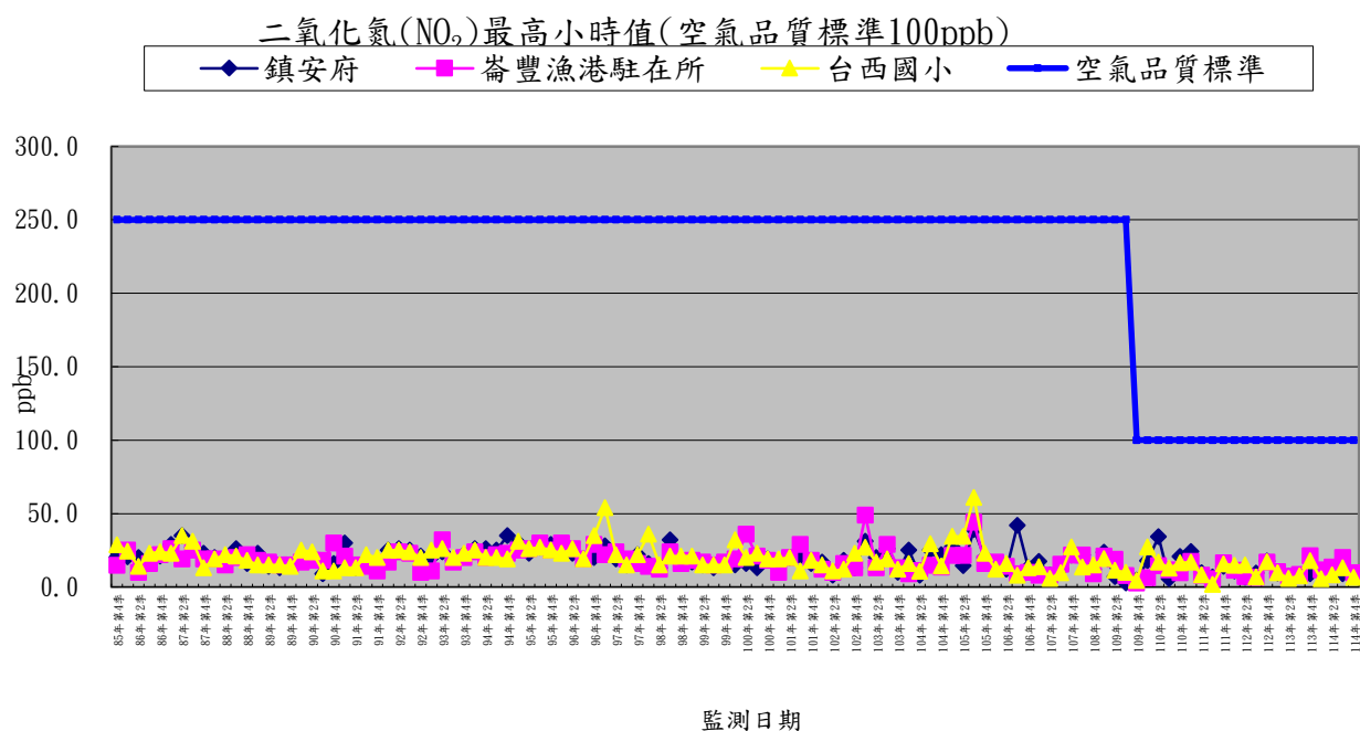
圖 3.1.1-3 本計畫歷次二氧化氮(NO 2 )最高小時值監測結果分析圖
