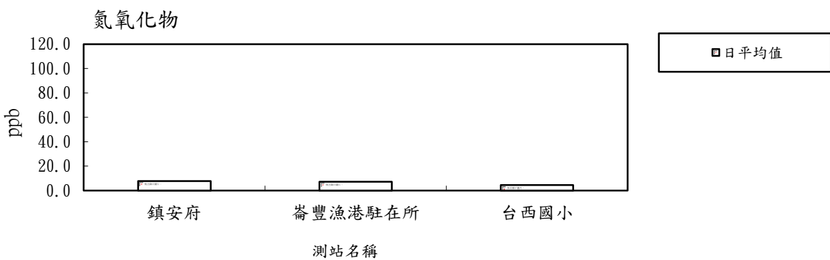
圖 2.1-3 114 年度第 4 季各測站氮氧化物(NO x )日平均值比較分析圖
