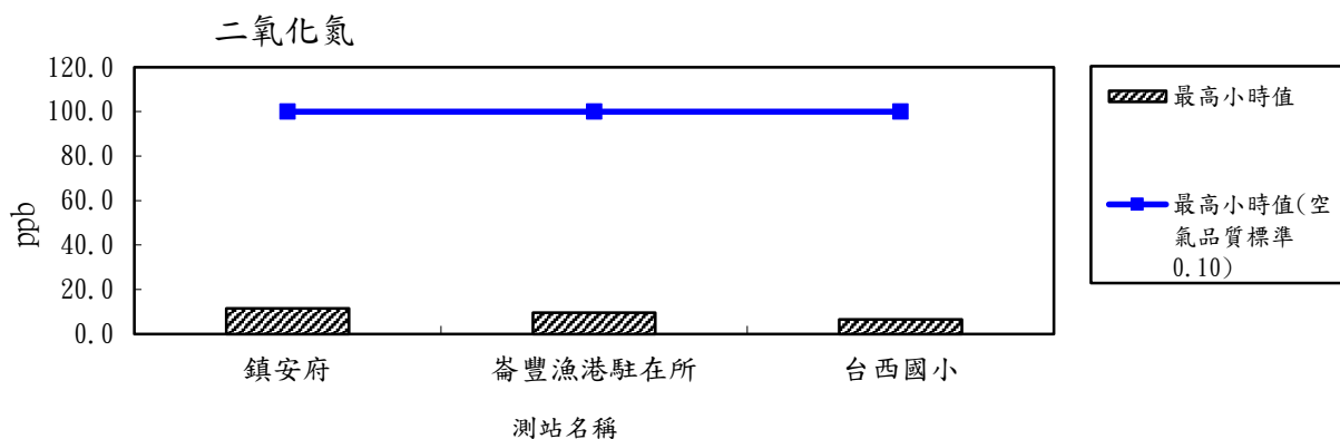
圖 2.1-4 114 年度第 4 季各測站二氧化氮(NO 2 )最高小時值比較分析圖
