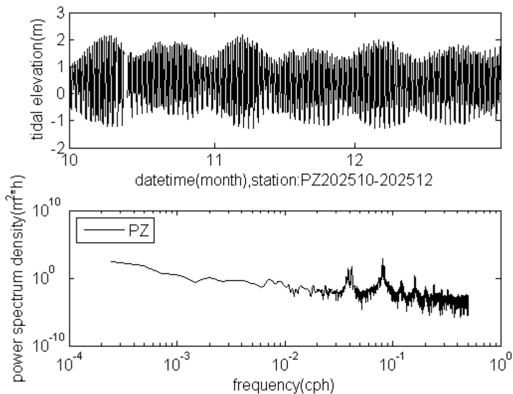
圖 2.13-4 PZ 測站 2025 年 10~12 月實測潮位頻譜與逐時變化圖
