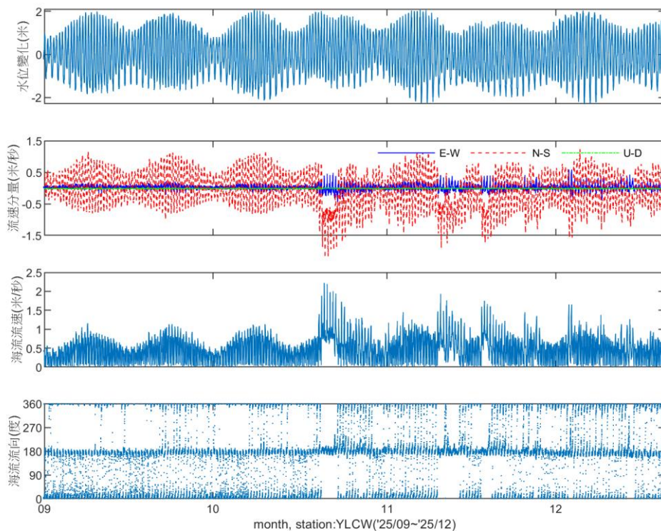
圖 2.13-10 YLCW 測站 2025 年 9 月~12 月海流分量與流速流向時序列
