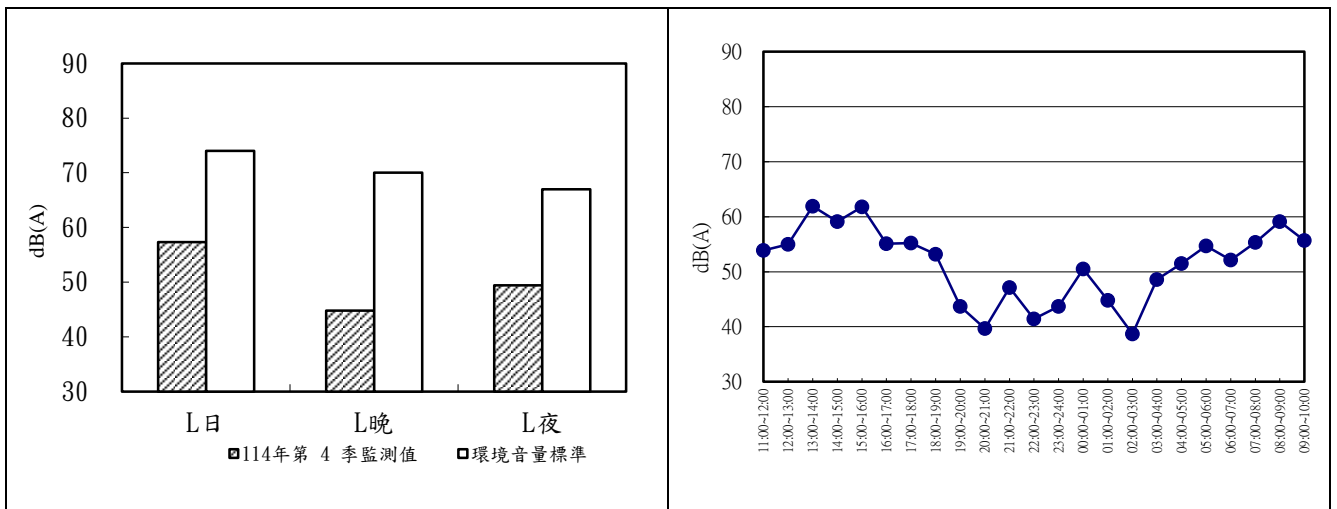
圖 2.2-5 五條港出入管制站 114 年第四季噪音監測成果分析圖及逐時變化圖
