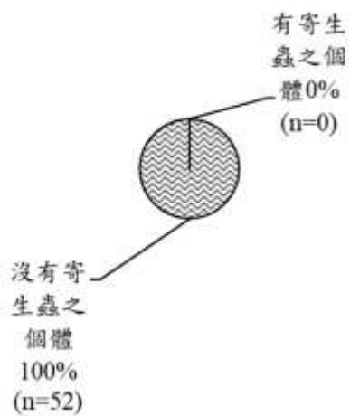
圖 III.6-24 本季螻蛄蝦被等足目寄生的百分率(n=52)。
