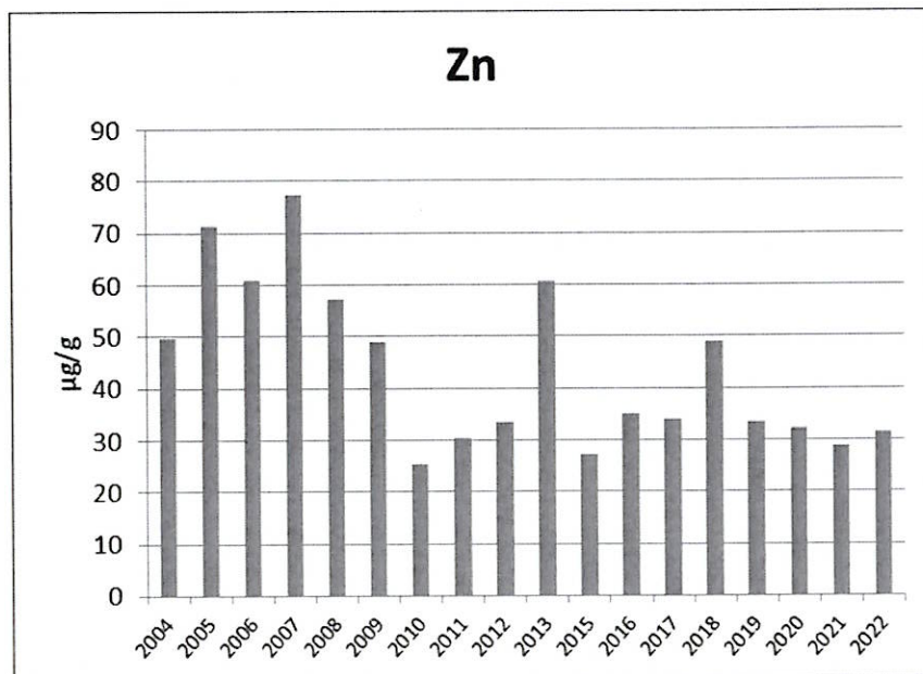
附錄 III.10-2 圖 12. 2004 至 2022 年 5 月漁舟蜆螺體內鋅含量之年度比較圖
