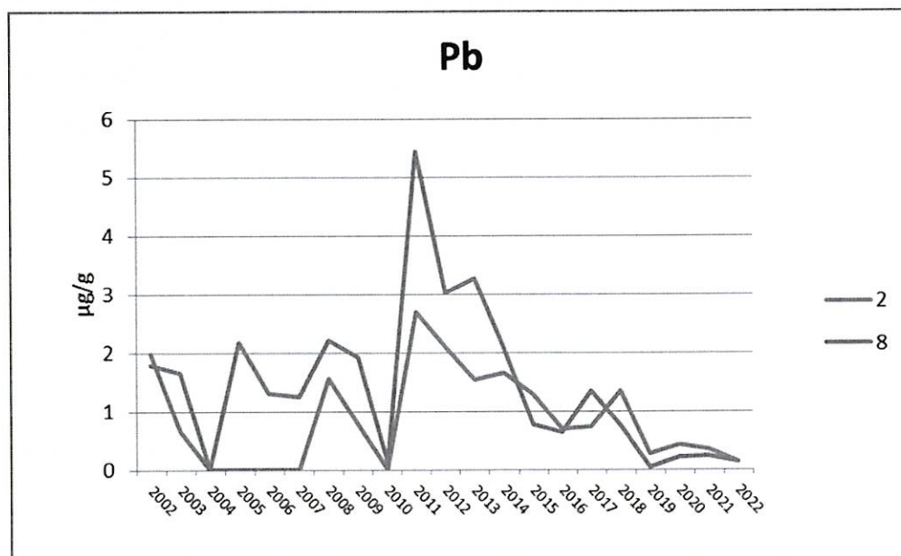
附錄 III.10-2 圖 14. 2002~2022 年 5 月測站 2 及 8 短指和尚蟹體內鉛含量之測站比較圖
