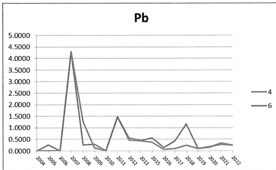
附錄 III.10-2 圖 18. 2004~2022 年 5 月測站 4 及 6 漁舟蜆螺體內鉛含量之測站比較圖
