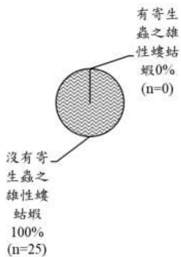
圖 III.6-26 本季雄性螻蛄蝦被等足目寄生的百分率(n=25)。
