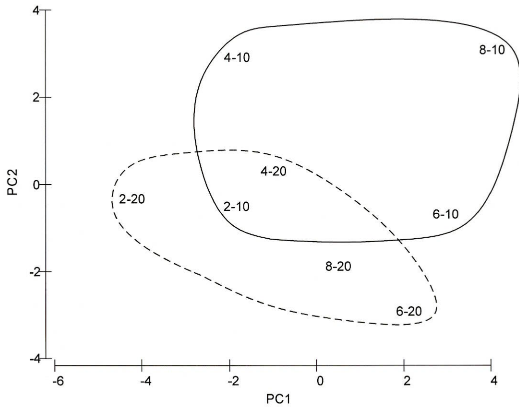
圖 3.10.2-3 民國 111 年 5 月彰濱工業區附近海域各測站浮游動物群聚分析圖(圖中第一個數字代表測站，第二個數字代表深度)
