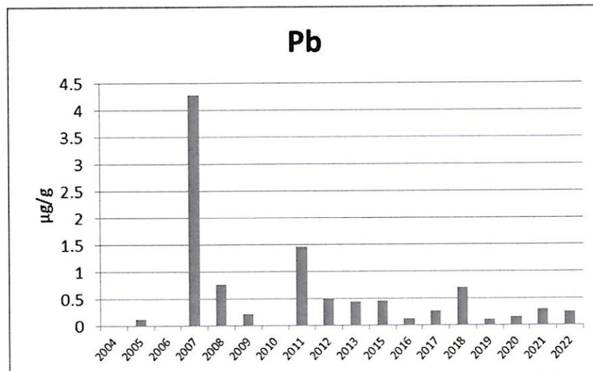
附錄 III.10-2 圖 10. 2004 至 2022 年 5 月漁舟蜆螺體內鉛含量之年度比較圖
