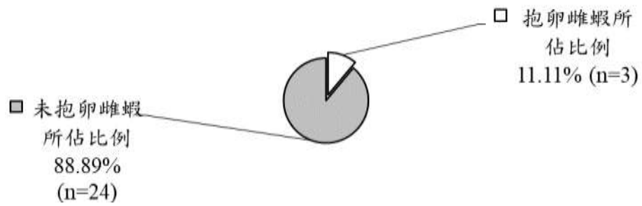
圖 III.6-20 本季伸港地區螻蛄蝦抱卵母蝦佔雌蝦之百分比(n=27)
