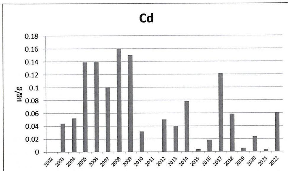
附錄 III.10-2 圖 7. 2002 至 2022 年 5 月短指和尚蟹體內鎘含量之年度比較圖
