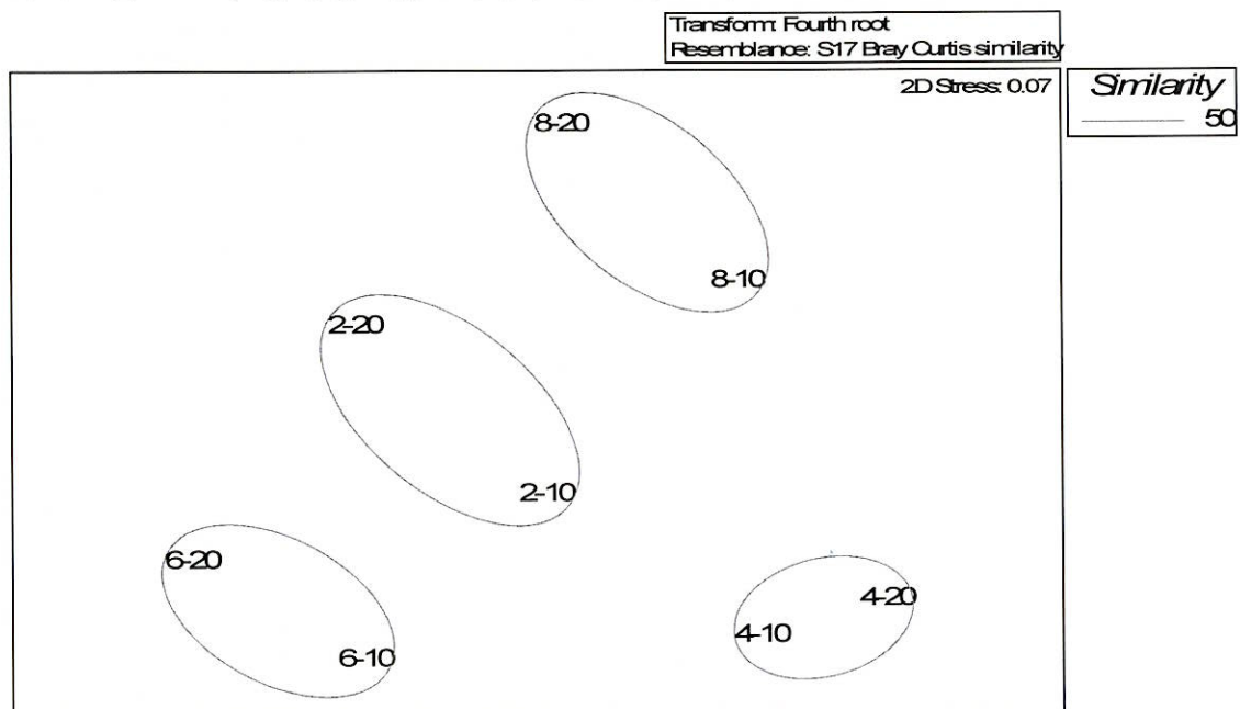
附錄III.10-1圖5 111年5月彰濱工業區附近海域亞潮帶各測站間底棲生物MDS分析圖
