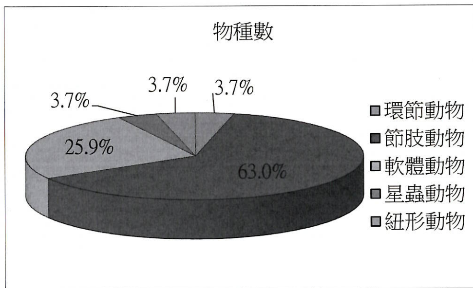
附錄III.10-1圖5 民國111年5月潮間帶各大類生物之物種數百分比
