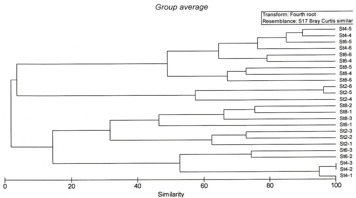
附錄III.10-2圖3 民國111年5月於彰濱工業區附近海域潮間帶各測站之群聚分析樹狀圖。
