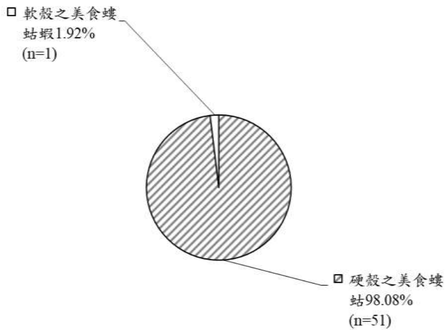
圖 III.6-15 本季螻蛄蝦之脫殼比例(n=52)
