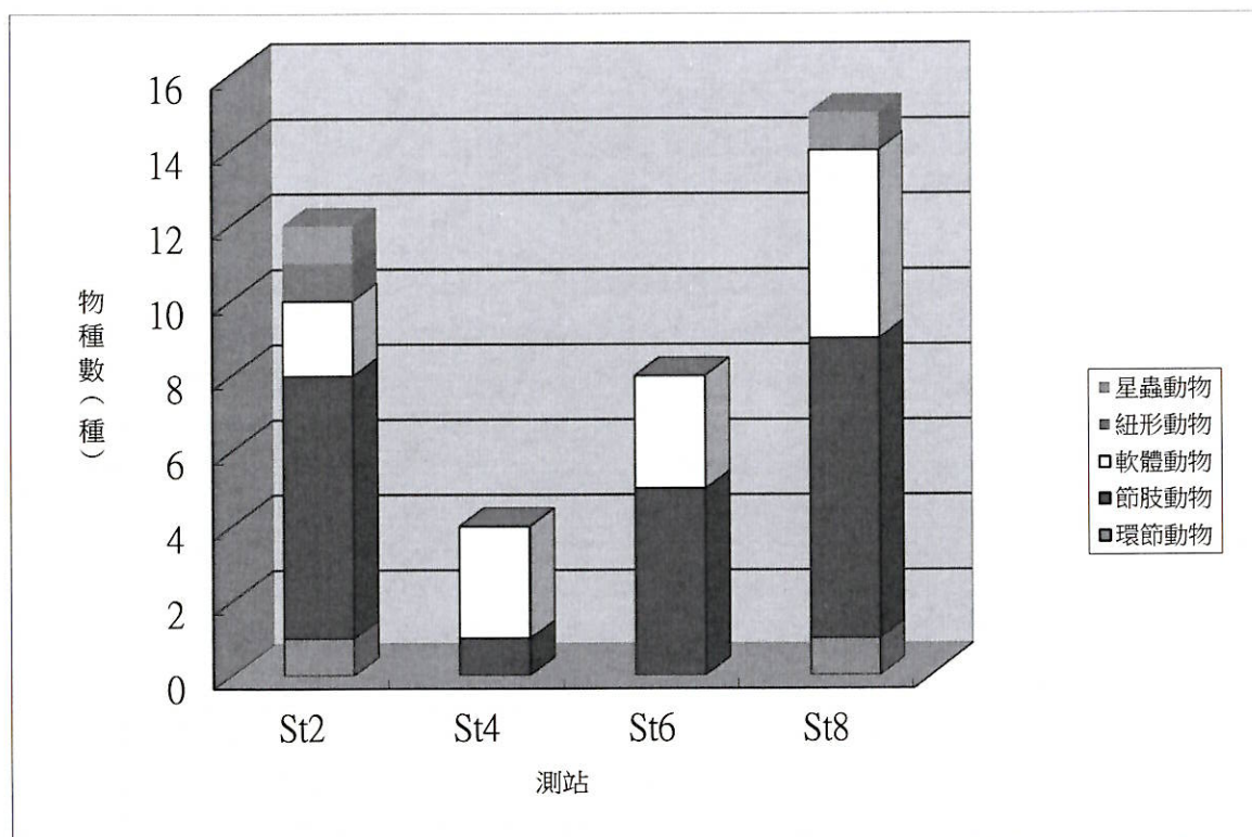
附錄III.10-1圖7 民國111年5月於彰濱工業區附近海域潮間帶各測站各大類生物之物種數比較圖
