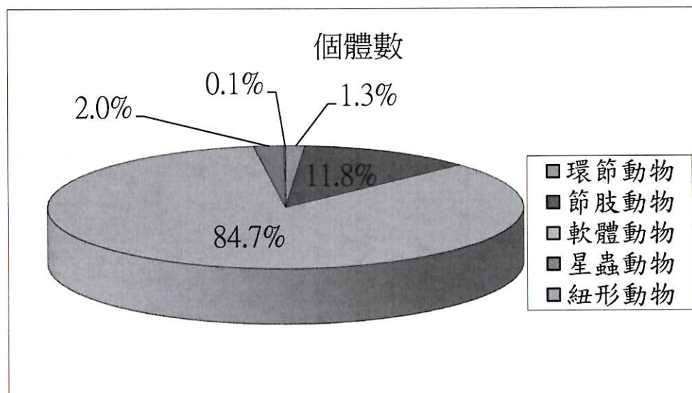
附錄III.10-1圖6 民國111年5月潮間帶各大類生物之個體數百分比
