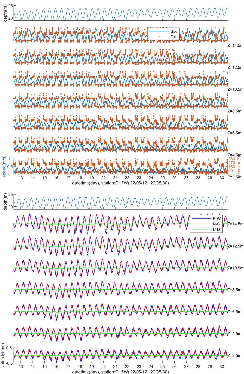
附錄III.11圖-1 CH7W流速、流向、南北向、東西向速度分量逐時變化圖
