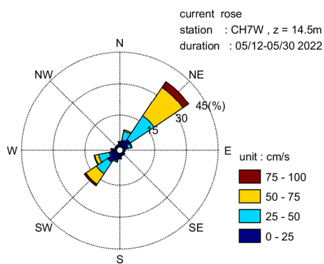
附錄III.11圖-5 CH7W流速流向玫瑰圖
