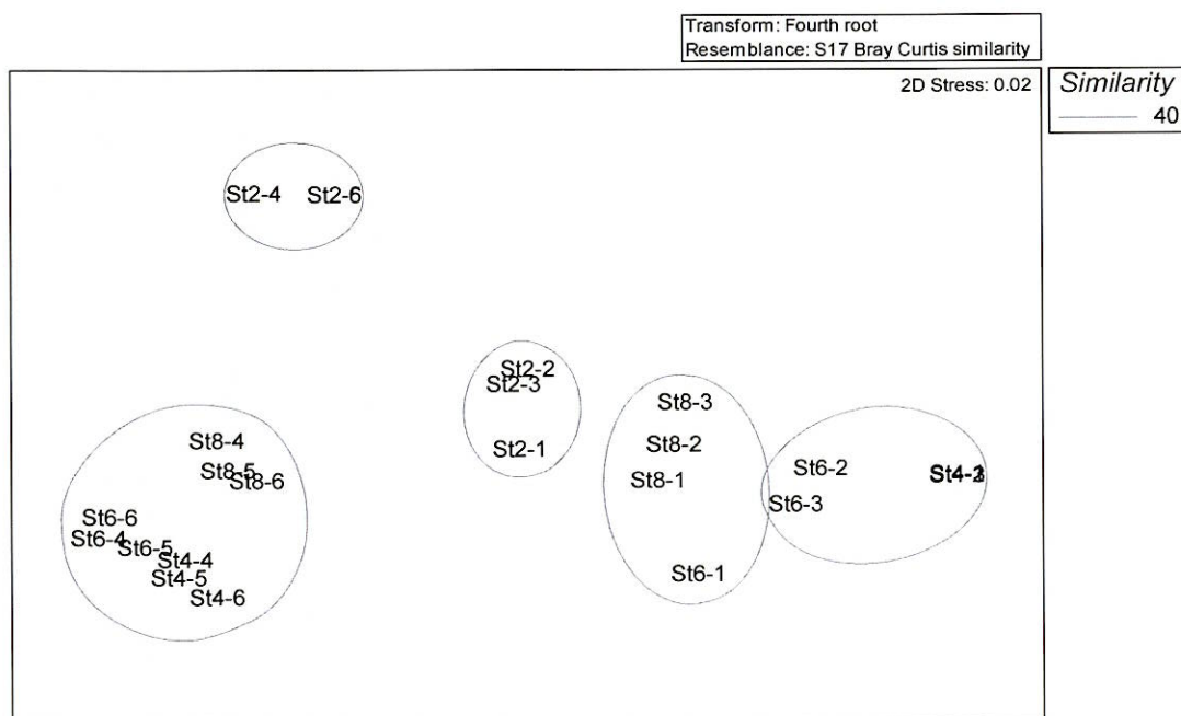
附錄III.10-2圖4 民國111年5月於彰濱工業區附近海域潮間帶各測站之群聚MDS圖。
