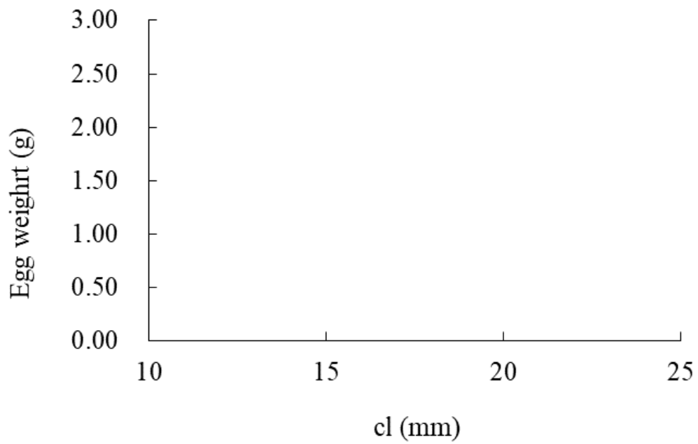
圖 III.6-23 本季螞蛄蝦抱卵母蝦(限未發眼卵)頭胸甲長(cl)與抱卵重(濕重)之關係
