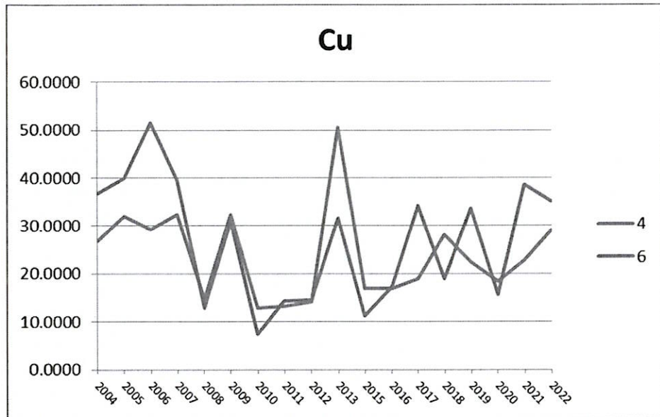
附錄 III.10-2 圖 17. 2004~2022 年 5 月測站 4 及 6 漁舟蜆螺體內銅含量之測站比較圖
