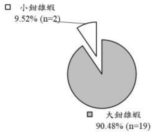
圖 III.6-14 本季螻蛄大小鉗雄蝦各佔之比例(n=21)
