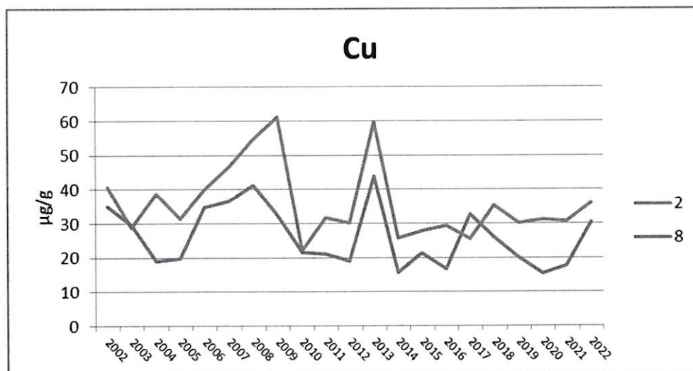
附錄 III.10-2 圖 13. 2002~2022 年 5 月測站 2 及 8 短指和尚蟹體內銅含量之測站比較圖
