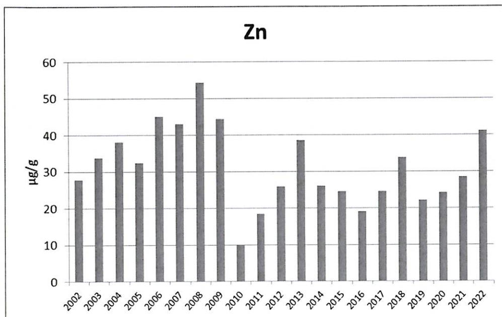
附錄 III.10-2 圖 8. 2002 至 2022 年 5 月短指和尚蟹體內鋅含量之年度比較圖
