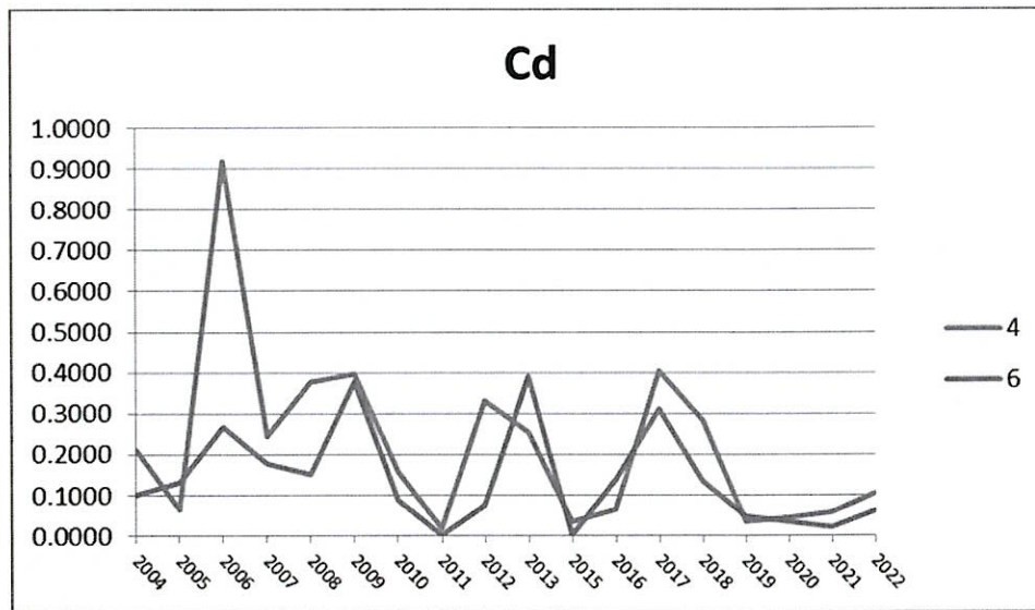
附錄 III.10-2 圖 19. 2004~2022 年 5 月測站 4 及 6 漁舟蜆螺體內鎘含量之測站比較圖
