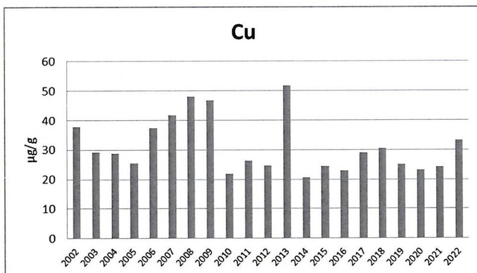
附錄 III.10-2 圖 5. 2002 至 2022 年 5 月短指和尚蟹體內銅含量之年度比較圖
