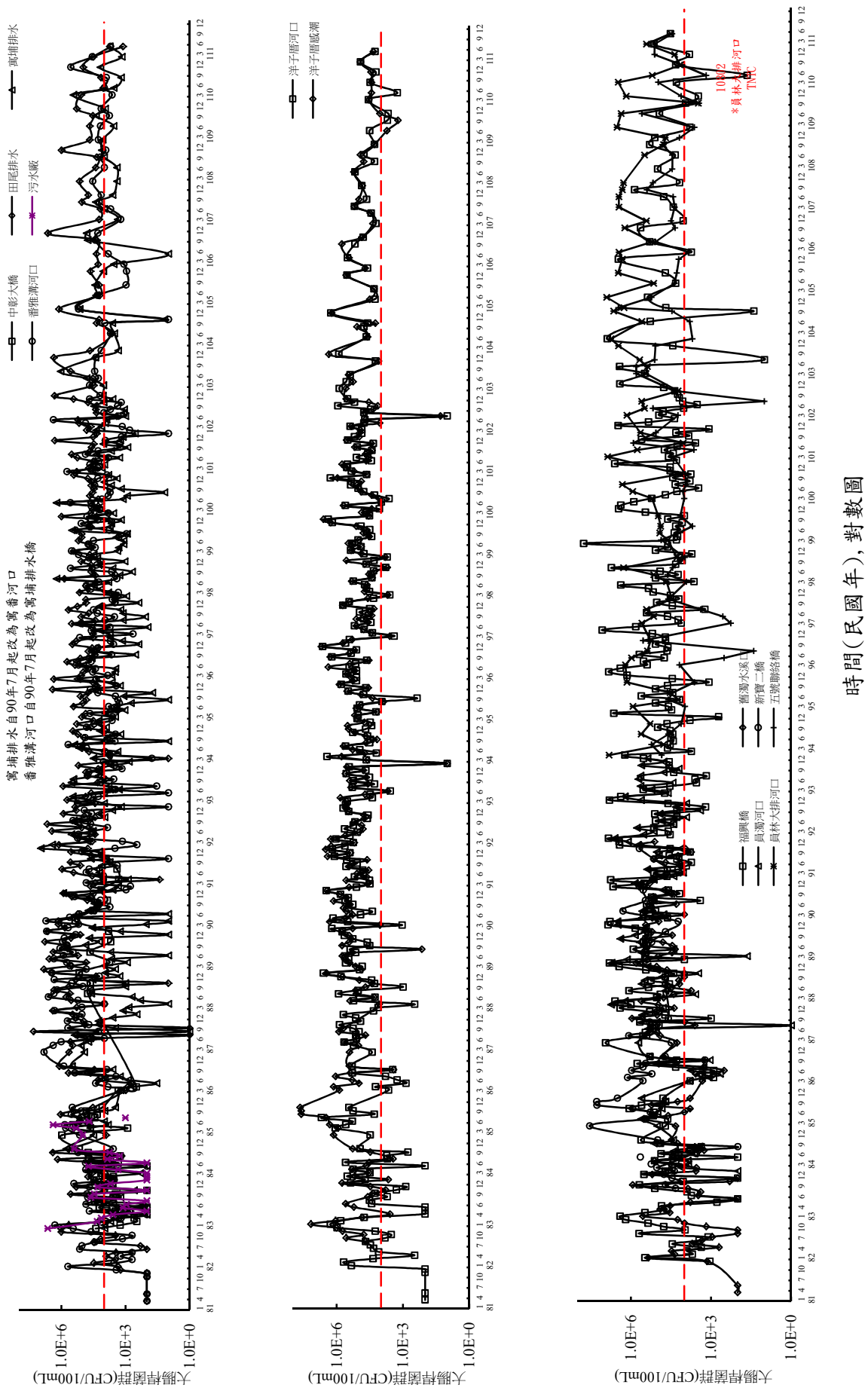
附圖III.7-10(b) 歷次彰濱河口退潮大腸桿菌群調查結果
