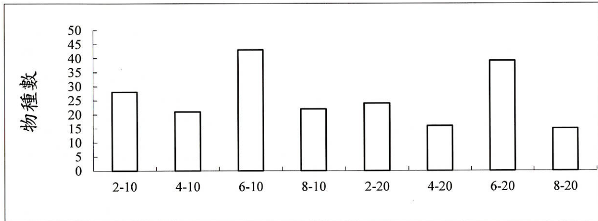
附錄III.10-1圖1 111年5月彰濱工業區附近海域亞潮帶各測站底棲生物物種數之比較
