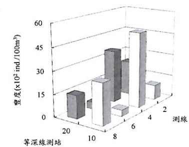
圖 2.10.2-2 民國 111 年 5 月彰化濱海工業區附近海域浮游動物主要優勢類群之豐度分布圖
