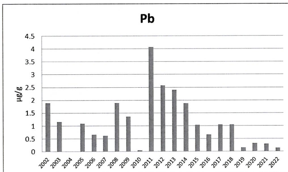
附錄 III.10-2 圖 6. 2002 至 2022 年 5 月短指和尚蟹體內鉛含量之年度比較圖
