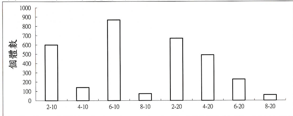
附錄III.10-1圖2 111年5月彰濱工業區附近海域亞潮帶各測站底棲生物個體數之比較
