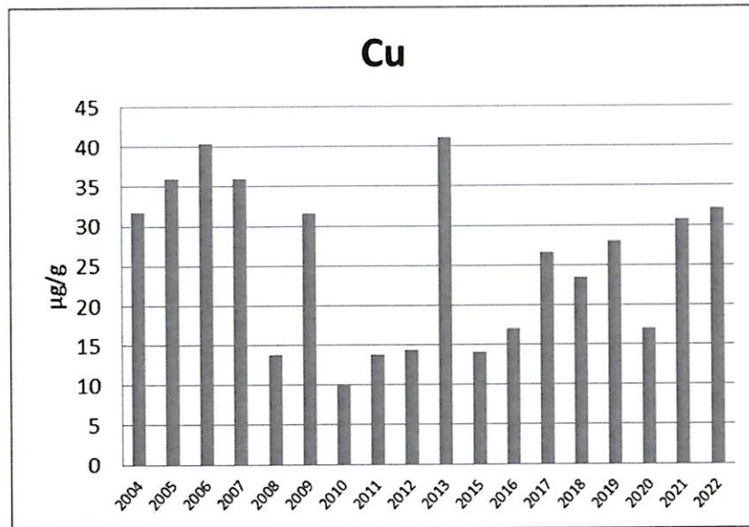
附錄 III.10-2 圖 9. 2004 至 2022 年 5 月漁舟蜆螺體內銅含量之年度比較圖
