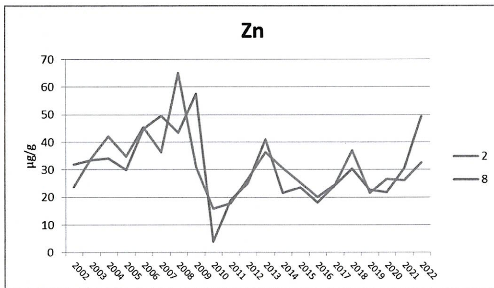
附錄 III.10-2 圖 16. 2002~2022 年 5 月測站 2 及 8 短指和尚蟹體內鋅含量之測站比較圖
