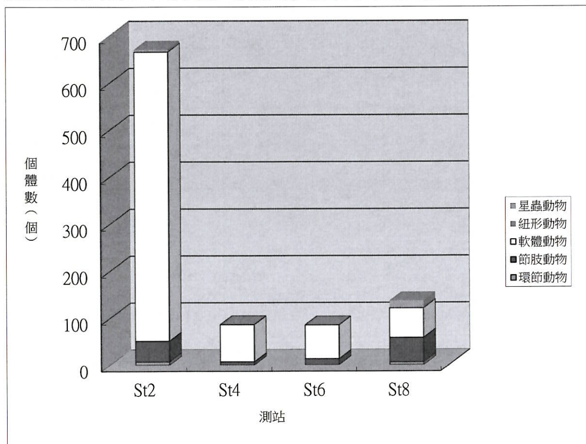
附錄III.10-1圖8 民國111年5月於彰濱工業區附近海域潮間帶各測站各大類生物之個體數比較圖
