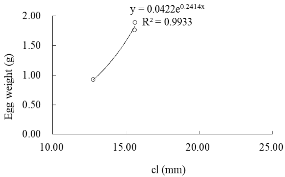
圖 III.6-22 本季螞蛄蝦抱卵母蝦(限發眼卵)頭胸甲長(cl)與抱卵重(濕重)之關係
