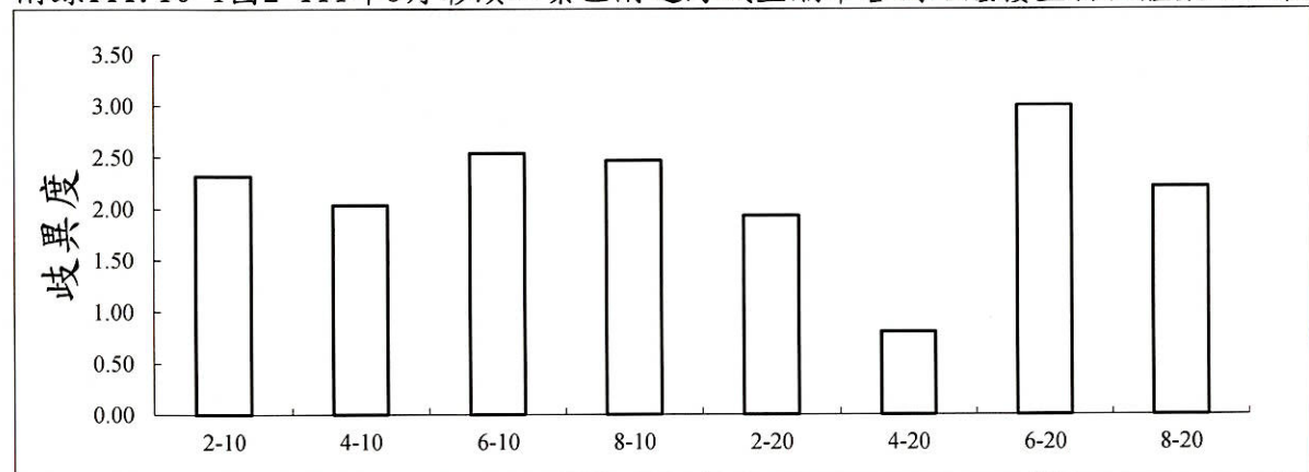
附錄III.10-1圖3 111年5月彰濱工業區附近海域亞潮帶各測站底棲生物歧異度之比較
