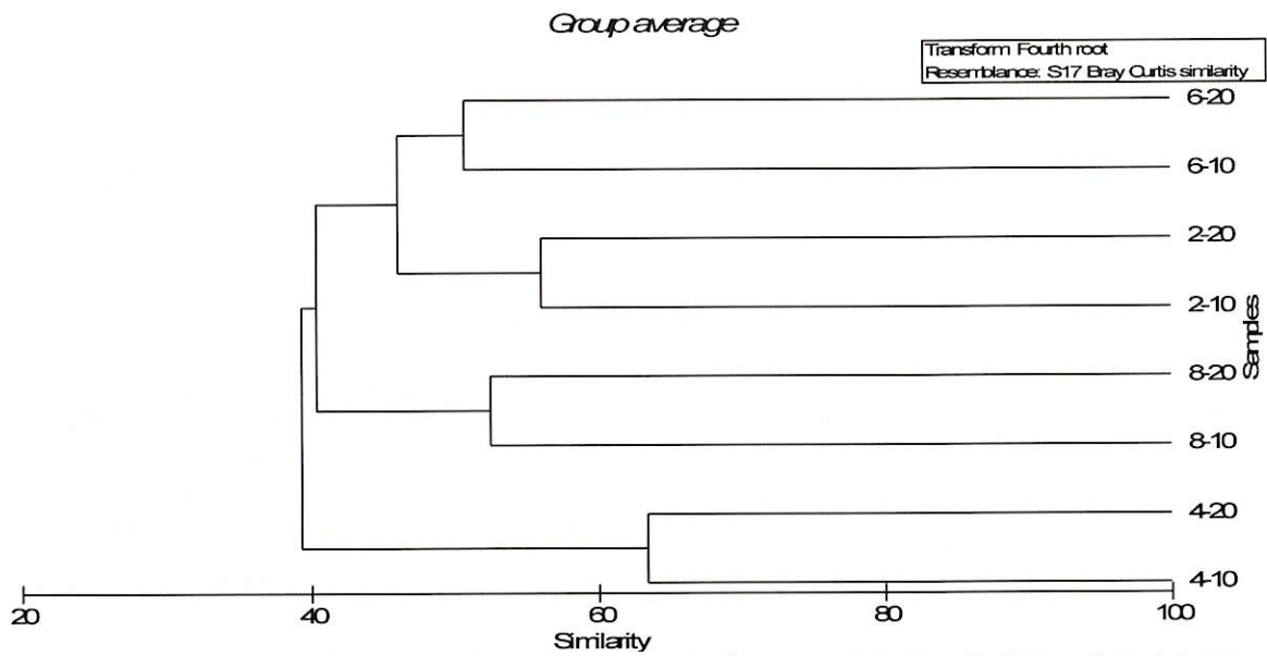
附錄III.10-1圖4 111年5月彰濱工業區附近海域亞潮帶各測站間底棲生物群聚之聚類分析圖
