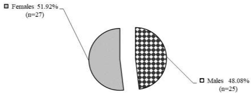
圖 III.6-17 本季伸港地區雌、雄螯蛄蝦之比例(n=52)
