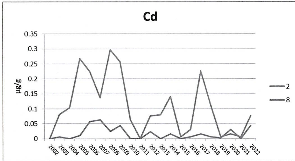
附錄 III.10-2 圖 15. 2002~2022 年 5 月測站 2 及 8 短指和尚蟹體內鎘含量之測站比較圖
