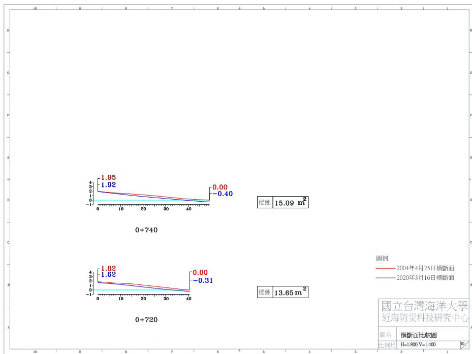
圖 4-4(a) 2020 年 3 月 16 日 A 監測區橫斷面比較圖
