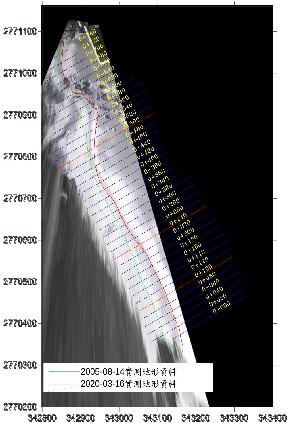
圖 4-22 實測地形水位線分析結果圖(2020/03/16)
