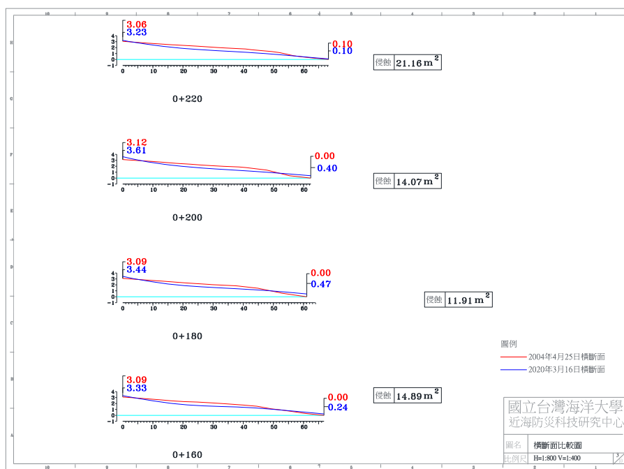
圖 4-4(h) 2020 年 3 月 16 日 A 監測區橫断面比較圖
