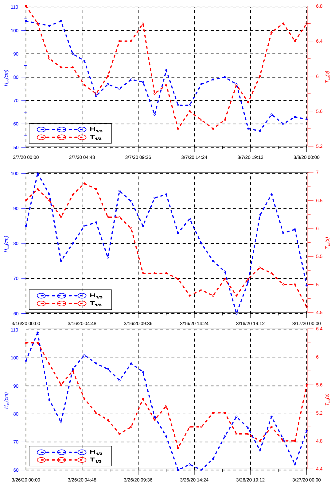
圖 2-3 波浪時序列變化圖
