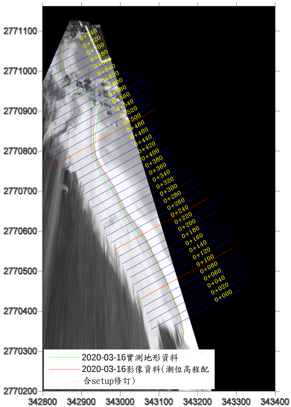
圖 3-22 水位線分析結果圖(2020/3/16)
