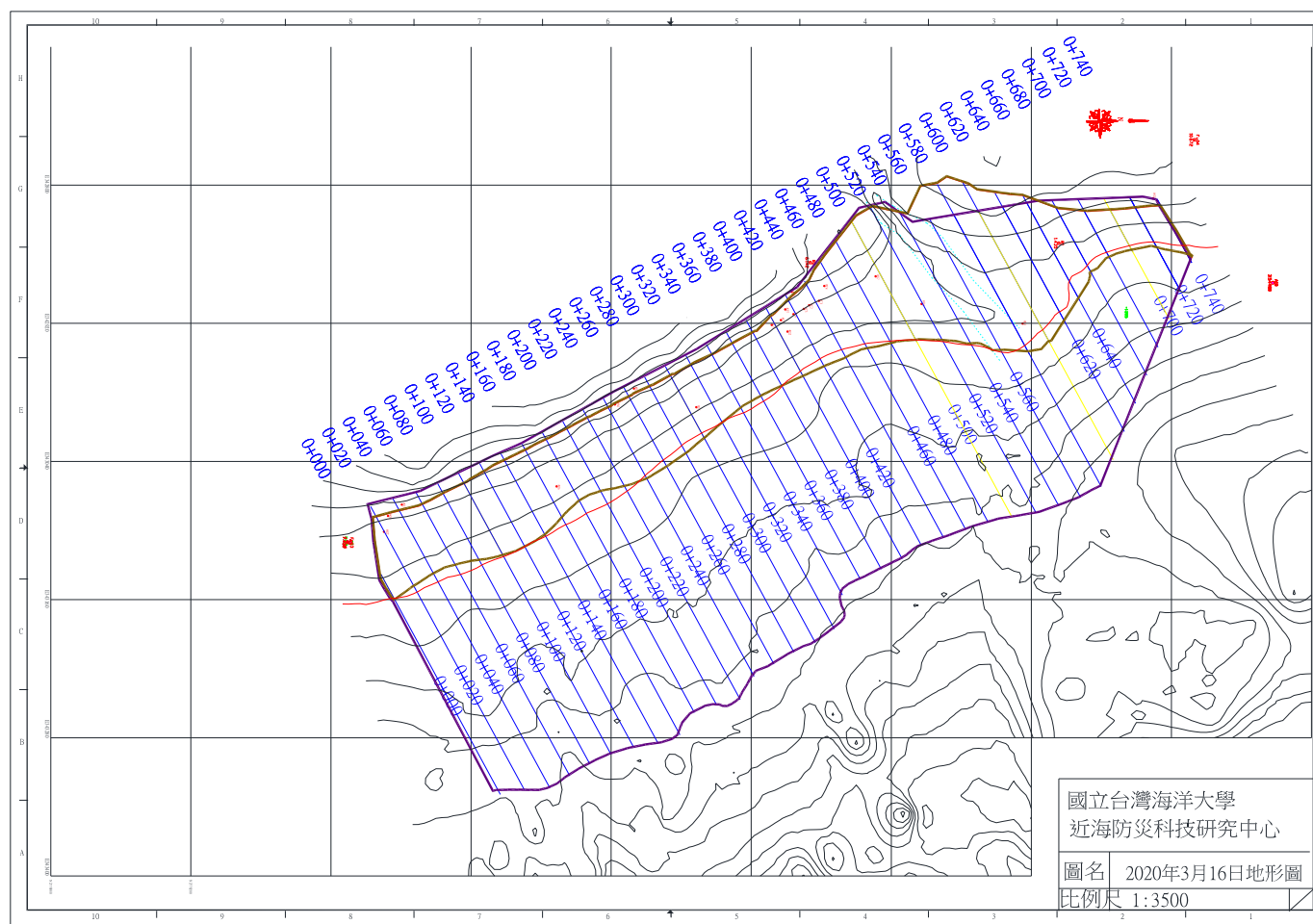
圖 4-1 2020 年 3 月 16 日監測地形圖
