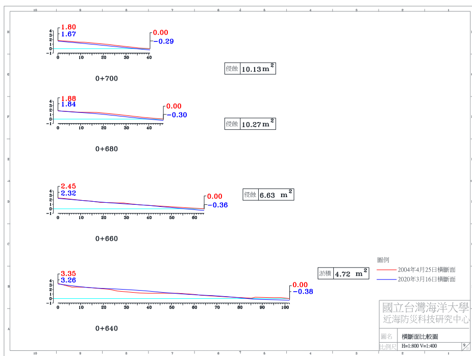
圖 4-4(b) 2020 年 3 月 16 日 A 監測區橫斷面比較圖
