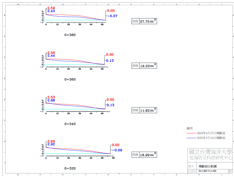
圖 4-4(f) 2020 年 3 月 16 日 A 監測區橫斷面比較圖
