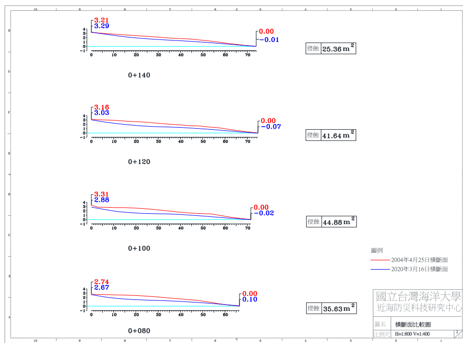
圖 4-4(i) 2020 年 3 月 16 日 A 監測區橫斷面比較圖
