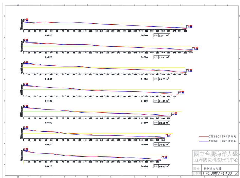
圖 4-5(c) 2020 年 3 月 16 日 B 監測區橫斷面比較圖
