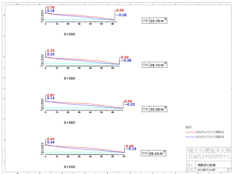
圖 4-4(g) 2020 年 3 月 16 日 A 監測區橫断面比較圖
