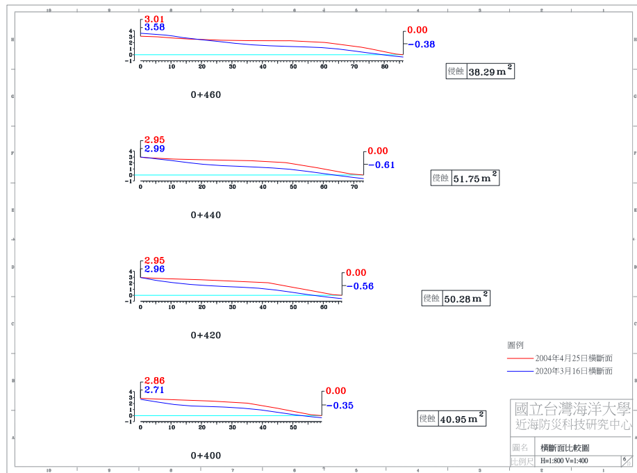
圖 4-4(e) 2020 年 3 月 16 日 A 監測區橫斷面比較圖
