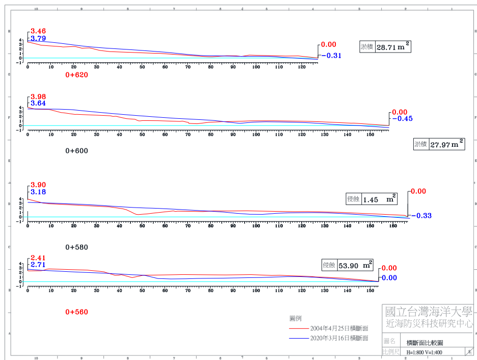
圖 4-4(c) 2020 年 3 月 16 日 A 監測區橫斷面比較圖
