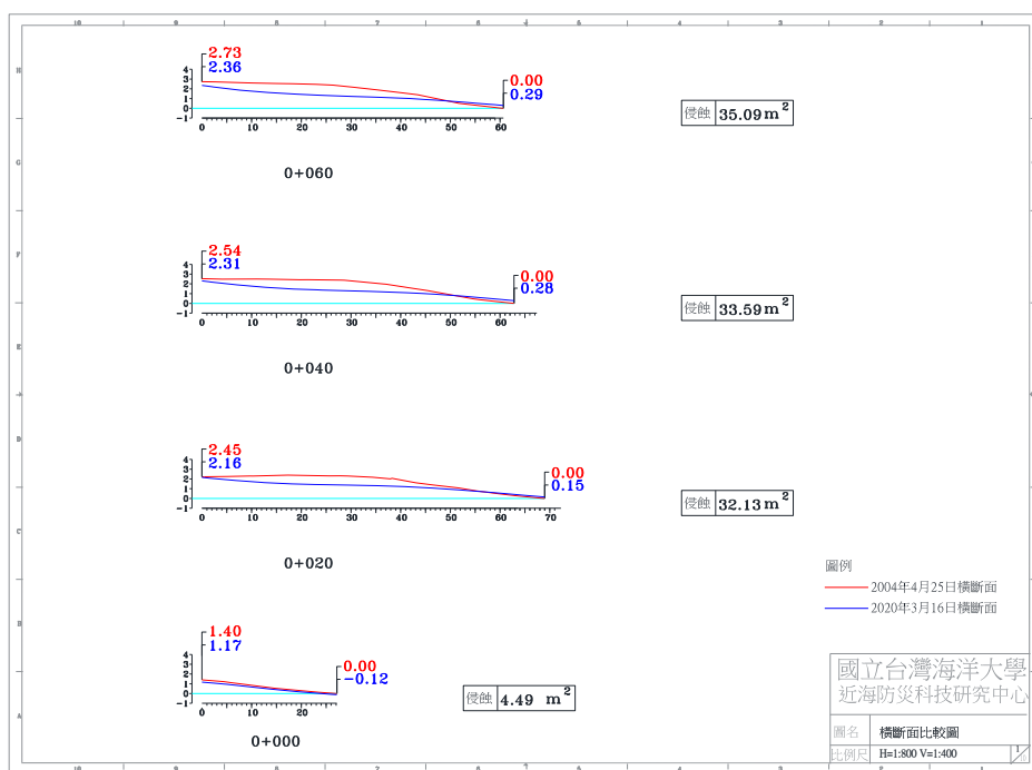
圖 4-4(j) 2020 年 3 月 16 日 A 監測區橫斷面比較圖
