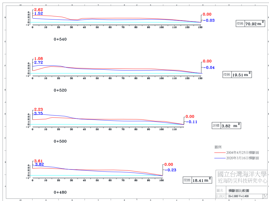
圖 4-4(d) 2020 年 3 月 16 日 A 監測區橫斷面比較圖
