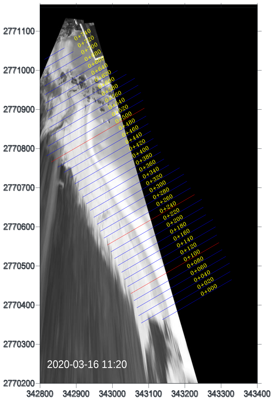
圖 4-19 鹽寮海岸地形影像全景圖(2020/03/16 11:20)
