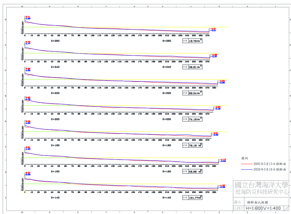
圖 4-5(e) 2020 年 3 月 16 日 B 監測區橫断面比較圖
