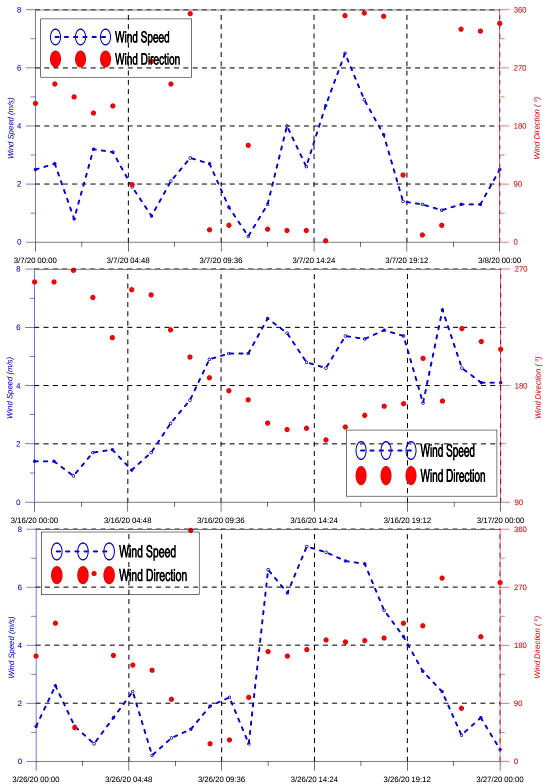
圖 2-2 風速風向時序列變化圖
