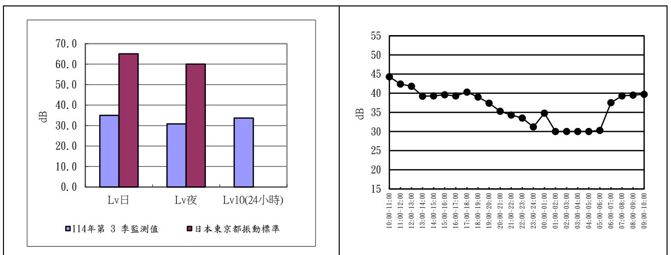
圖 2.3-3 崙豐國小 114 年度第 3 季振動監測成果分析圖及逐時變化圖
