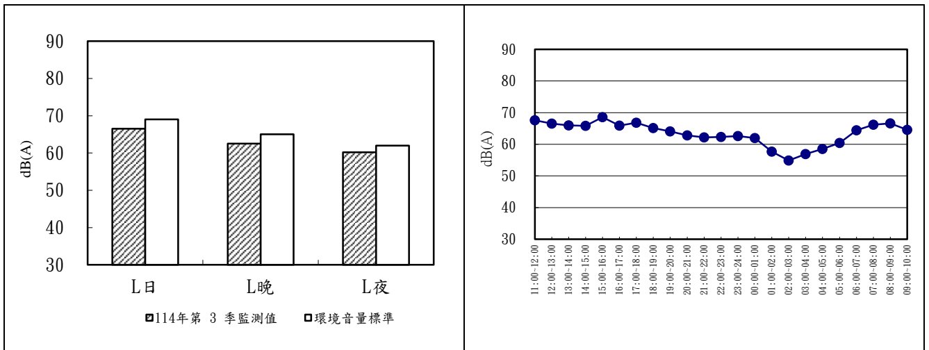
圖 2.2-3 崙豐國小 114 年第 3 季噪音監測成果分析圖及逐時變化圖
