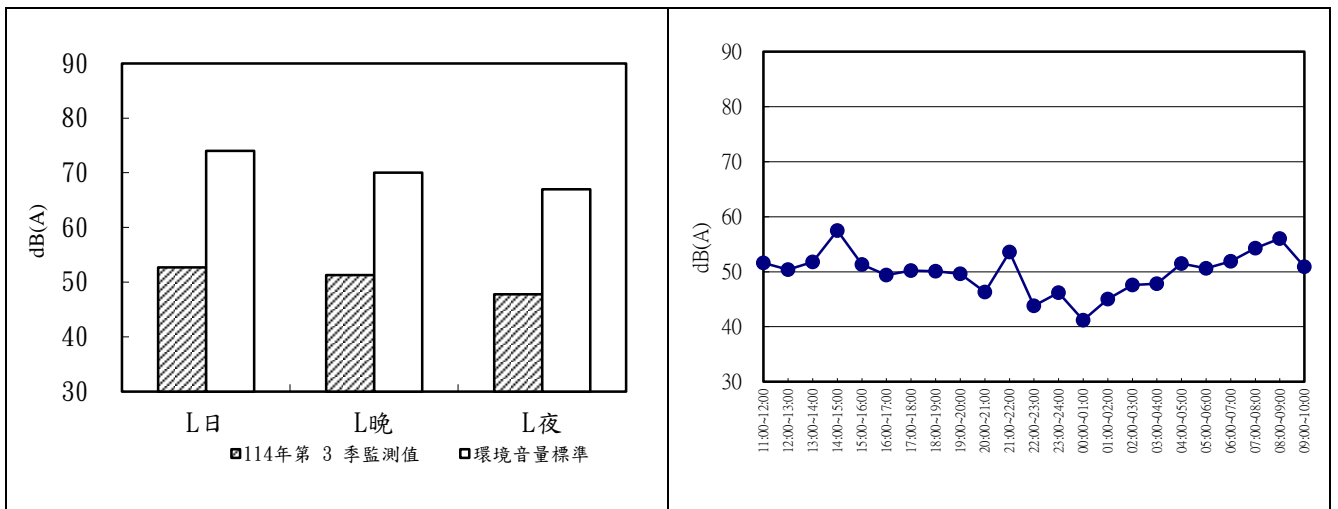
圖 2.2-5 五條港出入管制站 114 年第 3 季噪音監測成果分析圖及逐時變化圖
