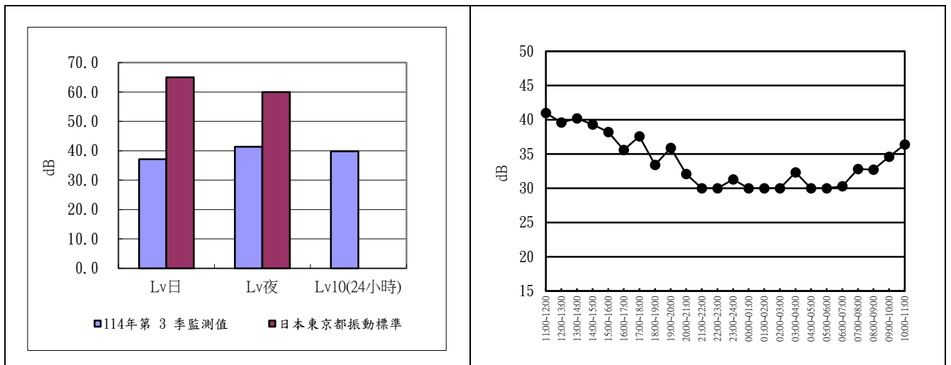
圖 2.3-2 海豐橋 114 年度第 3 季振動監測成果分析圖及逐時變化圖
