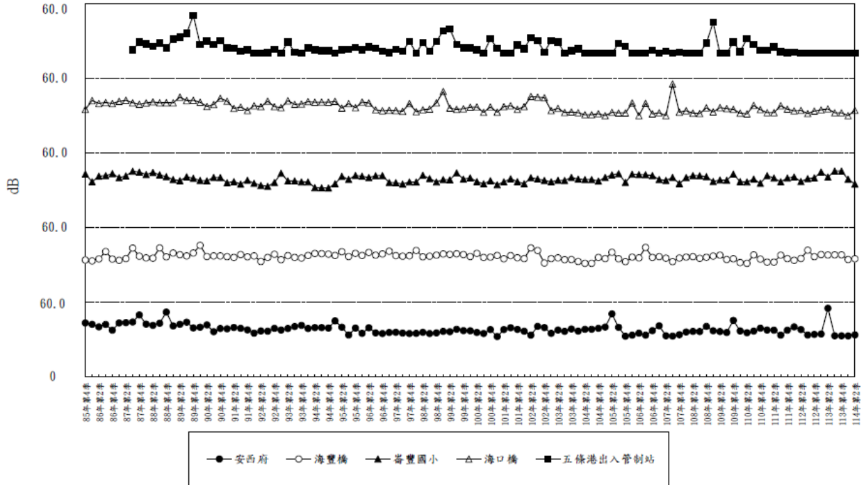
圖 3.1.3-1 本計畫歷次振動 L_{v10} 日 監測結果分析圖
