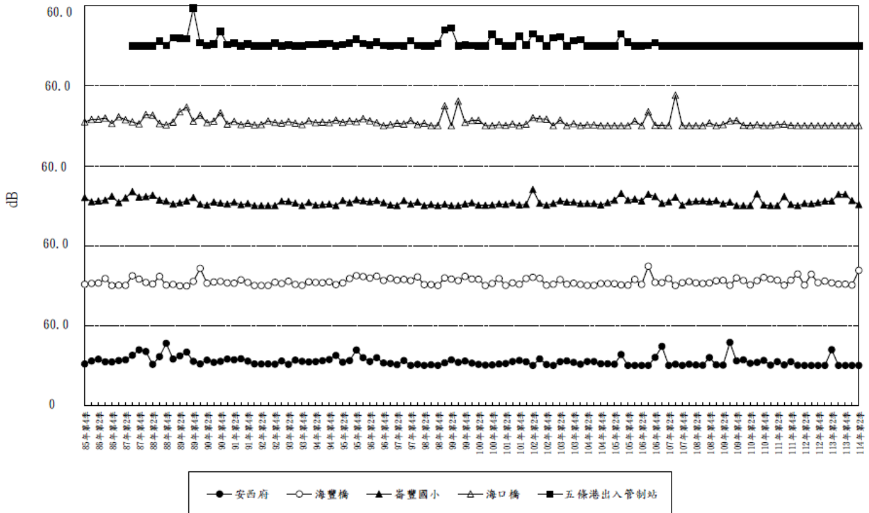
圖 3.1.3-2 本計畫歷次振動 L_{v10} 夜 監測結果分析圖
