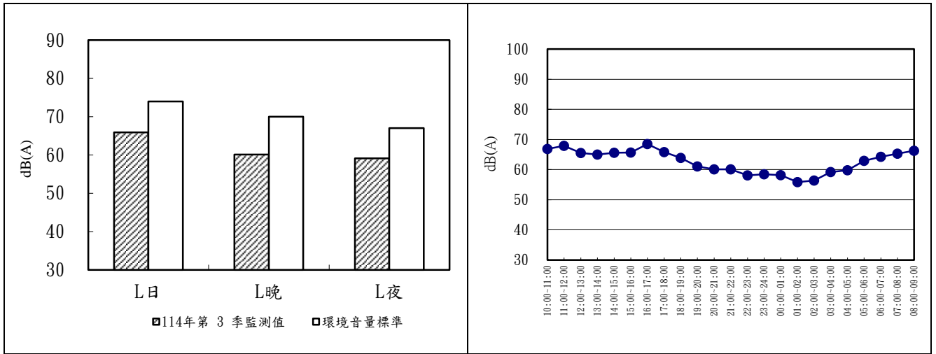
圖 2.2-1 安西府 114 年第 3 季噪音監測成果分析圖及逐時變化圖
