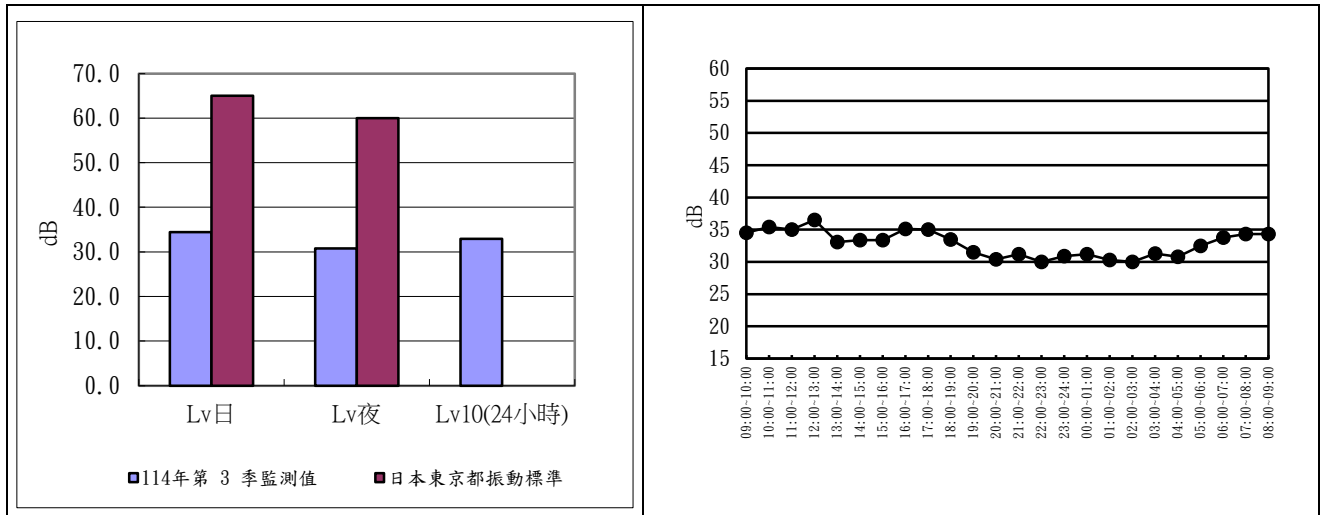
圖 2.3-1 安西府 114 年度第 3 季振動監測成果分析圖及逐時變化圖
