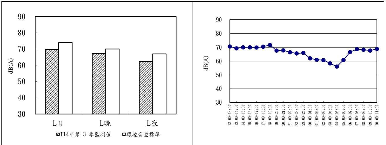
圖 2.2-2 海豐橋 114 年第 3 季噪音監測成果分析圖及逐時變化圖
