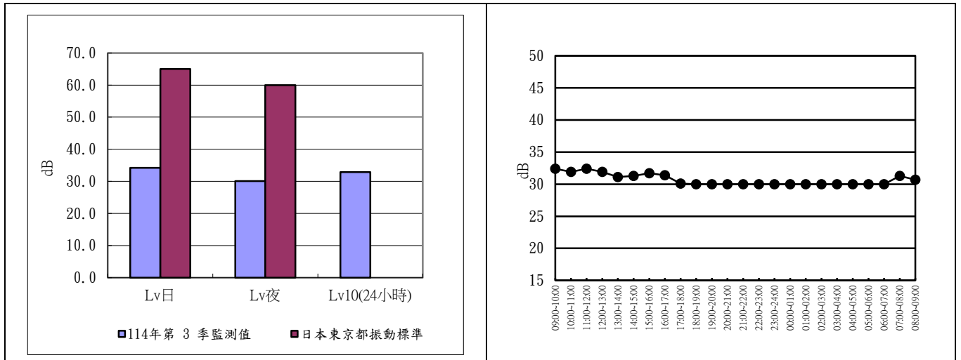
圖 2.3-4 海口橋 114 年度第 3 季振動監測成果分析圖及逐時變化圖
