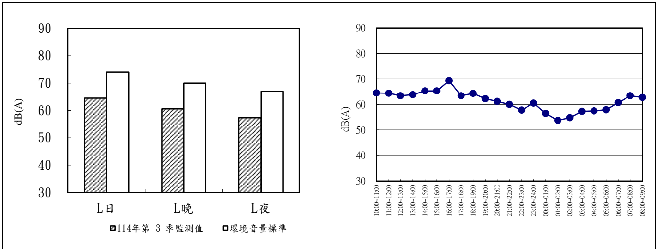
圖 2.2-4 海口橋 114 年第 3 季噪音監測成果分析圖及逐時變化圖
