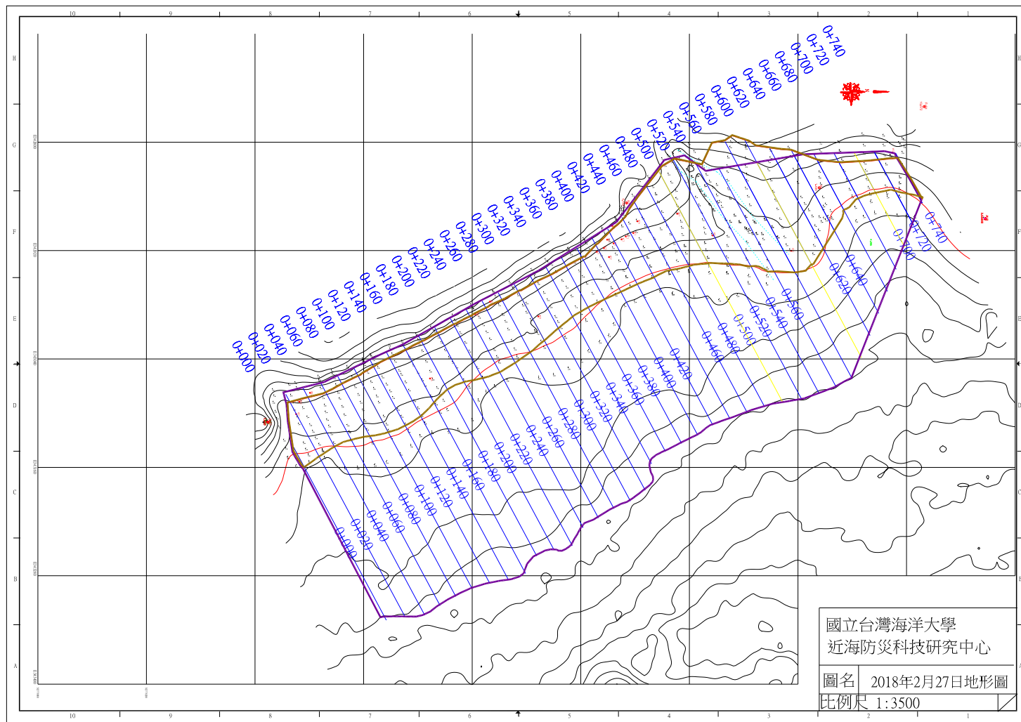
圖 4-1 2018 年 2 月 27 日監測地形圖
