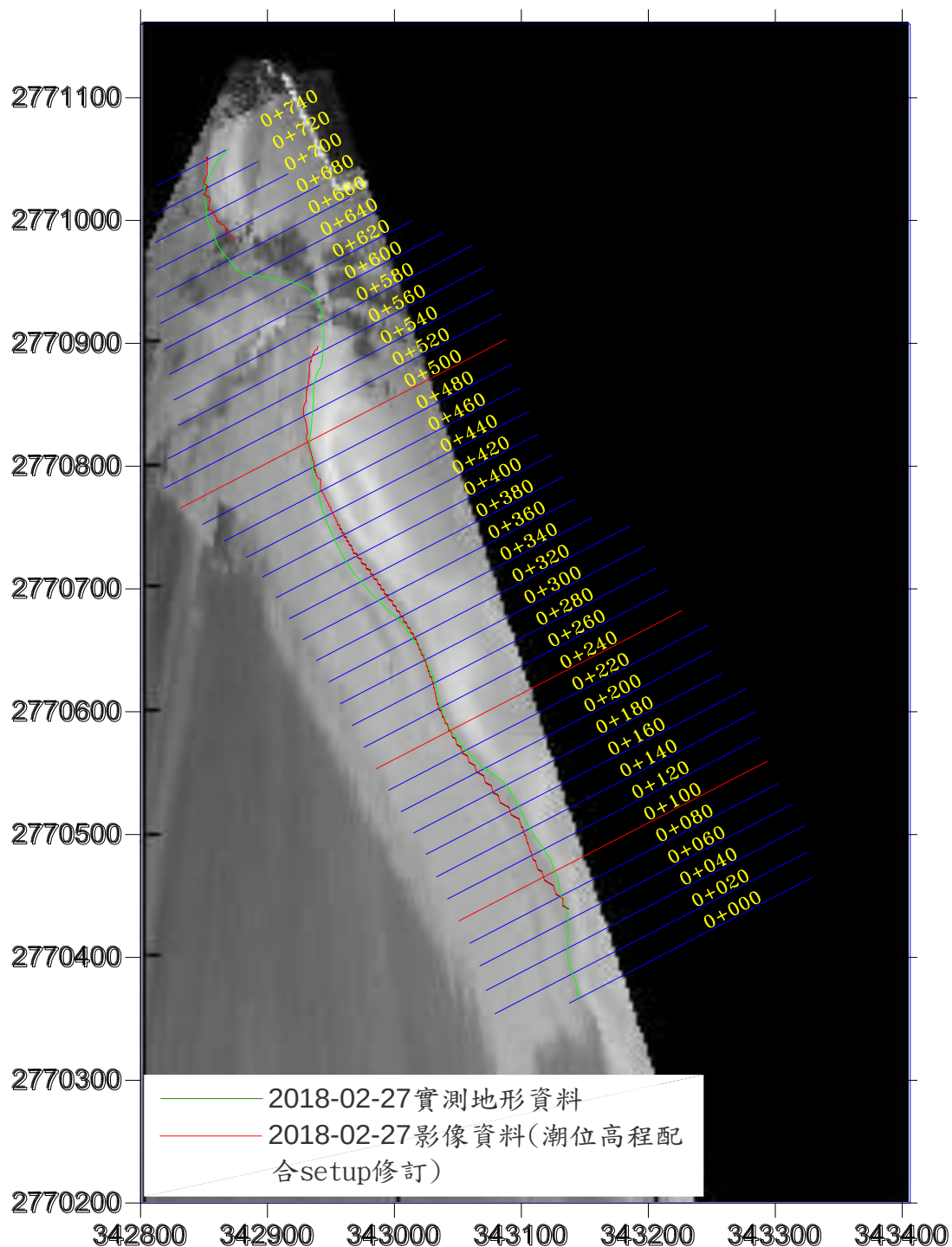
圖 3-22 水位線分析結果圖(2018/2/27)
