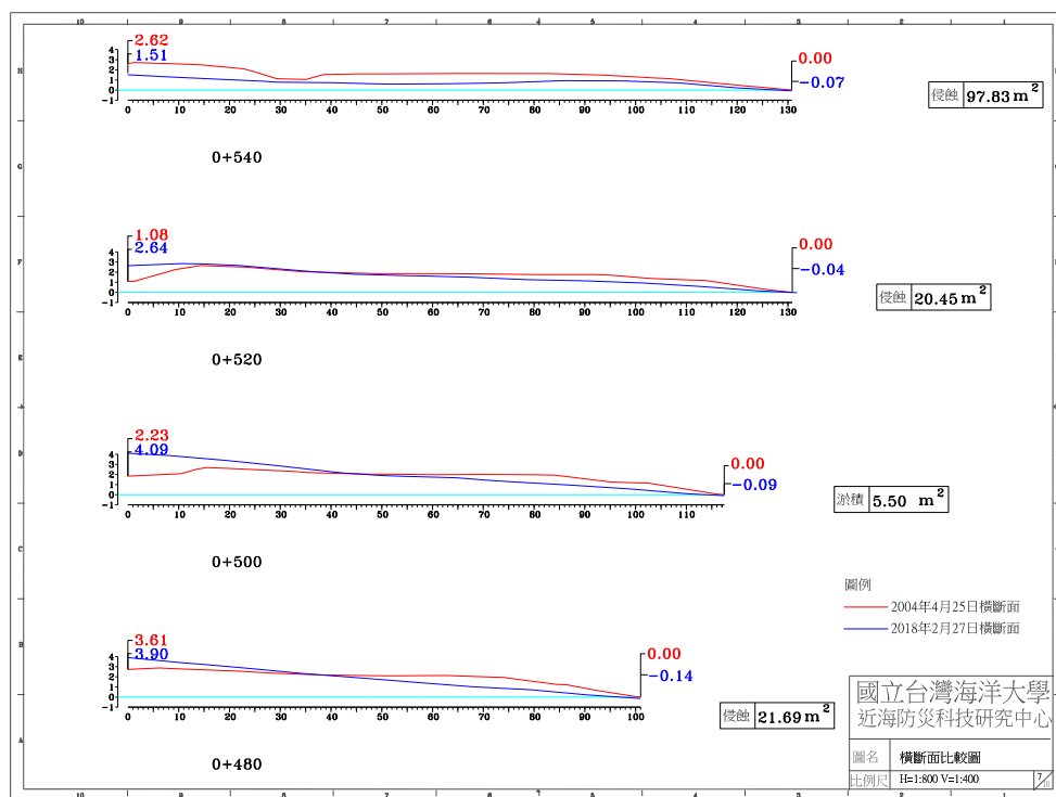
圖 4-4(d) 2018 年 2 月 27 日 A 監測區橫斷面比較圖
