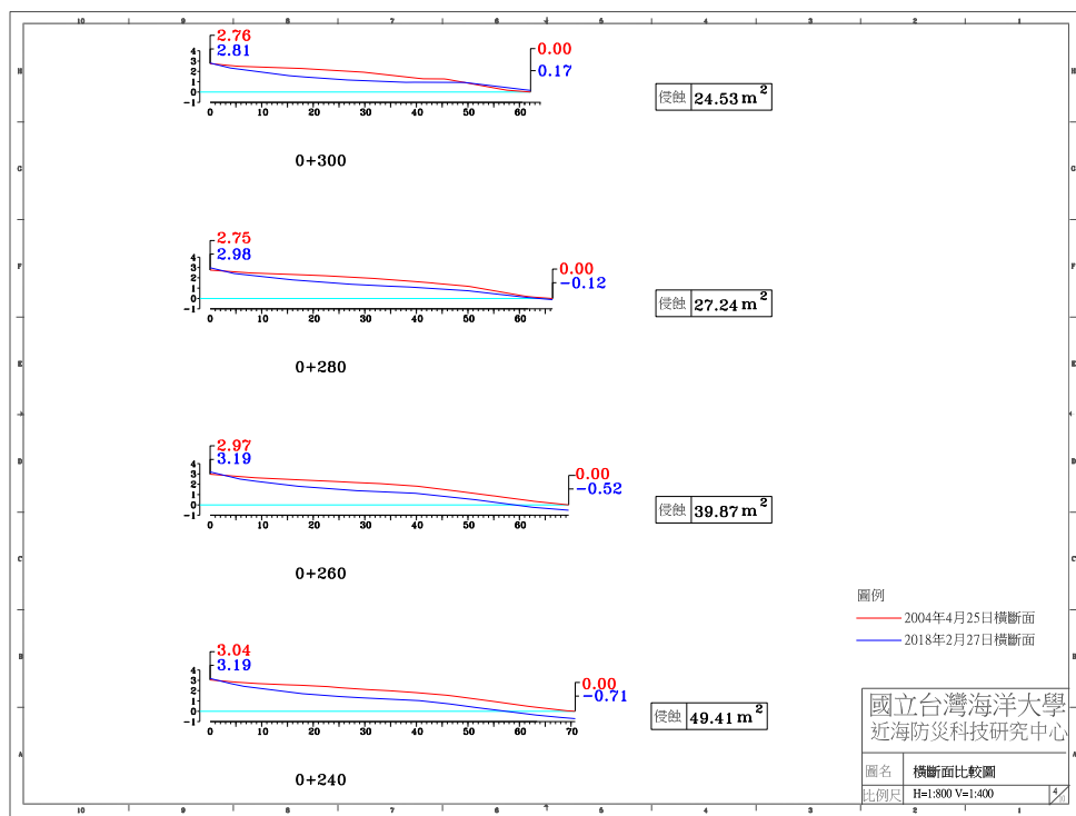
圖 4-4(g) 2018 年 2 月 27 日 A 監測區橫斷面比較圖
