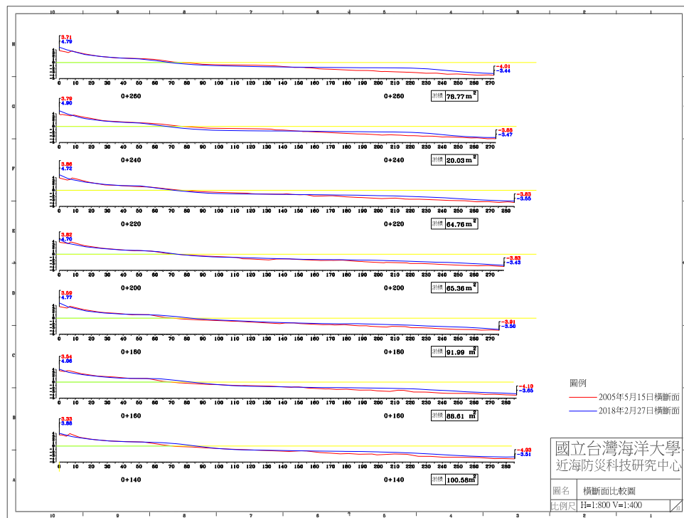
圖 4-5(e) 2018 年 2 月 27 日 B 監測區橫斷面比較圖
