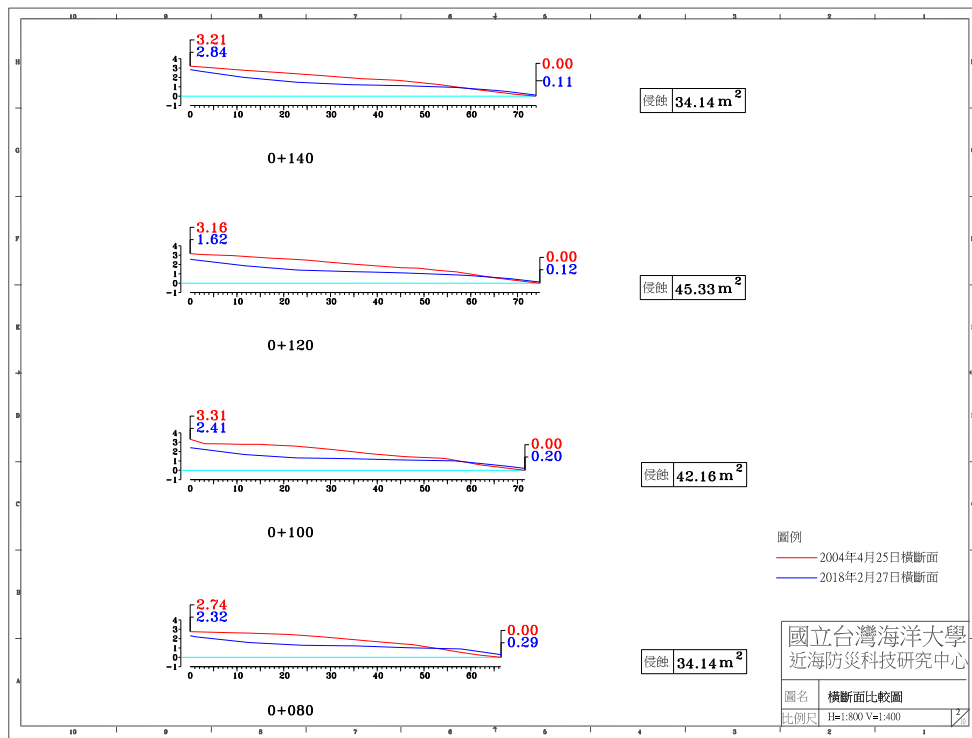
圖 4-4(i) 2018 年 2 月 27 日 A 監測區橫斷面比較圖
