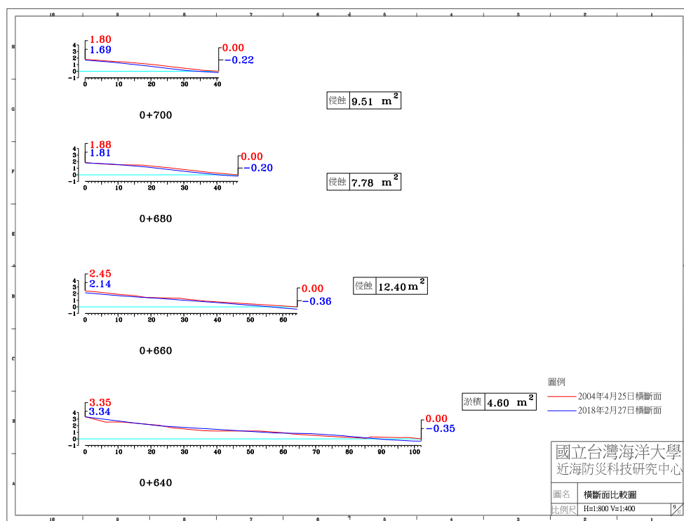
圖 4-4(b) 2018 年 2 月 27 日 A 監測區橫斷面比較圖
