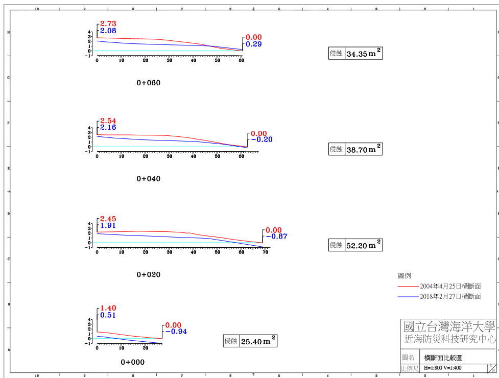
圖 4-4(j) 2018 年 2 月 27 日 A 監測區橫斷面比較圖
