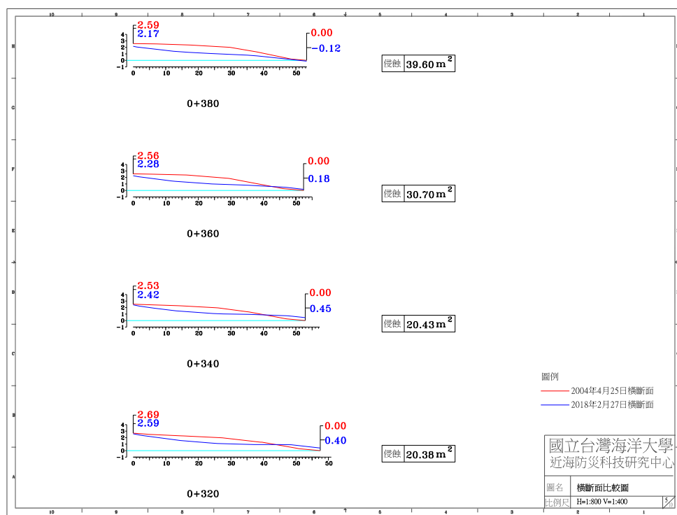
圖 4-4(f) 2018 年 2 月 27 日 A 監測區橫斷面比較圖
