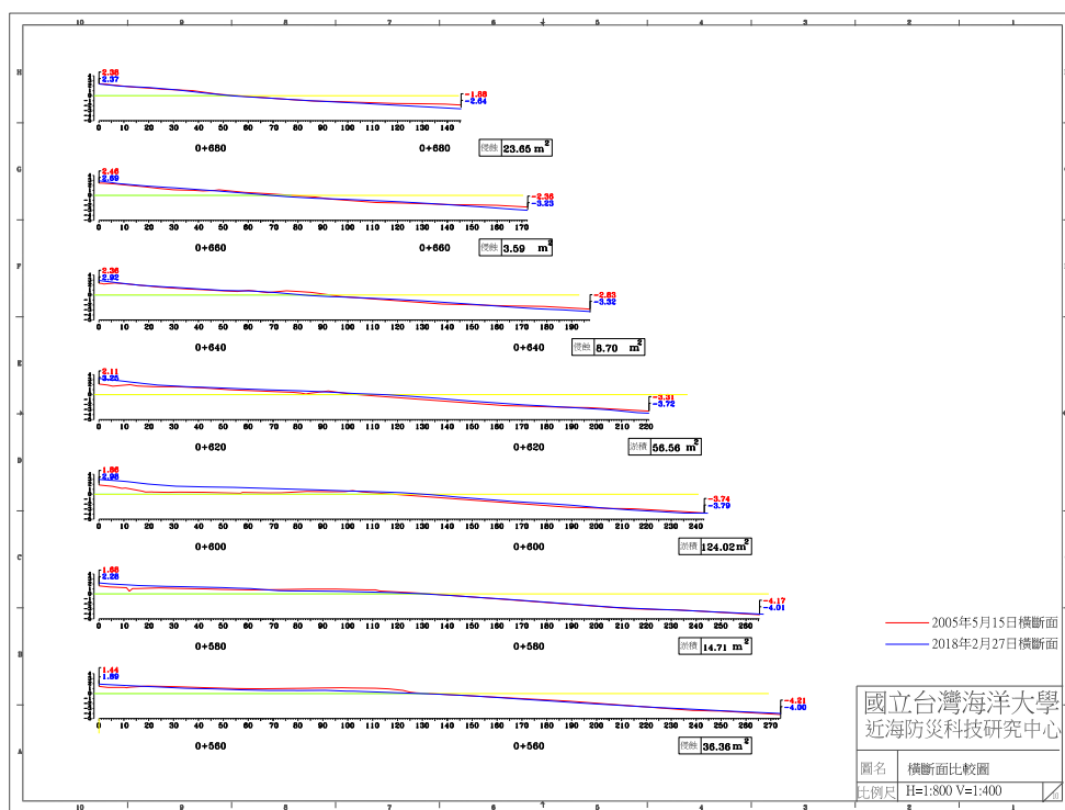
圖 4-5(b) 2018 年 2 月 27 日 B 監測區橫斷面比較圖
