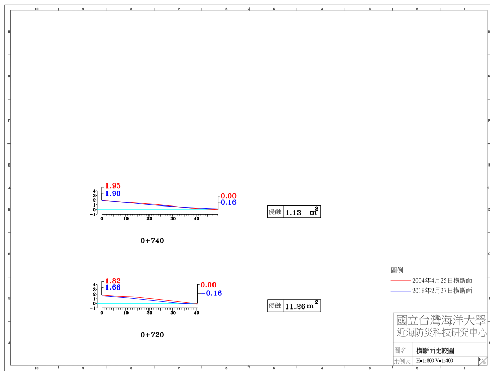
圖 4-4(a) 2018 年 2 月 27 日 A 監測區橫斷面比較圖
