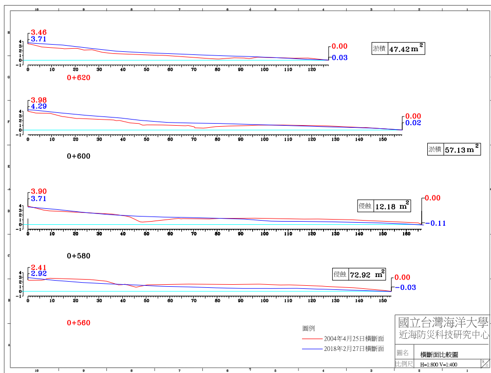
圖 4-4(c) 2018 年 2 月 27 日 A 監測區橫斷面比較圖
