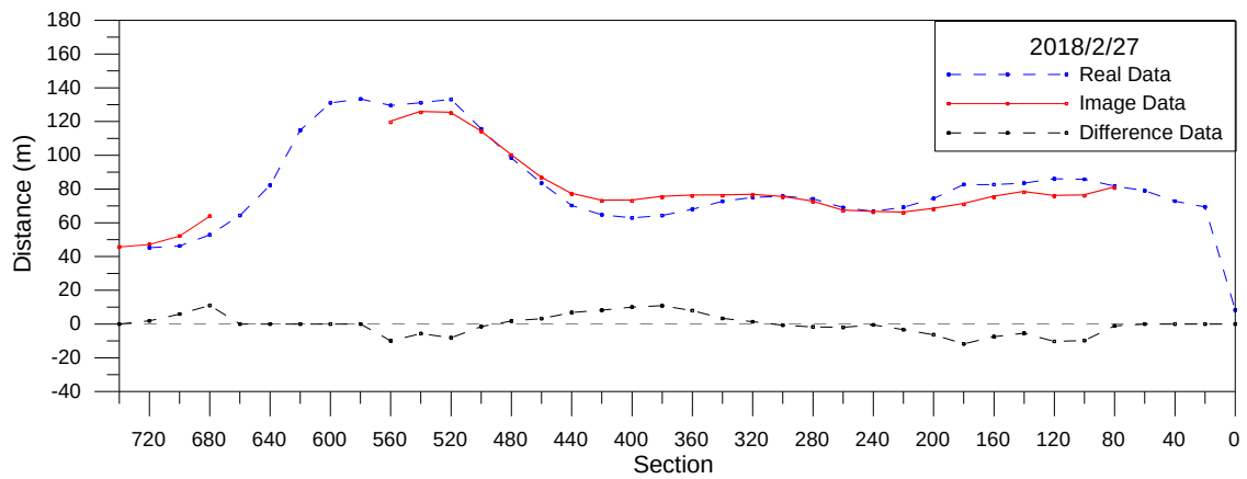
圖 3-23 海岸線分析比較圖(2018/2/27)
