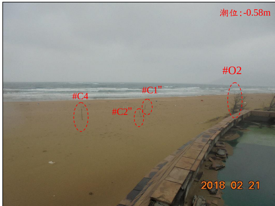
附圖 2-5 小舞台南側輔助觀測樁位置圖(2018/2/21)
