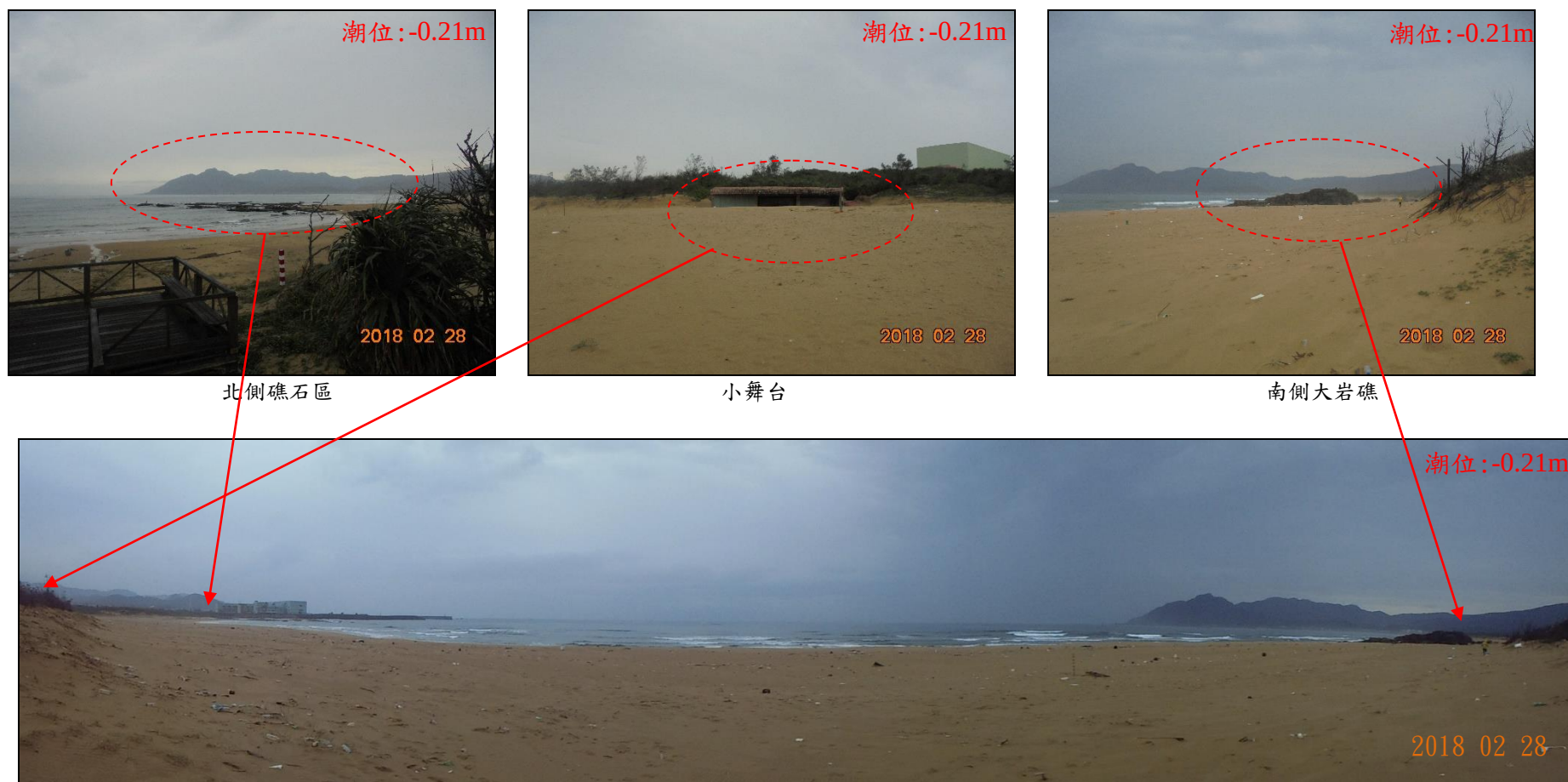
圖 3-6 鹽寮海岸短期性養灘區地形地貌圖(2018/02/28)
