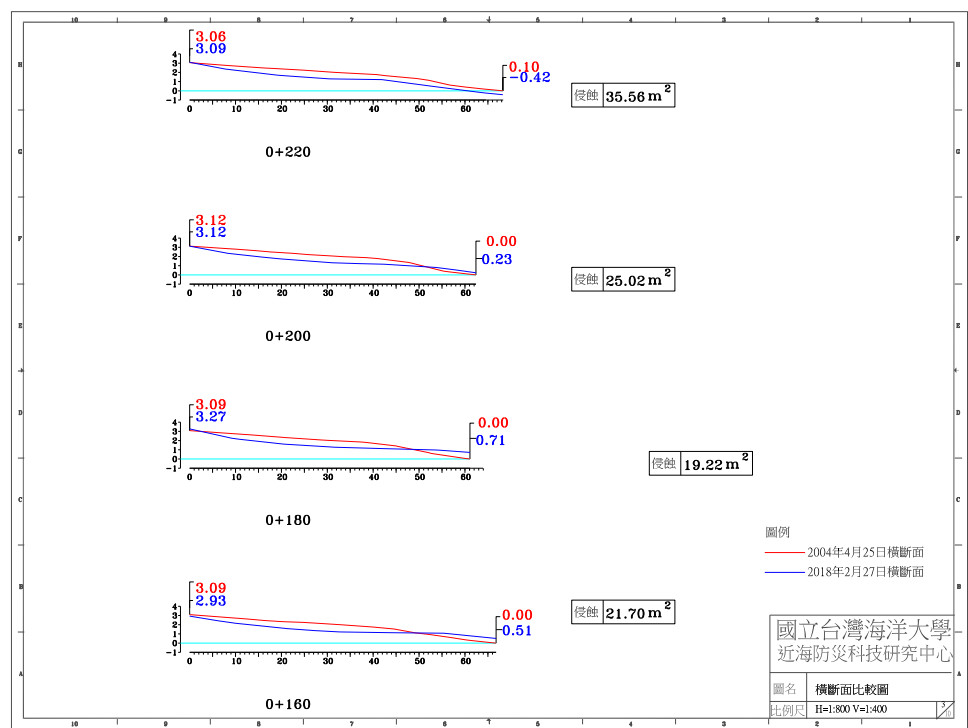
圖 4-4(h) 2018 年 2 月 27 日 A 監測區橫斷面比較圖
