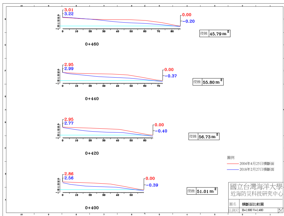
圖 4-4(e) 2018 年 2 月 27 日 A 監測區橫斷面比較圖
