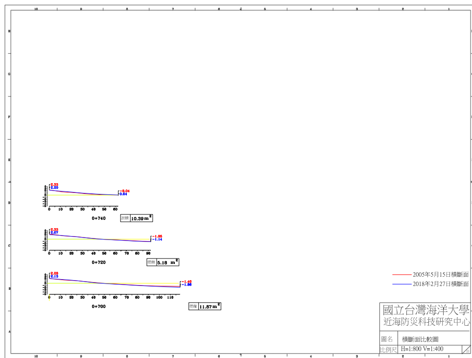
圖 4-5(a) 2018 年 2 月 27 日 B 監測區橫斷面比較圖
