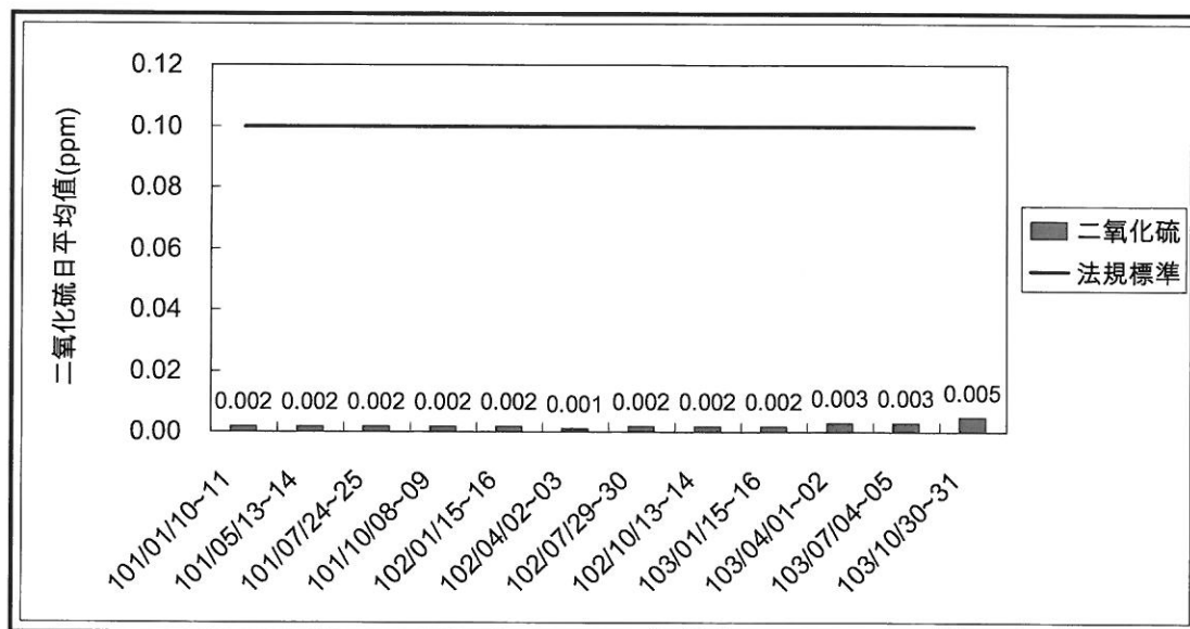
圖 2.1-4 二氧化硫日平均值監測成果彙整
