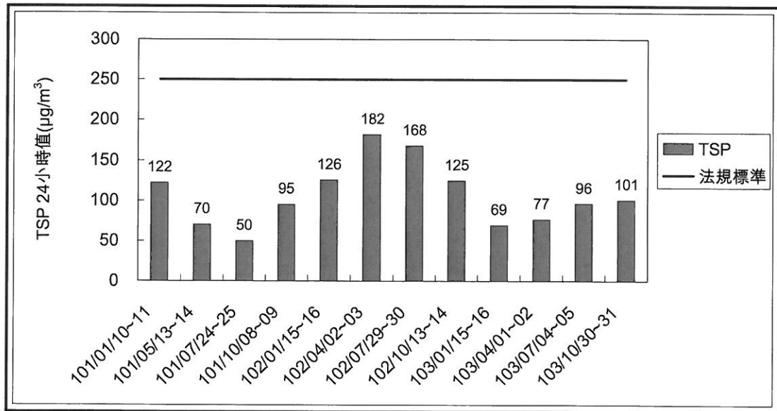
圖 2.1-1 總懸浮微粒 24 小時值監測成果彙整
