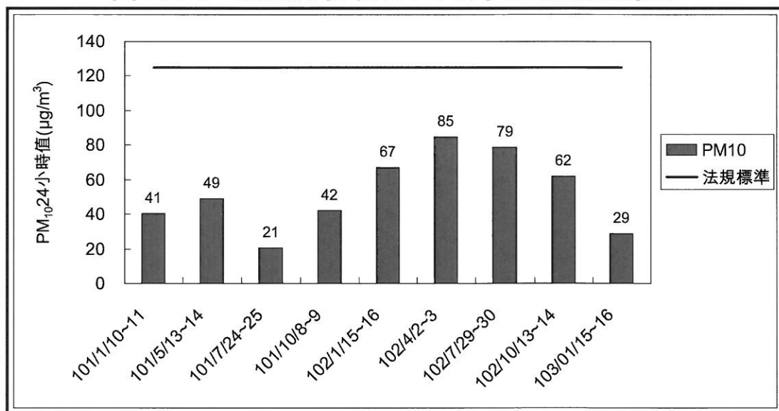
圖 2.1-2 粒徑 \leq 10\mu\text{m} 之懸浮微粒 24 小時值監測成果彙整
