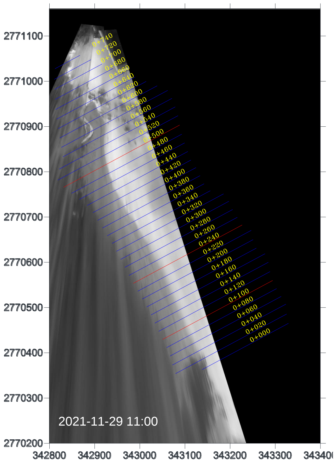
圖 4-14 鹽寮海岸地形影像全景圖(2021/11/29 11 : 00)
