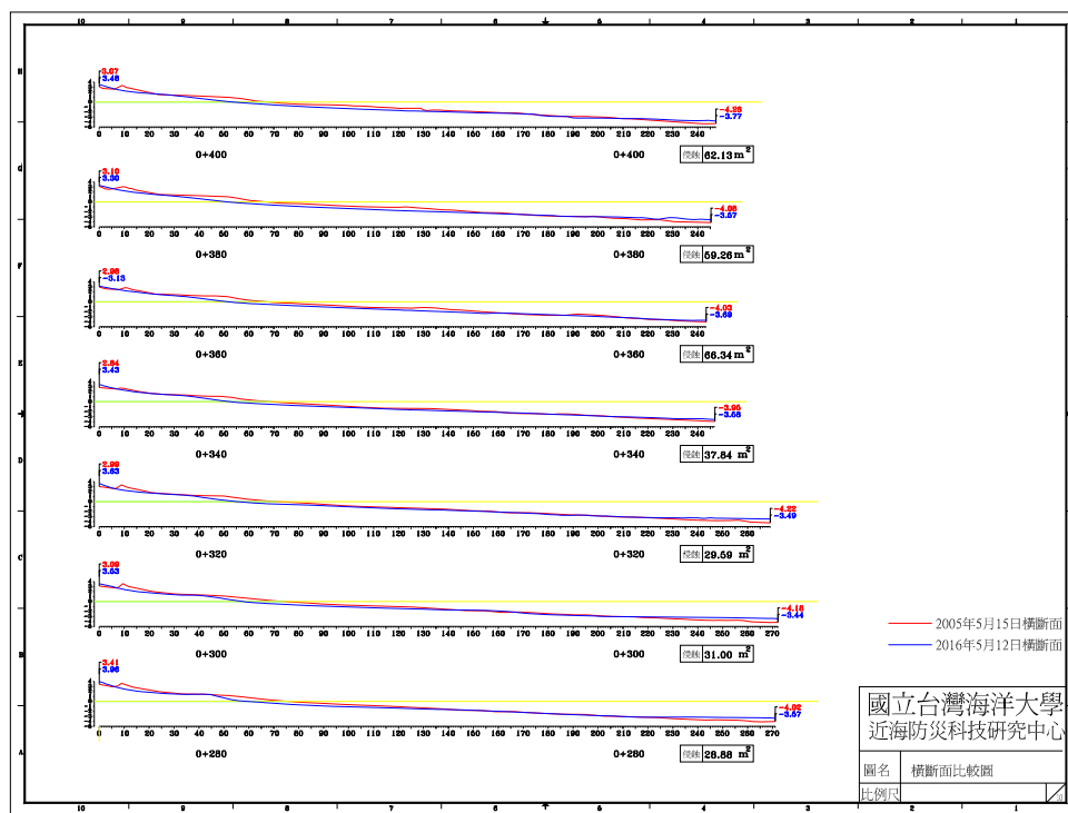
圖 4-5(d) 2016 年 5 月 12 日 B 監測區橫斷面比較圖
