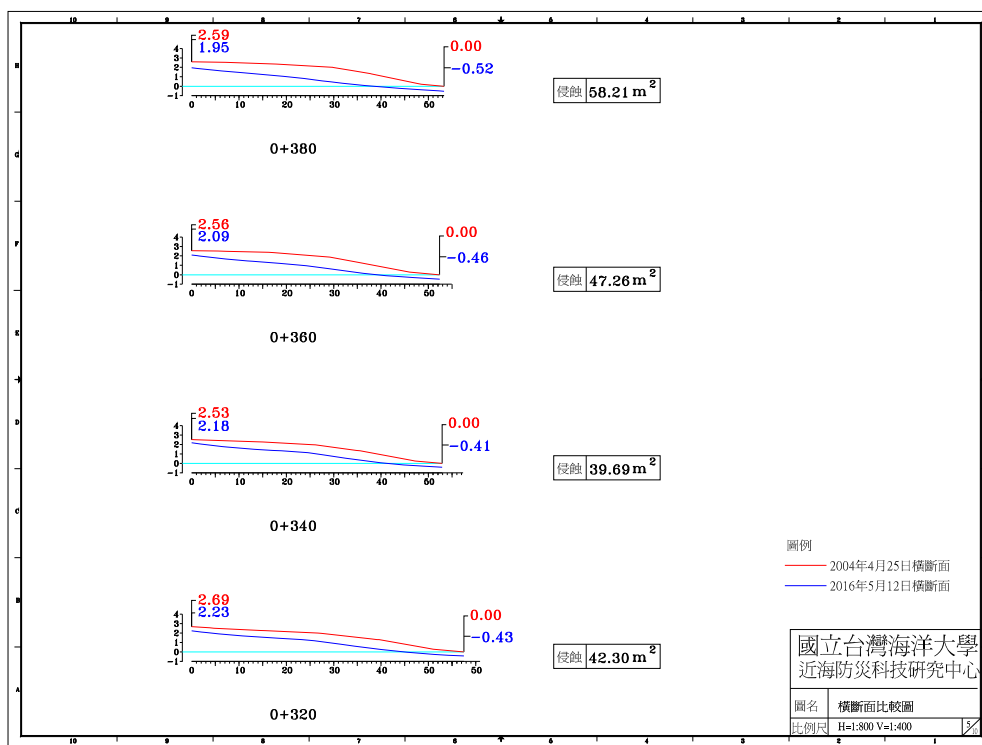
圖 4-4(f) 2016 年 5 月 12 日 A 監測區橫斷面比較圖
