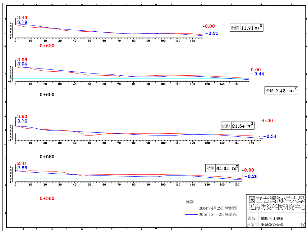
圖 4-4(c) 2016 年 5 月 12 日 A 監測區橫斷面比較圖
