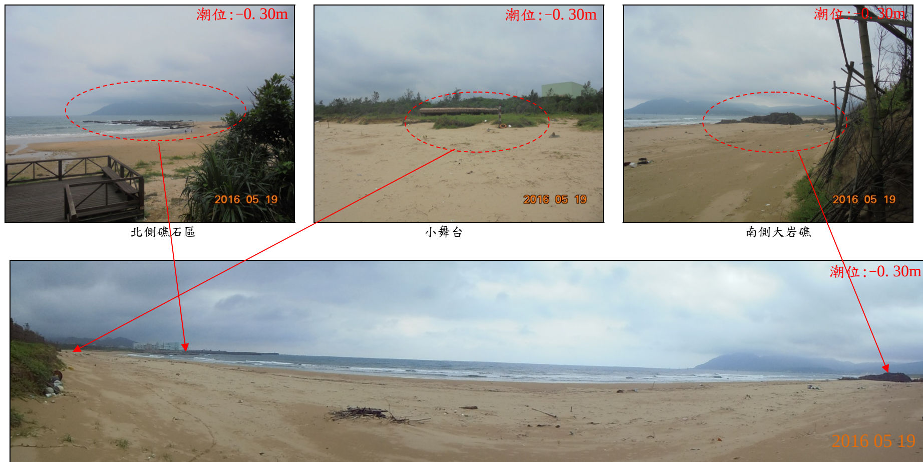
圖 3-6 鹽寮海岸短期性養灘區地形地貌圖(2016/5/19)
