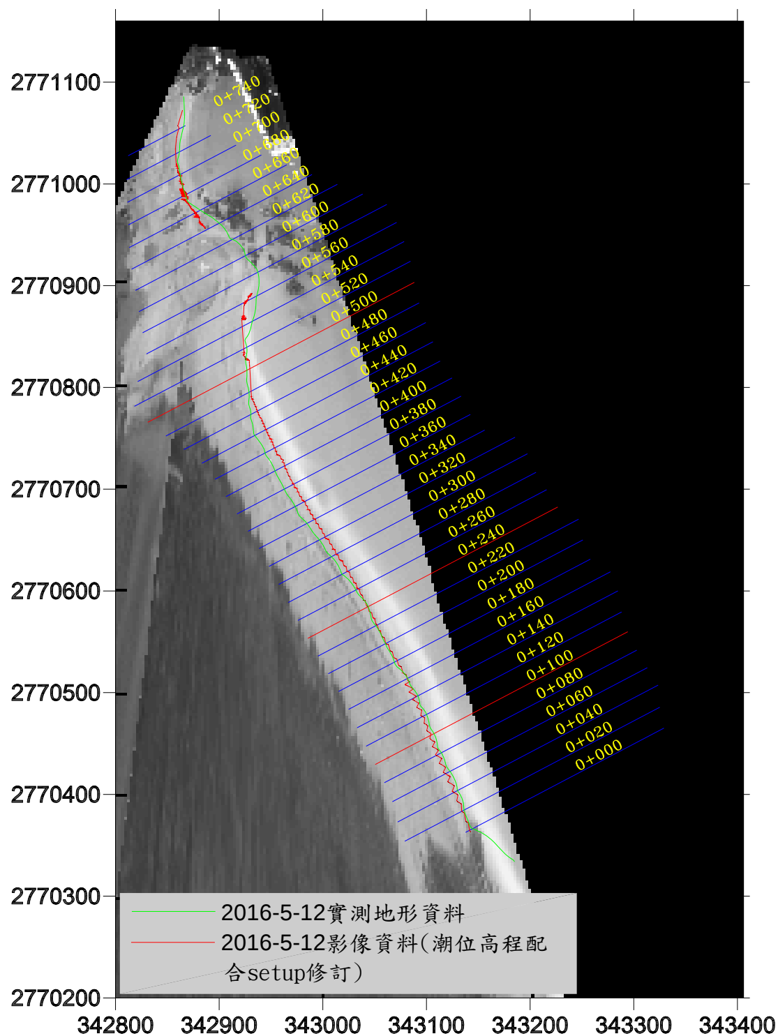
圖 3-22 水位線分析結果圖(2016/5/12)
