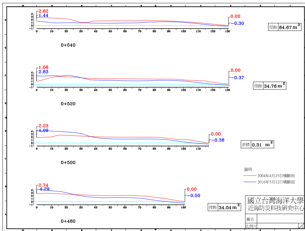
圖 4-4(d) 2016 年 5 月 12 日 A 監測區橫斷面比較圖
