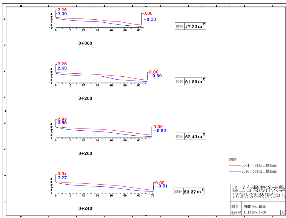
圖 4-4(g) 2016 年 5 月 12 日 A 監測區橫斷面比較圖
