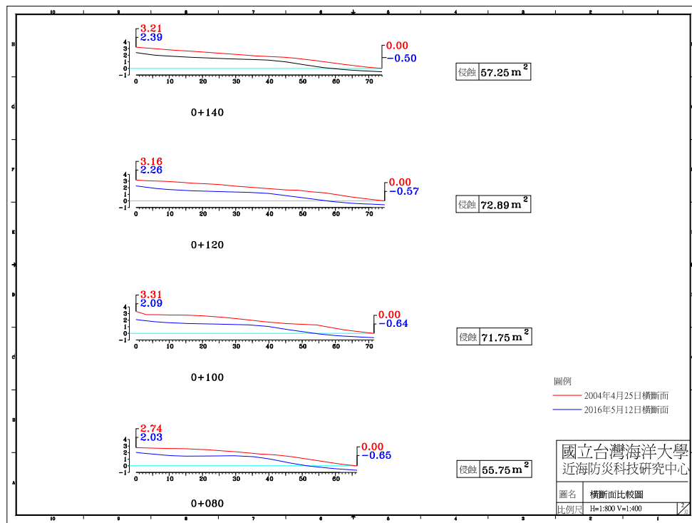
圖 4-4(i) 2016 年 5 月 12 日 A 監測區橫斷面比較圖
