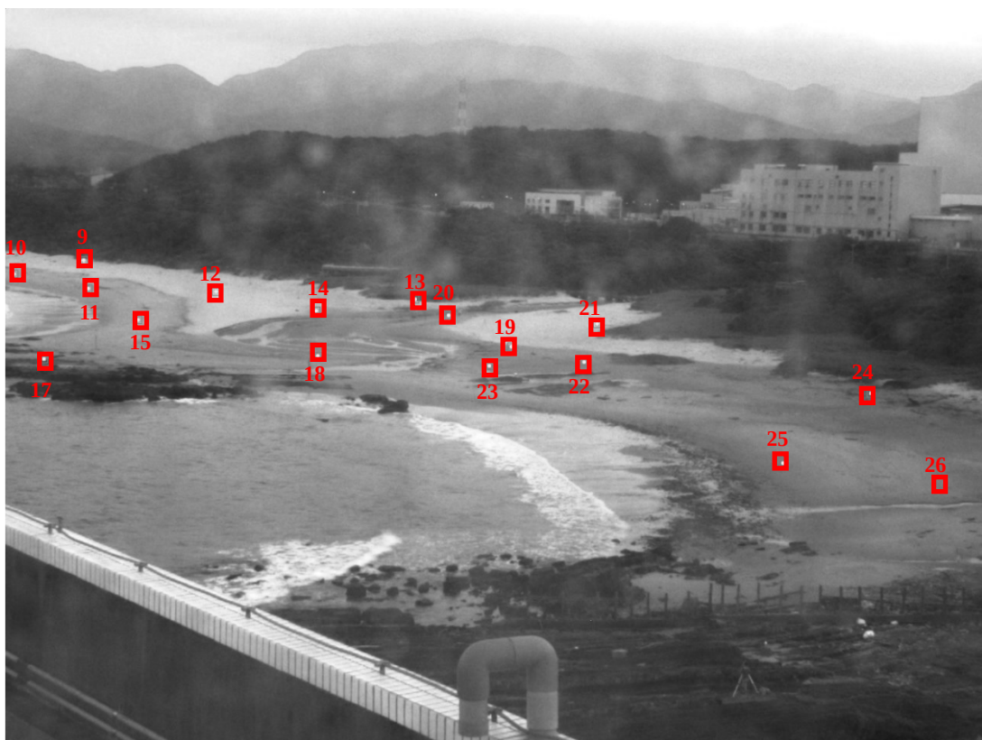
圖 3-21 視角 2(Cam2)地面控制點位置分佈圖例(2016/05/12)
