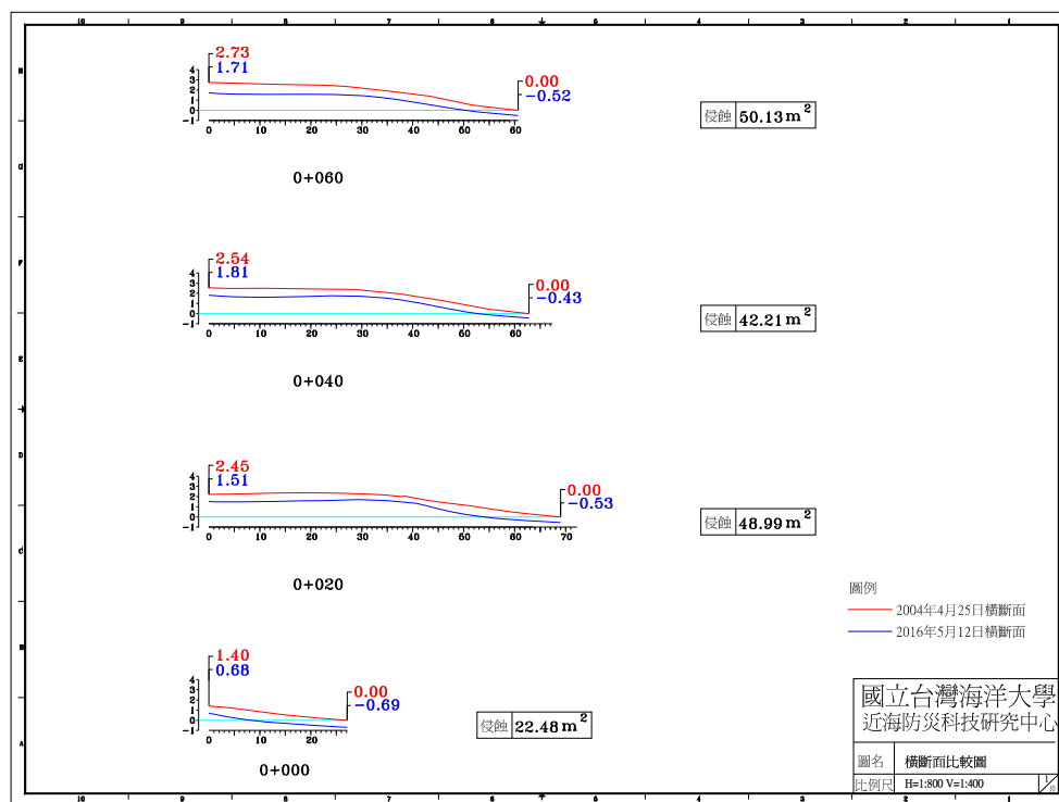
圖 4-4(j) 2016 年 5 月 12 日 A 監測區橫斷面比較圖
