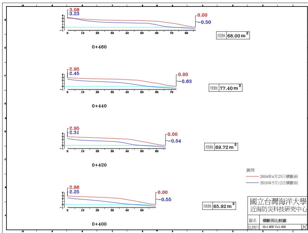
圖 4-4(e) 2016 年 5 月 12 日 A 監測區橫斷面比較圖
