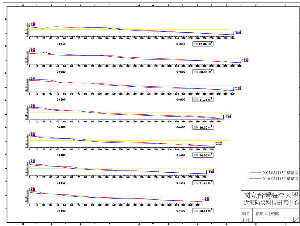
圖 4-5(c) 2016 年 5 月 12 日 B 監測區橫斷面比較圖
