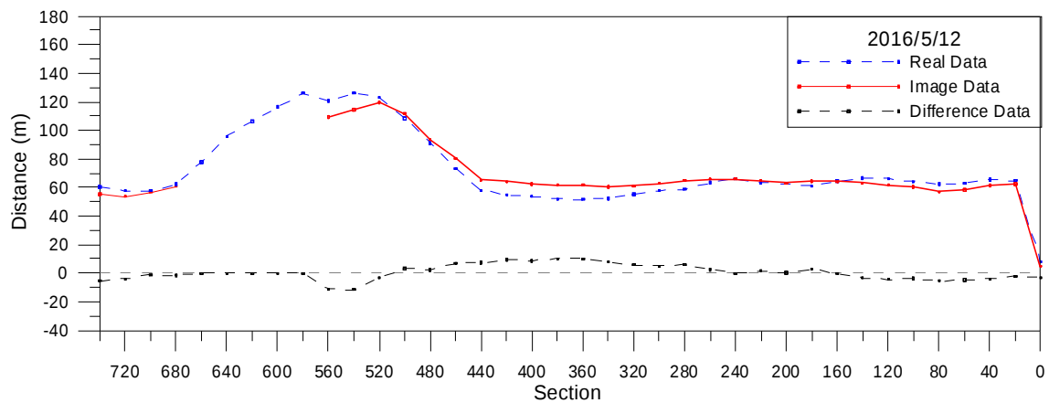
圖 3-23 海岸線分析比較圖(2016/5/12)
