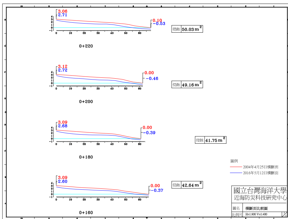
圖 4-4(h) 2016 年 5 月 12 日 A 監測區橫斷面比較圖
