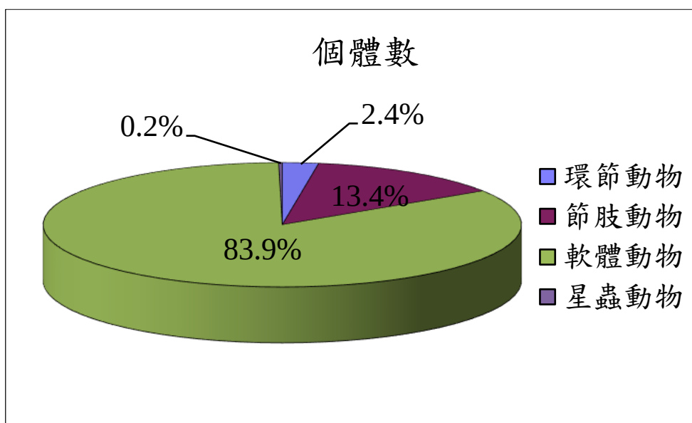
附錄 III.10-1 圖 6 民國 113 年 10 月潮間帶各大類生物之個體數百分比
