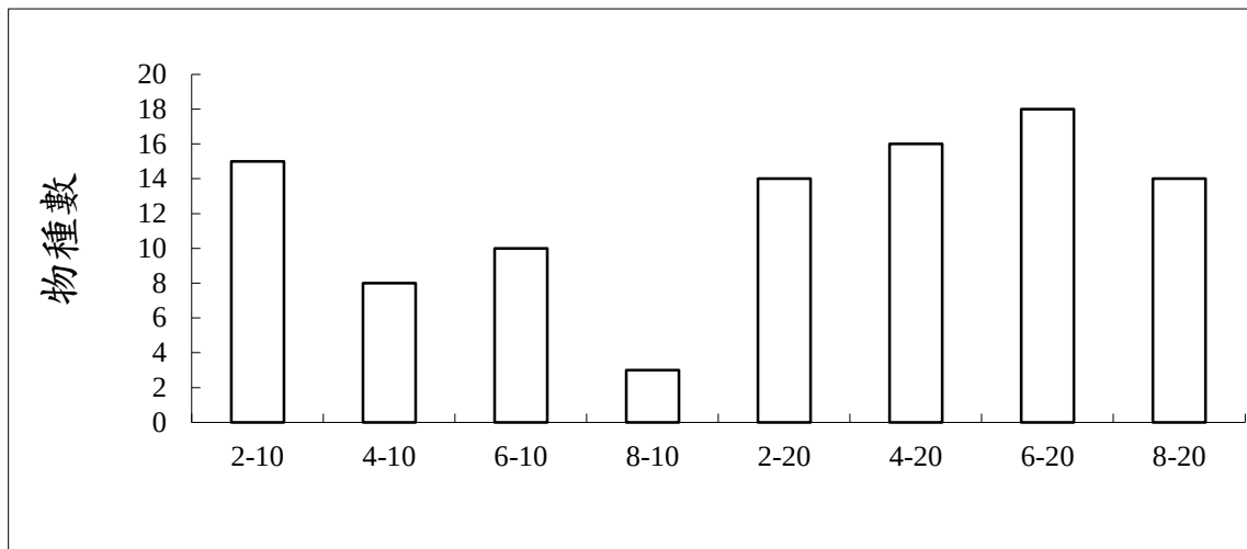
附錄 III.10-1 圖 1 113 年 10 月彰濱產業園區附近海域亞潮帶各測站底棲生物物種數之比較
