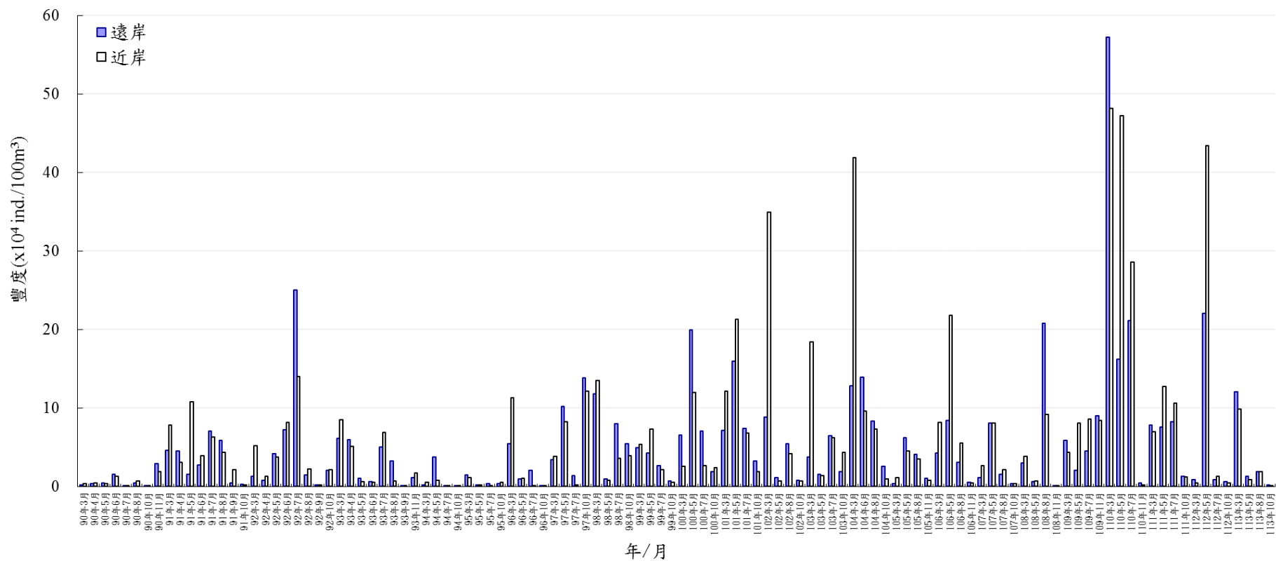
附錄 III.10-2 圖 2 民國 90 年 3 月至 113 年 10 月期間於彰濱產業園區附近海域浮游動物平均豐度之月別變化圖
