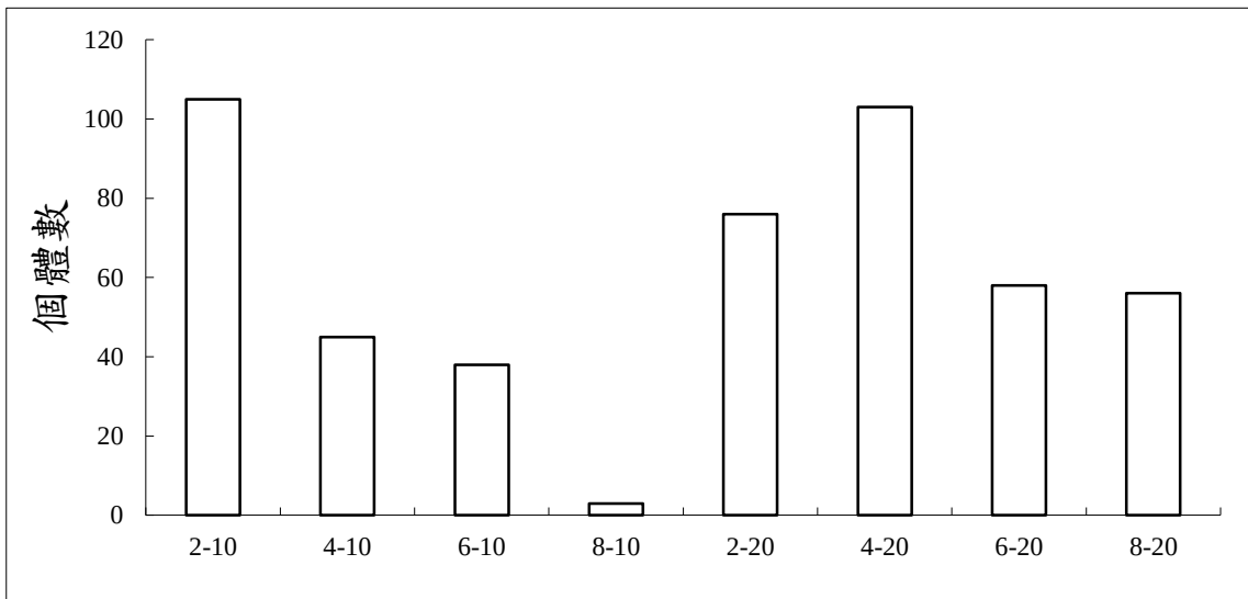
附錄 III.10-1 圖 2 113 年 10 月彰濱產業園區附近海域亞潮帶各測站底棲生物個體數之比較
