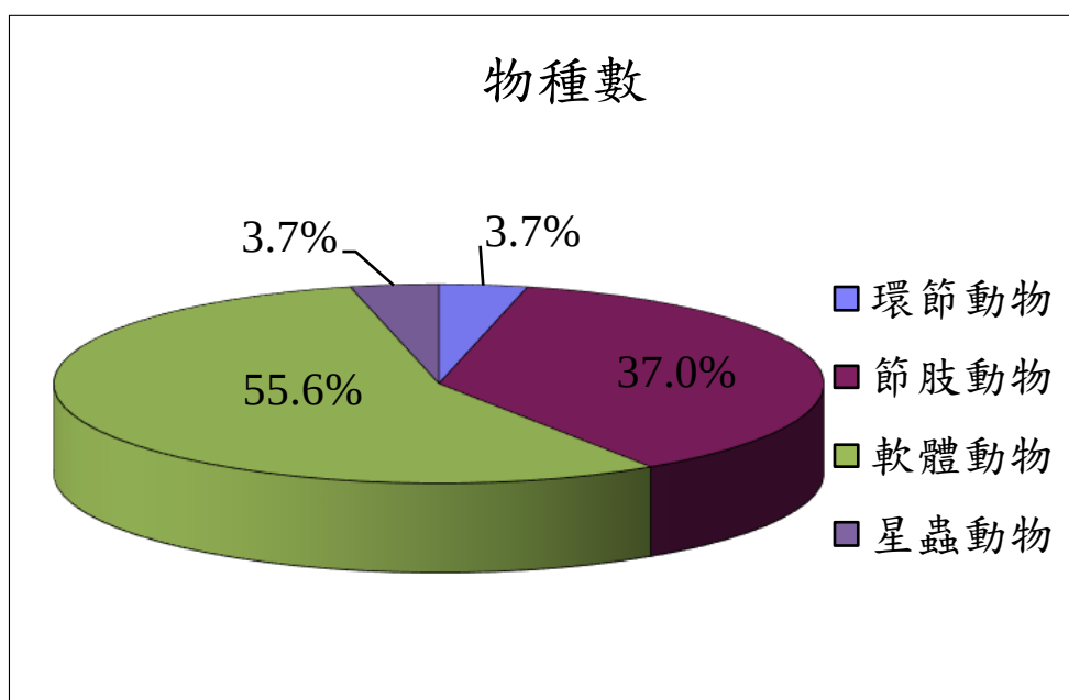
附錄 III.10-1 圖 5 民國 113 年 10 月潮間帶各大類生物之物種數百分比
