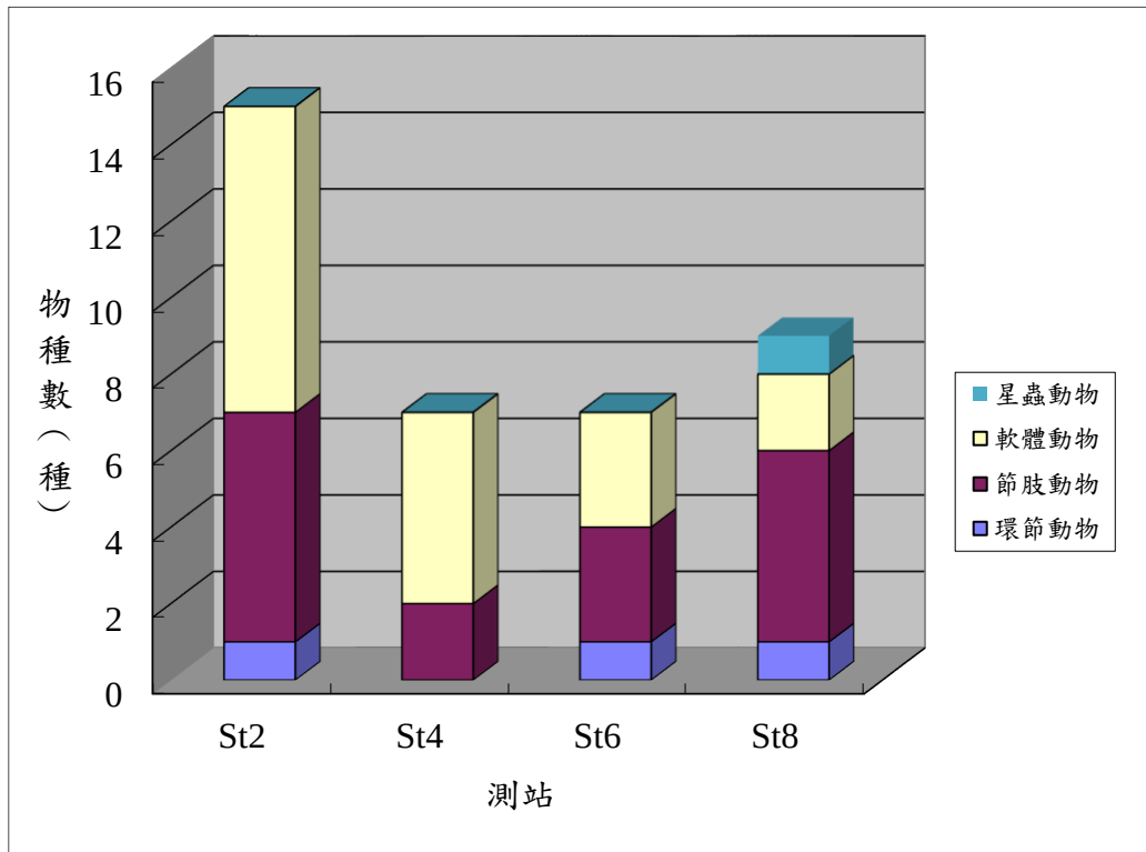
附錄 III.10-1 圖 7 民國 113 年 10 月於彰濱產業園區附近海域潮間帶各測站各大類生物之物種數比較圖
