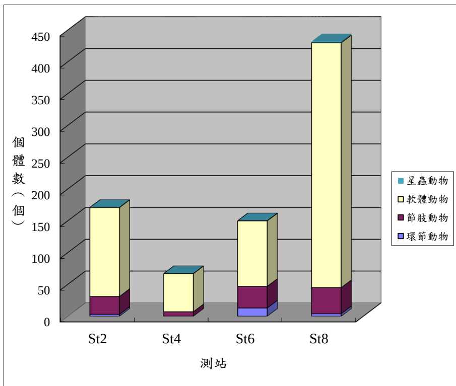
附錄 III.10-1 圖 8 民國 113 年 10 月於彰濱產業園區附近海域潮間帶各測站各大類生物之個體數比較圖
