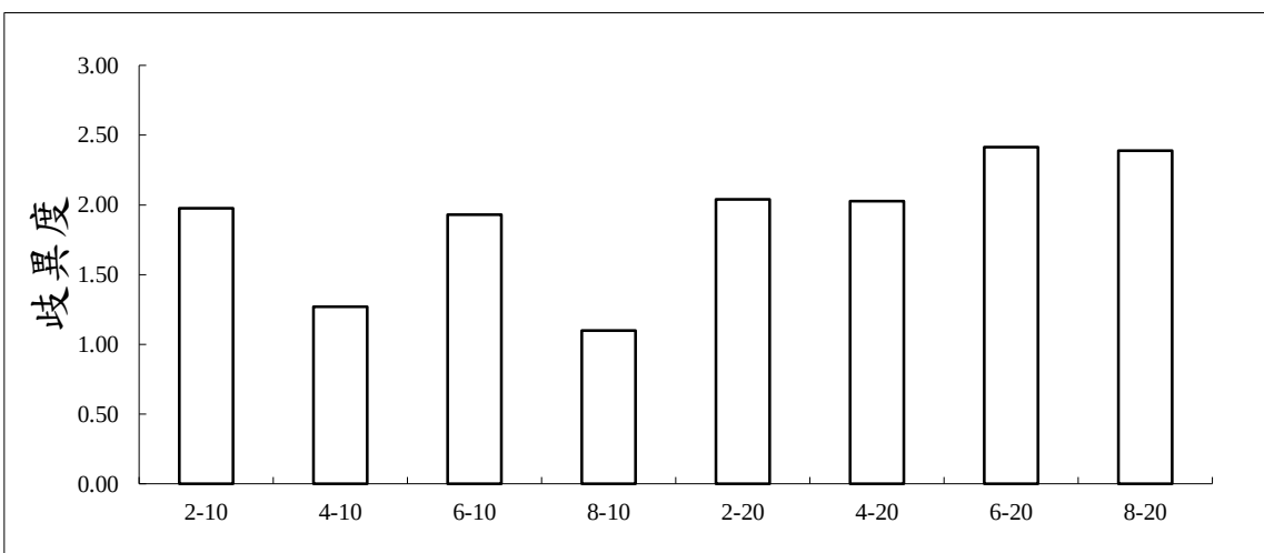
附錄 III.10-1 圖 3 113 年 10 月彰濱產業園區附近海域亞潮帶各測站底棲生物歧異度之比較
