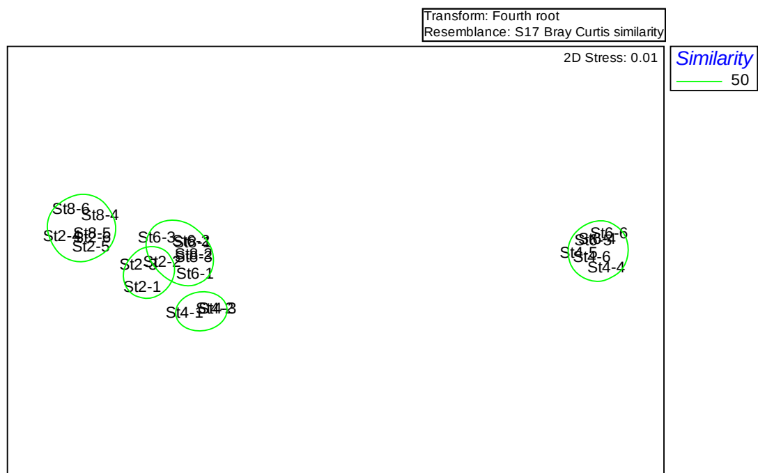
附錄 III.10-2 圖 4 民國 113 年 10 月於彰濱產業園區附近海域潮間帶各測站之群聚 MDS 圖
