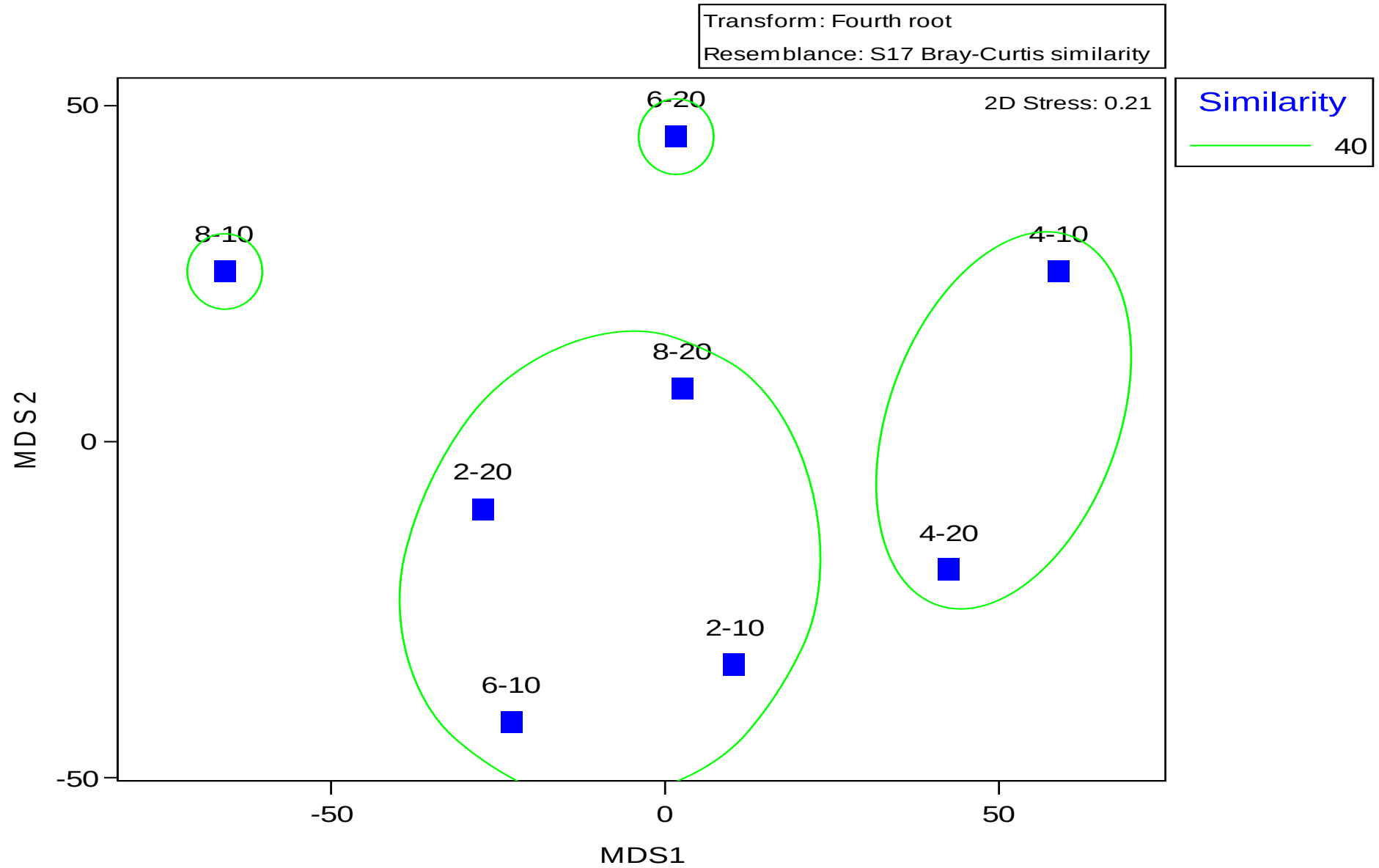
附錄 III.10-1 圖 5 113 年 10 月彰濱產業園區附近海域亞潮帶各測站間底棲生物 MDS 分析圖
