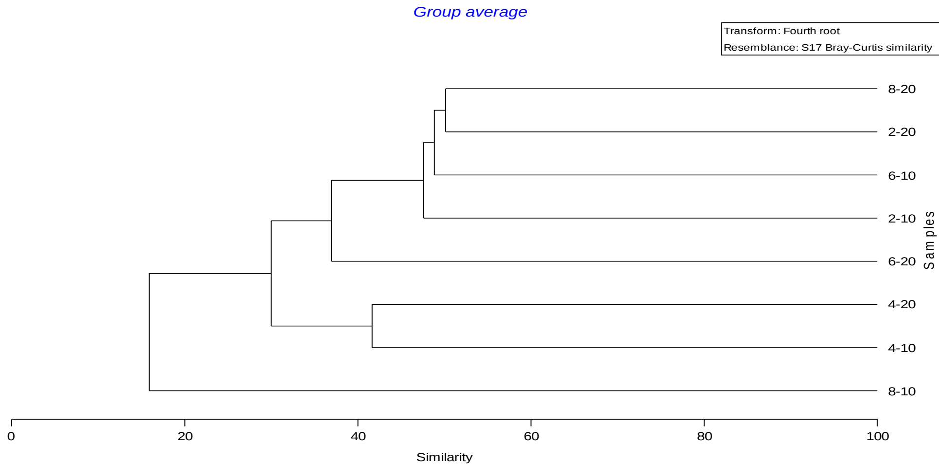
附錄 III.10-1 圖 4 113 年 10 月彰濱產業園區附近海域亞潮帶各測站間底棲生物群聚之聚類分析圖
