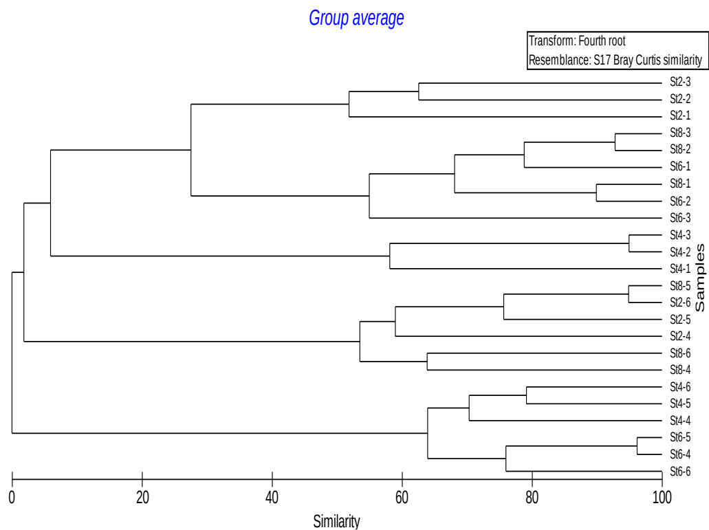
附錄 III.10-2 圖 3 民國 113 年 10 月於彰濱產業園區附近海域潮間帶各測站之群聚分析樹狀圖
