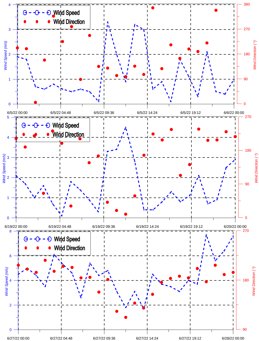
圖 2-3 風速風向時序列變化圖
