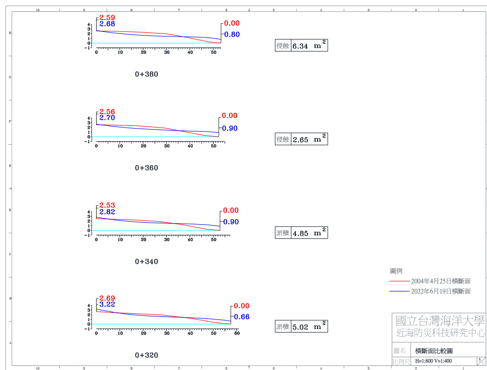
圖 4-4(f) 2022 年 6 月 19 日 A 監測區橫斷面比較圖
