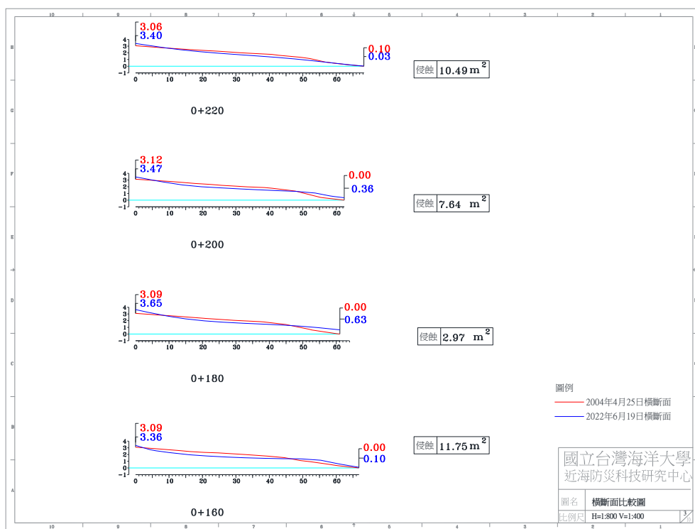
圖 4-4(h) 2022 年 6 月 19 日 A 監測區橫斷面比較圖
