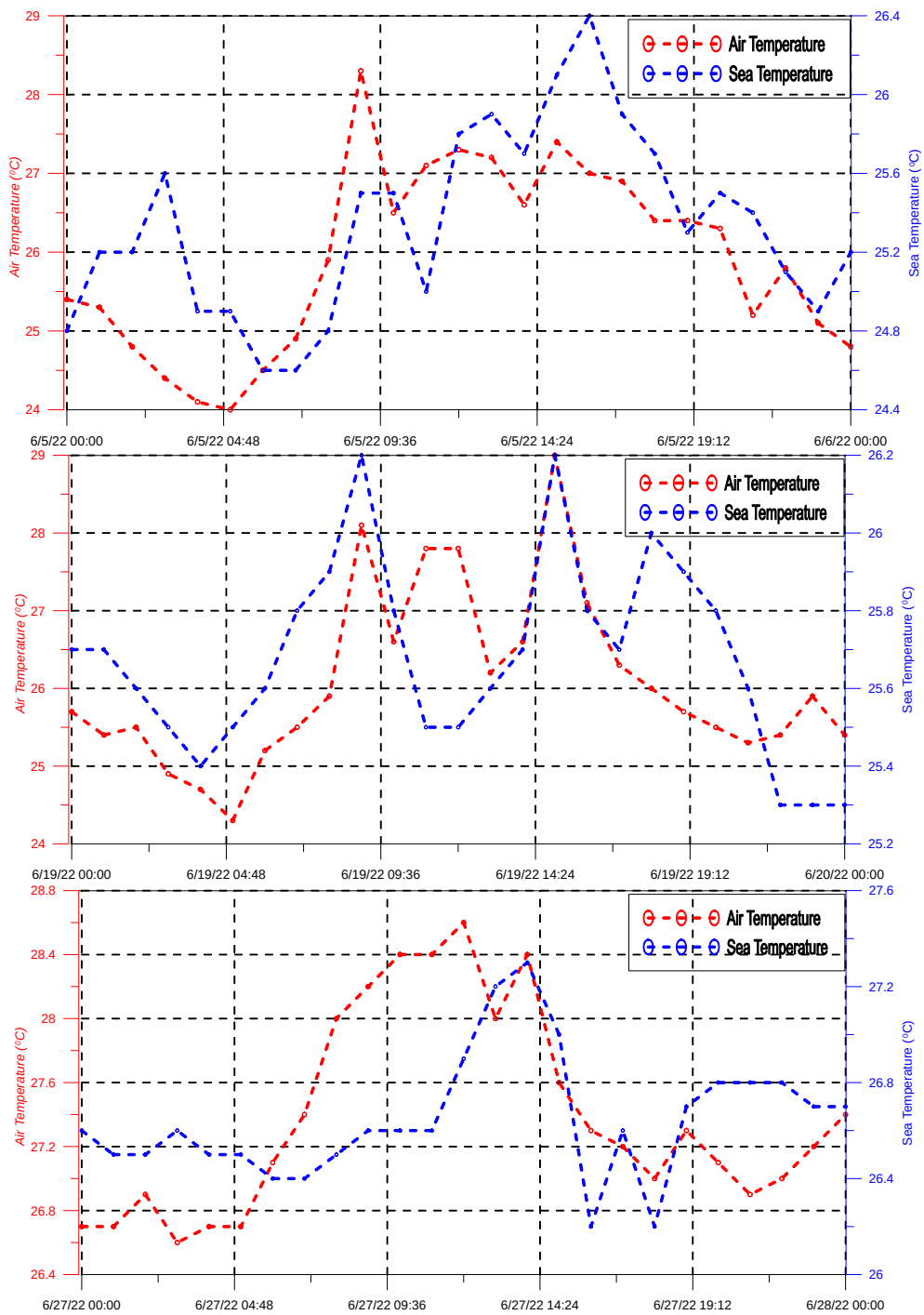
圖 2-5 溫度時序列變化圖
