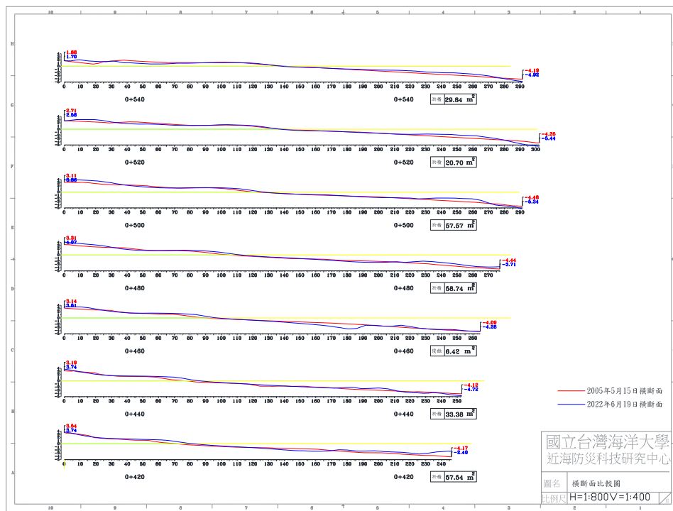
圖 4-5(c) 2022 年 6 月 19 日 B 監測區橫斷面比較圖
