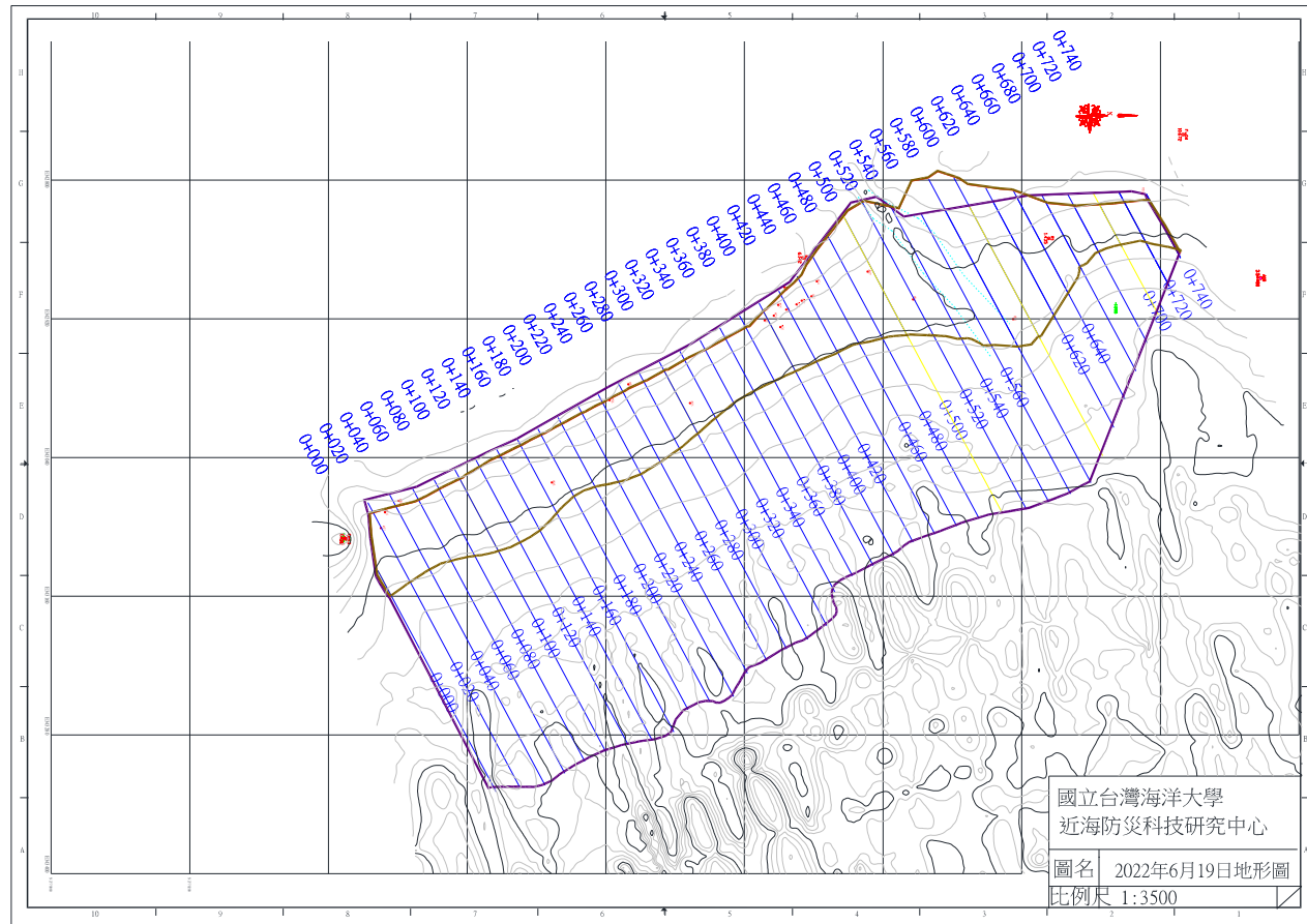
圖 4-1 2022 年 6 月 19 日監測地形
