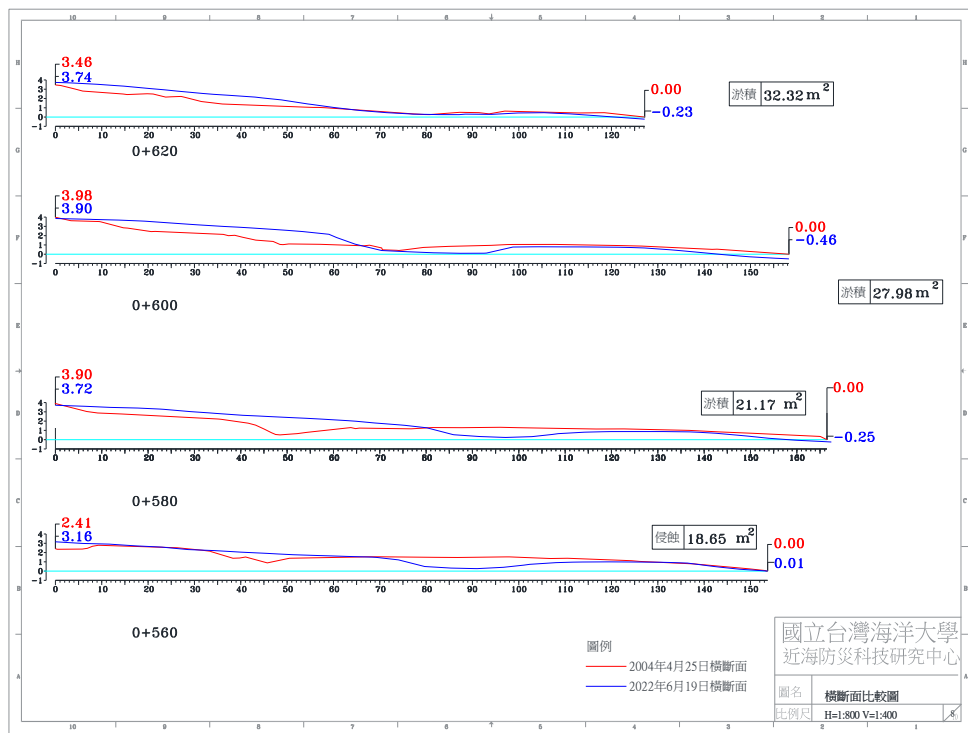
圖 4-4(c) 2022 年 6 月 19 日 A 監測區橫斷面比較圖
