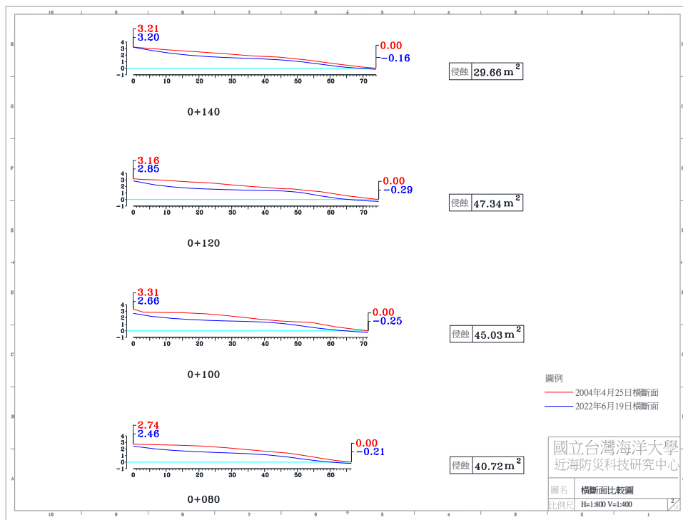
圖 4-4(i) 2022 年 6 月 19 日 A 監測區橫斷面比較圖
