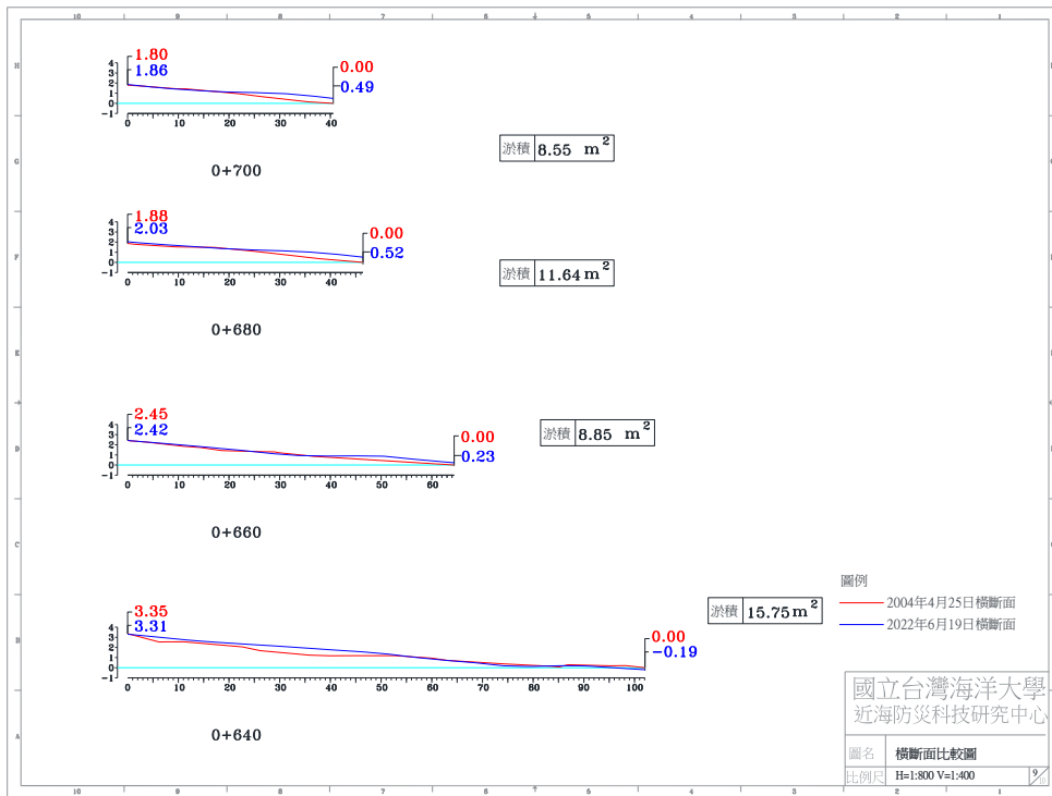
圖 4-4(b) 2022 年 6 月 19 日 A 監測區橫斷面比較圖
