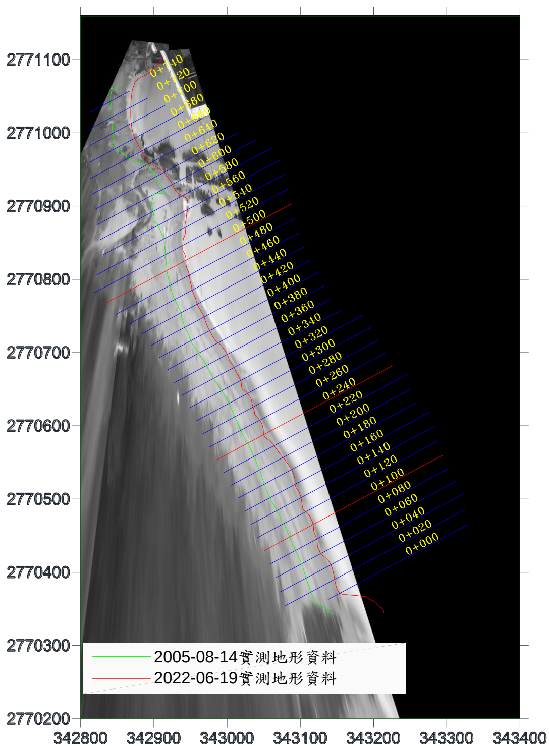
圖 4-22 長期實測 0 m 灘線比對平面示意圖(2022/06/19)
