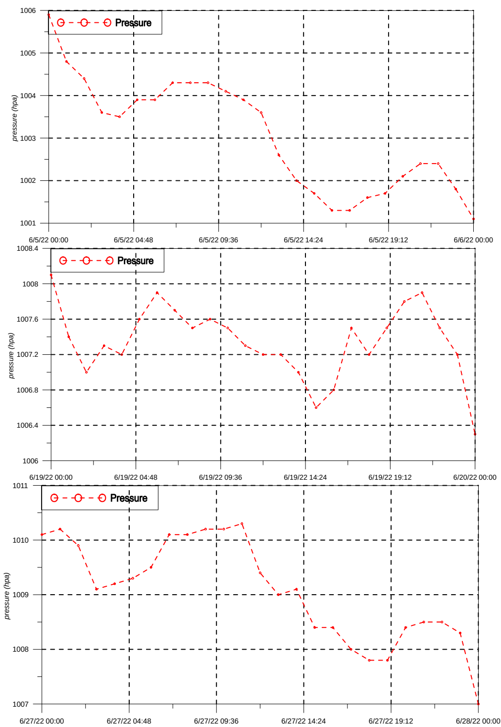
圖 2-6 壓力時序列變化圖
