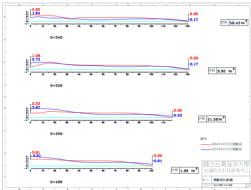
圖 4-4(d) 2022 年 6 月 19 日 A 監測區橫斷面比較圖
