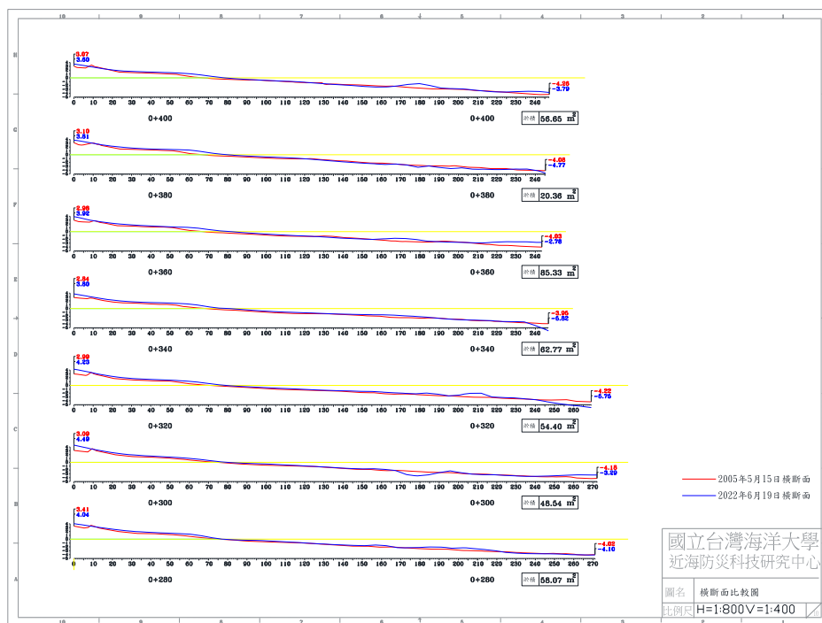
圖 4-5(d) 2022 年 6 月 19 日 B 監測區橫斷面比較圖
