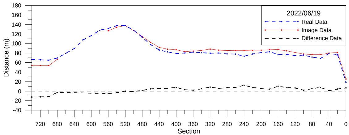
圖 3-23 海岸線分析比較圖(2022/06/19)
