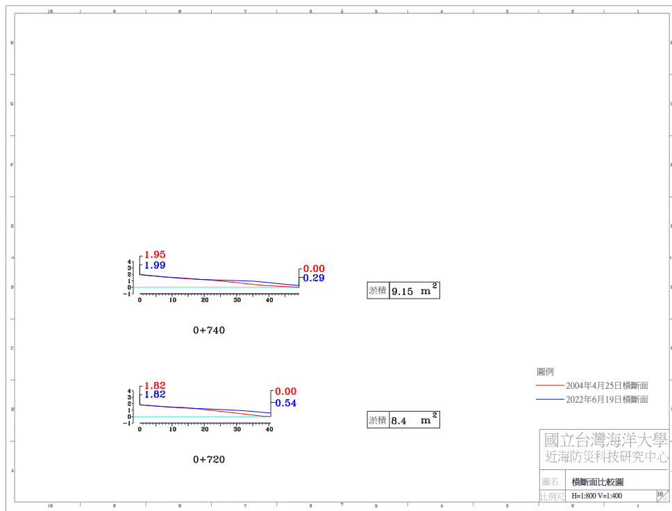
圖 4-4(a) 2022 年 6 月 19 日 A 監測區橫斷面比較圖
