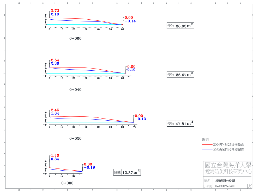
圖 4-4(j) 2022 年 6 月 19 日 A 監測區橫斷面比較圖
