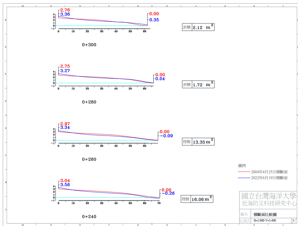
圖 4-4(g) 2022 年 6 月 19 日 A 監測區橫斷面比較圖
