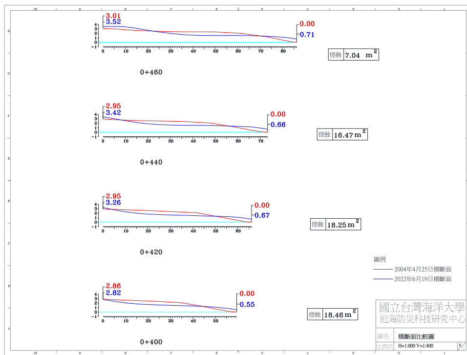
圖 4-4(e) 2022 年 6 月 19 日 A 監測區橫斷面比較圖
