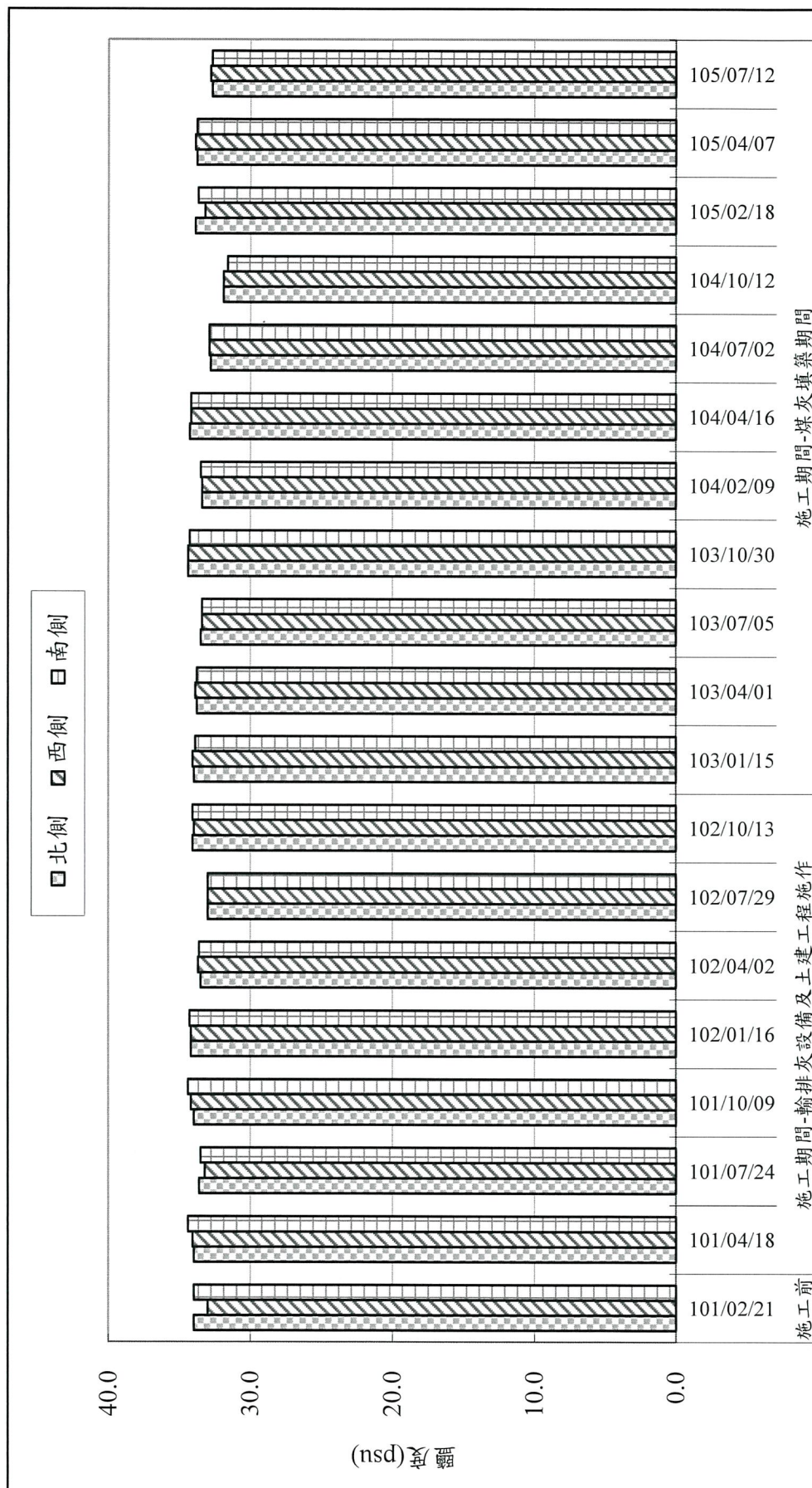
圖 2.2-4 歷季各測站鹽度監測成果彙整
