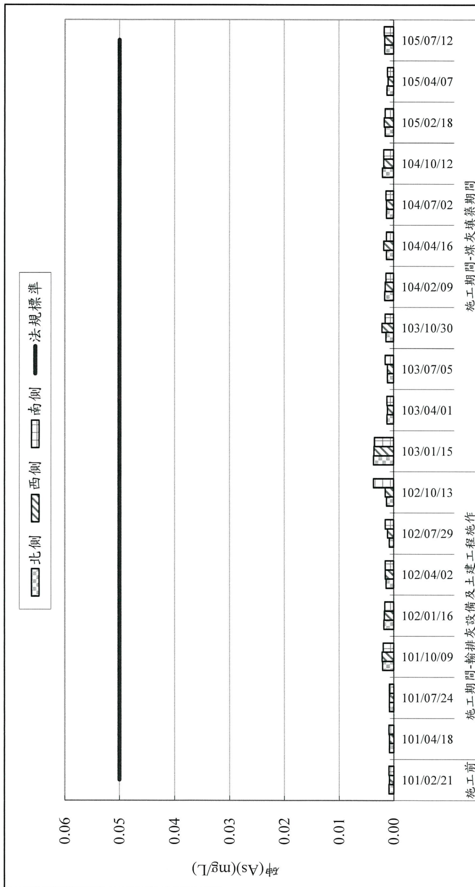
圖 2.2-14 歷季各測站砷(As)監測成果彙整
