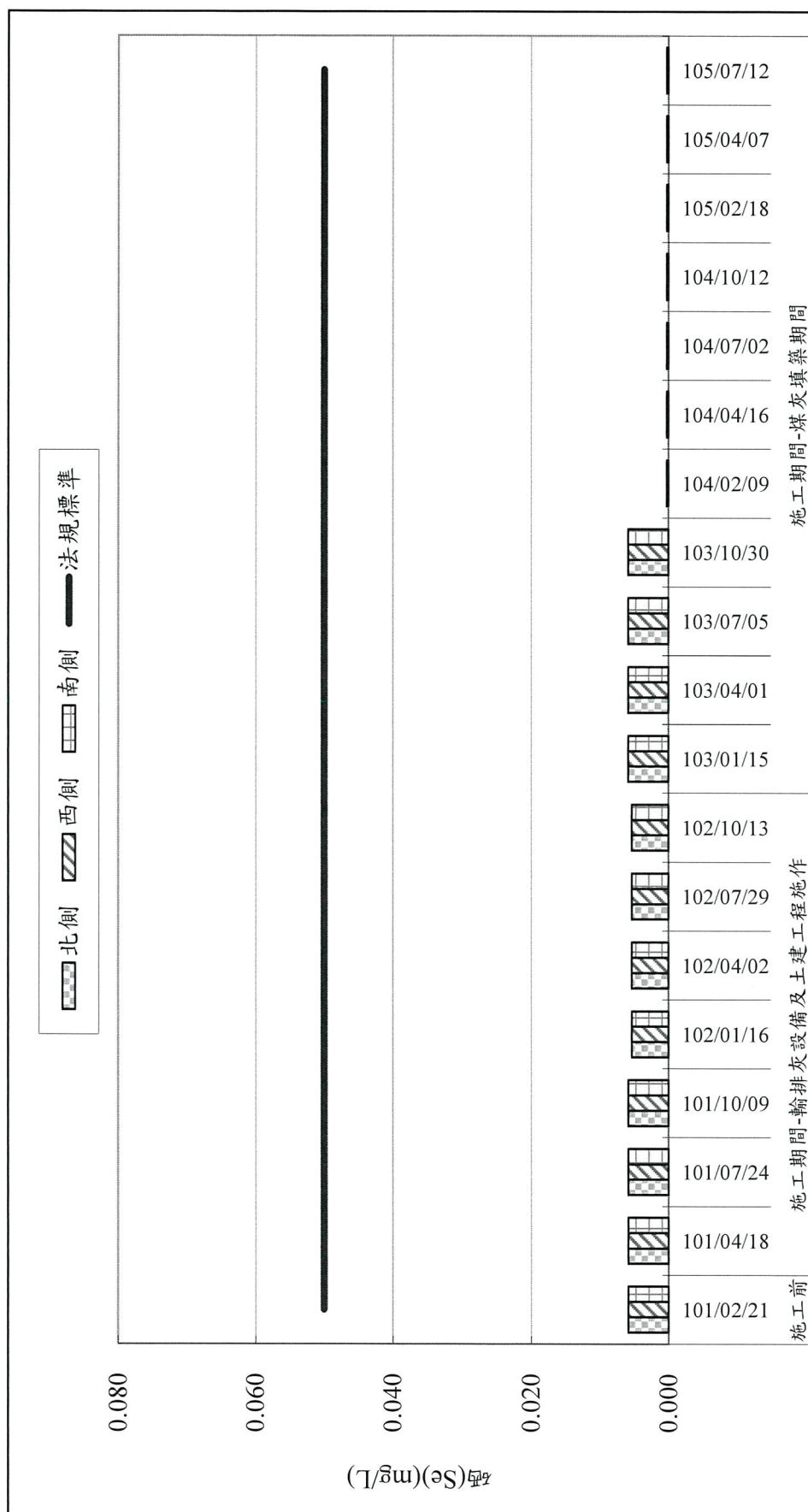
圖 2.2-8 歷季各測站硒(Se)監測成果彙整
