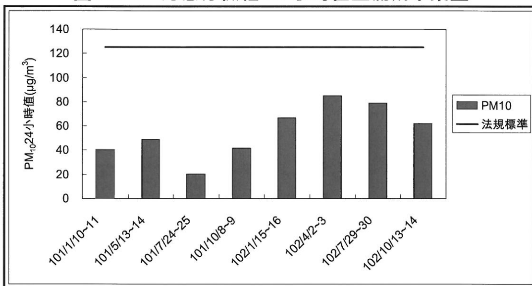
圖 2.1-2 粒徑 \leq 10\mu\text{m} 之懸浮微粒 24 小時值監測成果彙整
