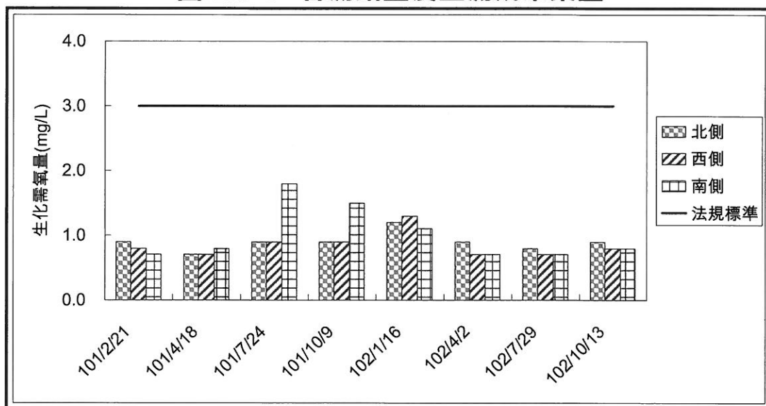
圖 2.2-5 各測站生化需氧量監測成果彙整
