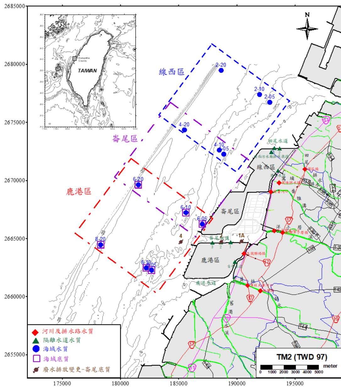
圖 1.4-11 彰濱工業區110年開發期間河川及排水路、隔離水道與海域水質(含底質)監測點位示意圖
