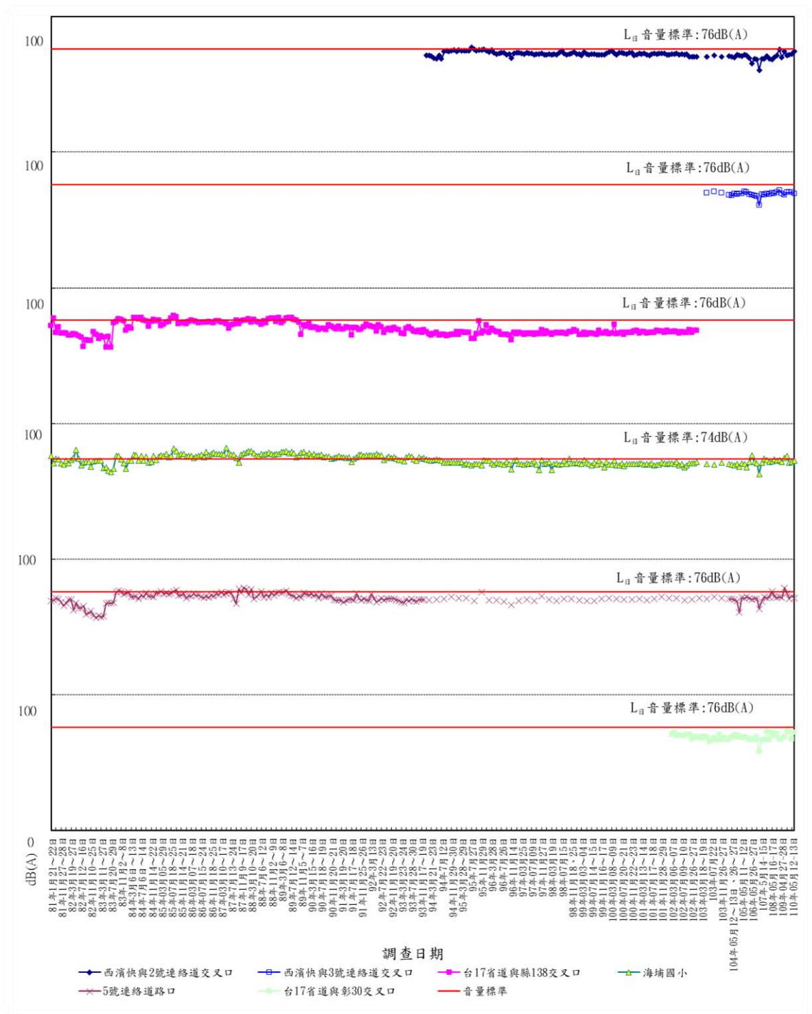
圖 3.1.2-1 彰濱地區歷次噪音 L d 監測結果
