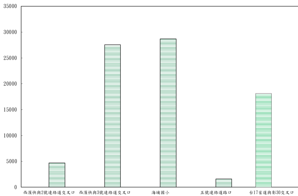
圖 2.4-1 本季各測站主要道路交通流量(PCU/日)調查結果分析圖
