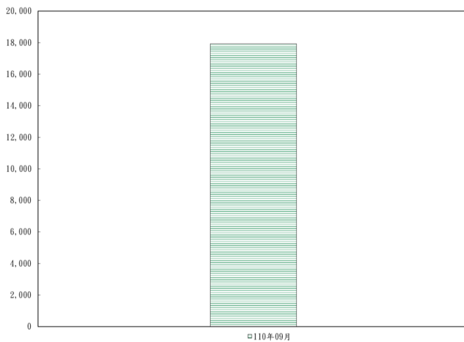
圖 2.4-2 彰濱工業區重要連絡道路本季交通流量(PCU/日)調查結果分析圖
