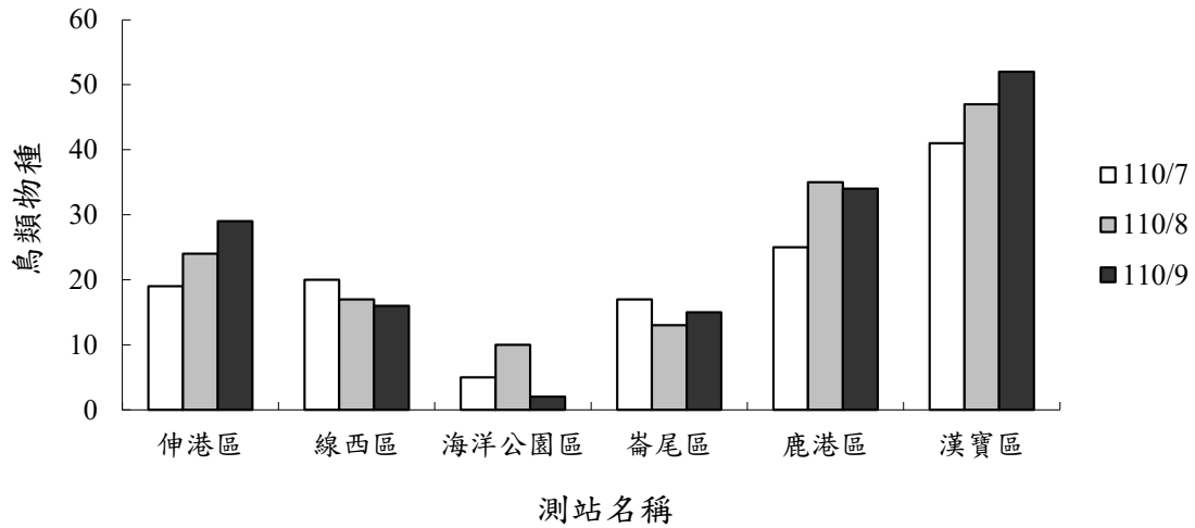
圖 2.5-1 本季各測站鳥類種數分布圖
