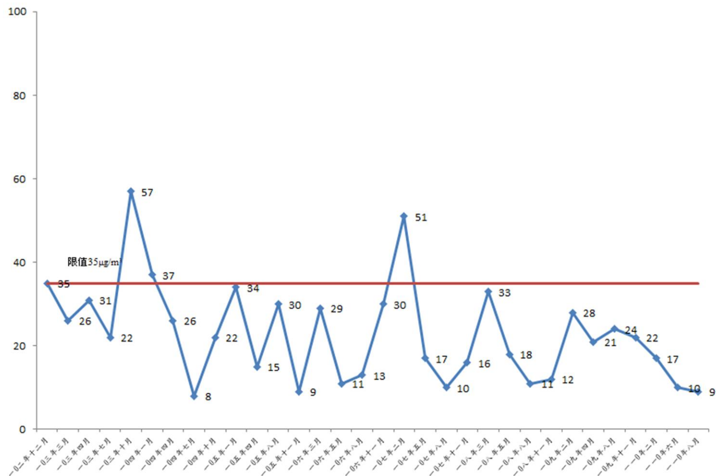
圖 3.1.1-8 彰濱地區-線工南一路歷年粒徑小於 2.5\mu\text{m} 之懸浮微粒(PM 2.5 )日平均值監測結果分析圖
