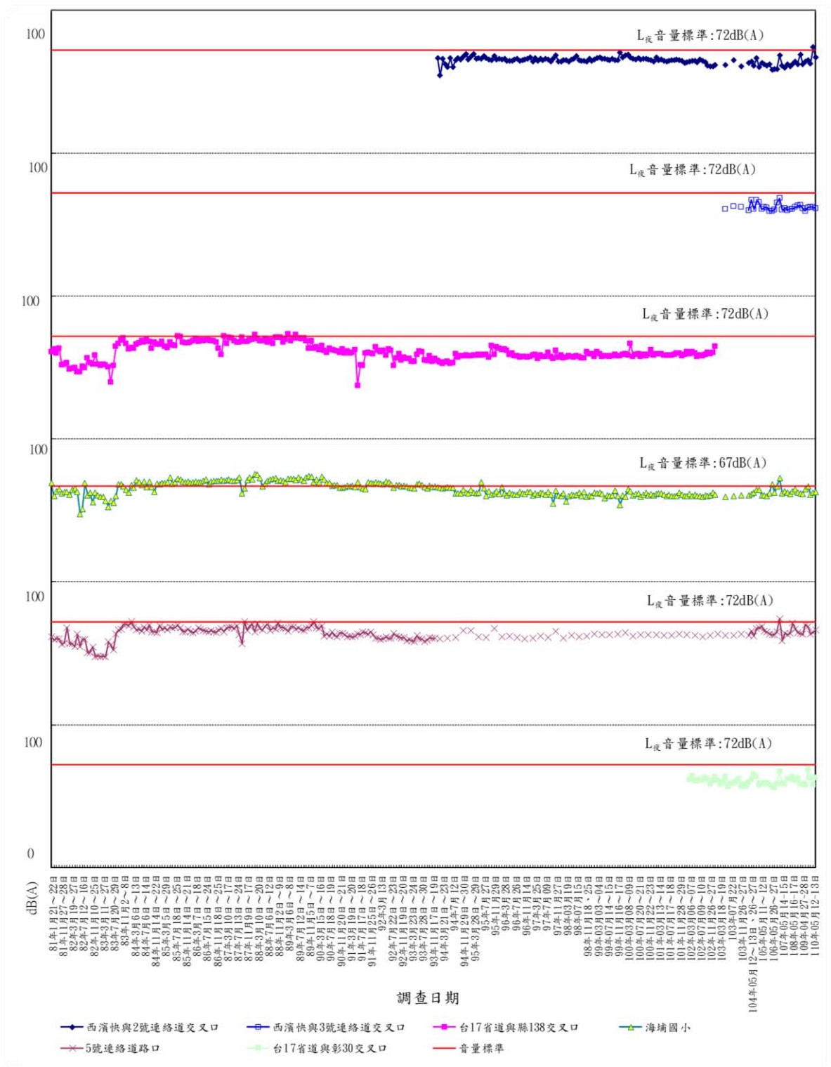
圖 3.1.2-3 彰濱地區歷次噪音 L 夜 監測結果
