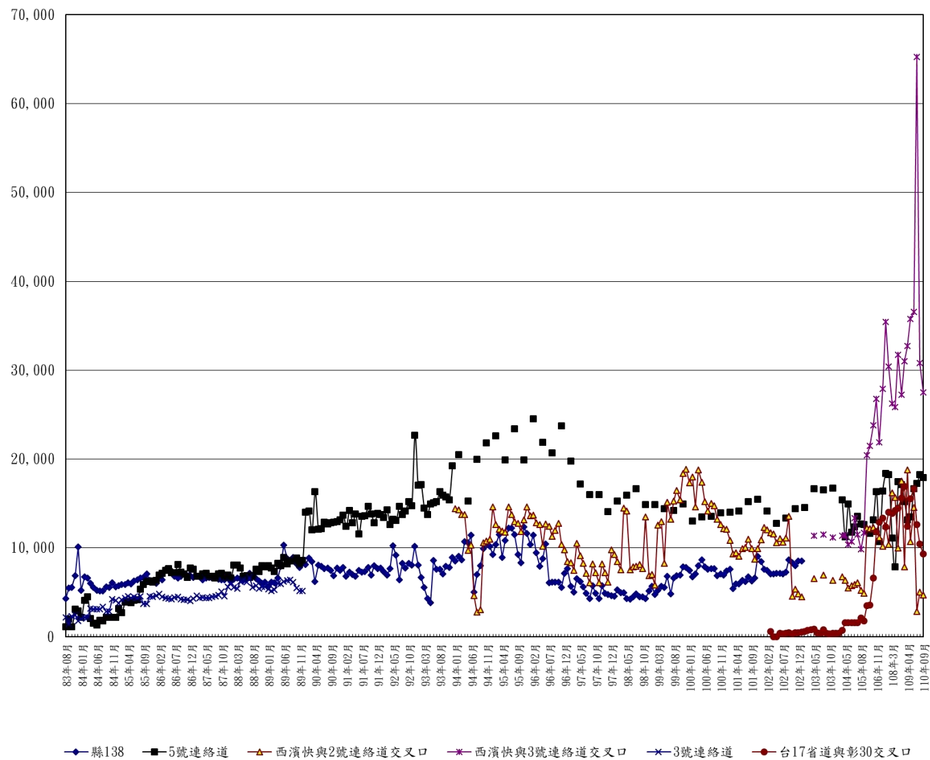
圖 3.1.4-1 彰濱地區歷次交通流量監測結果(2/2)
