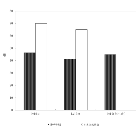
圖 2.3-1 西濱快與 2 號連絡道交叉口本季振動調查結果分析圖
