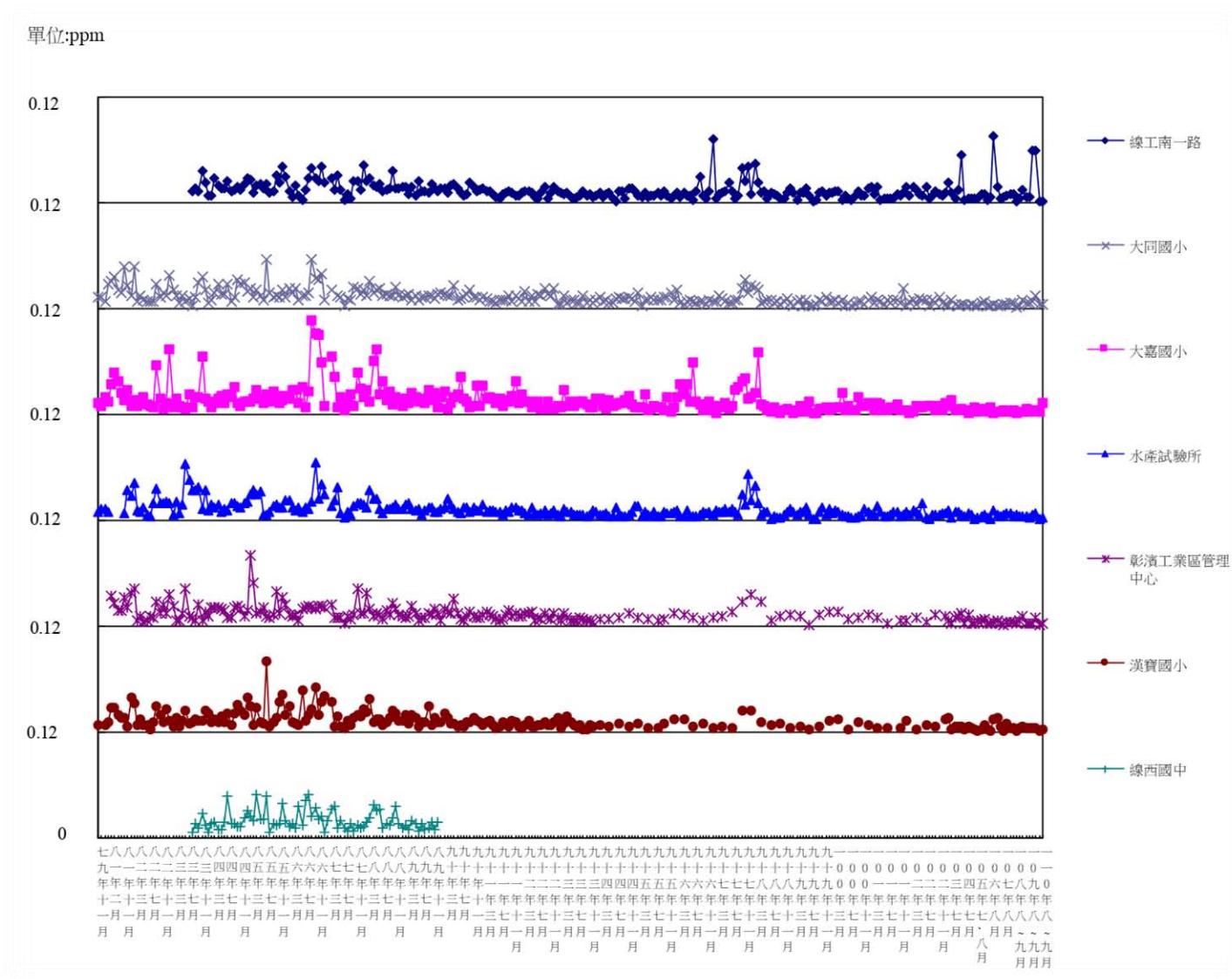
圖 3.1.1-2 彰濱地區歷年二氧化硫(SO 2 )最高小時值監測結果分析圖
