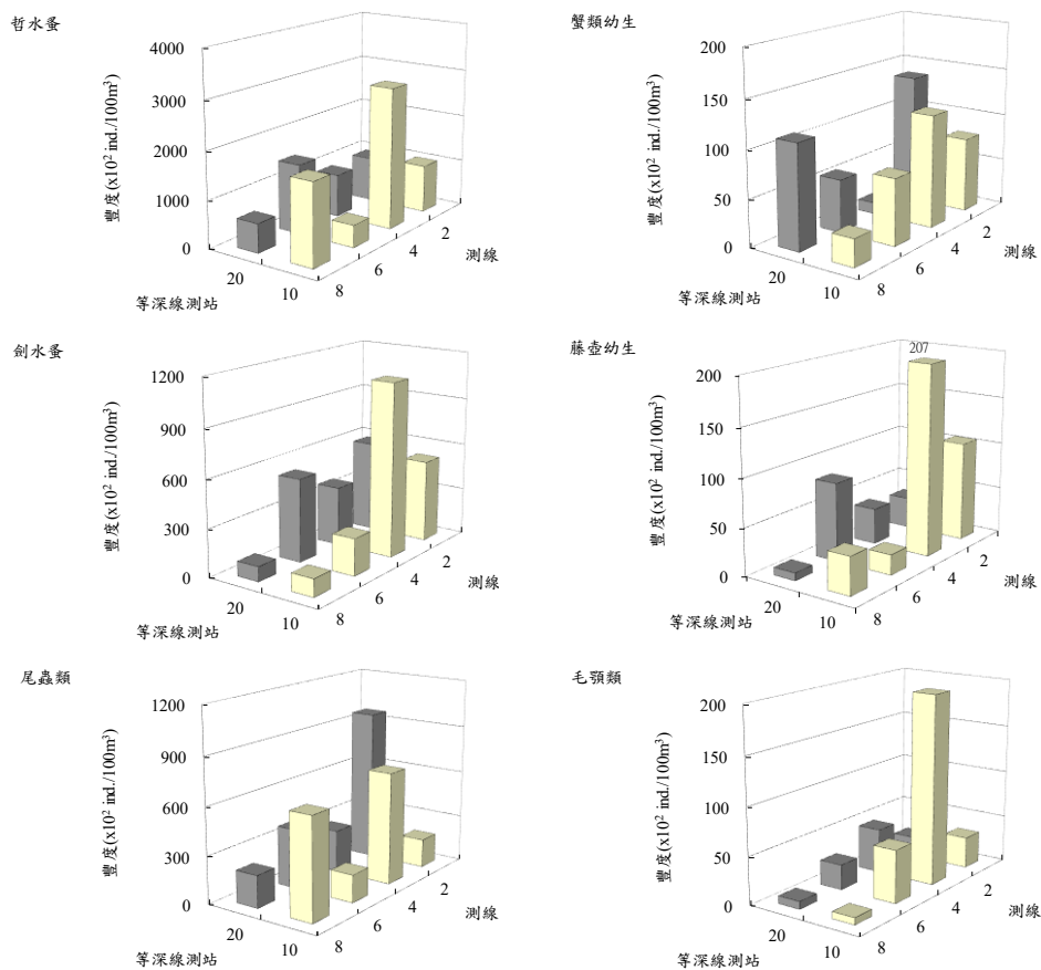
圖 2.10.2-2 民國 110 年 7 月彰化濱海工業區附近海域浮游動物主要優勢類群之豐度分布圖
