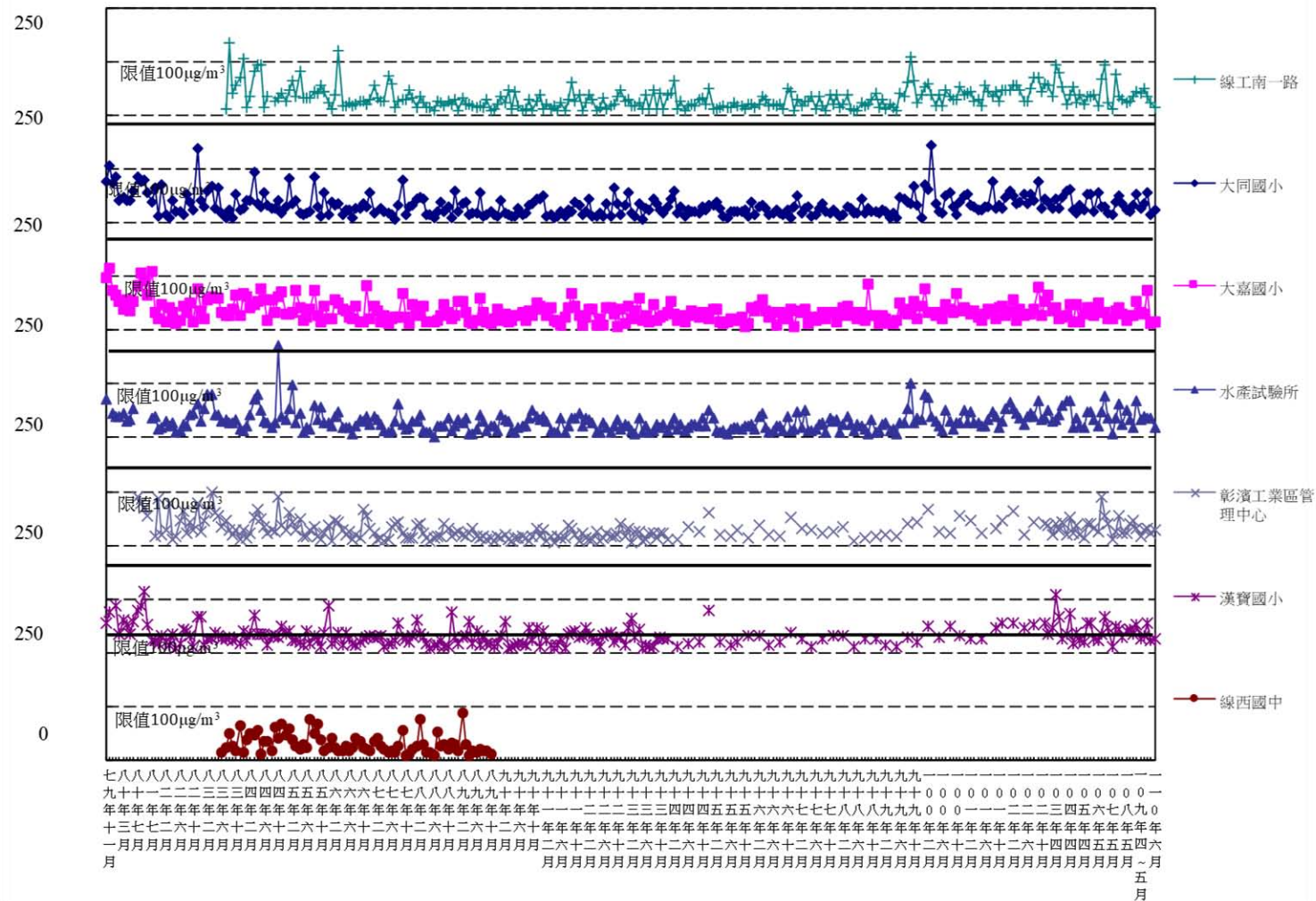
圖 3.1.1-7 彰濱地區歷年粒徑小於 10\mu\text{m} 之懸浮微粒(PM 10 )日平均值監測結果分析圖
