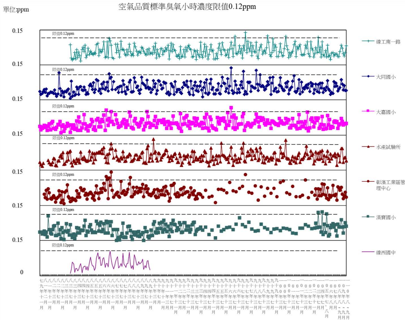
圖 3.1.1-4 彰濱地區歷年臭氧(O 3 )最高小時值監測結果分析圖
