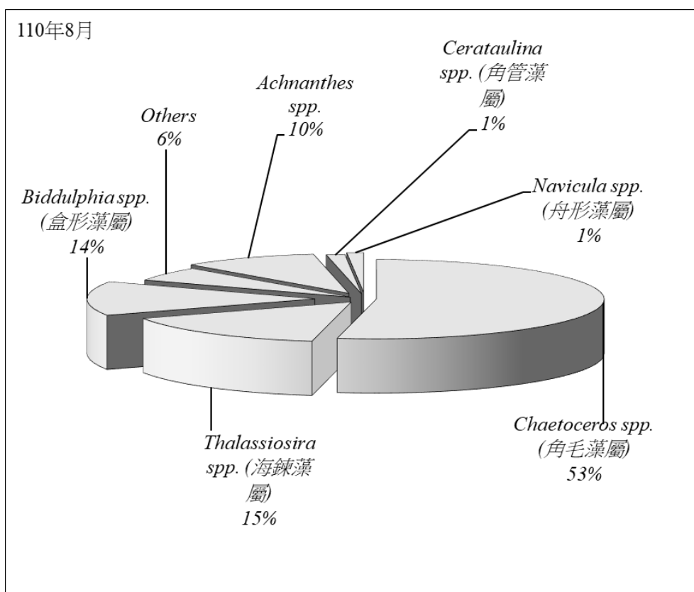
圖 2.10.1-1 民國 110 年 8 月於彰化濱海工業區附近海域各測站之浮游植物豐度分析圖
