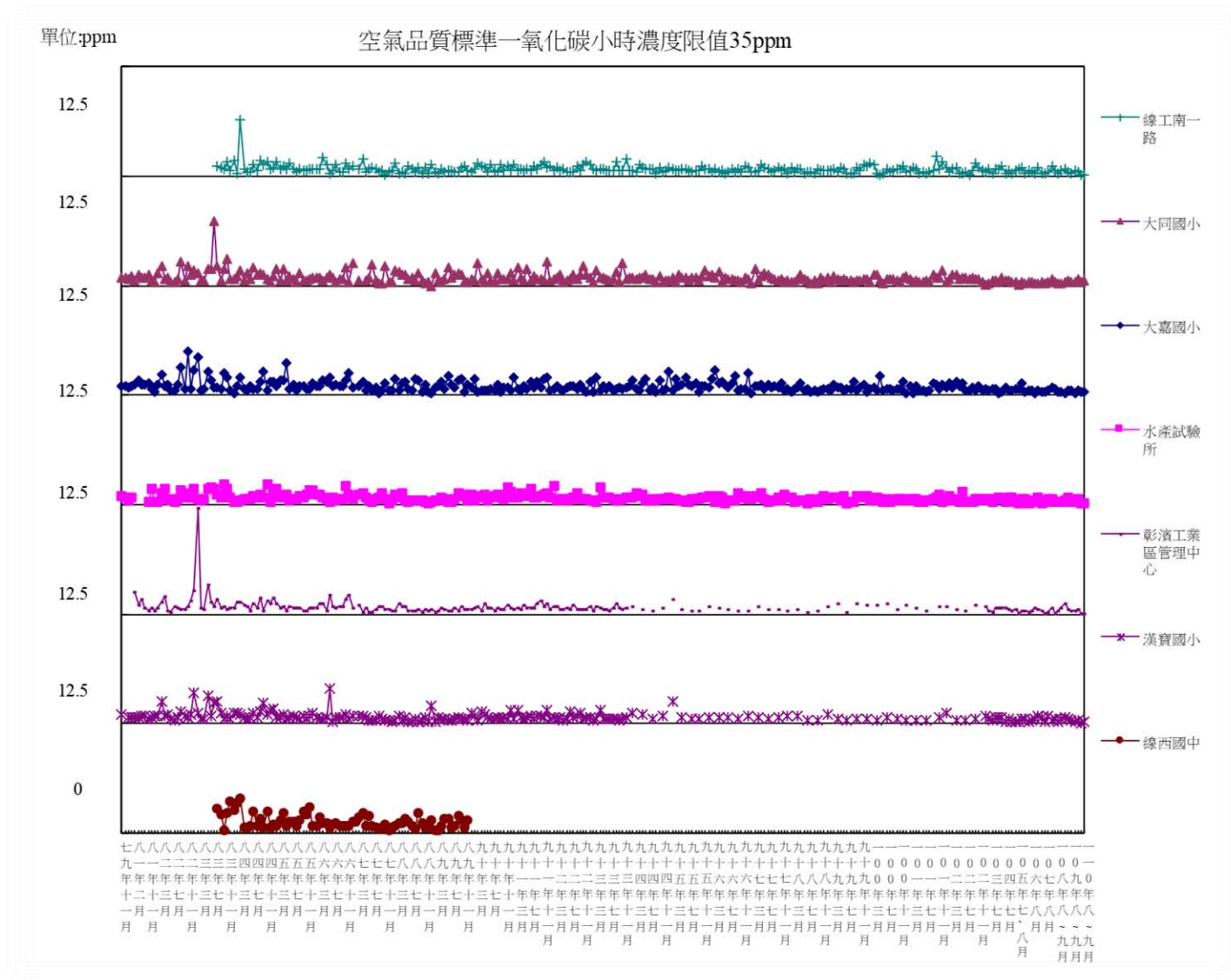
圖 3.1.1-1 彰濱地區歷年一氧化碳(CO)最高小時值監測結果分析圖
