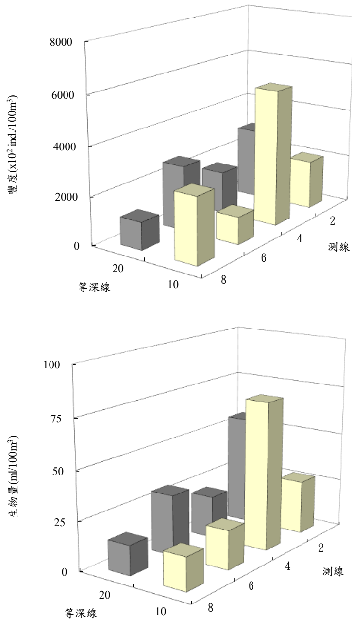
圖 2.10.2-1 民國 110 年 7 月彰化濱海工業區附近海域浮游動物之豐度及生物量分布圖
