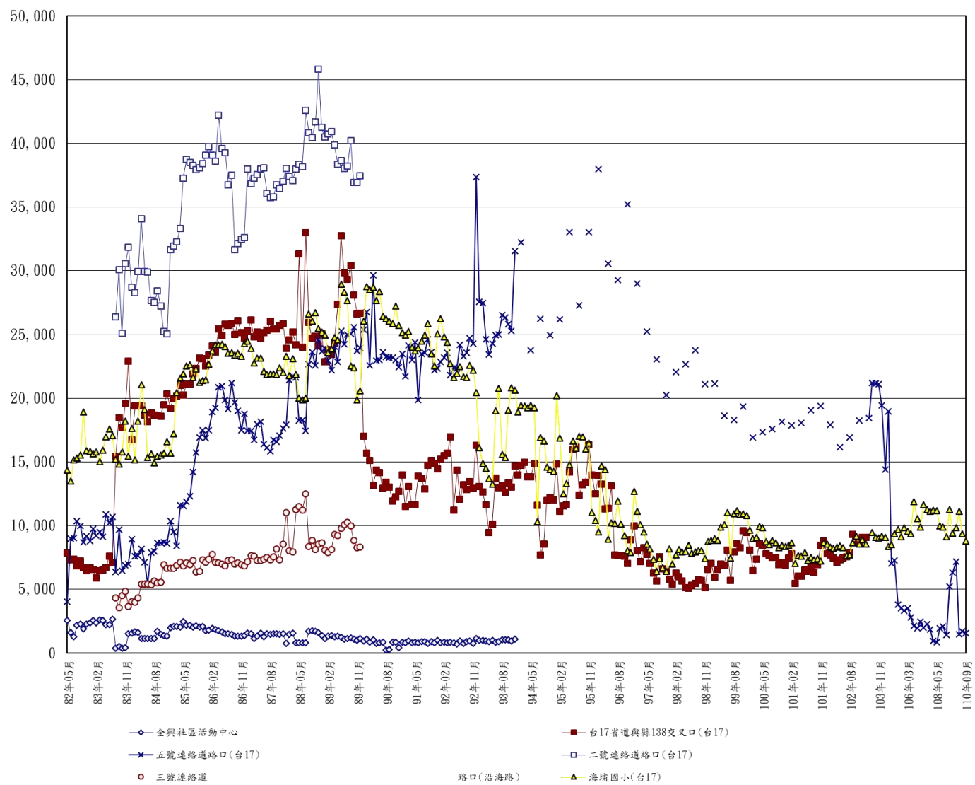
圖 3.1.4-1 彰濱地區歷次交通流量監測結果(1/2)
