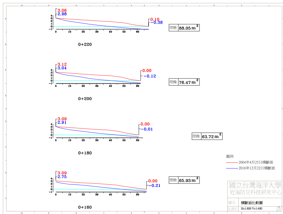
圖 4-4(h) 2016 年 12 月 22 日 A 監測區橫斷面比較圖
