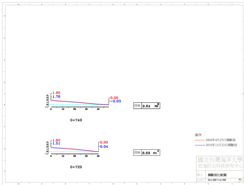
圖 4-4(a) 2016 年 12 月 22 日 A 監測區橫斷面比較圖
