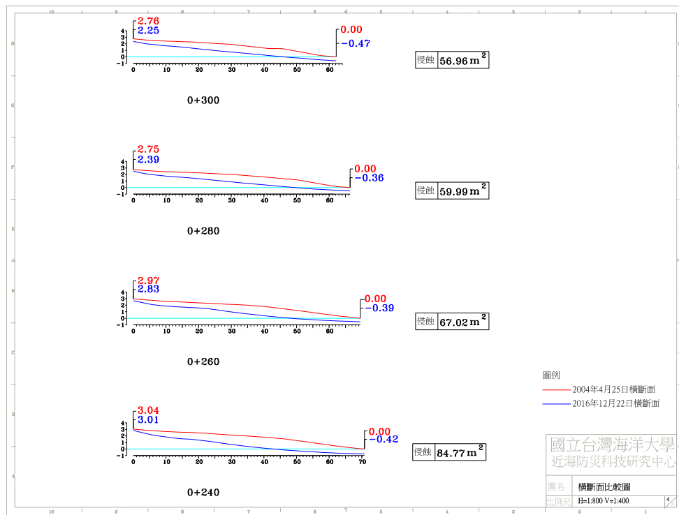
圖 4-4(g) 2016 年 12 月 22 日 A 監測區橫斷面比較圖
