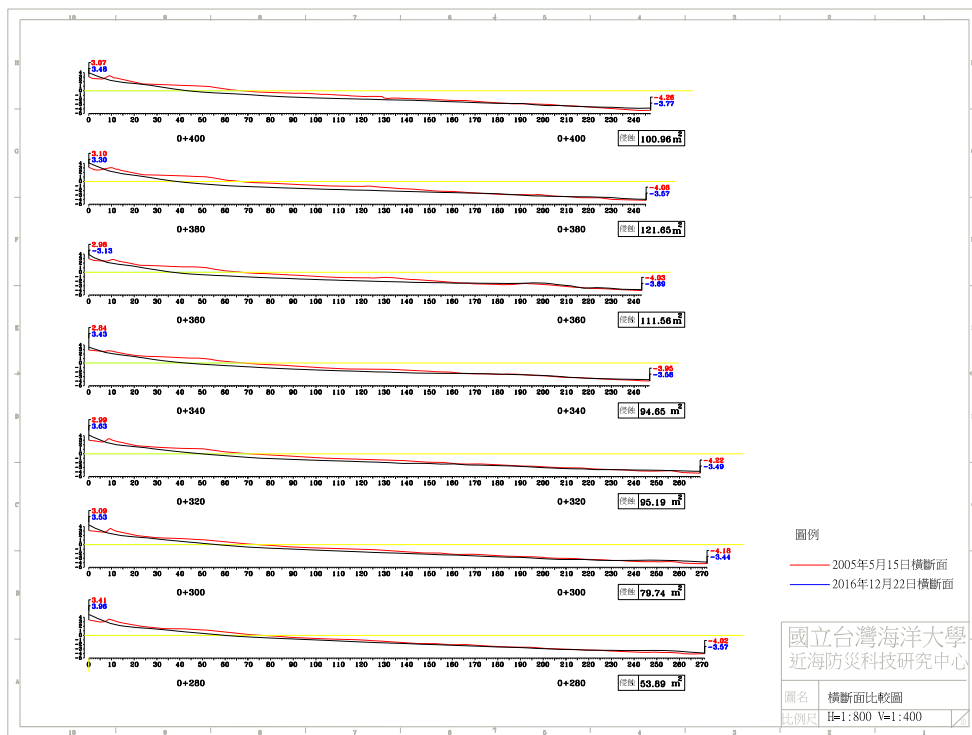
圖 4-5(d) 2016 年 12 月 22 日 B 監測區橫斷面比較圖
