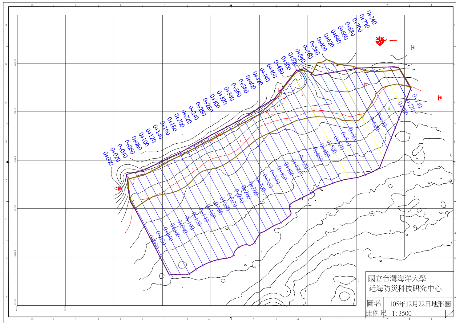
圖 4-1 2016 年 12 月 22 日監測地形圖
