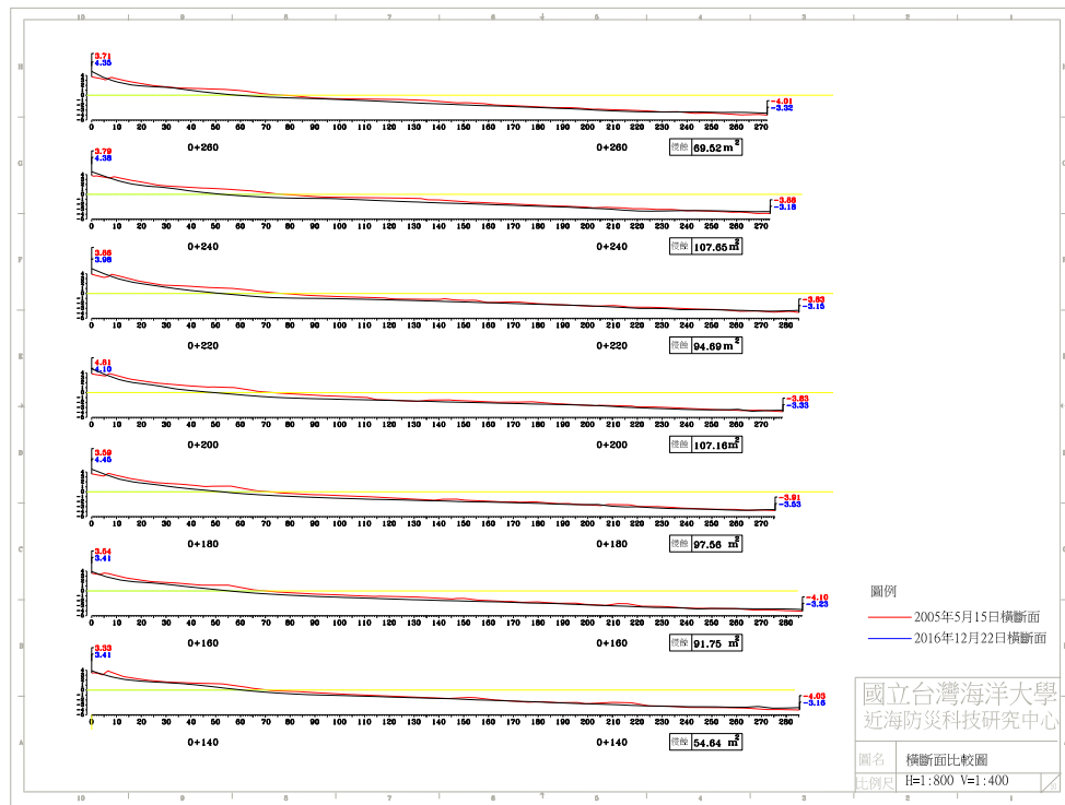
圖 4-5(e) 2016 年 12 月 22 日 B 監測區橫斷面比較圖
