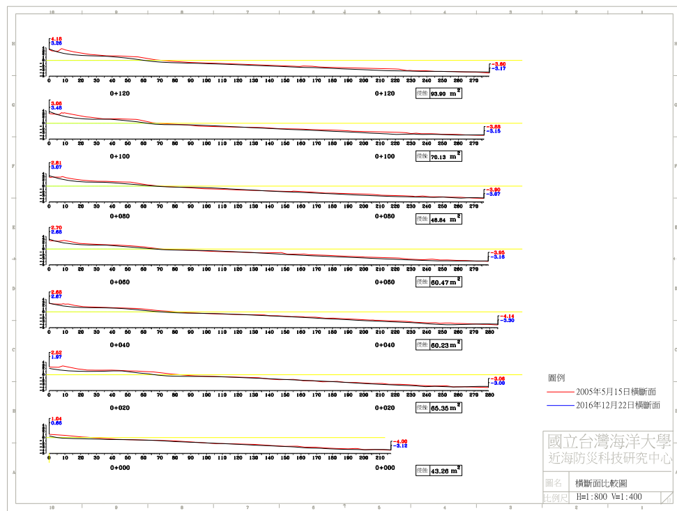
圖 4-5(f) 2016 年 12 月 22 日 B 監測區橫斷面比較圖
