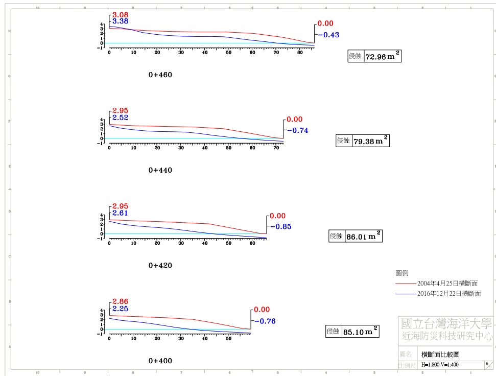
圖 4-4(e) 2016 年 12 月 22 日 A 監測區橫斷面比較圖
