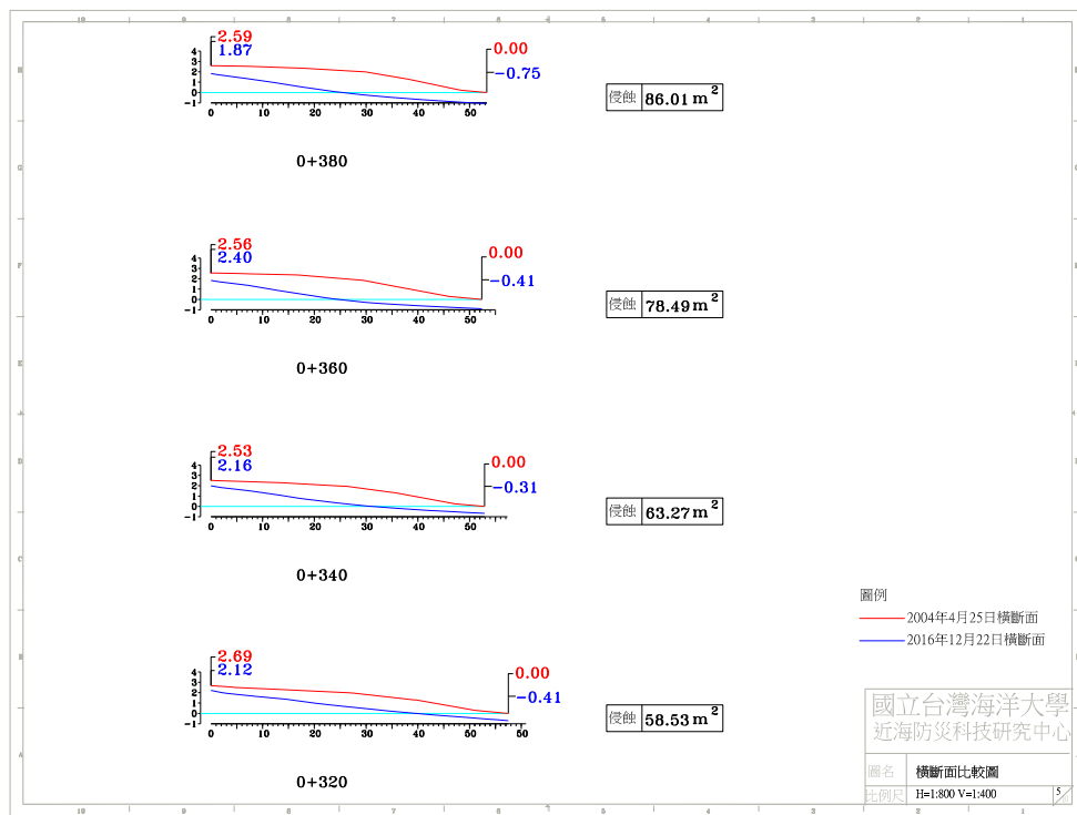
圖 4-4(f) 2016 年 12 月 22 日 A 監測區橫斷面比較圖
