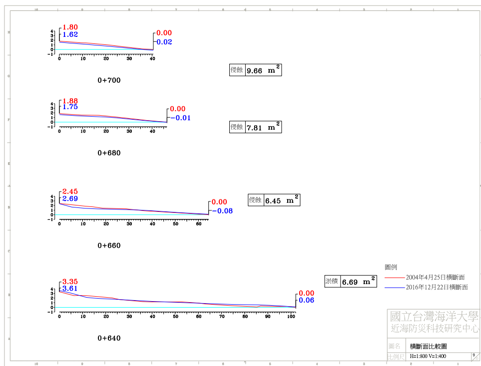
圖 4-4(b) 2016 年 12 月 22 日 A 監測區橫斷面比較圖
