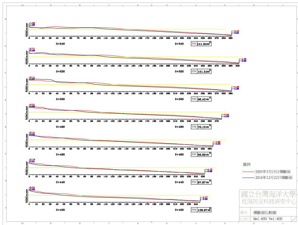
圖 4-5(c) 2016 年 12 月 22 日 B 監測區橫斷面比較圖
