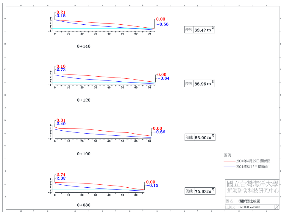
圖 4-4(j) 2021 年 8 月 2 日 A 監測區橫斷面比較圖
