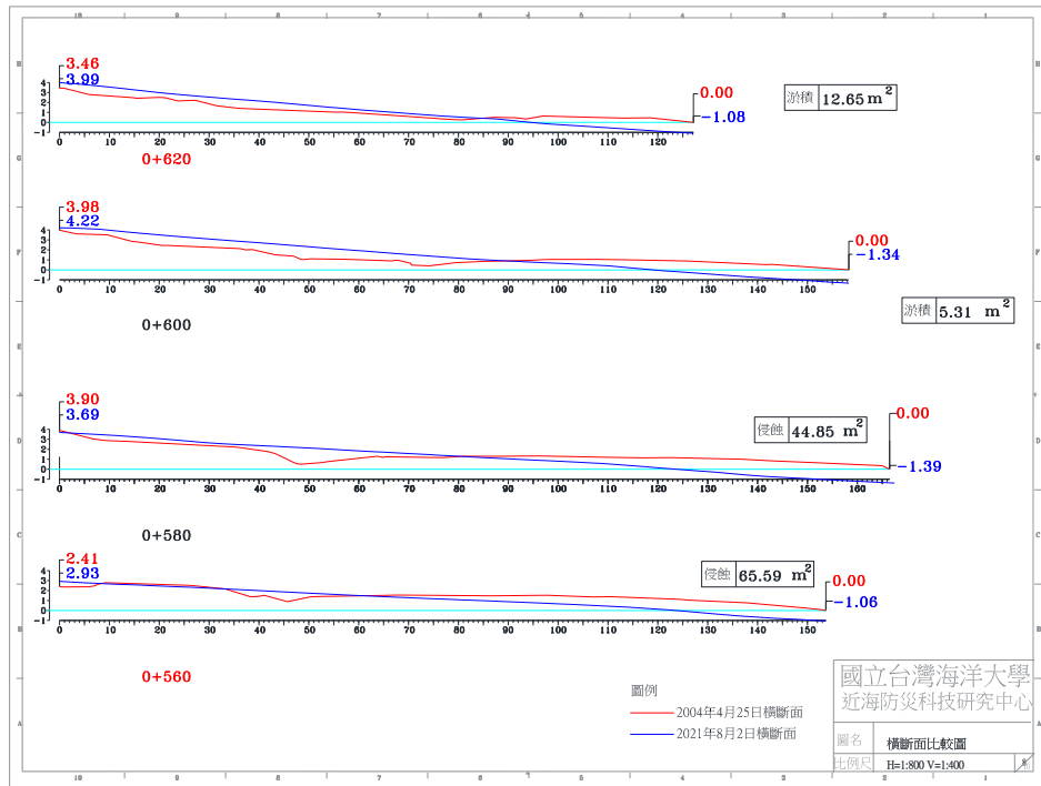
圖 4-4(c) 2021 年 8 月 2 日 A 監測區橫斷面比較圖
