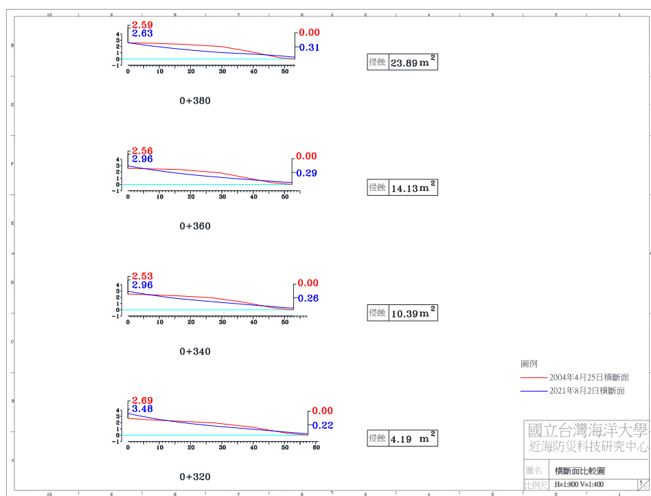
圖 4-4(f) 2021 年 8 月 2 日 A 監測區橫斷面比較圖
