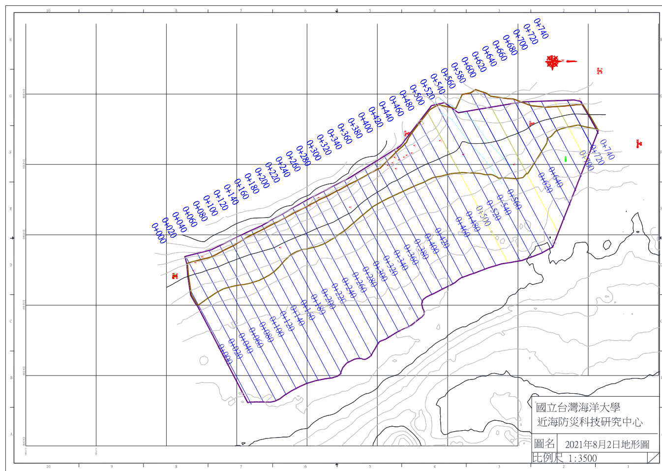
圖 4-1 2021 年 8 月 2 日監測地形圖
