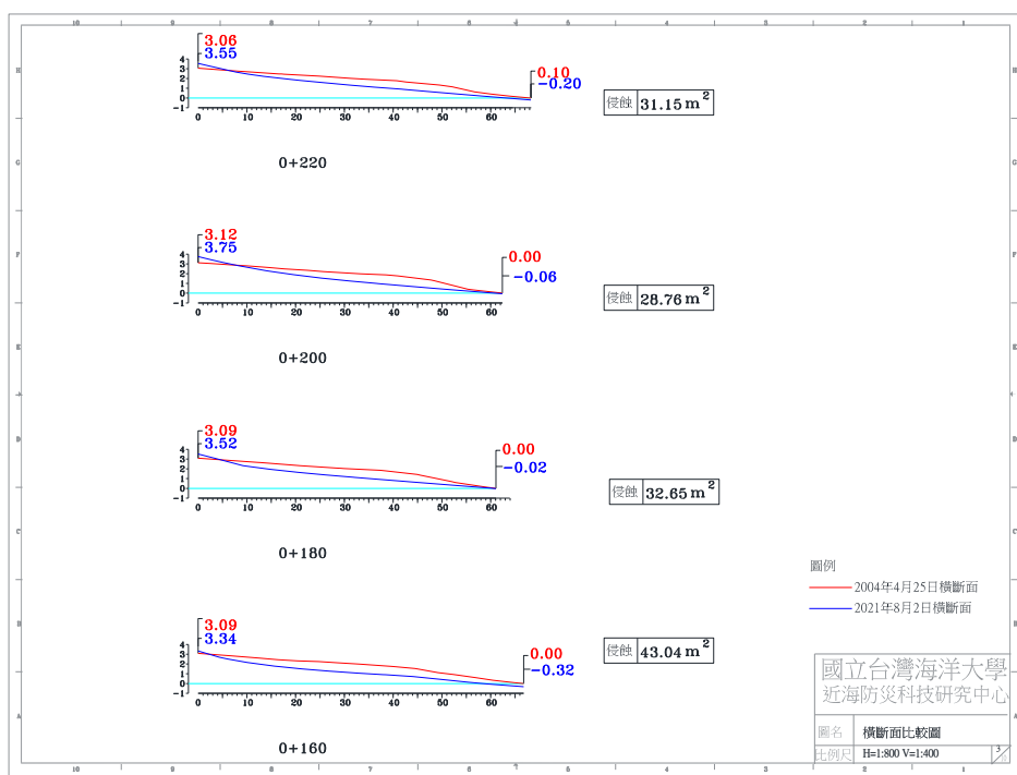
圖 4-4(i) 2021 年 8 月 2 日 A 監測區橫斷面比較圖
