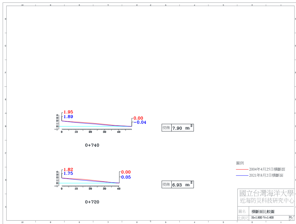
圖 4-4(a) 2021 年 8 月 2 日 A 監測區橫斷面比較圖
