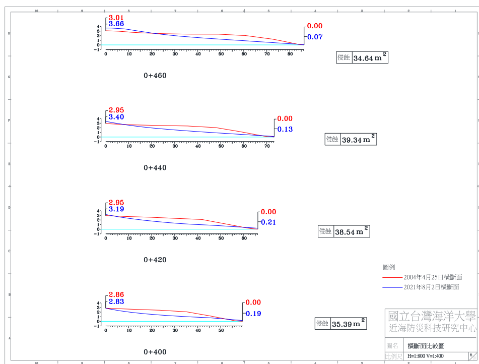
圖 4-4(e) 2021 年 8 月 2 日 A 監測區橫斷面比較圖
