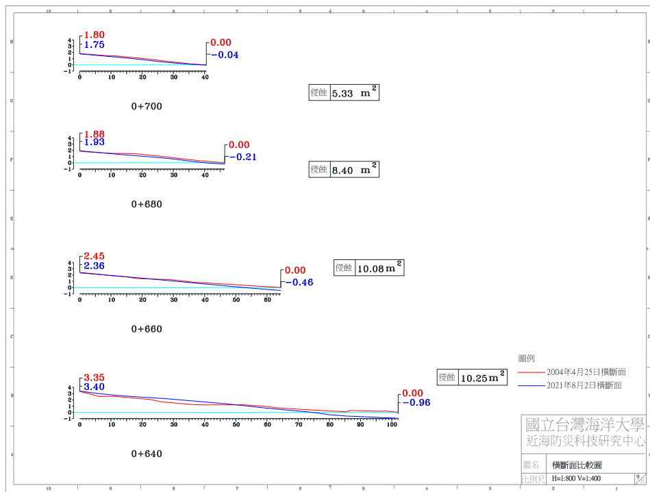
圖 4-4(b) 2021 年 8 月 2 日 A 監測區橫斷面比較圖
