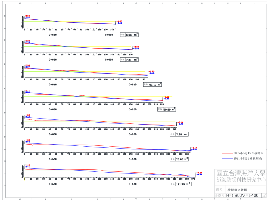
圖 4-5(b) 2021 年 8 月 2 日 B 監測區橫断面比較圖
