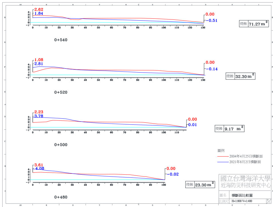
圖 4-4(d) 2021 年 8 月 2 日 A 監測區橫斷面比較圖
