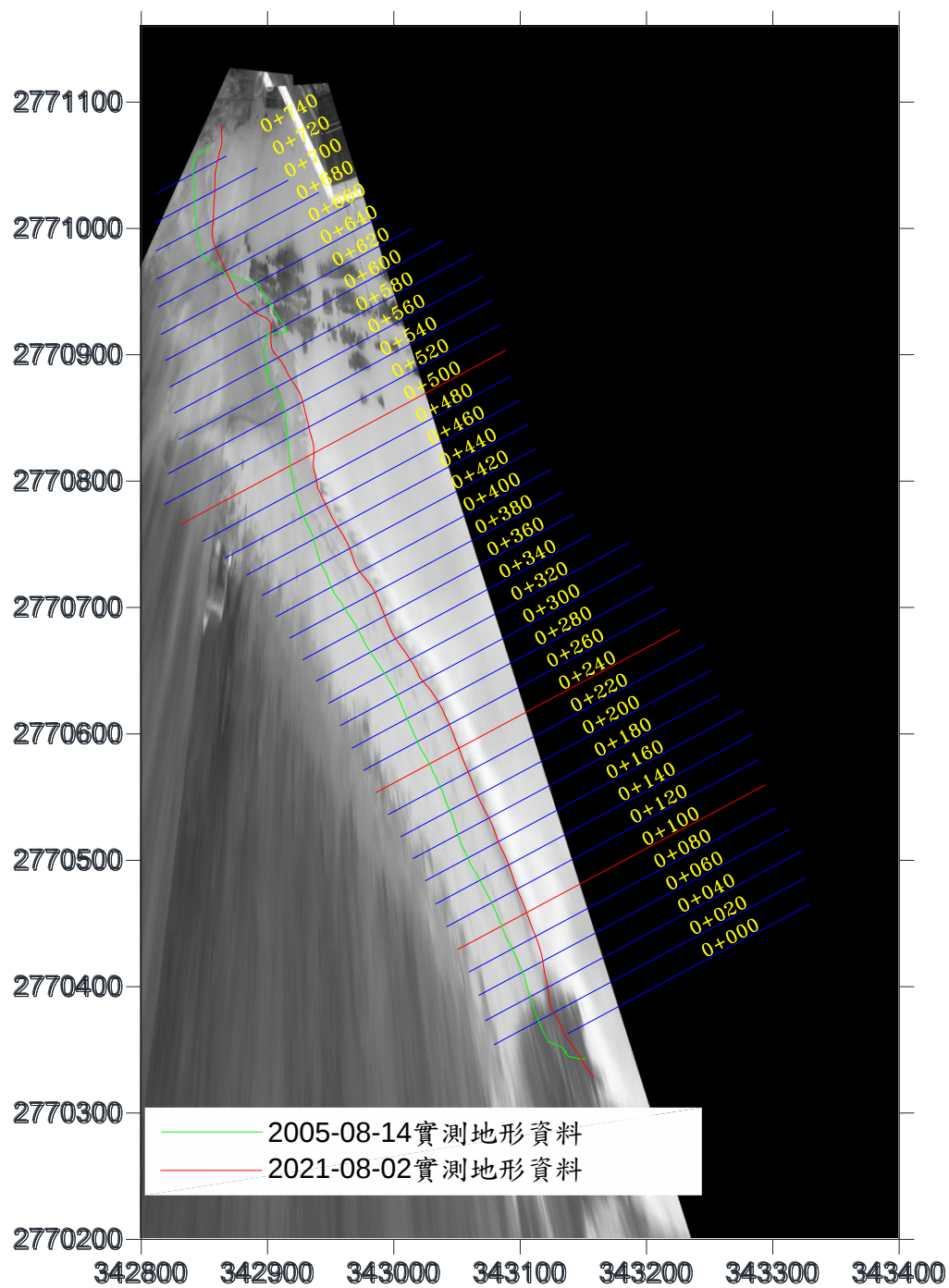
圖 4-22 實測地形水位線分析結果圖(2021/08/02)
