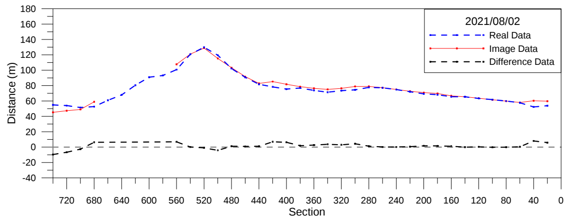
圖 3-23 海岸線分析比較圖(2021/08/02)
