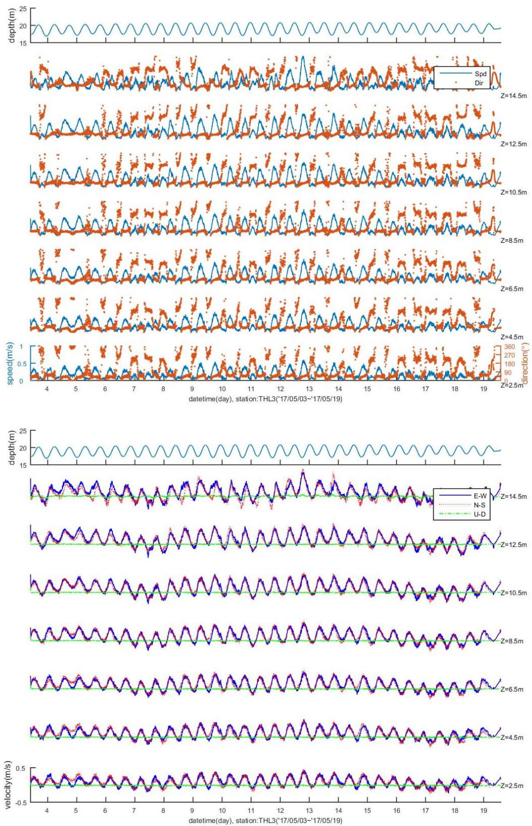
附錄III.11圖-2 THL3流速、流向、南北向、東西向速度分量逐時變化圖
