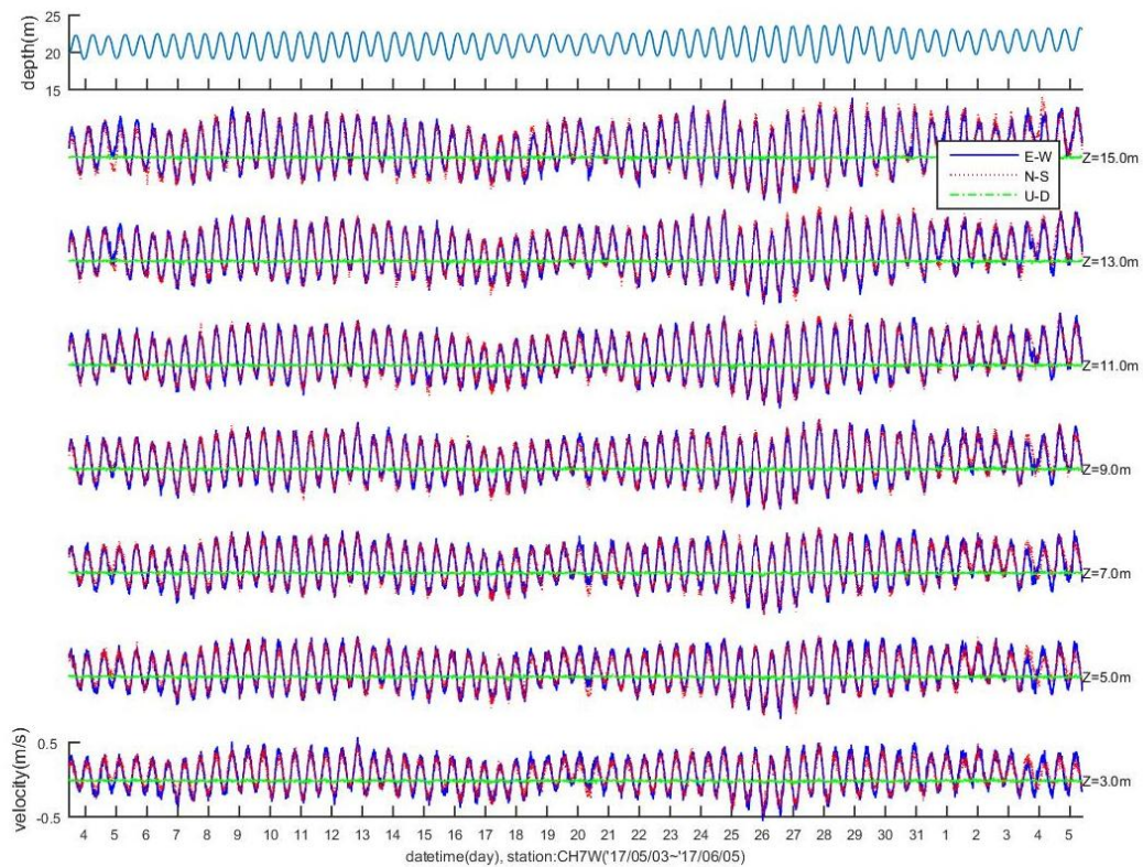
附錄III.11圖-1 CH7W流速、流向、南北向、東西向速度分量逐時變化圖
