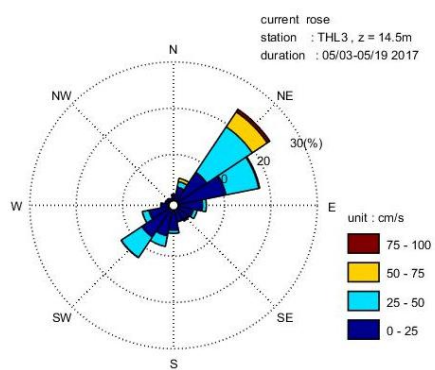
附錄III.11圖-6 THL3流速流向玫瑰圖
