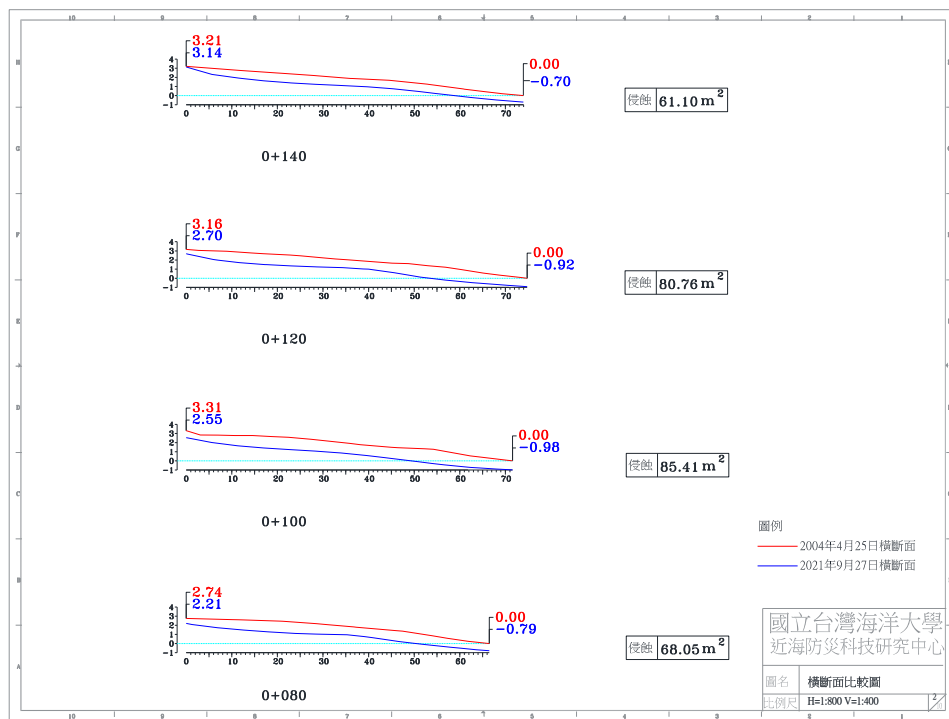
圖 4-4(i) 2021 年 9 月 27 日 A 監測區橫斷面比較圖
