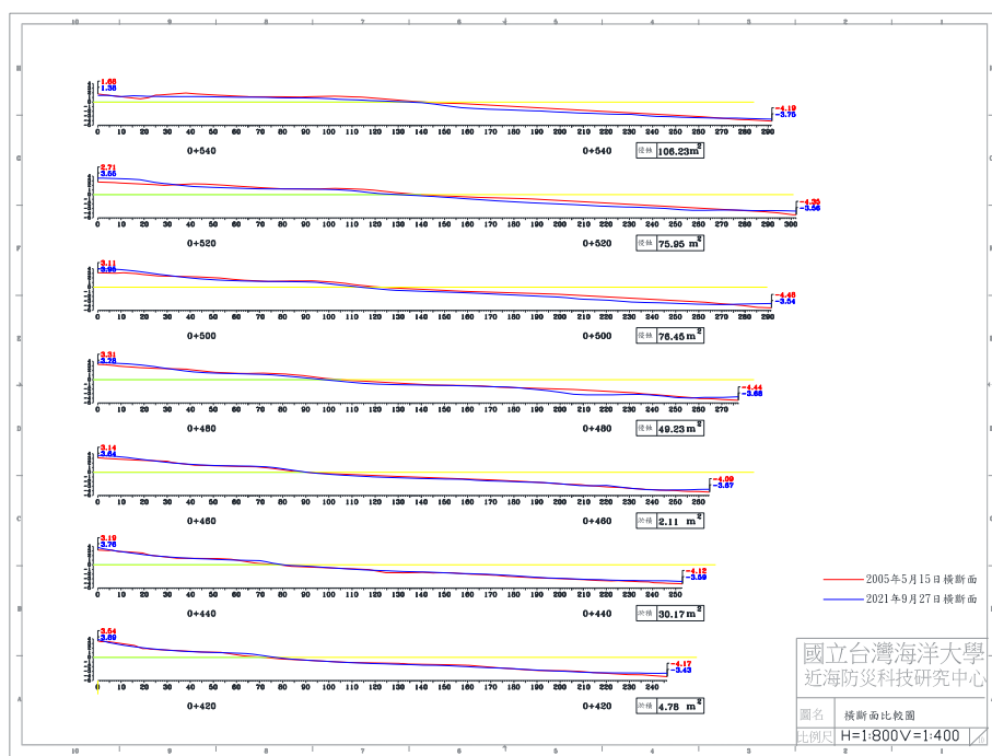
圖 4-5(c) 2021 年 9 月 27 日 B 監測區橫斷面比較圖
