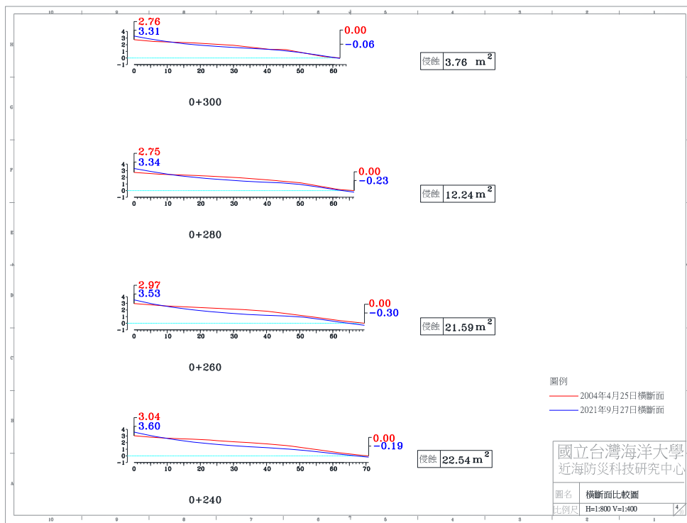
圖 4-4(g) 2021 年 9 月 27 日 A 監測區橫斷面比較圖
