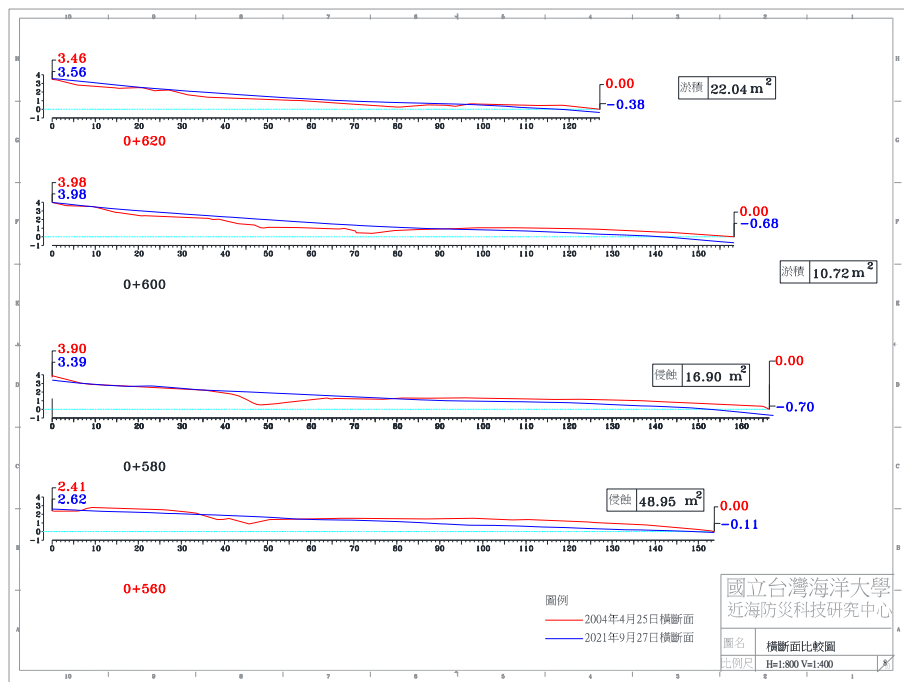
圖 4-4(c) 2021 年 9 月 27 日 A 監測區橫斷面比較圖
