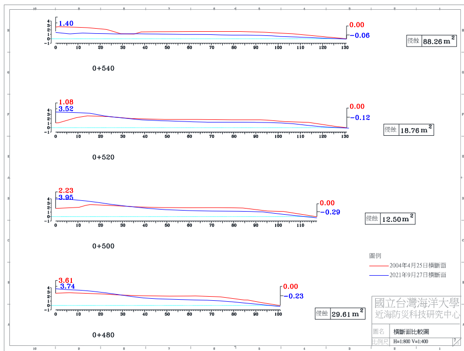
圖 4-4(d) 2021 年 9 月 27 日 A 監測區橫斷面比較圖
