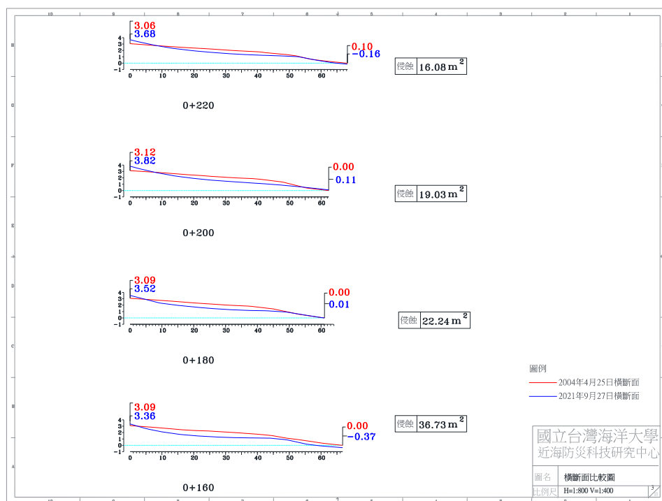
圖 4-4(h) 2021 年 9 月 27 日 A 監測區橫斷面比較圖
