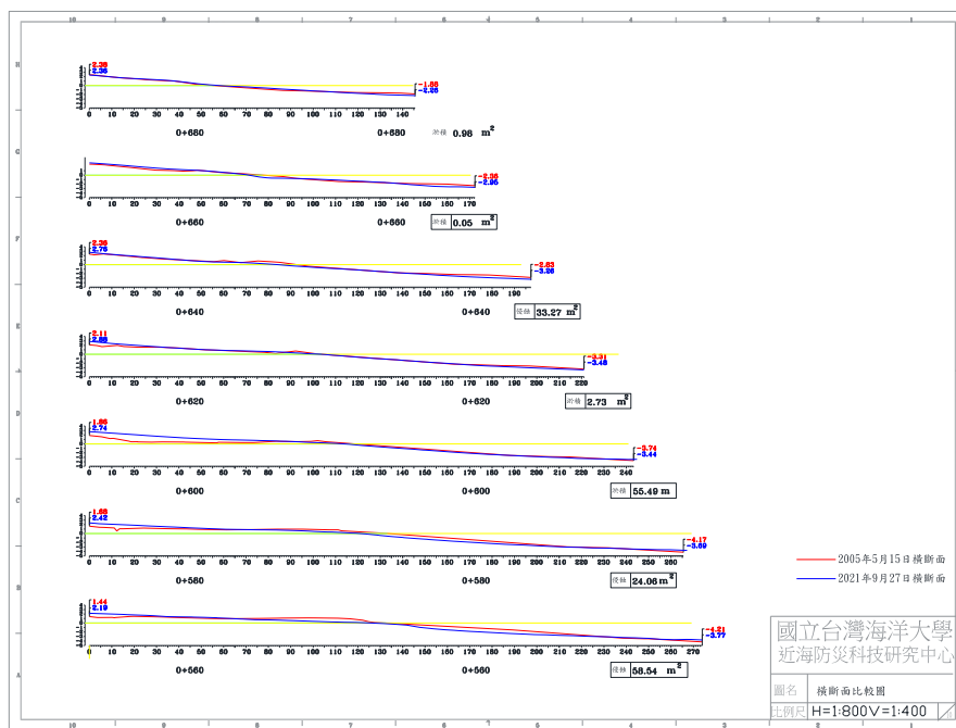
圖 4-5(b) 2021 年 9 月 27 日 B 監測區橫斷面比較圖
