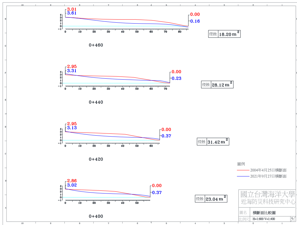
圖 4-4(e) 2021 年 9 月 27 日 A 監測區橫斷面比較圖
