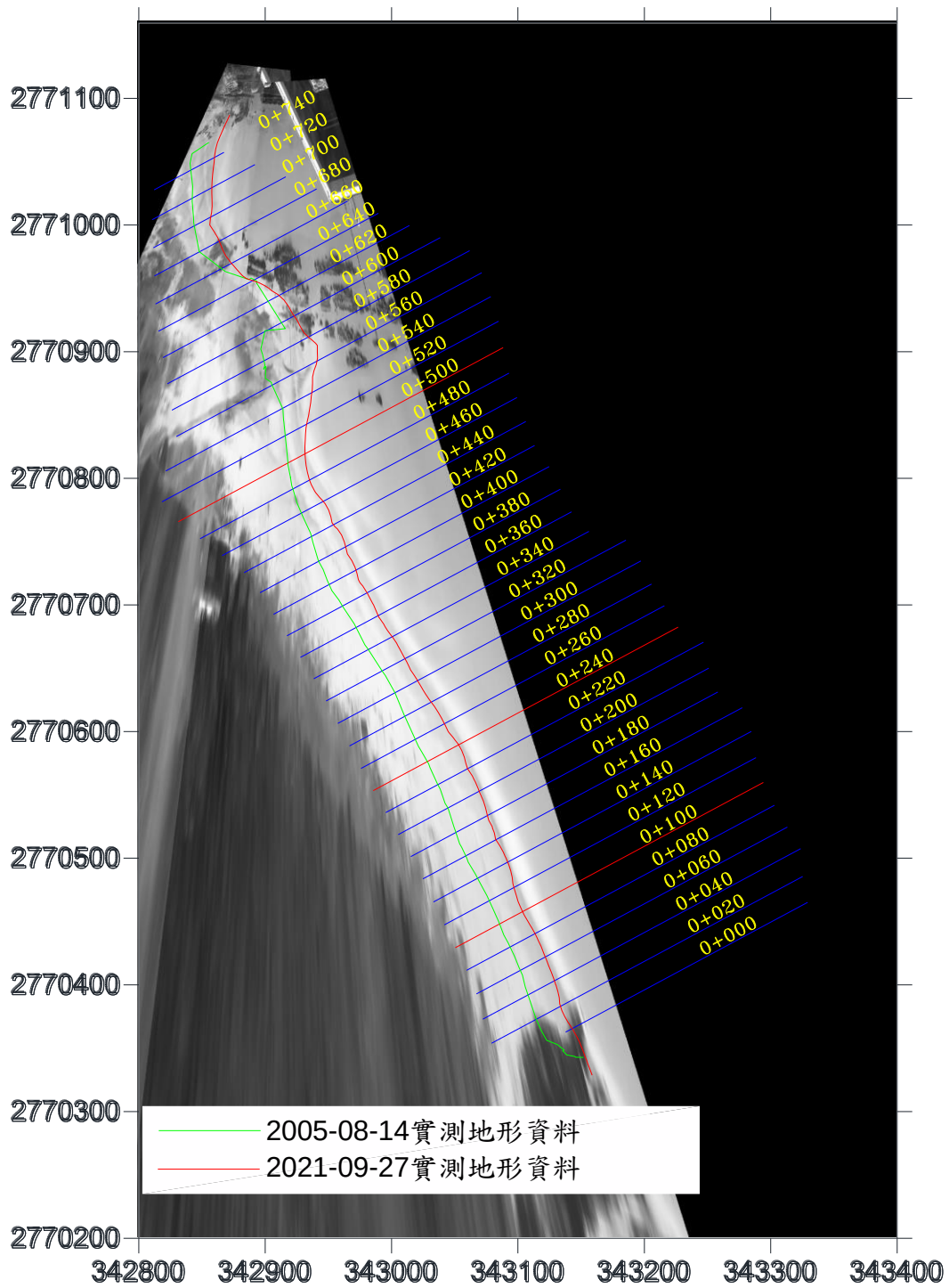
圖 4-22 實測地形水位線分析結果圖(2021/09/27)
