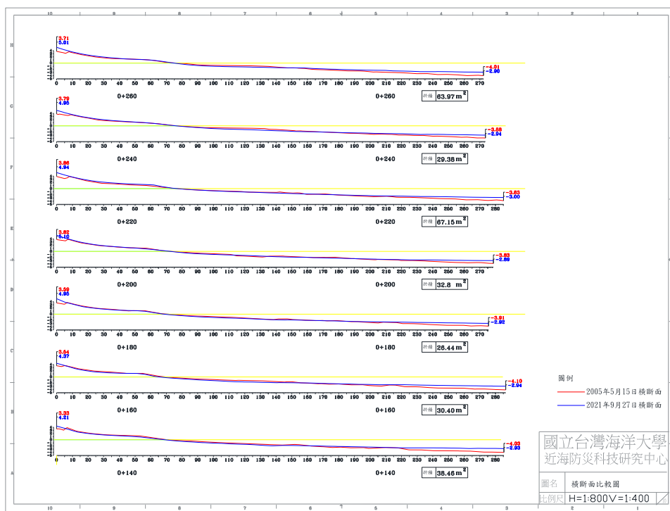
圖 4-5(e) 2021 年 9 月 27 日 B 監測區橫断面比較圖
