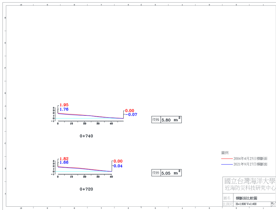
圖 4-4(a) 2021 年 9 月 27 日 A 監測區橫斷面比較圖
