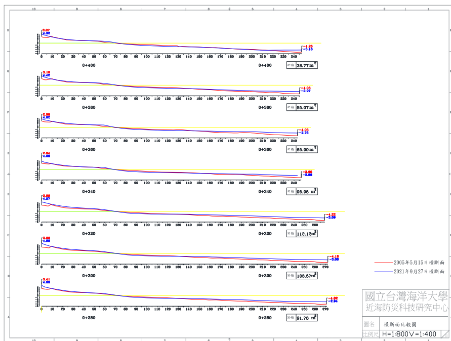
圖 4-5(d) 2021 年 9 月 27 日 B 監測區橫斷面比較圖
