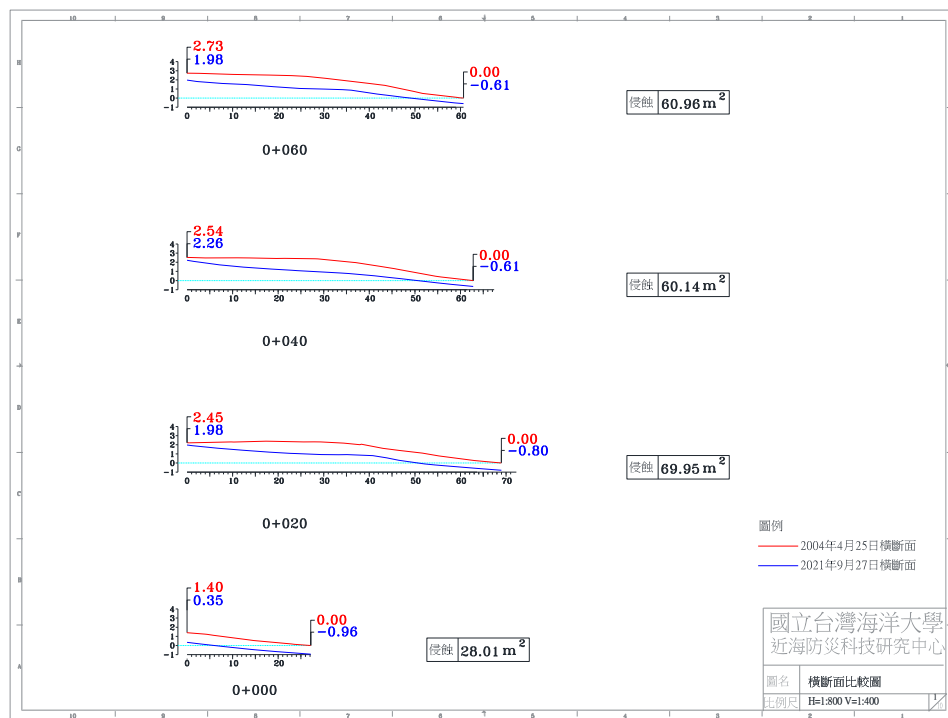
圖 4-4(j) 2021 年 9 月 27 日 A 監測區橫斷面比較圖
