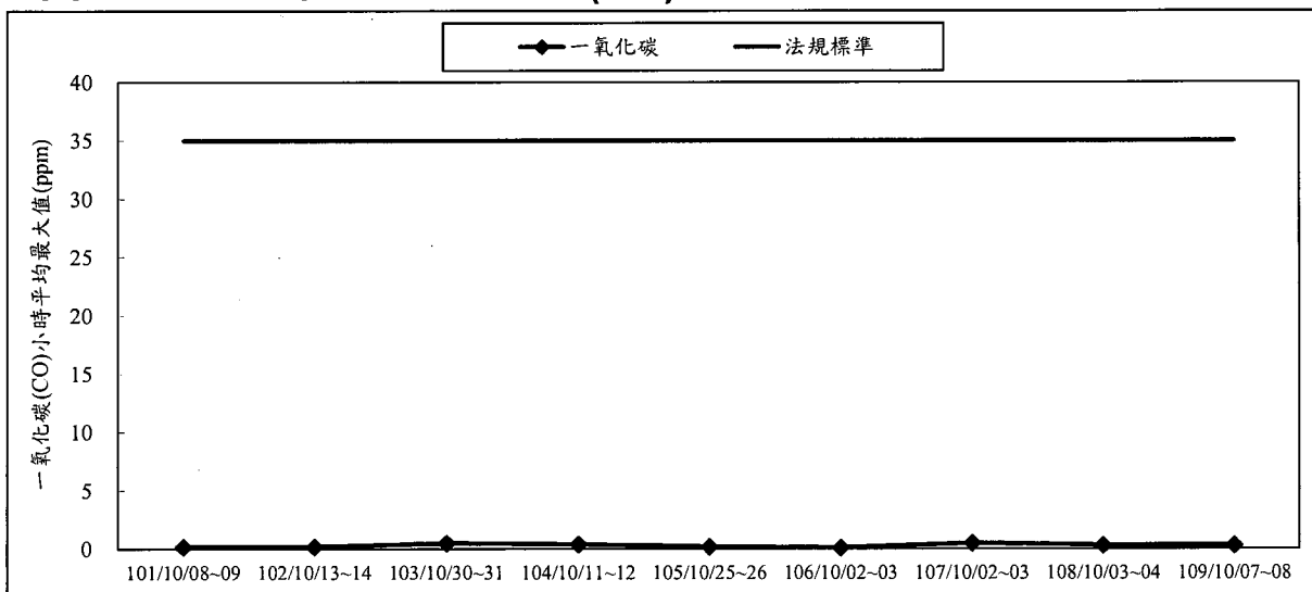
圖 3.1-8 歷年同期一氧化碳(CO)小時平均最大值監測成果彙整
