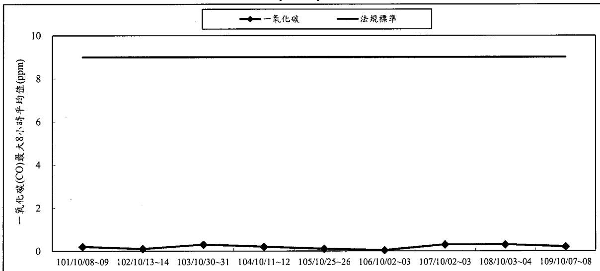
圖 3.1-7 歷年同期一氧化碳(CO)最大 8 小時平均值監測成果彙整
