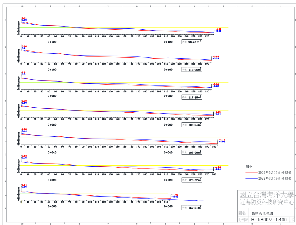
圖 4-5(l) 2022 年 3 月 19 日 B 監測區橫断面比較圖
