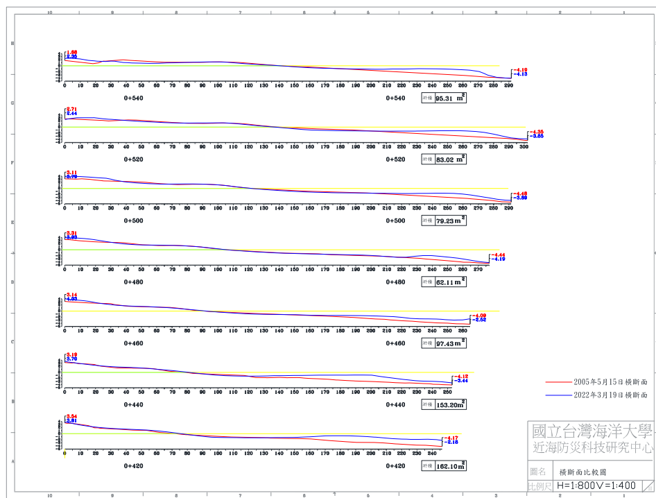
圖 4-5(i) 2022 年 3 月 19 日 B 監測區橫斷面比較圖
