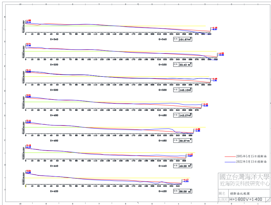
圖 4-5(c) 2022 年 3 月 13 日 B 監測區橫斷面比較圖
