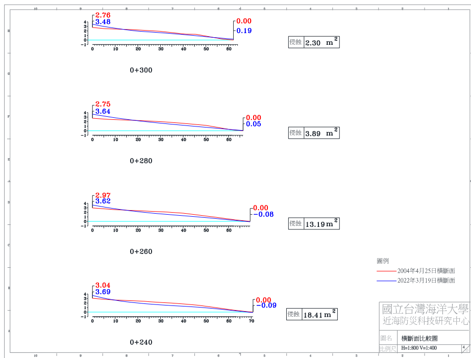
圖 4-4(q) 2022 年 3 月 19 日 A 監測區橫斷面比較圖
