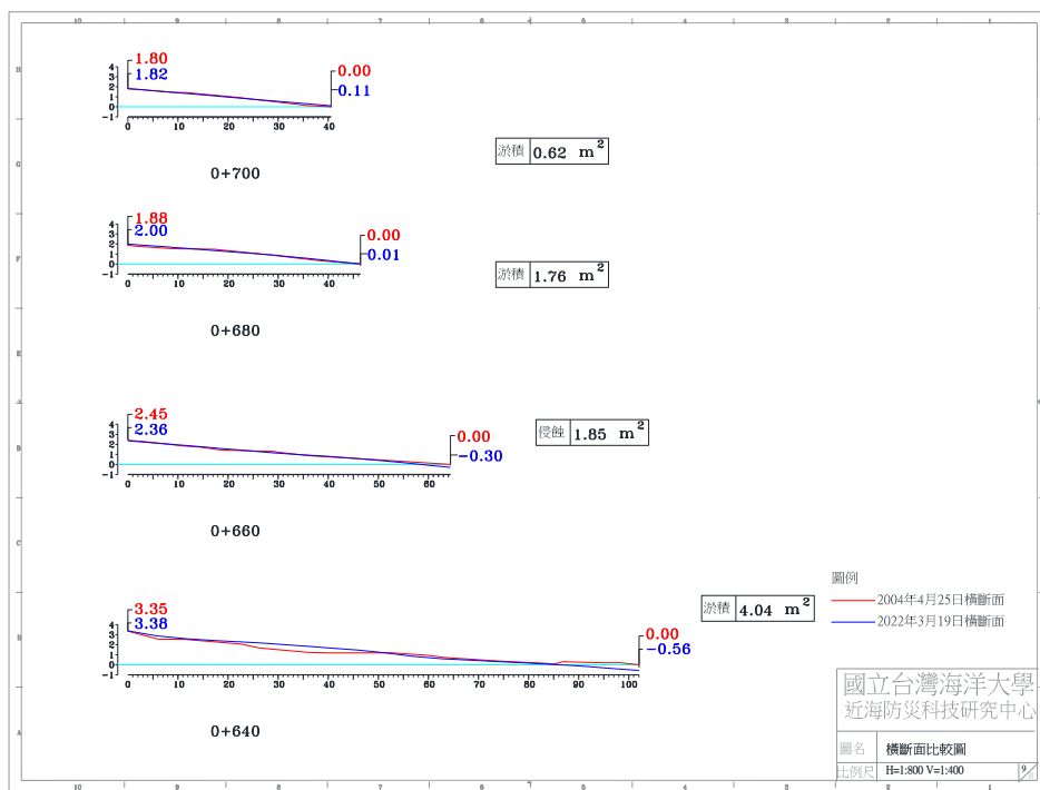
圖 4-4(l) 2022 年 3 月 19 日 A 監測區橫斷面比較圖
