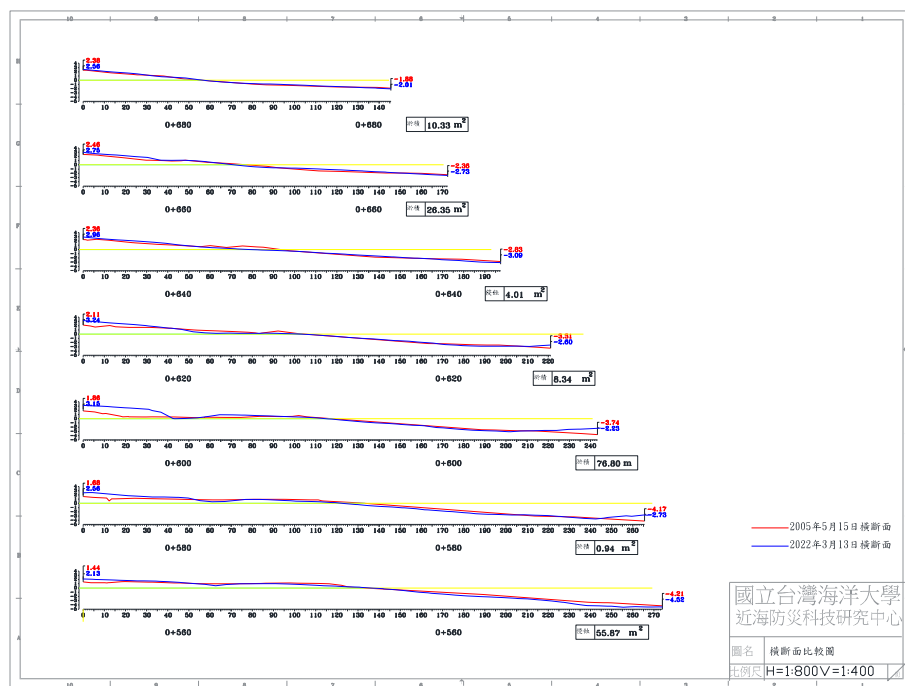
圖 4-5(b) 2022 年 3 月 13 日 B 監測區橫斷面比較圖
