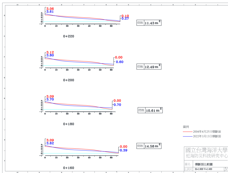
圖 4-4(h) 2022 年 3 月 13 日 A 監測區橫斷面比較圖
