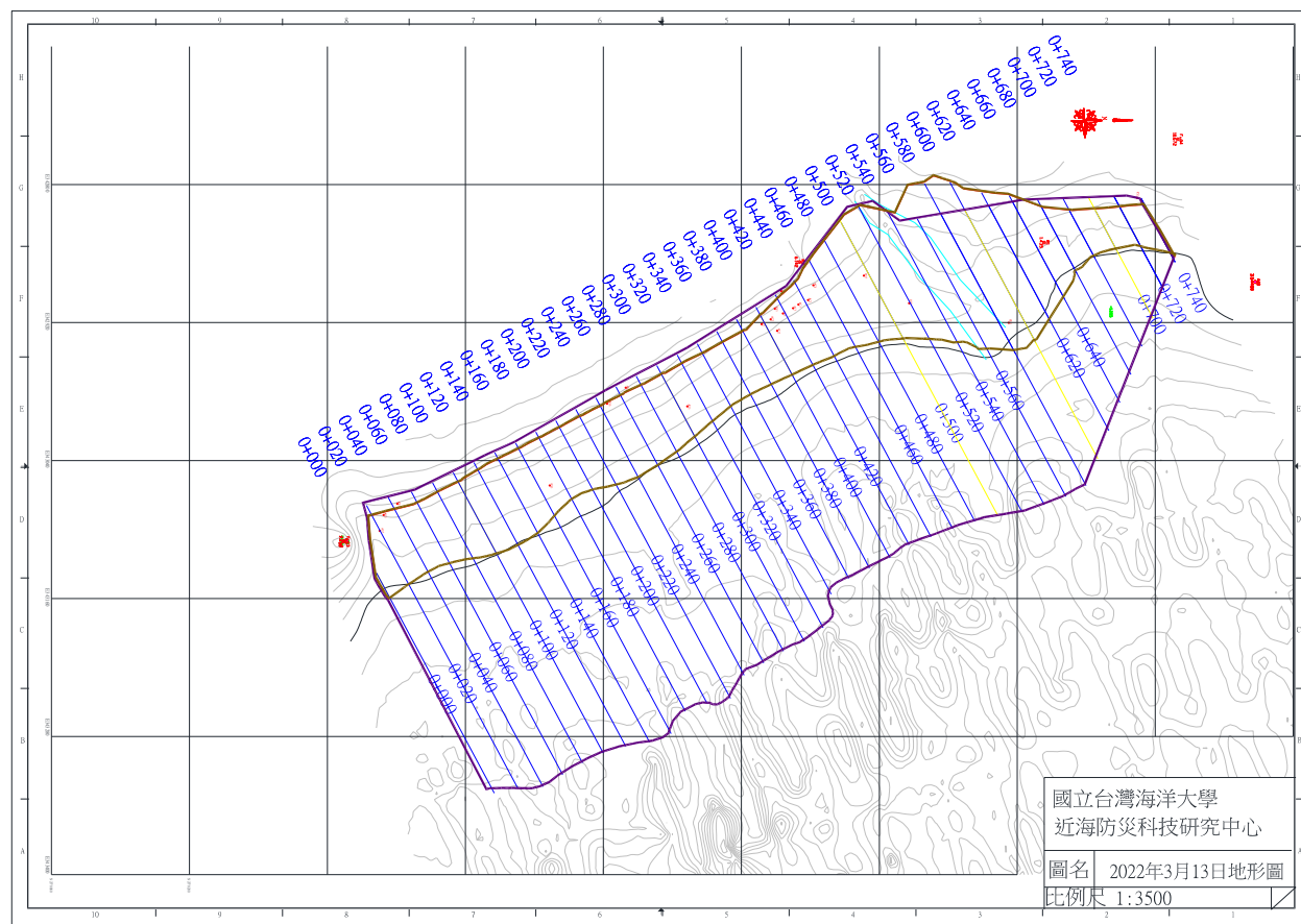
圖 4-1-1 2022 年 3 月 13 日監測地形圖
