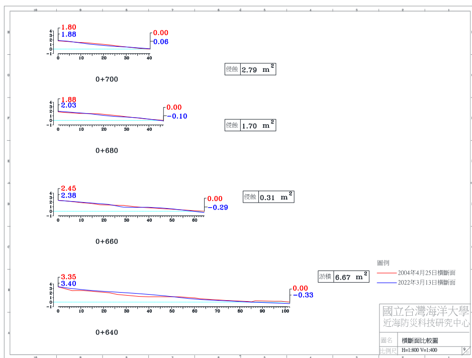
圖 4-4(b) 2022 年 3 月 13 日 A 監測區橫斷面比較圖
