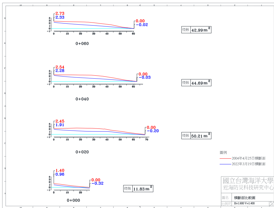
圖 4-4(t) 2022 年 3 月 19 日 A 監測區橫斷面比較圖
