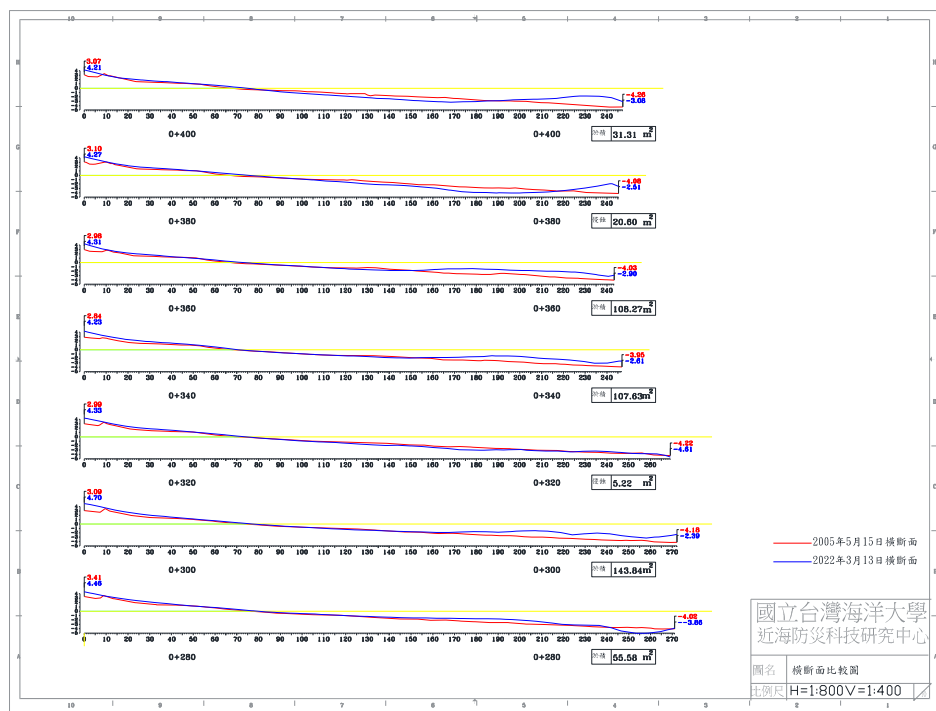
圖 4-5(d) 2022 年 3 月 13 日 B 監測區橫斷面比較圖
