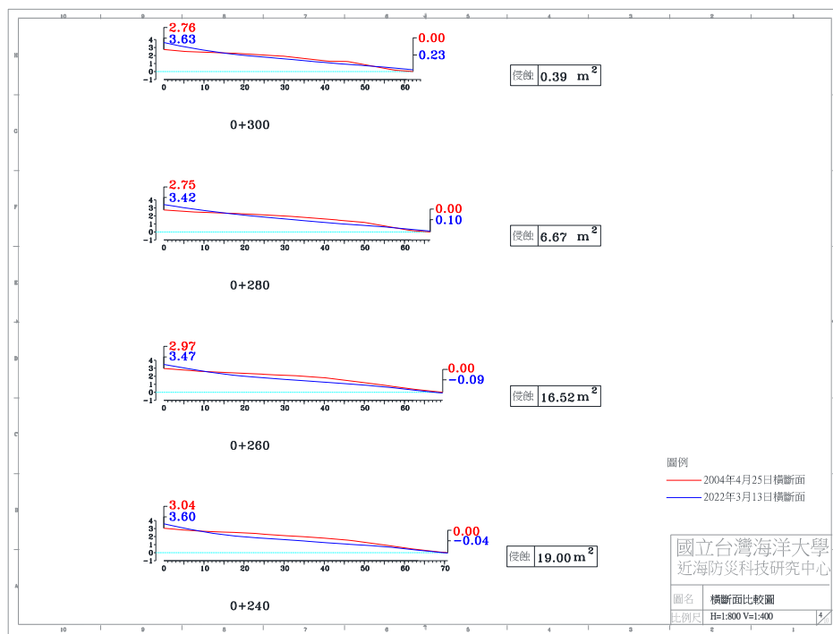
圖 4-4(g) 2022 年 3 月 13 日 A 監測區橫斷面比較圖
