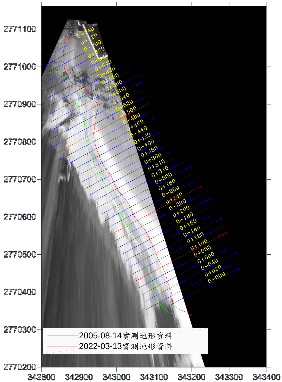
圖 4-22-1 實測地形水位線分析結果圖(2022/03/13)
