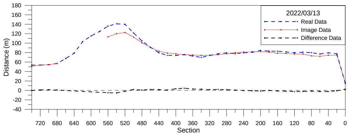
圖 3-23-1 海岸線分析比較圖(2022/03/13)
