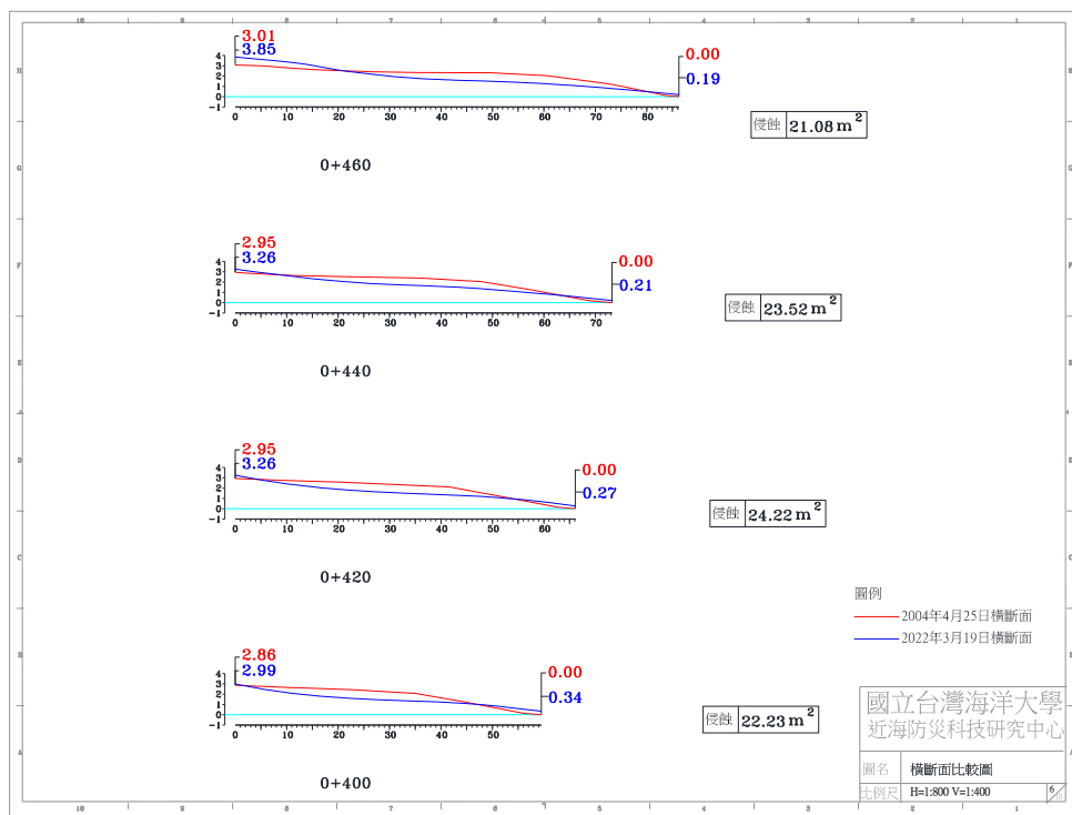
圖 4-4(o) 2022 年 3 月 19 日 A 監測區橫斷面比較圖
