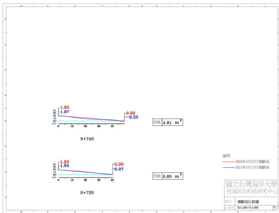
圖 4-4(a) 2022 年 3 月 13 日 A 監測區橫斷面比較圖
