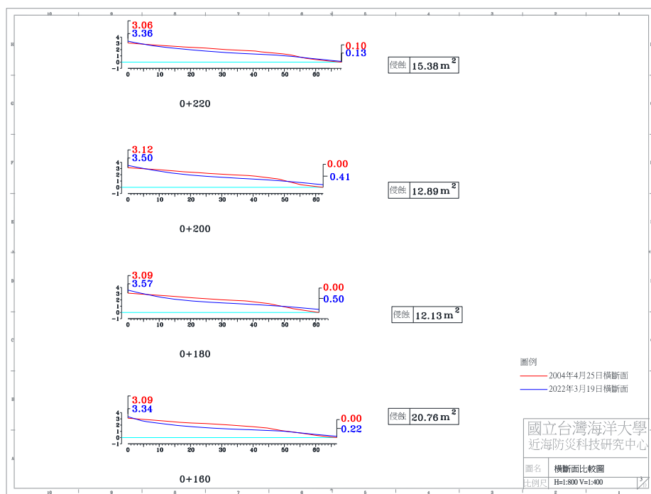
圖 4-4(r) 2022 年 3 月 19 日 A 監測區橫斷面比較圖
