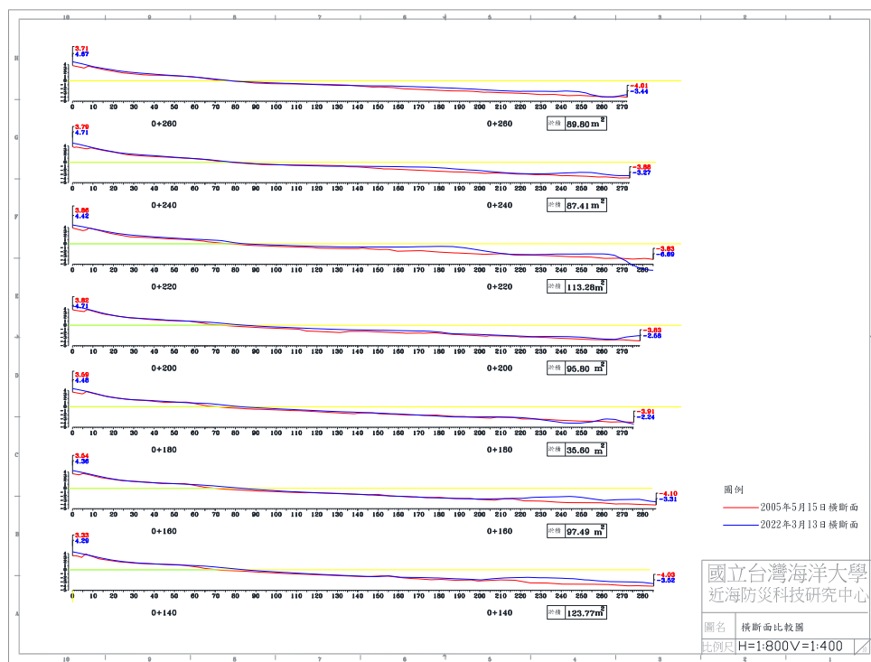
圖 4-5(e) 2022 年 3 月 13 日 B 監測區橫断面比較圖
