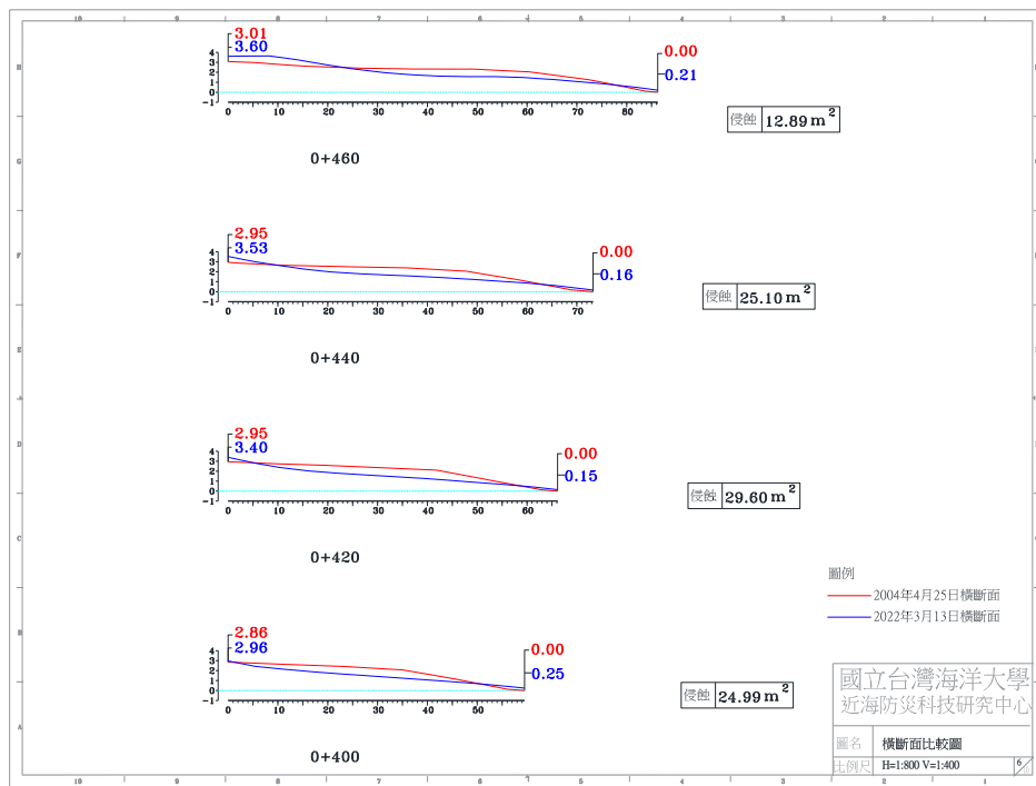
圖 4-4(e) 2022 年 3 月 13 日 A 監測區橫斷面比較圖
