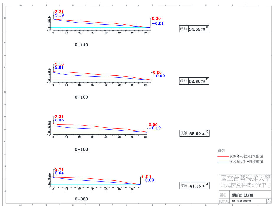
圖 4-4(s) 2022 年 3 月 19 日 A 監測區橫斷面比較圖
