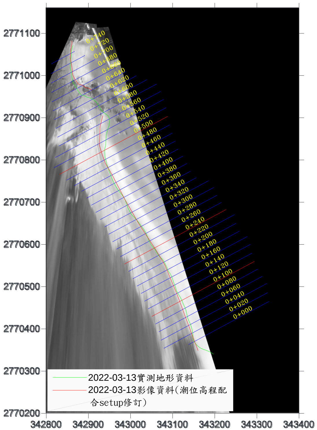
圖 3-22-1 水位線分析結果圖(2022/03/13)
