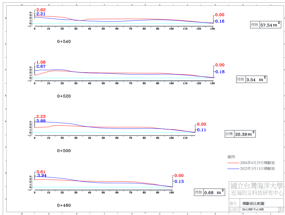
圖 4-4(d) 2022 年 3 月 13 日 A 監測區橫斷面比較圖
