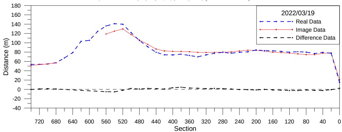
圖 3-23-2 海岸線分析比較圖(2022/03/19)
