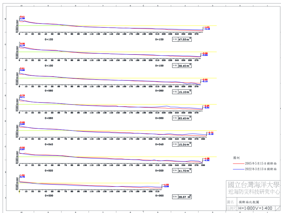
圖 4-5(f) 2022 年 3 月 13 日 B 監測區橫断面比較圖
