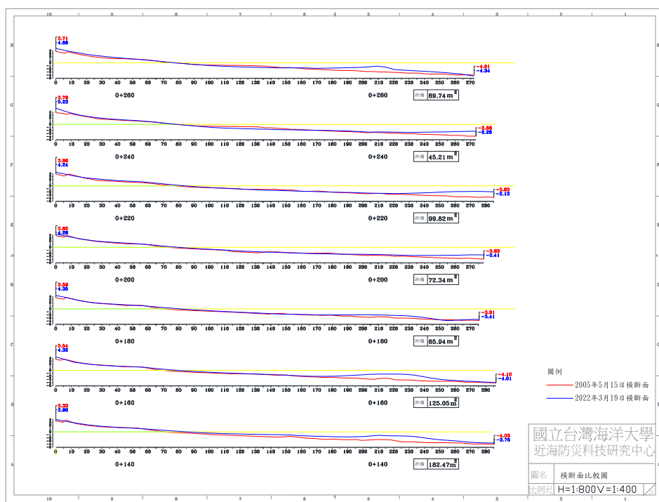
圖 4-5(k) 2022 年 3 月 19 日 B 監測區橫断面比較圖
