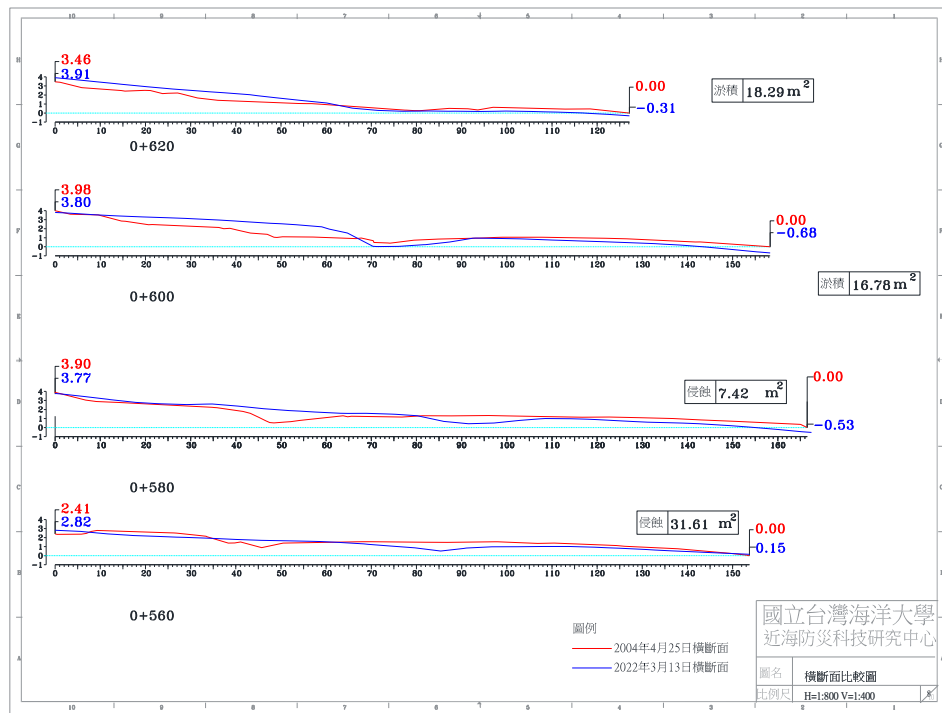
圖 4-4(c) 2022 年 3 月 13 日 A 監測區橫斷面比較圖
