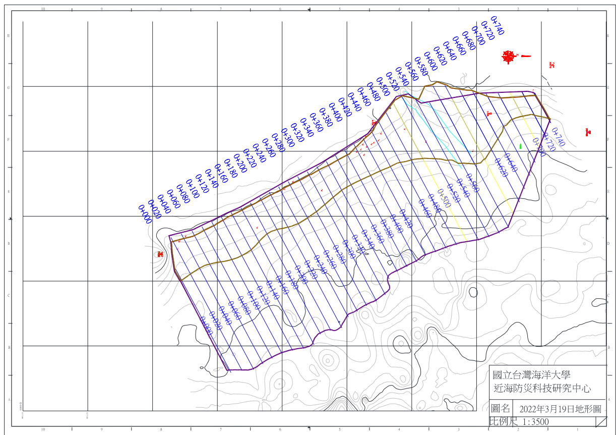
圖 4-1-2 2022 年 3 月 19 日監測地形圖
