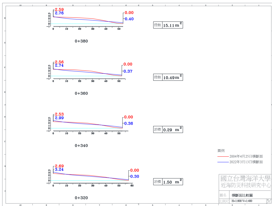
圖 4-4(f) 2022 年 3 月 13 日 A 監測區橫斷面比較圖
