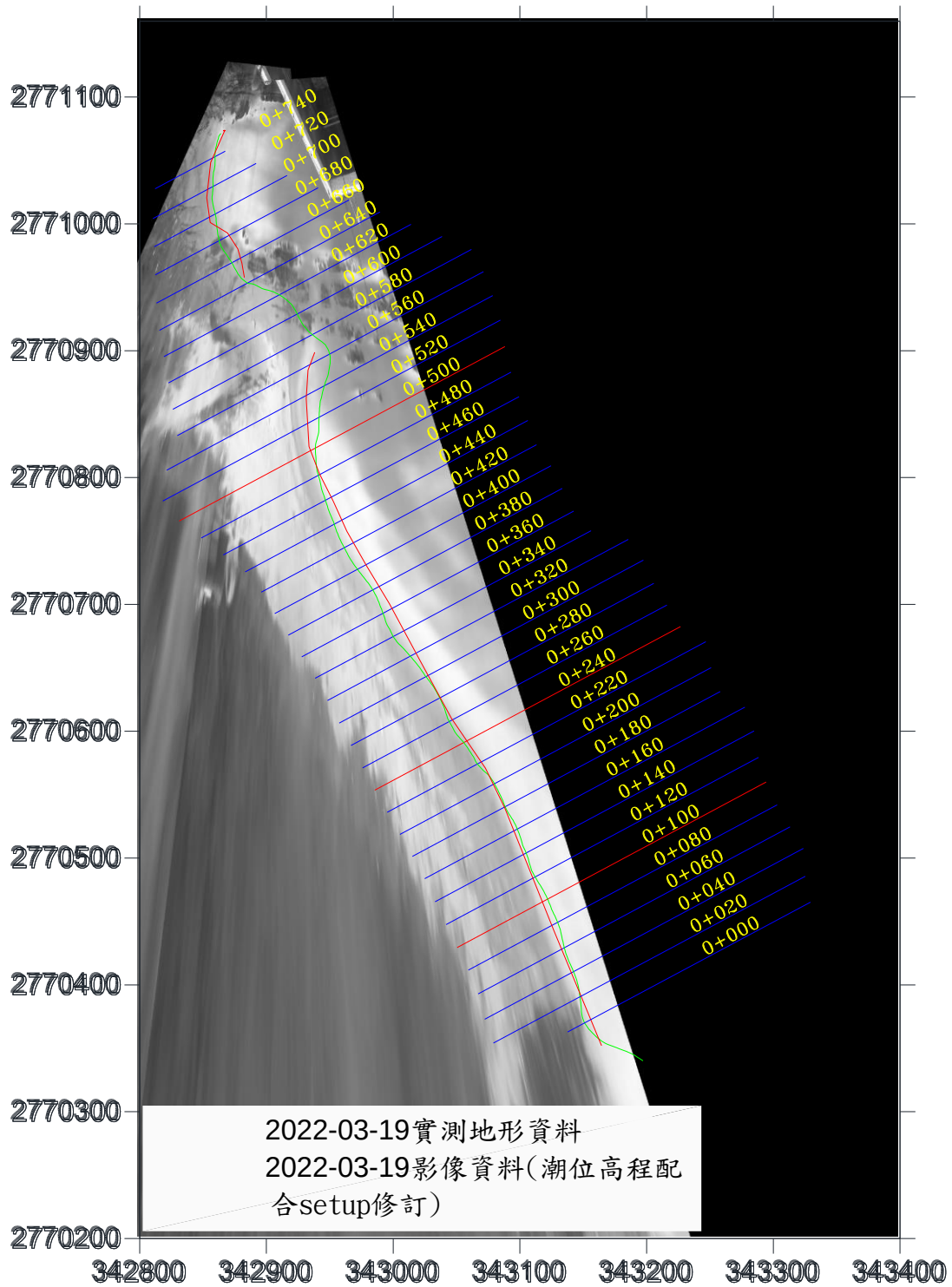
圖 3-22-2 水位線分析結果圖(2022/03/19)
