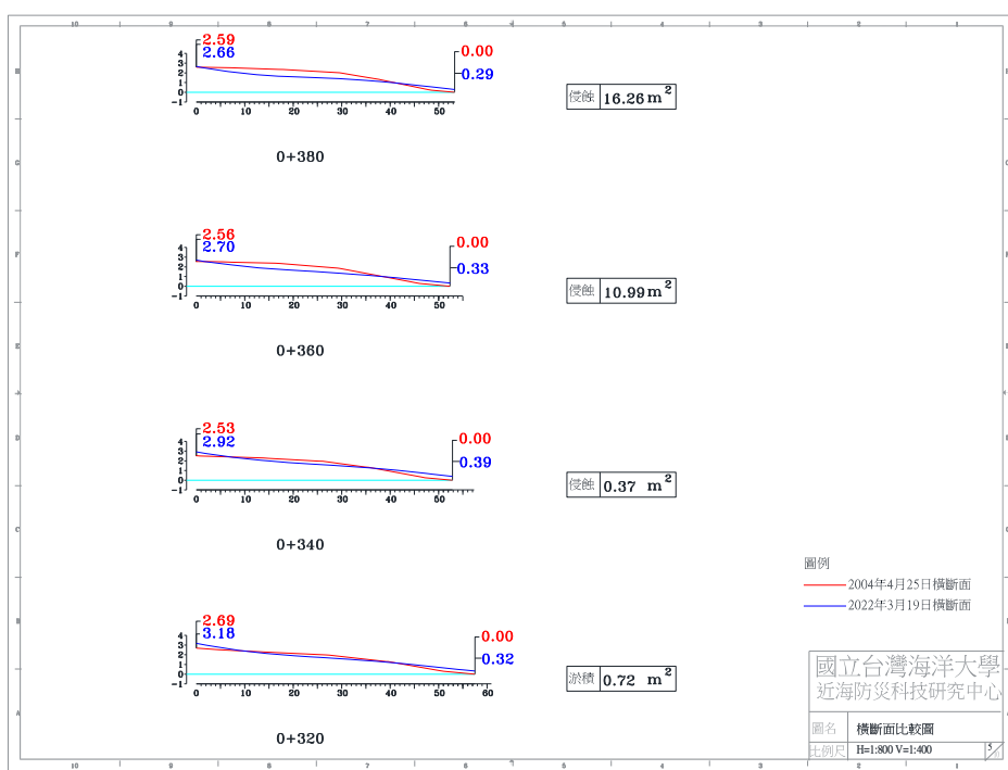
圖 4-4(p) 2022 年 3 月 19 日 A 監測區橫斷面比較圖
