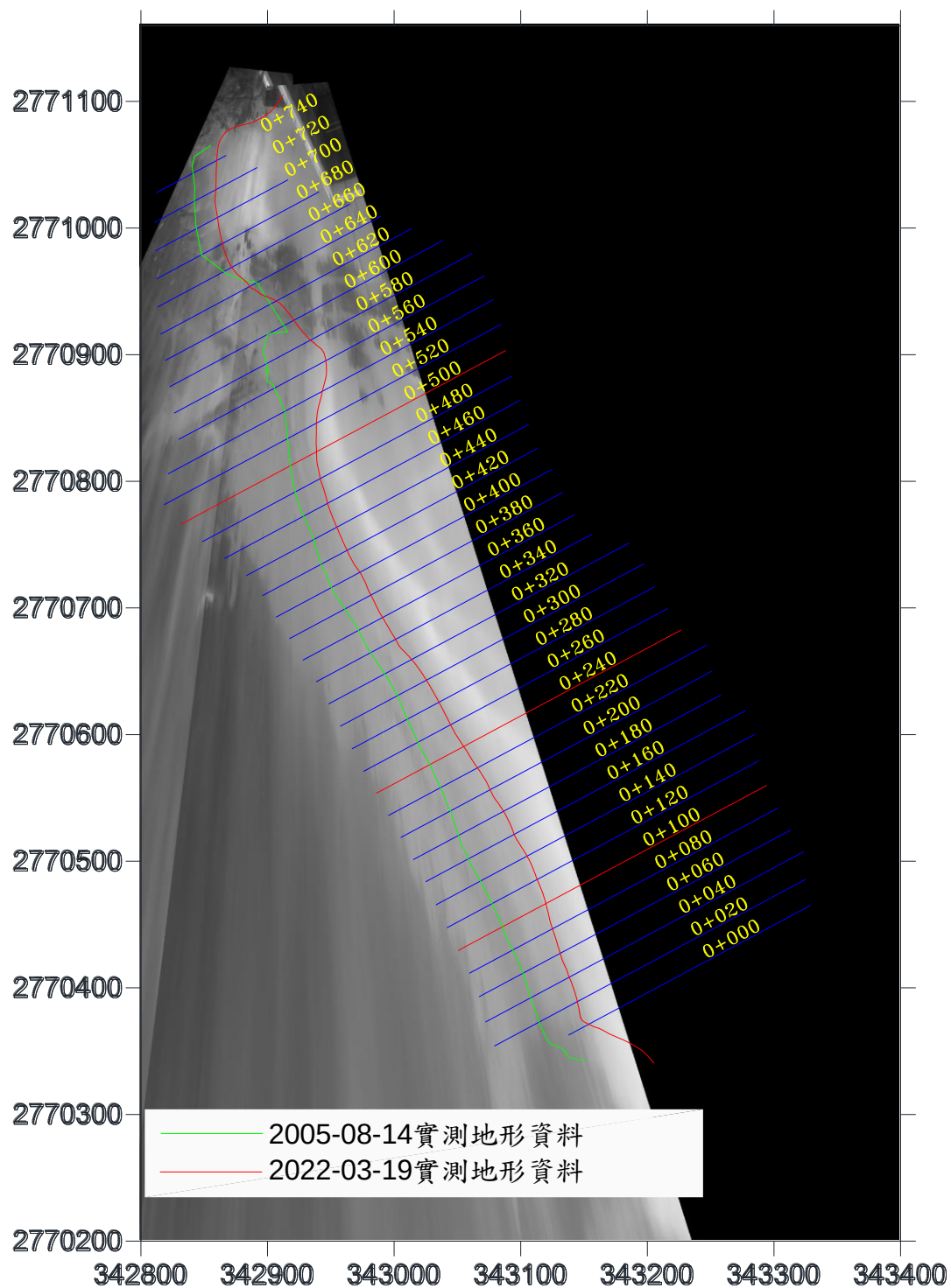
圖 4-22-2 實測地形水位線分析結果圖(2022/03/19)
