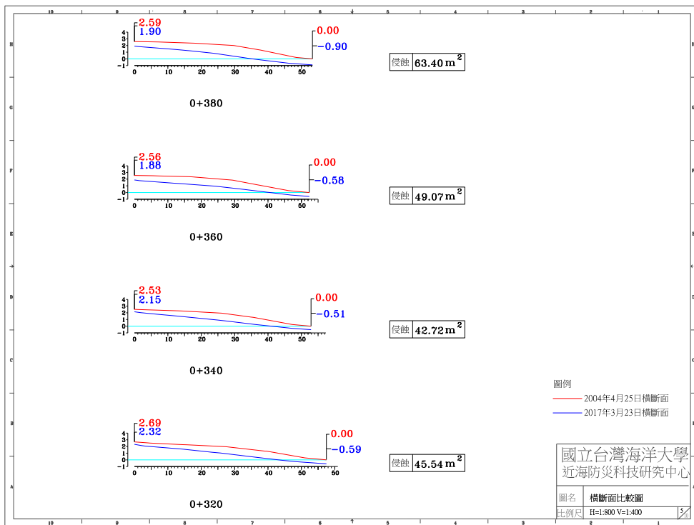
圖 4-4(f) 2017 年 3 月 23 日 A 監測區橫斷面比較圖
