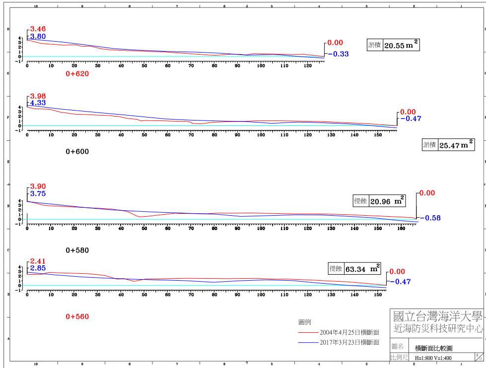
圖 4-4(c) 2017 年 3 月 23 日 A 監測區橫斷面比較圖
