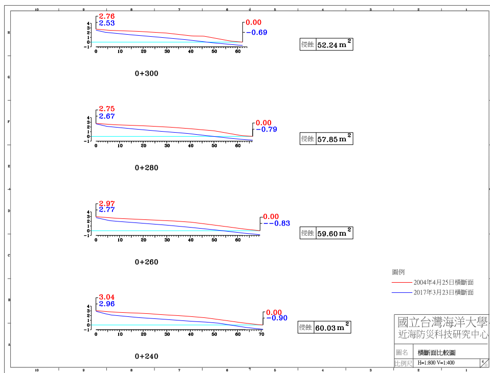
圖 4-4(g) 2017 年 3 月 23 日 A 監測區橫斷面比較圖
