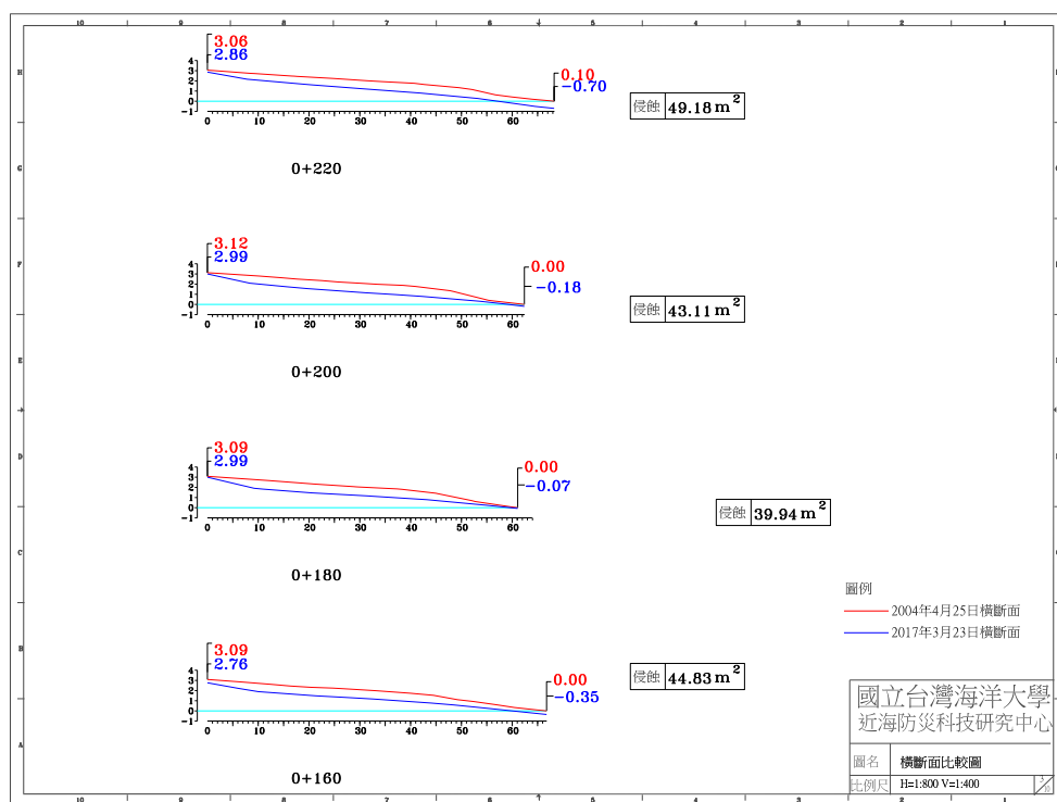
圖 4-4(h) 2017 年 3 月 23 日 A 監測區橫斷面比較圖
