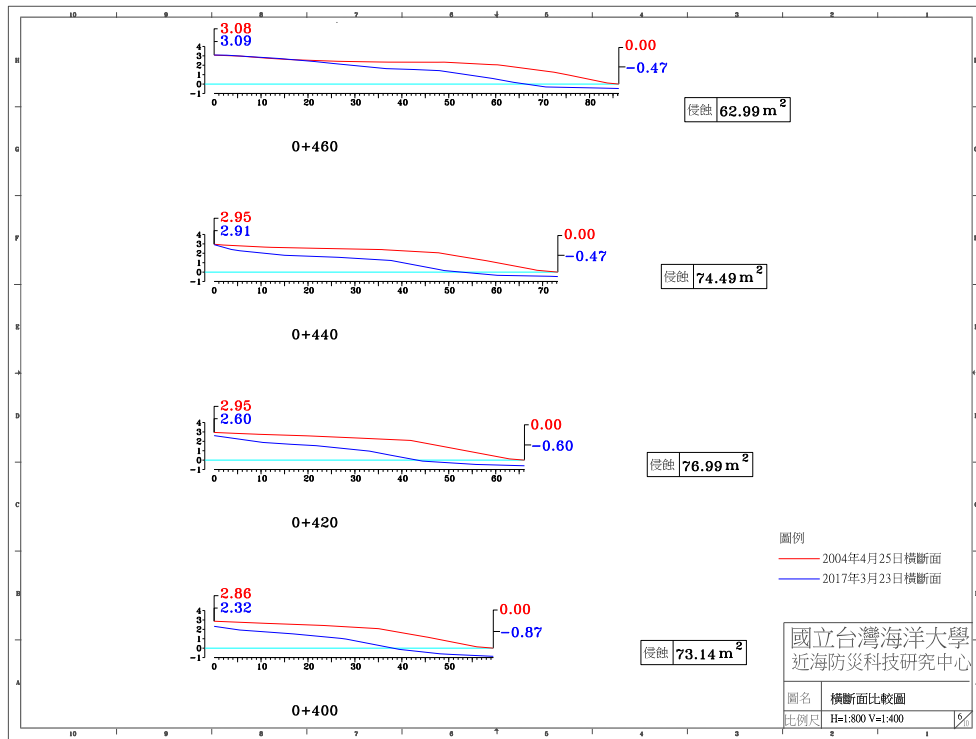
圖 4-4(e) 2017 年 3 月 23 日 A 監測區橫斷面比較圖
