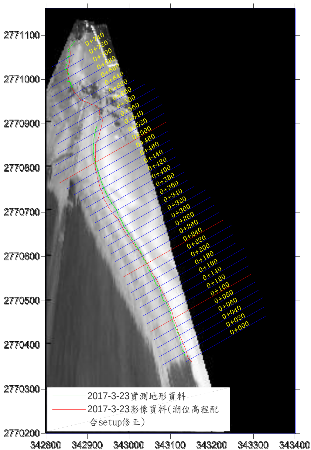
圖 3-22 水位線分析結果圖(2017/3/23)
