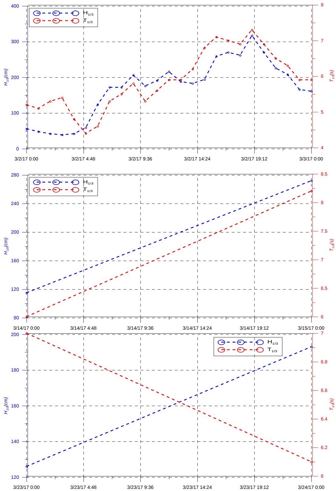
圖 2-3 波浪時序列變化圖
