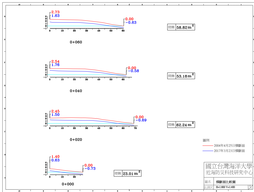
圖 4-4(j) 2017 年 3 月 23 日 A 監測區橫斷面比較圖
