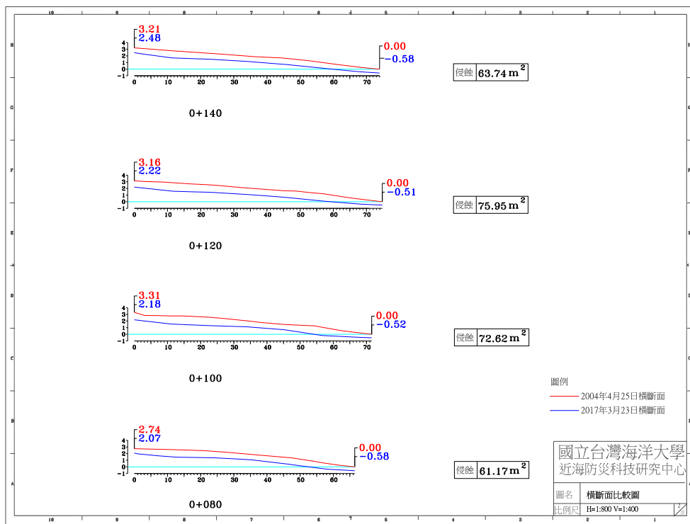
圖 4-4(i) 2017 年 3 月 23 日 A 監測區橫斷面比較圖
