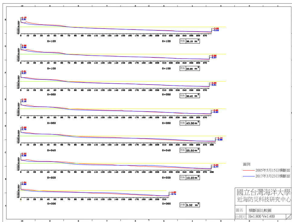
圖 4-5(f) 2017 年 3 月 23 日 B 監測區橫斷面比較圖
