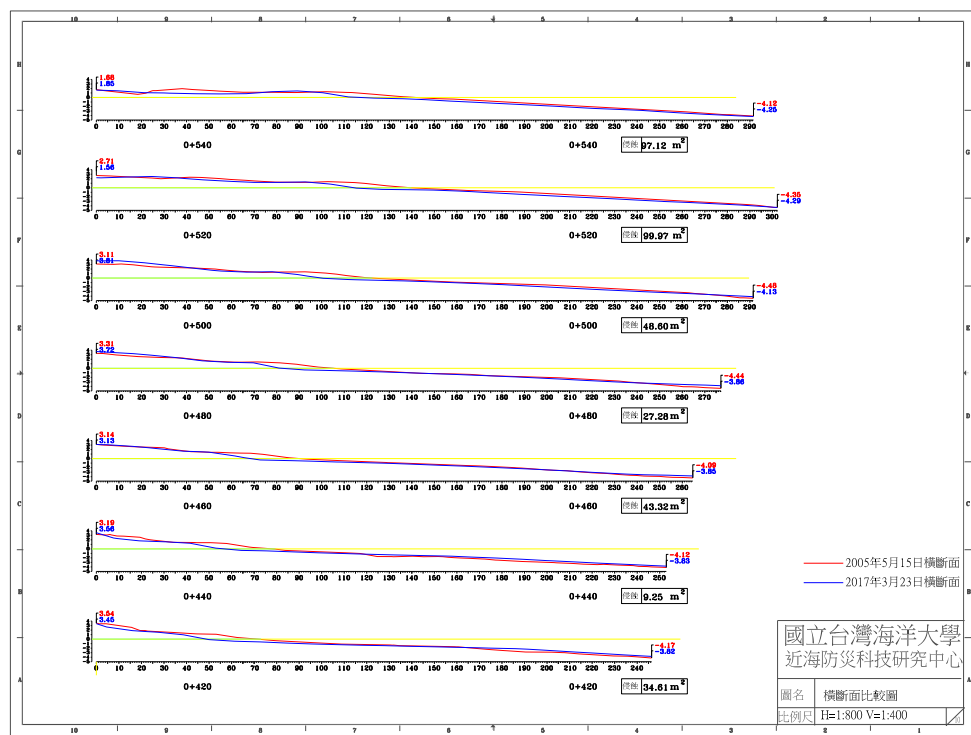
圖 4-5(c) 2017 年 3 月 23 日 B 監測區橫斷面比較圖
