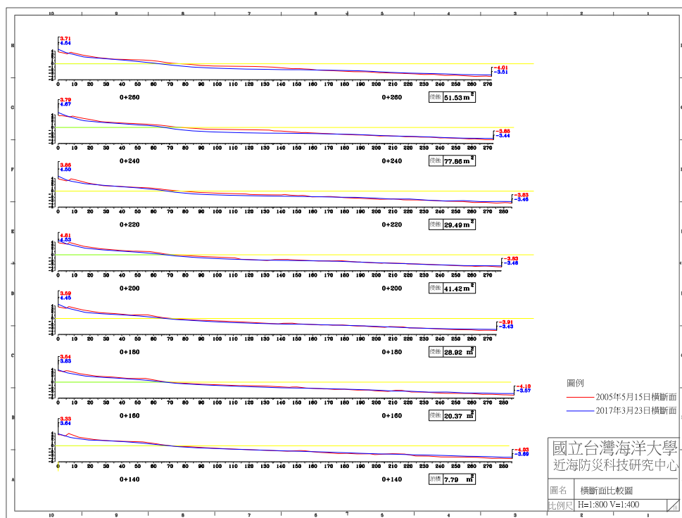
圖 4-5(e) 2017 年 3 月 23 日 B 監測區橫斷面比較圖
