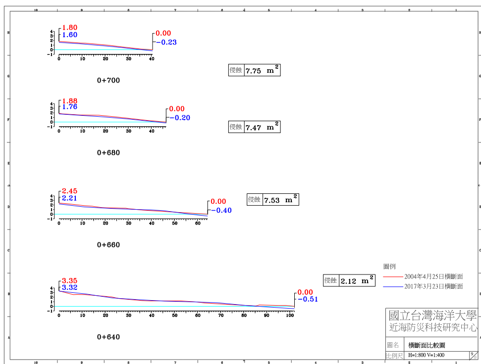
圖 4-4(b) 2017 年 3 月 23 日 A 監測區橫斷面比較圖
