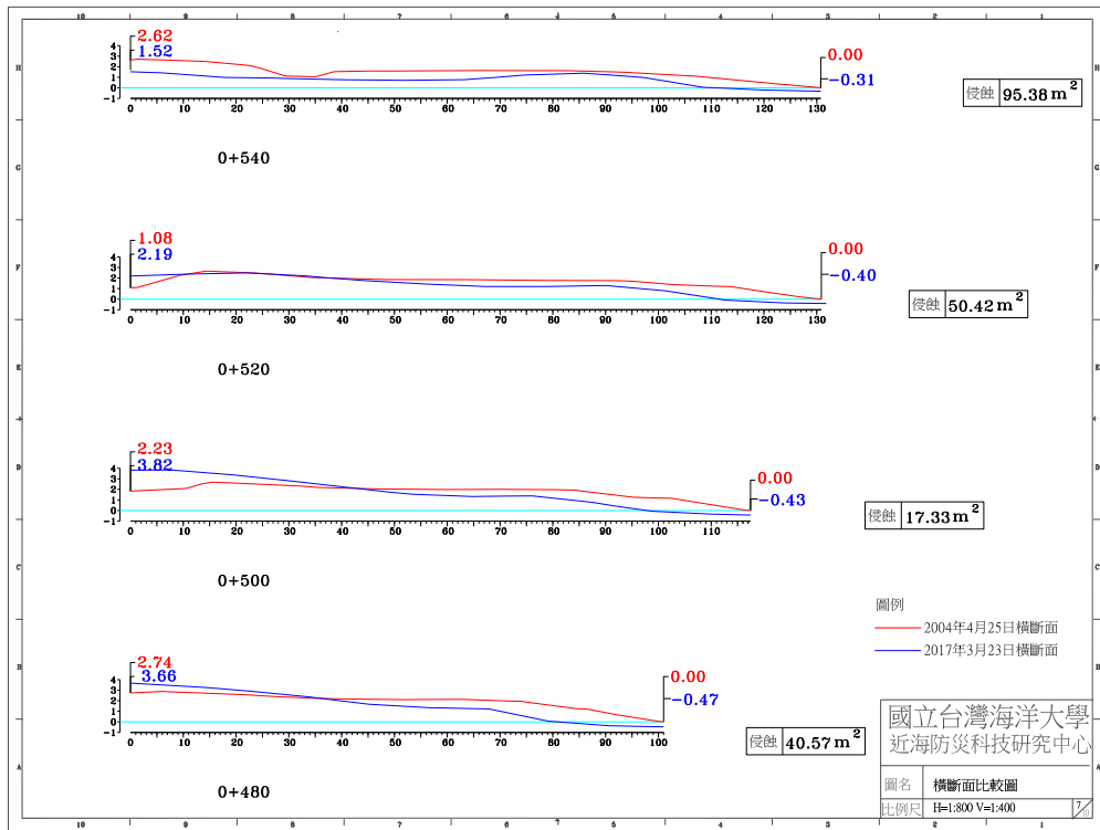
圖 4-4(d) 2017 年 3 月 23 日 A 監測區橫斷面比較圖
