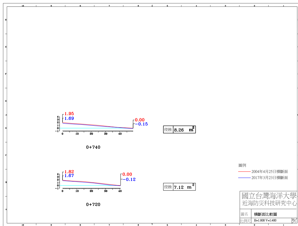
圖 4-4(a) 2017 年 3 月 23 日 A 監測區橫斷面比較圖
