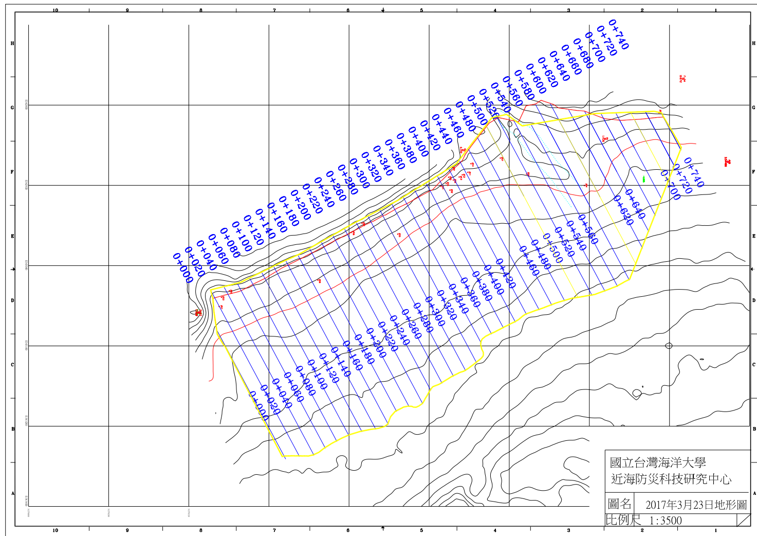
圖 4-1 2017 年 3 月 23 日監測地形圖
